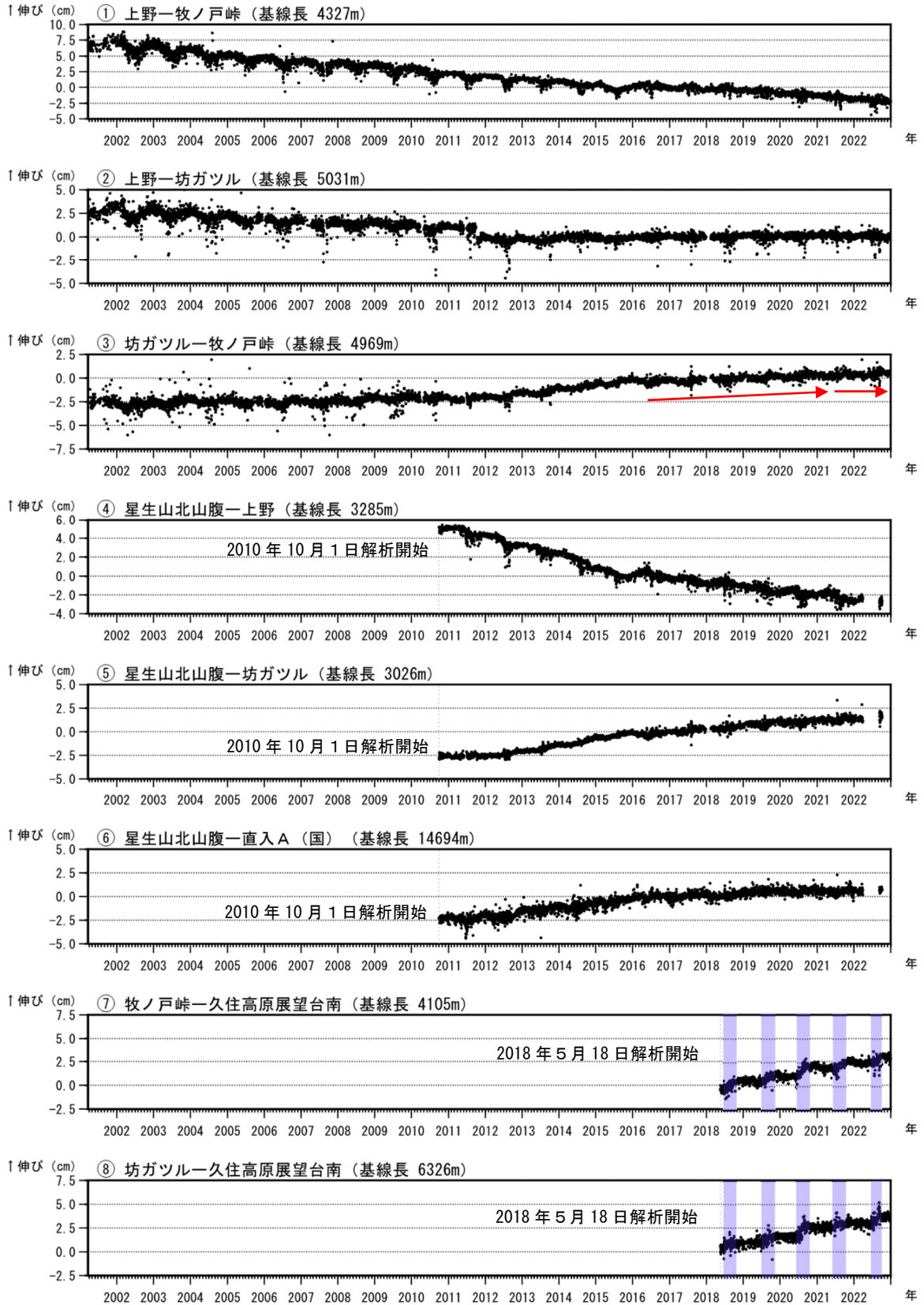
図5 九重山 GNSS連続観測による基線長変化（2001年4月～2022年12月）
