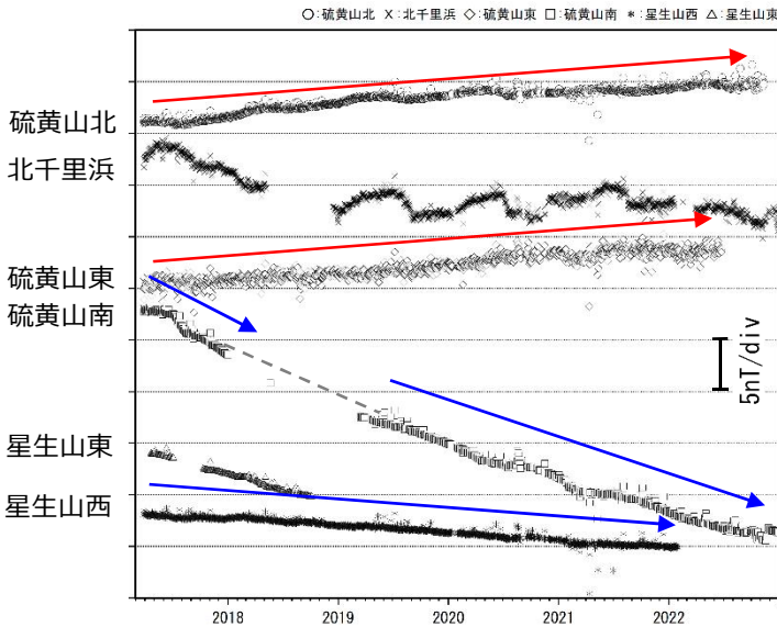
図 4-1 九重山 連続観測による全磁力の変化 (2017年3月～2022年12月30日)
