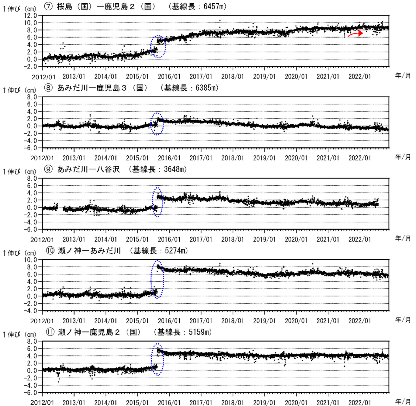
図 7-2 桜島 GNSS 連続観測による基線長変化 (2012 年 1 月～2022 年 11 月)
