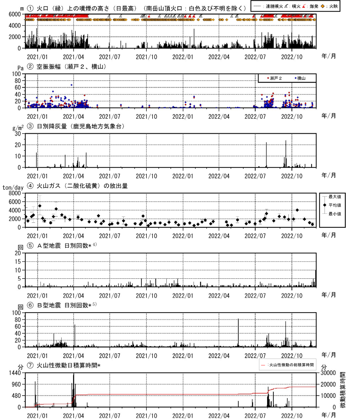
図5 桜島 最近2年間の活動経過図（2020年12月～2022年11月）
