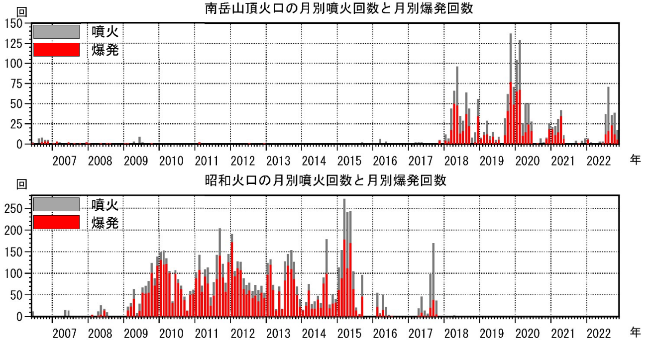
図3 桜島 南岳山頂火口（上図）と昭和火口（下図）の月別噴火回数と月別爆発回数 （2006年6月～2022年11月）
