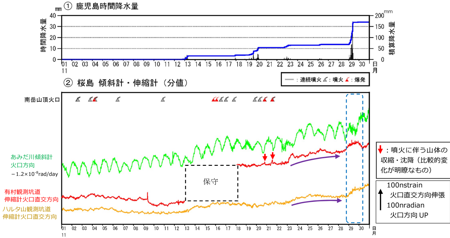
図6 桜島 傾斜計及び伸縮計による地殻変動の状況（2022年11月）
