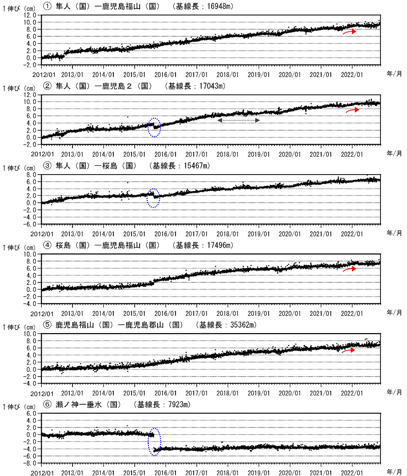
図 7-1 桜島 GNSS 連続観測による基線長変化（2012 年 1 月～2022 年 11 月）
