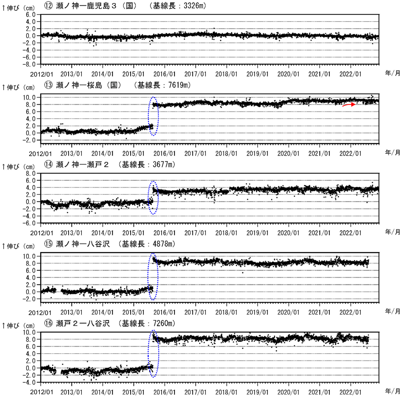
図 7-3 桜島 GNSS 連続観測による基線長変化 (2012 年 1 月～2022 年 11 月)
