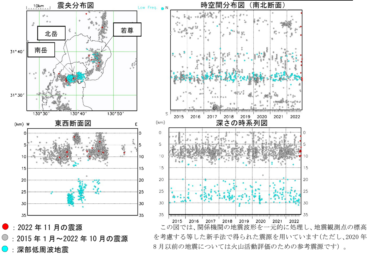
図 2-1 桜島 始良カルデラ周辺の震源分布図（2015年1月～2022年11月）
