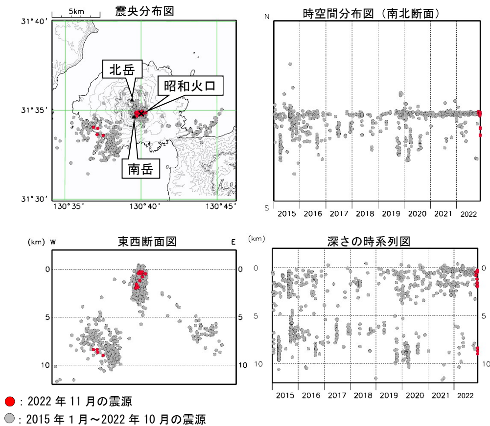
図 2-2 桜島 桜島付近の震源分布図（2015年1月～2022年11月）
