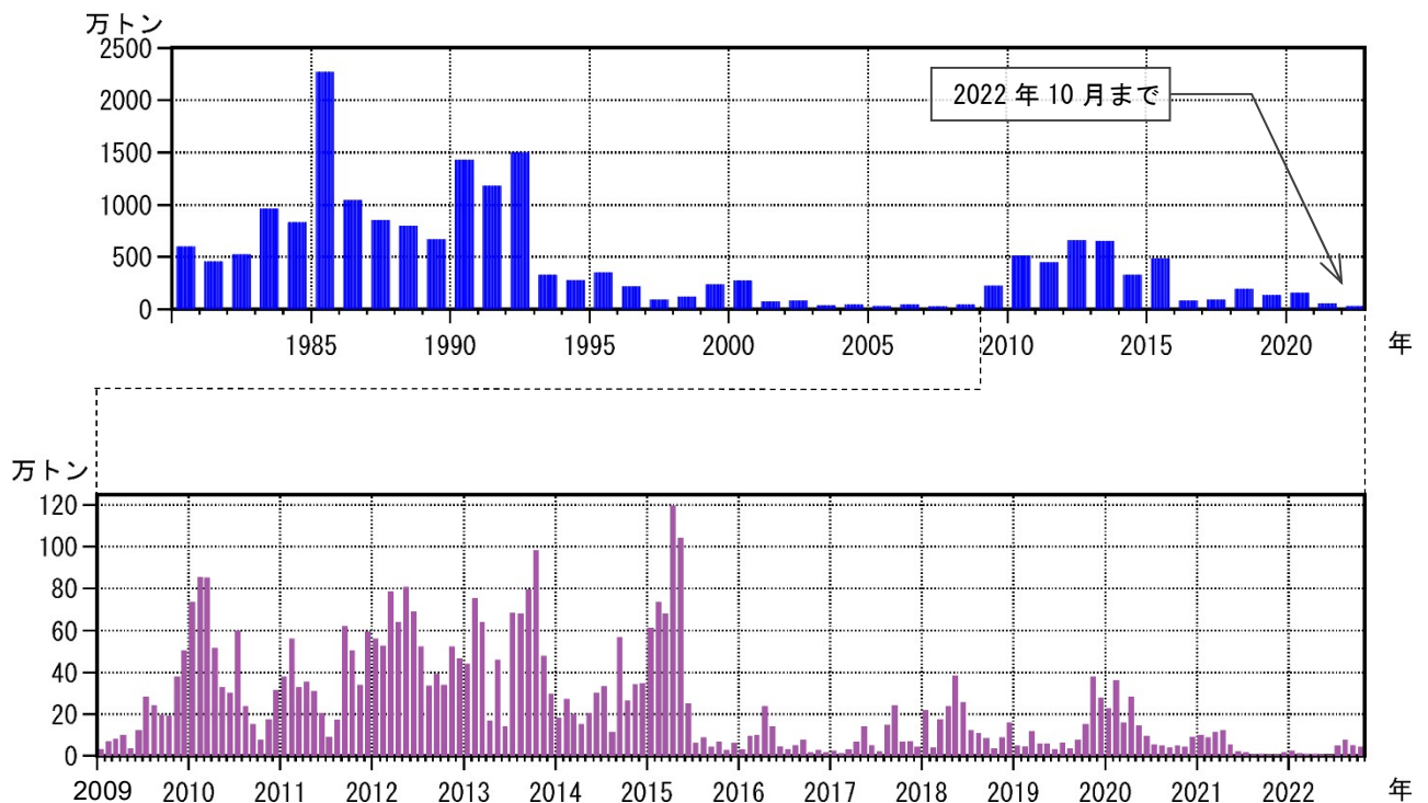
図4 桜島 鹿児島県が実施している降灰の観測データから推定した火山灰の総噴出量 （上段：1980年1月～2022年10月の年別値、下段：2009年1月～2022年10月の月別値）
