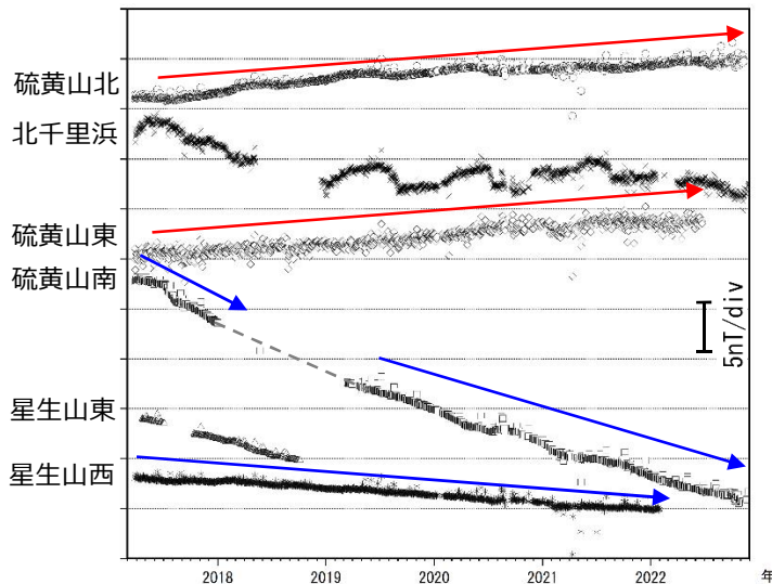
図 4-1 九重山 連続観測による全磁力の変化 (2017年3月～2022年11月)
