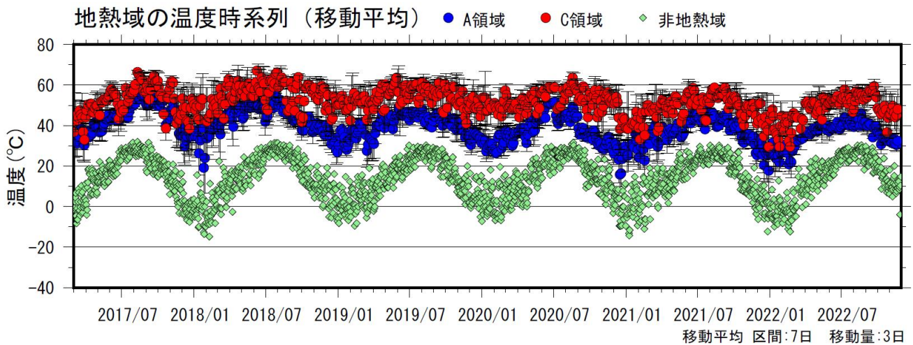
図 1-2 九重山 星生山北尾根の赤外熱映像装置による日別最高温度（2017年3月～2022年11月）
