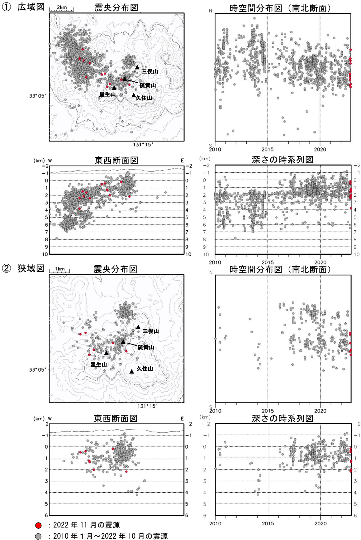
図3 九重山 震源分布図 ①広域図②狭域図（2010年1月～2022年11月）
