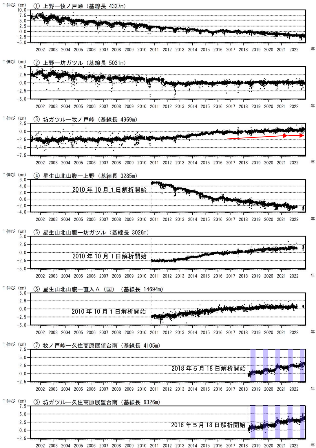
図5 九重山 GNSS 連続観測による基線長変化（2001年4月～2022年11月）
