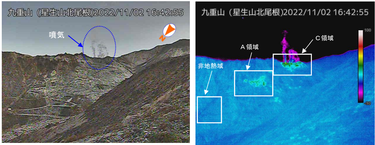
図 1-1 九重山 硫黄山の噴気及び地熱域の状況（11月2日 星生山北尾根監視カメラ）
