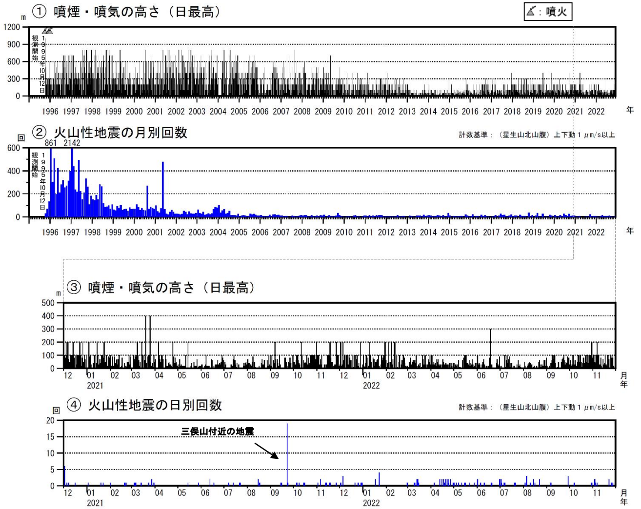
図2 九重山 火山活動経過図（1995年1月～2022年11月）
