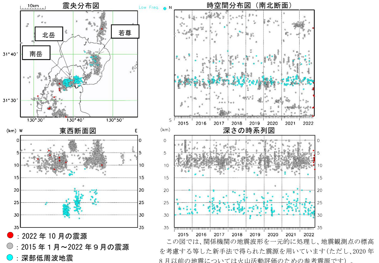
図 5-1 桜島 始良カルデラ周辺の震源分布図（2015年1月～2022年10月）
