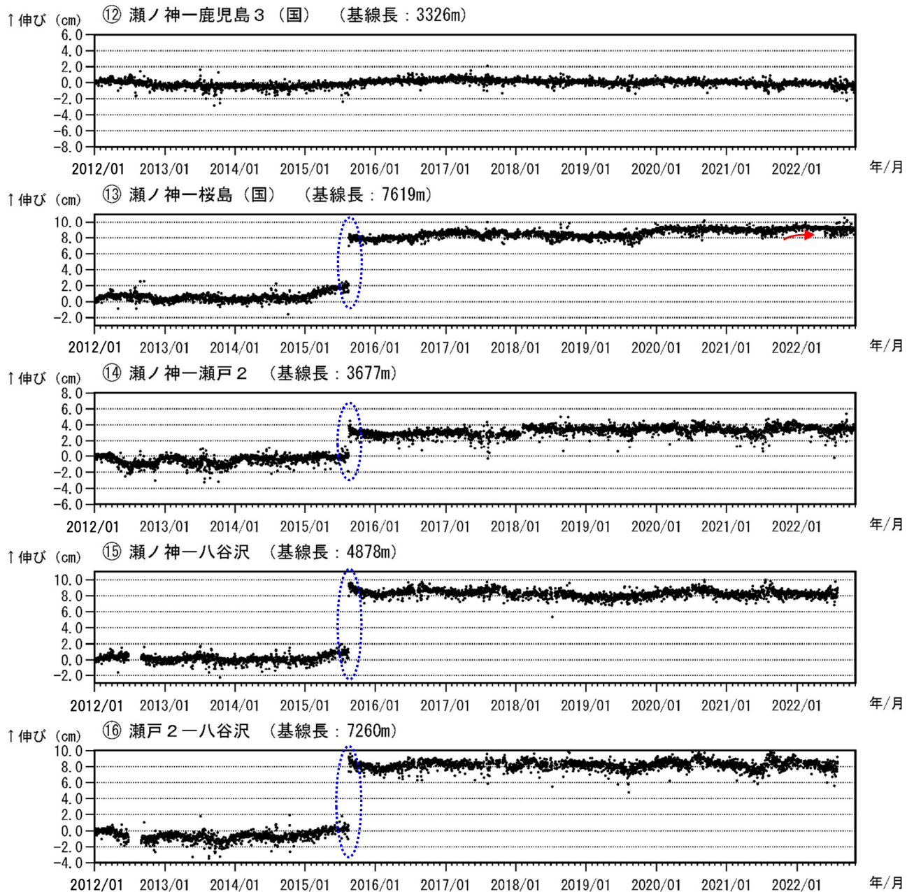
図 10-3 桜島 GNSS 連続観測による基線長変化（2012 年 1 月～2022 年 10 月）
