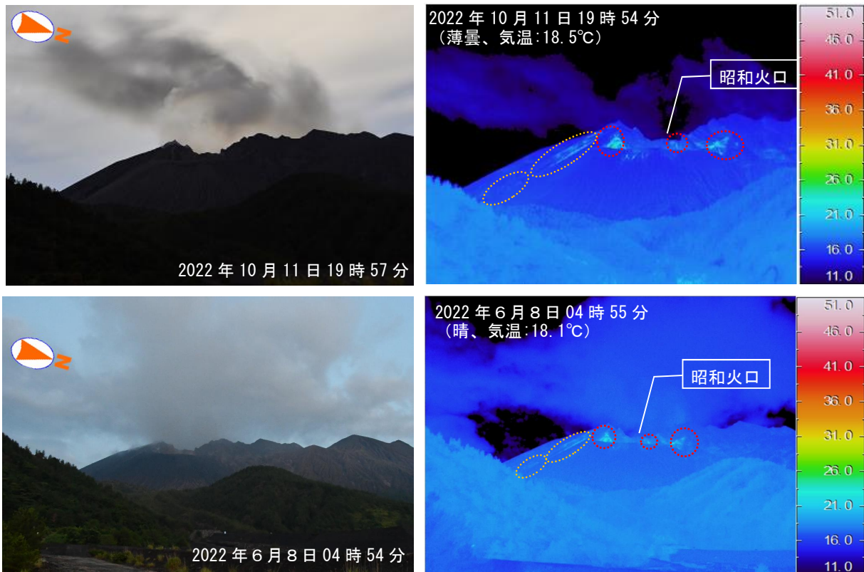
図 4-1 桜島 昭和火口周辺の状況（黒神町（黒神河原）から観測）
