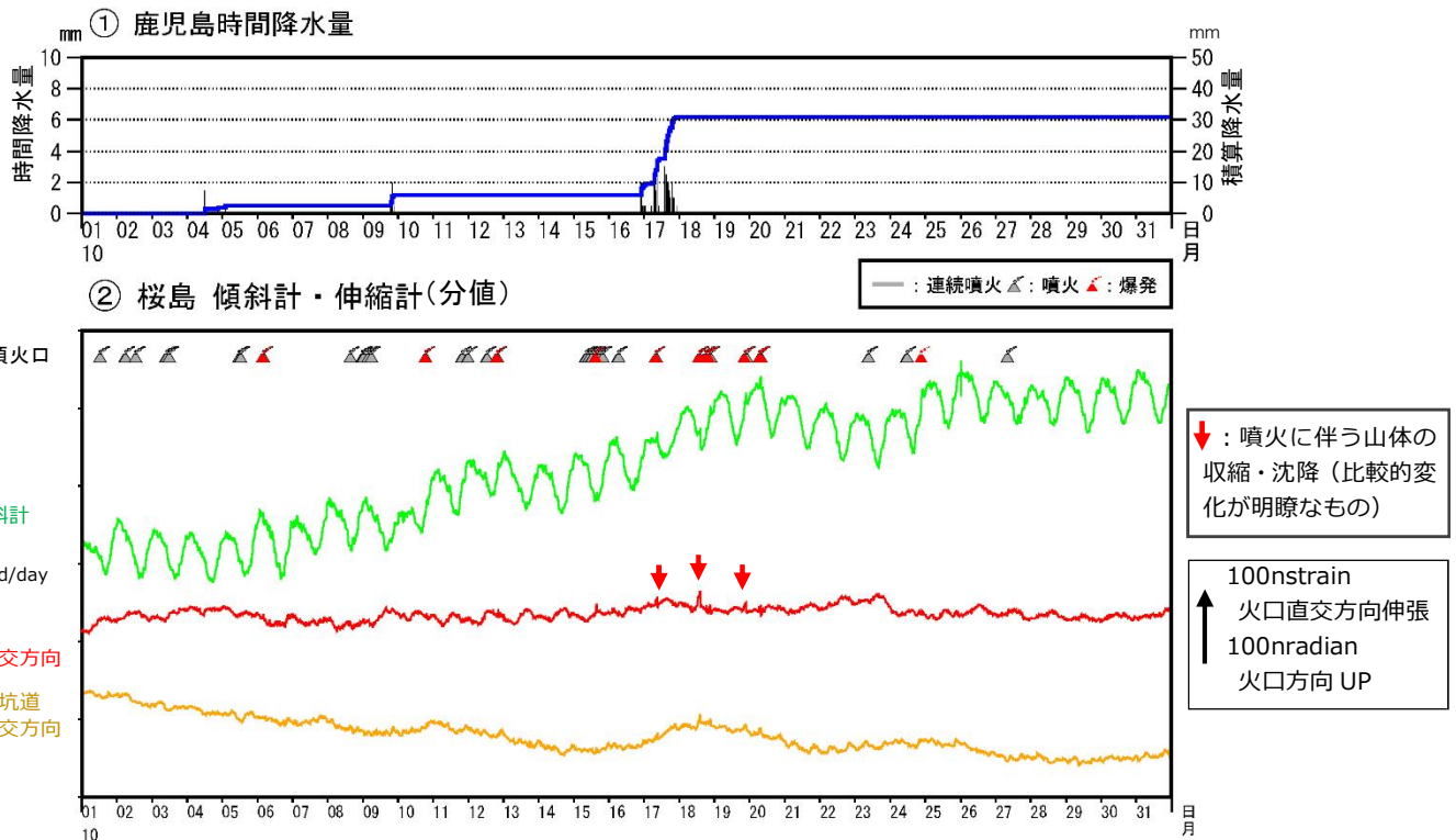
図9 桜島 傾斜計及び伸縮計による地殻変動の状況（2022年10月）
