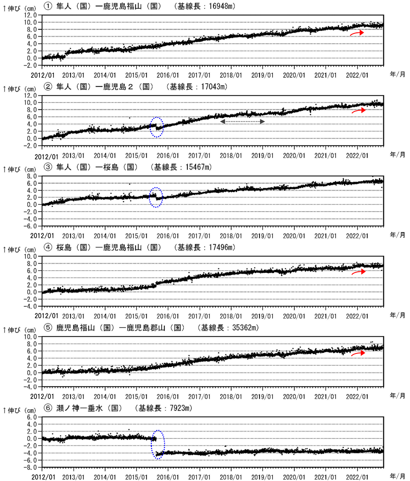
図 10-1 桜島 GNSS 連続観測による基線長変化（2012年1月～2022年10月）
