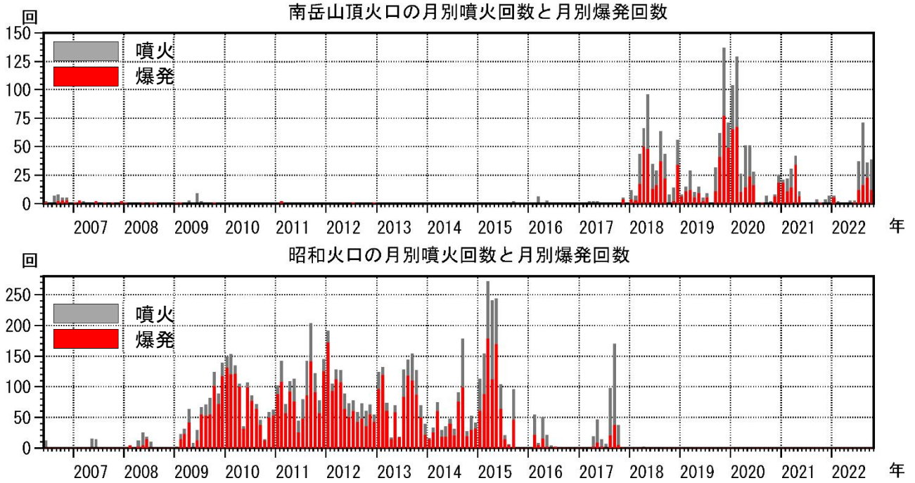
図6 桜島 南岳山頂火口（上図）と昭和火口（下図）の月別噴火回数と月別爆発回数 （2006年6月～2022年10月）
