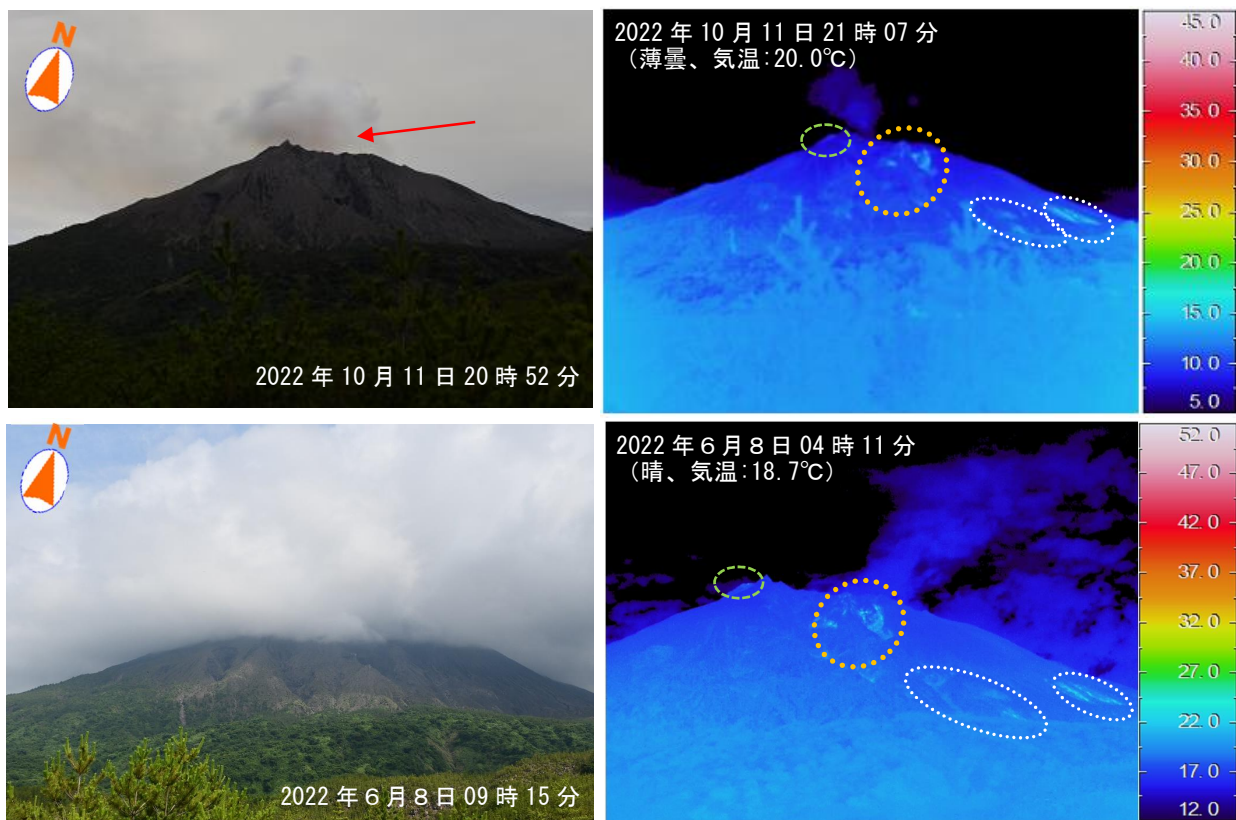
図 4-2 桜島 南岳山頂及び南側山腹付近の状況（有村町（有村溶岩展望所）から観測）
