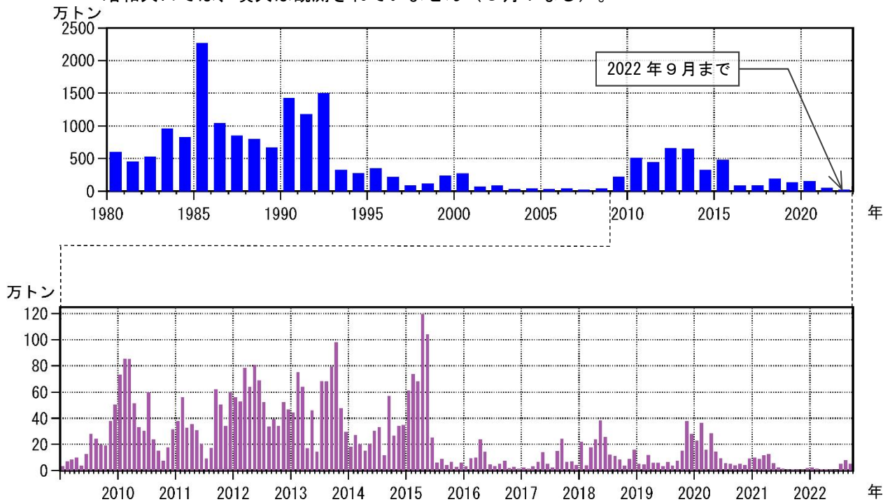
図7 桜島 鹿児島県が実施している降灰の観測データから推定した火山灰の総噴出量 （上段：1980年1月～2022年9月の年別値、下段：2009年1月～2022年9月の月別値）
