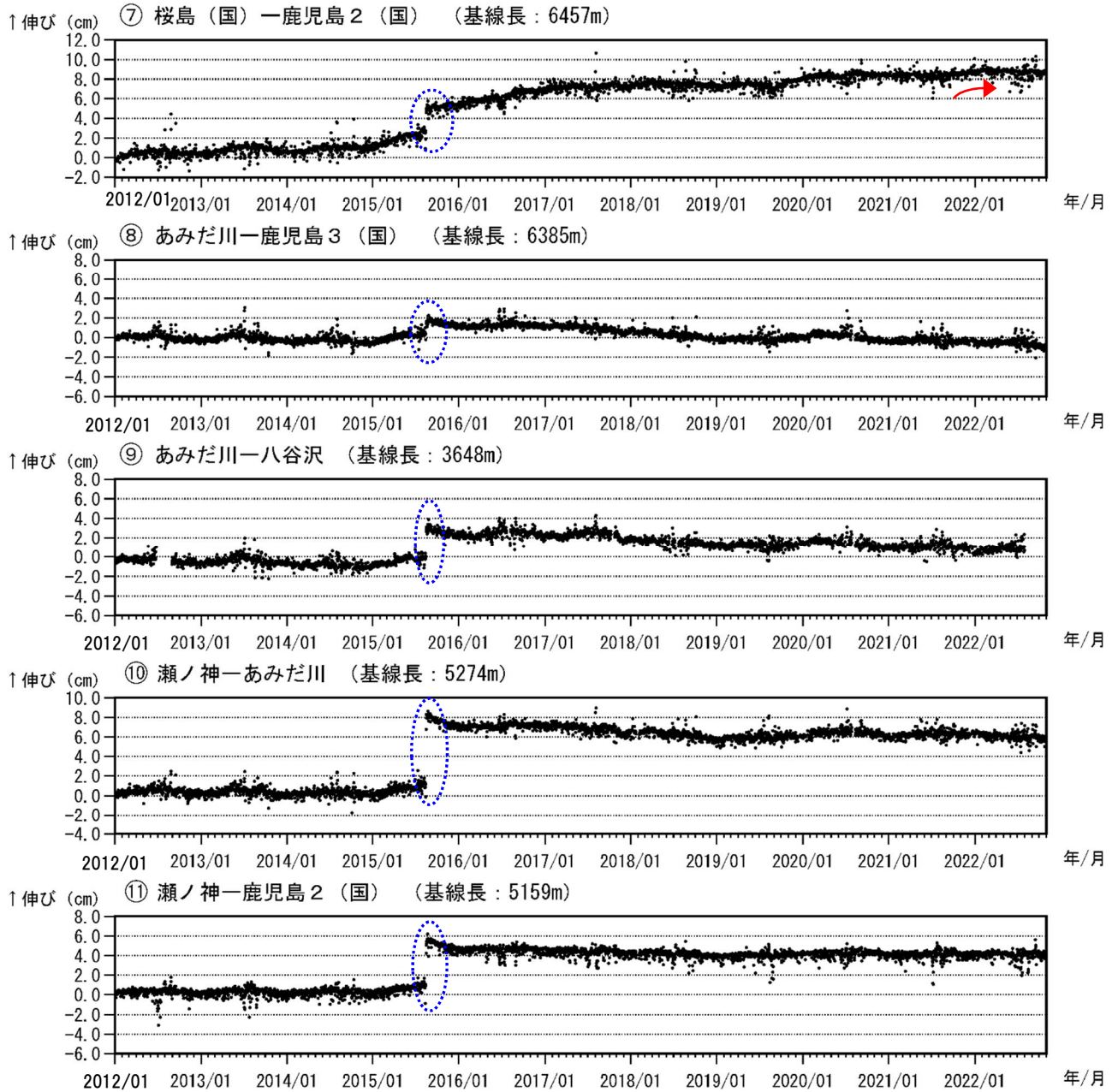
図 10-2 桜島 GNSS 連続観測による基線長変化（2012 年 1 月～2022 年 10 月）
