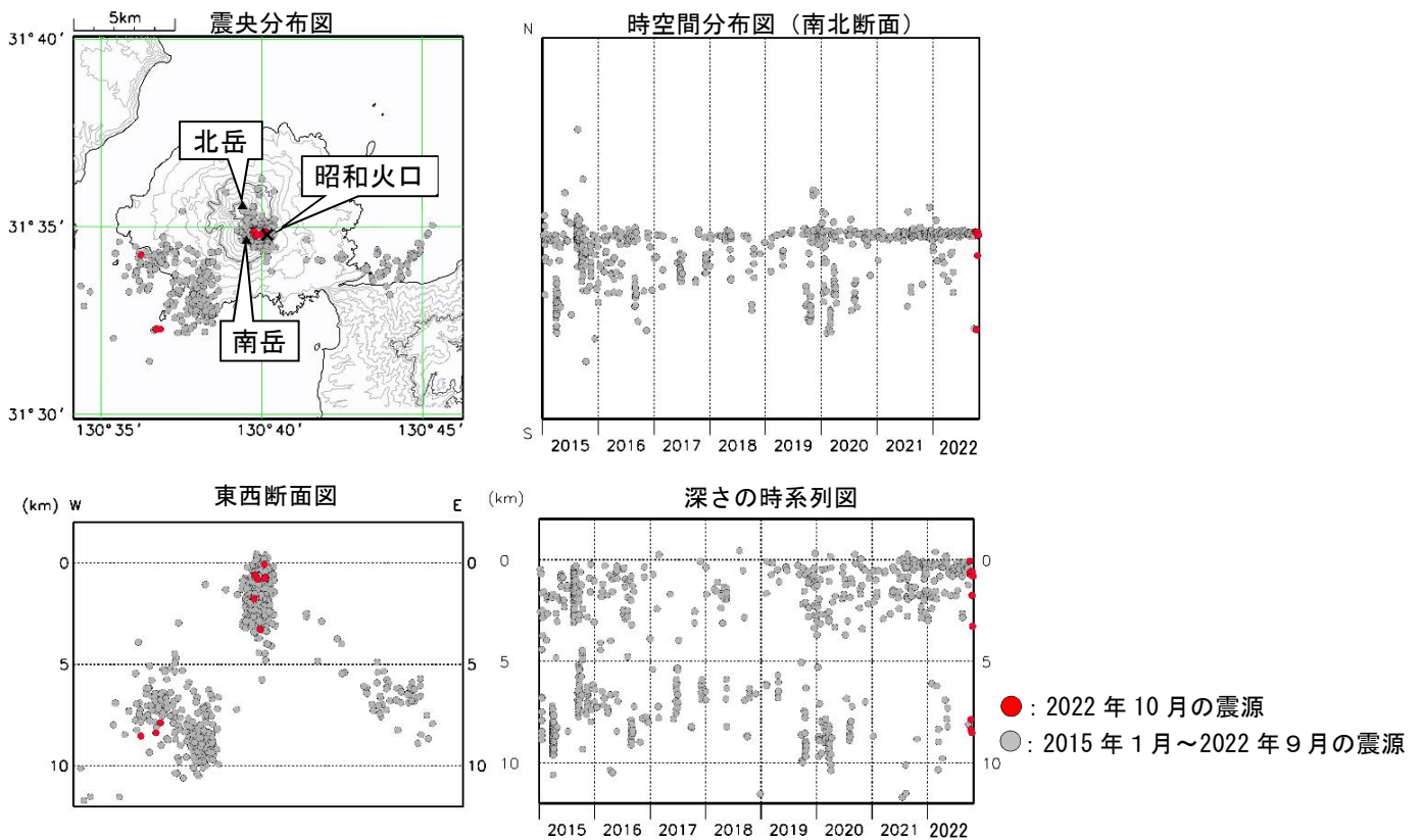
図 5-2 桜島 桜島付近の震源分布図（2015年1月～2022年10月）
