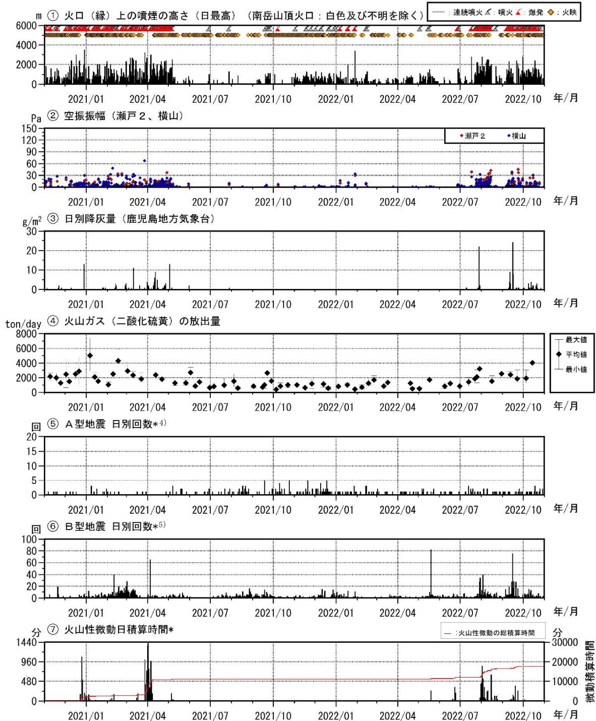
図8 桜島 最近2年間の活動経過図（2020年11月～2022年10月）
