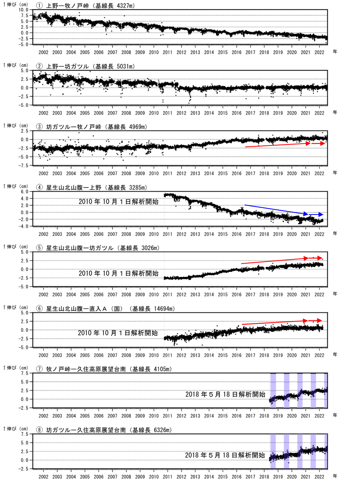
図5 九重山 GNSS連続観測による基線長変化（2001年4月～2022年8月）
