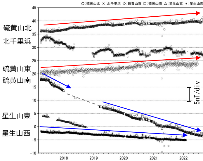
図 4-1 九重山 連続観測による全磁力の変化（2017年3月～2022年8月）
