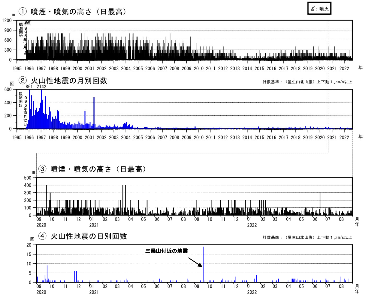
図2 九重山 火山活動経過図（1995年1月～2022年8月）
