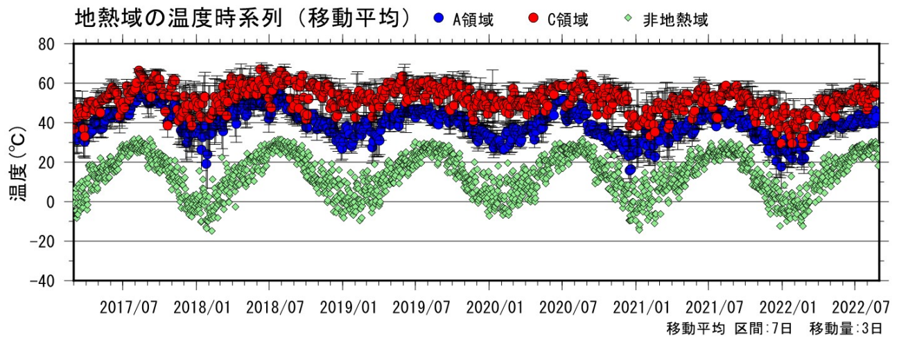
図 1-2 九重山 星生山北尾根の赤外熱映像装置による日別最高温度（2017年3月～2022年8月）
