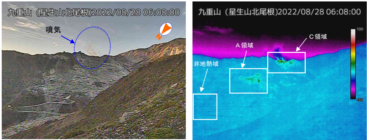
図 1-1 九重山 硫黄山の噴気及び地熱域の状況（8月28日 星生山北尾根監視カメラ）
