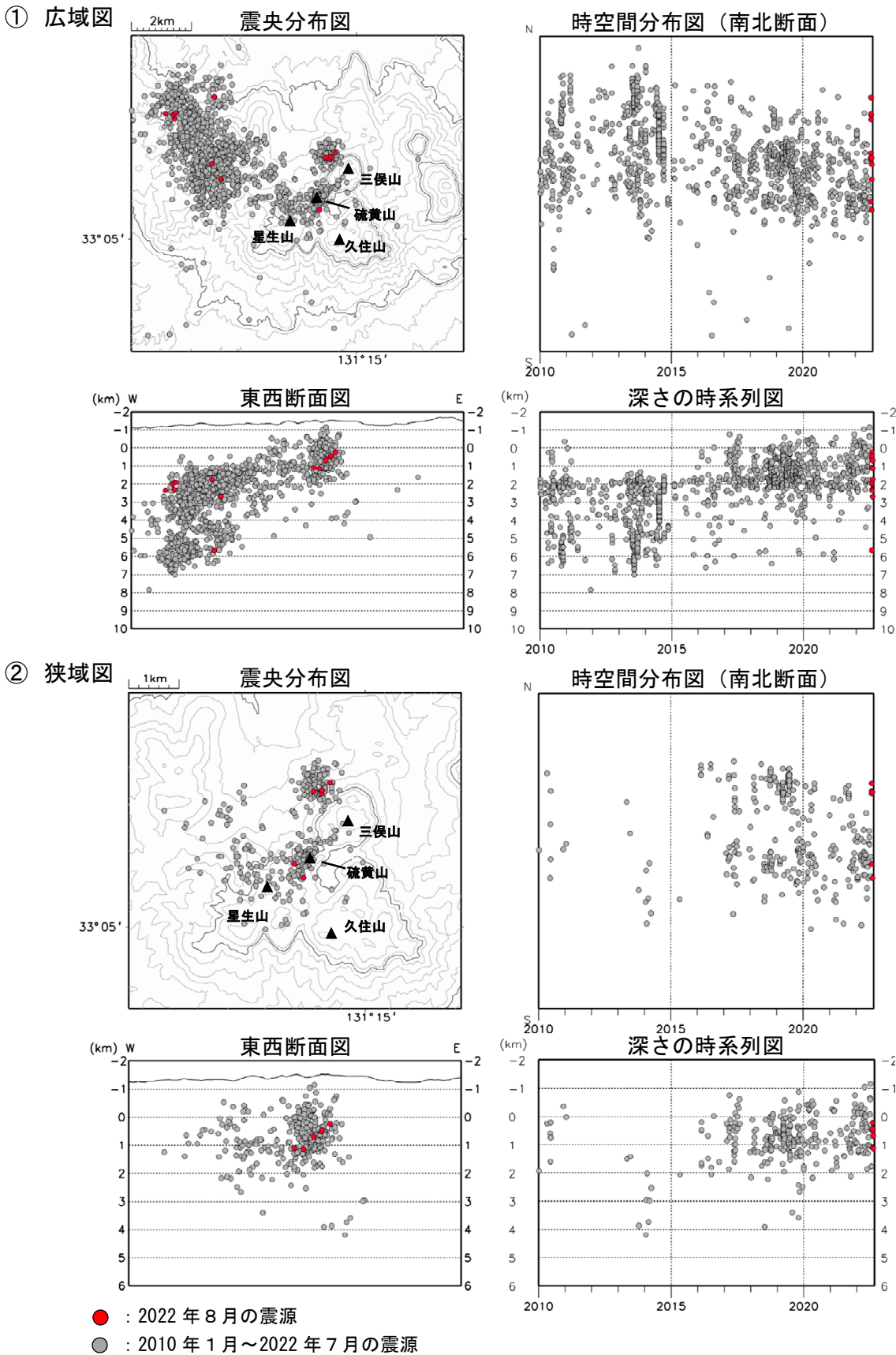
図3 九重山 震源分布図 ①広域図②狭域図（2010年1月～2022年8月）
