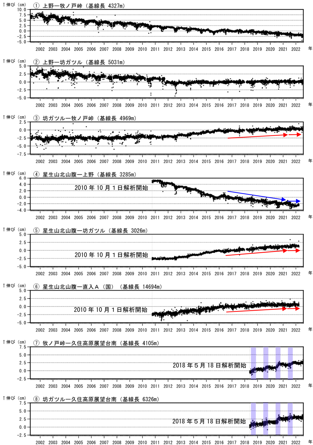
図5 九重山 GNSS連続観測による基線長変化（2001年4月～2022年7月）
