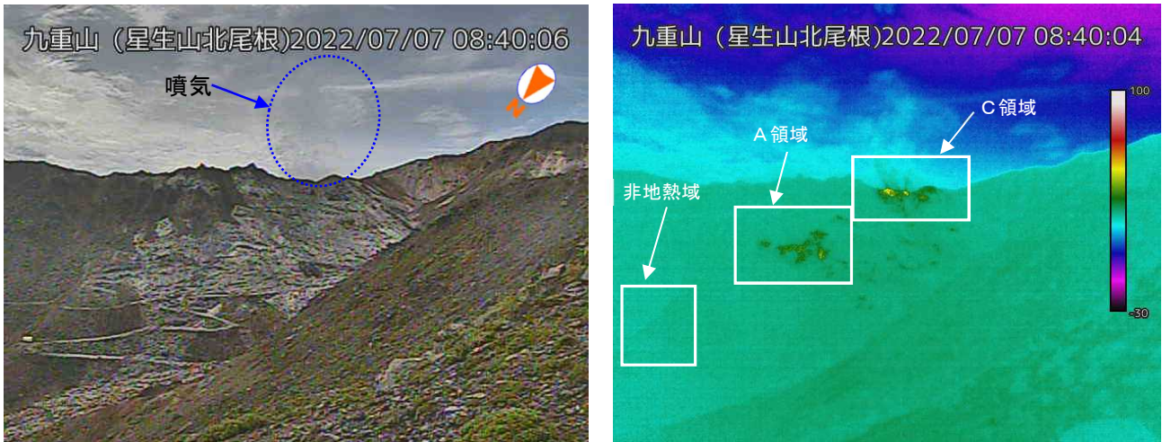
図 1-1 九重山 硫黄山の噴気及び地熱域の状況（7月7日 星生山北尾根監視カメラ）
