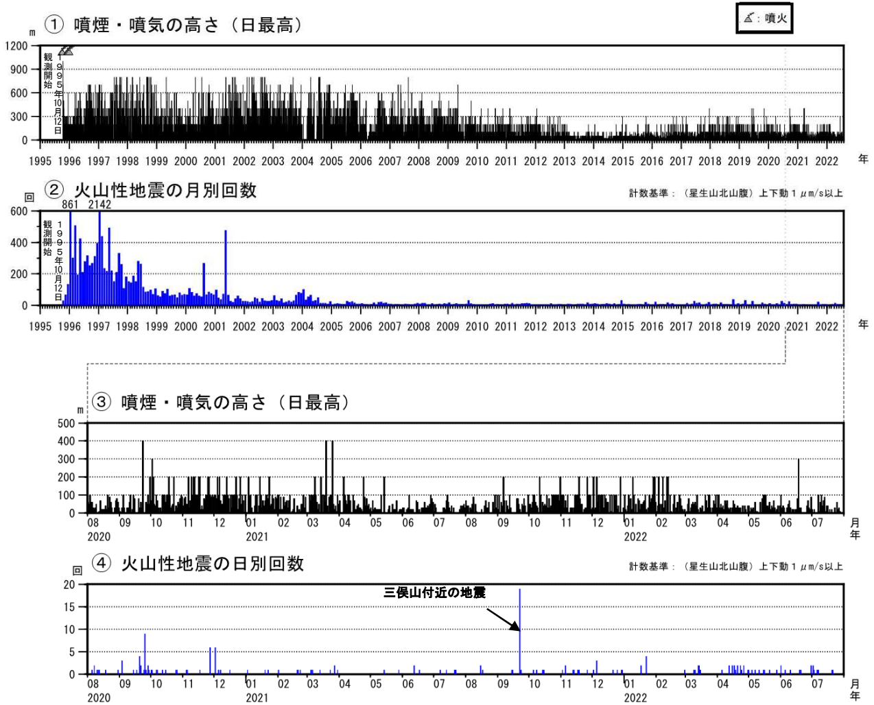
図2 九重山 火山活動経過図（1995年1月～2022年7月）
