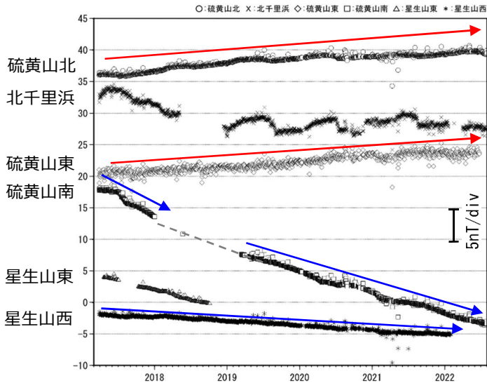
図 4-1 九重山 連続観測による全磁力の変化 (2017年3月～2022年7月)
