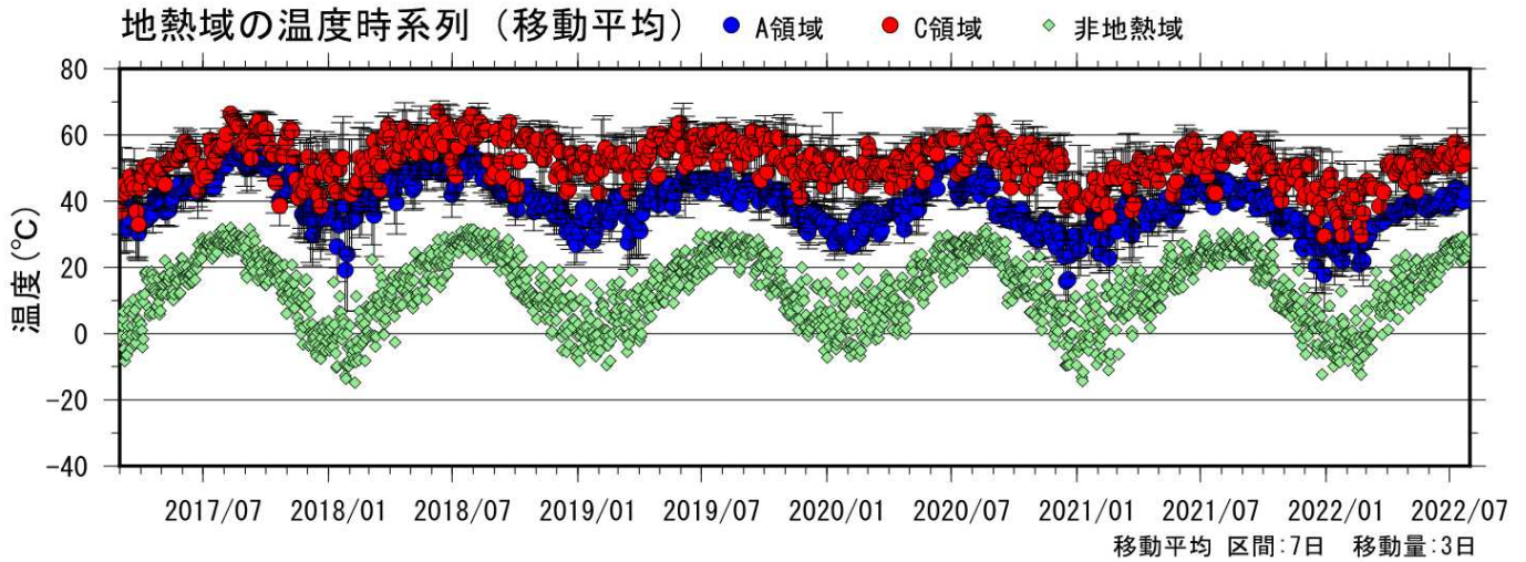
図 1-2 九重山 星生山北尾根の赤外熱映像装置による日別最高温度（2017年3月～2022年7月）
