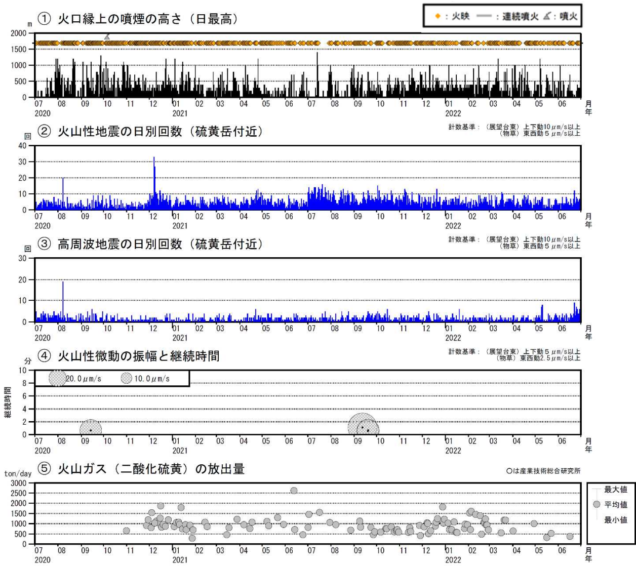
図4 薩摩硫黄島 火山活動経過図（2020年7月～2022年6月）
