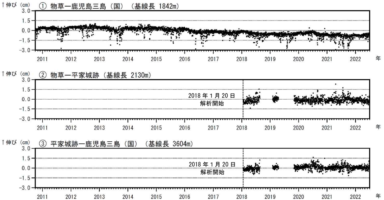
図6 薩摩硫黄島 GNSS連続観測による基線長変化 (2010年10月～2022年6月)
