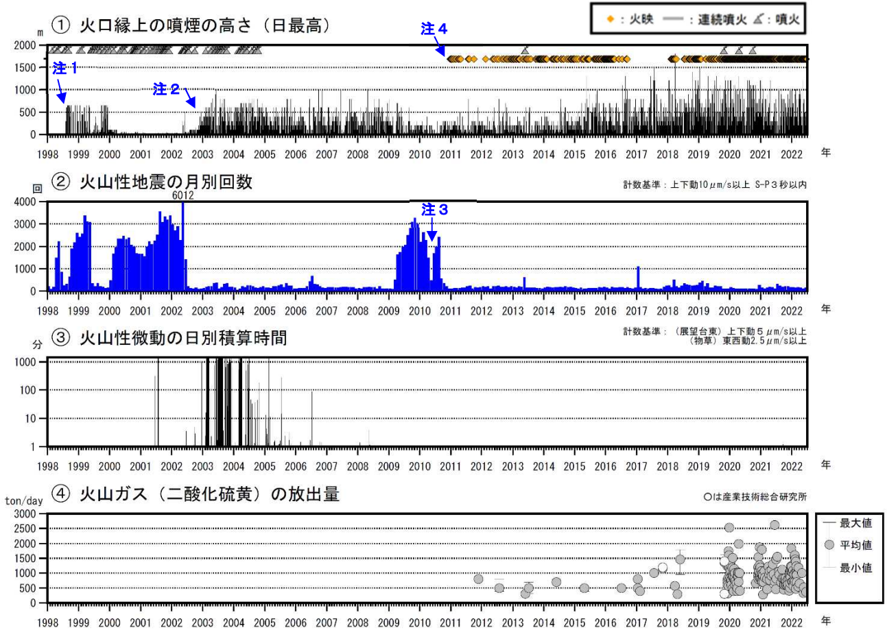
図3 薩摩硫黄島 火山活動経過図（1998年1月～2022年6月）
