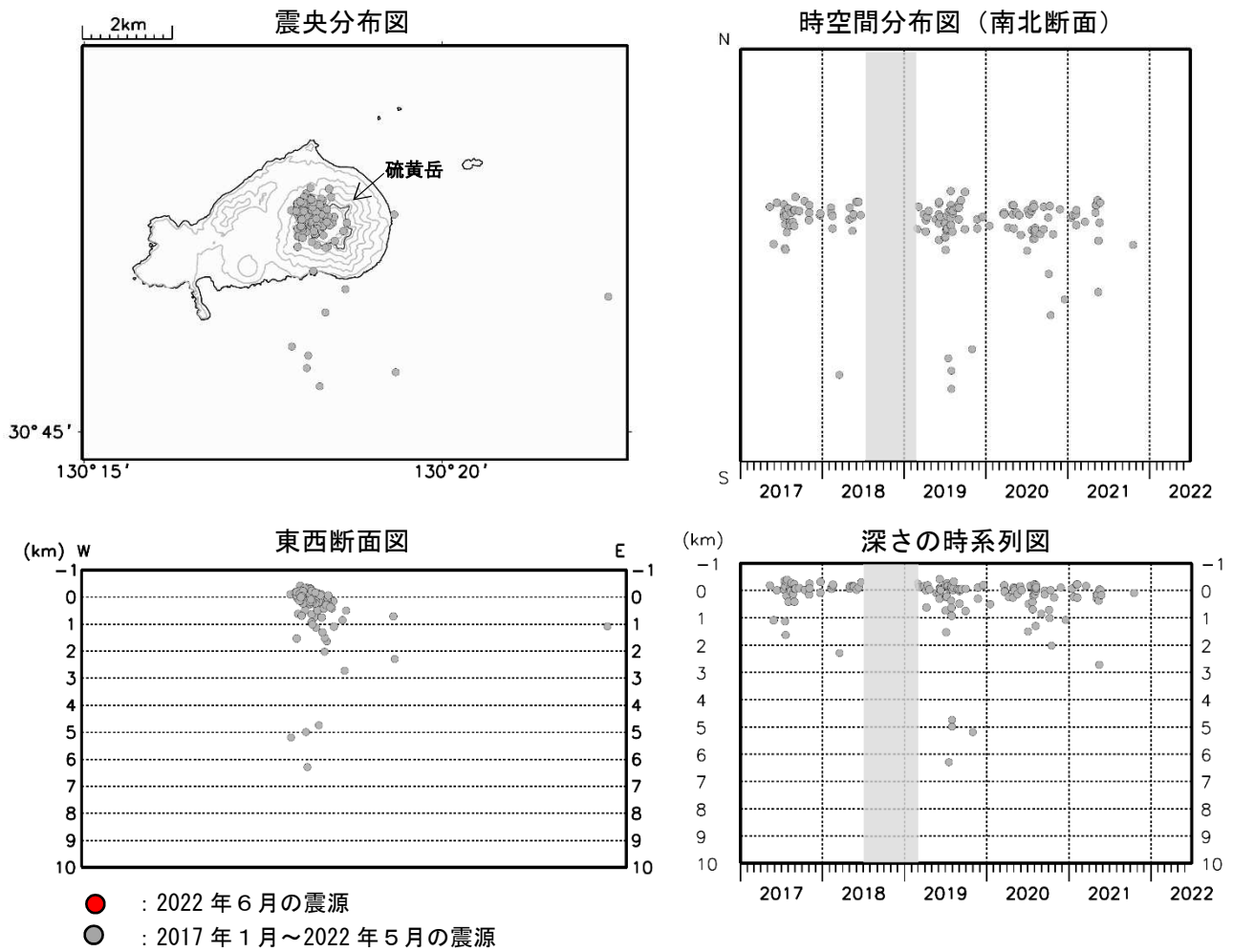
図5 薩摩硫黄島 火山性地震の震源分布図（2017年1月～2022年6月）
