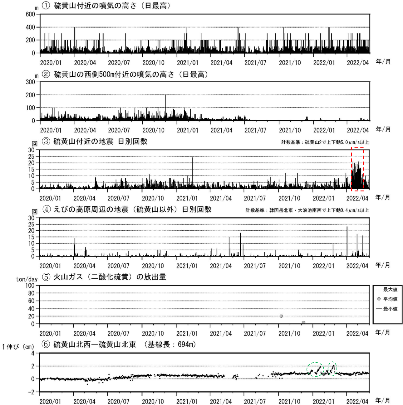
図5 霧島山（えびの高原（硫黄山）周辺） 火山活動経過図（2020年1月～2022年5月）
