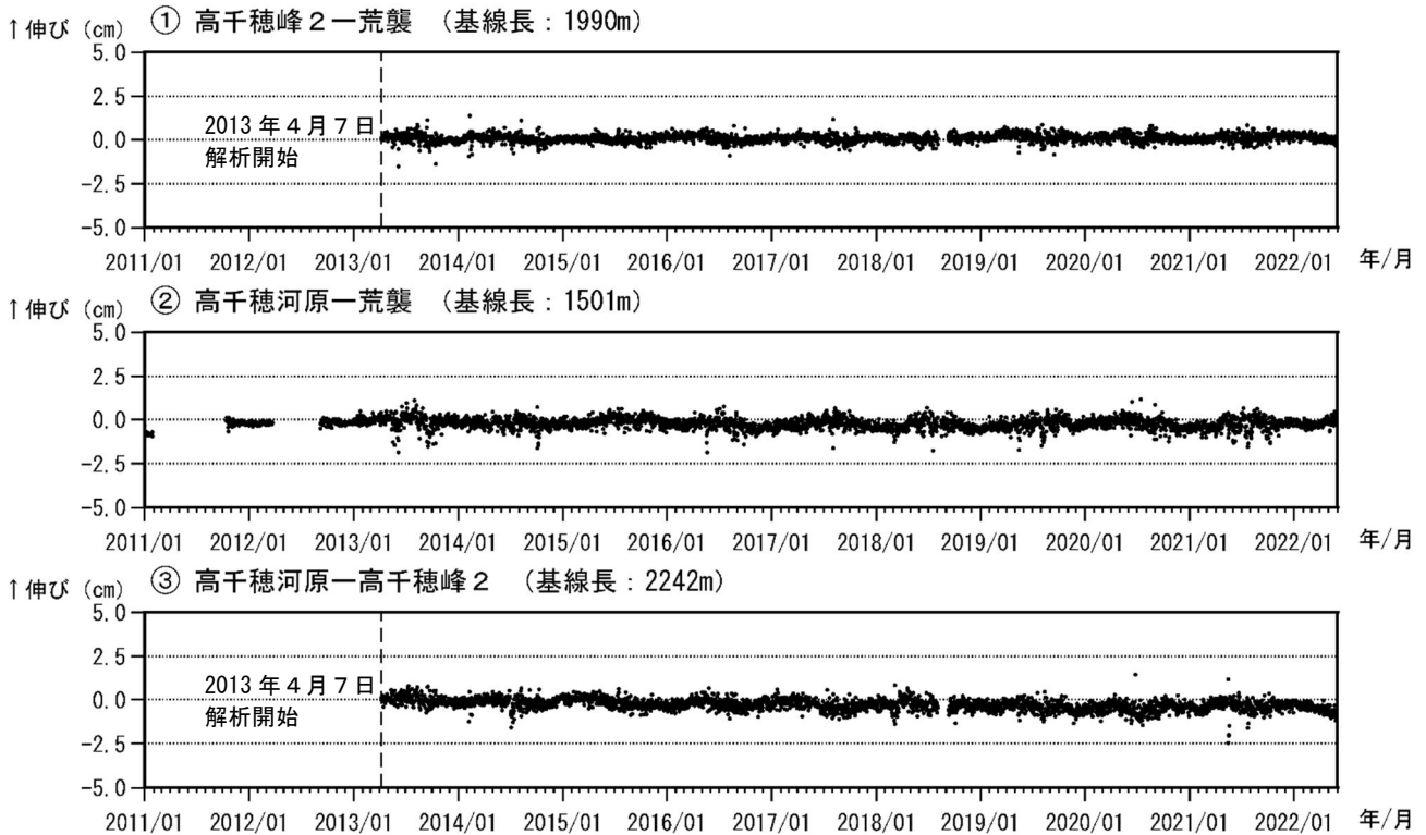
図6 霧島山（御鉢） GNSS 連続観測による基線長変化（2011年1月～2022年5月）
