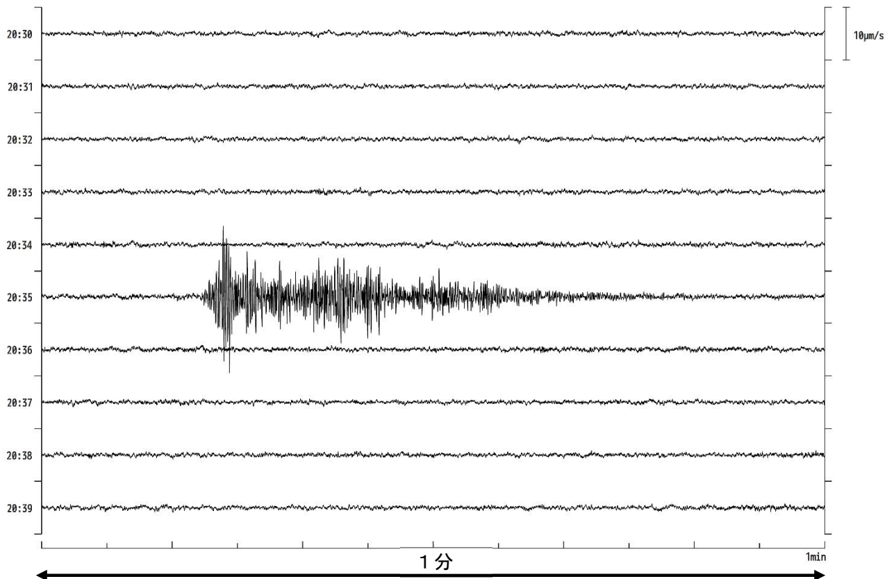
図4 霧島山（新燃岳） 5月13日20時35分に発生した火山性微動の状況 （2022年5月13日20時30分～40分、新燃岳南西地震計：速度波形南北動成分）
