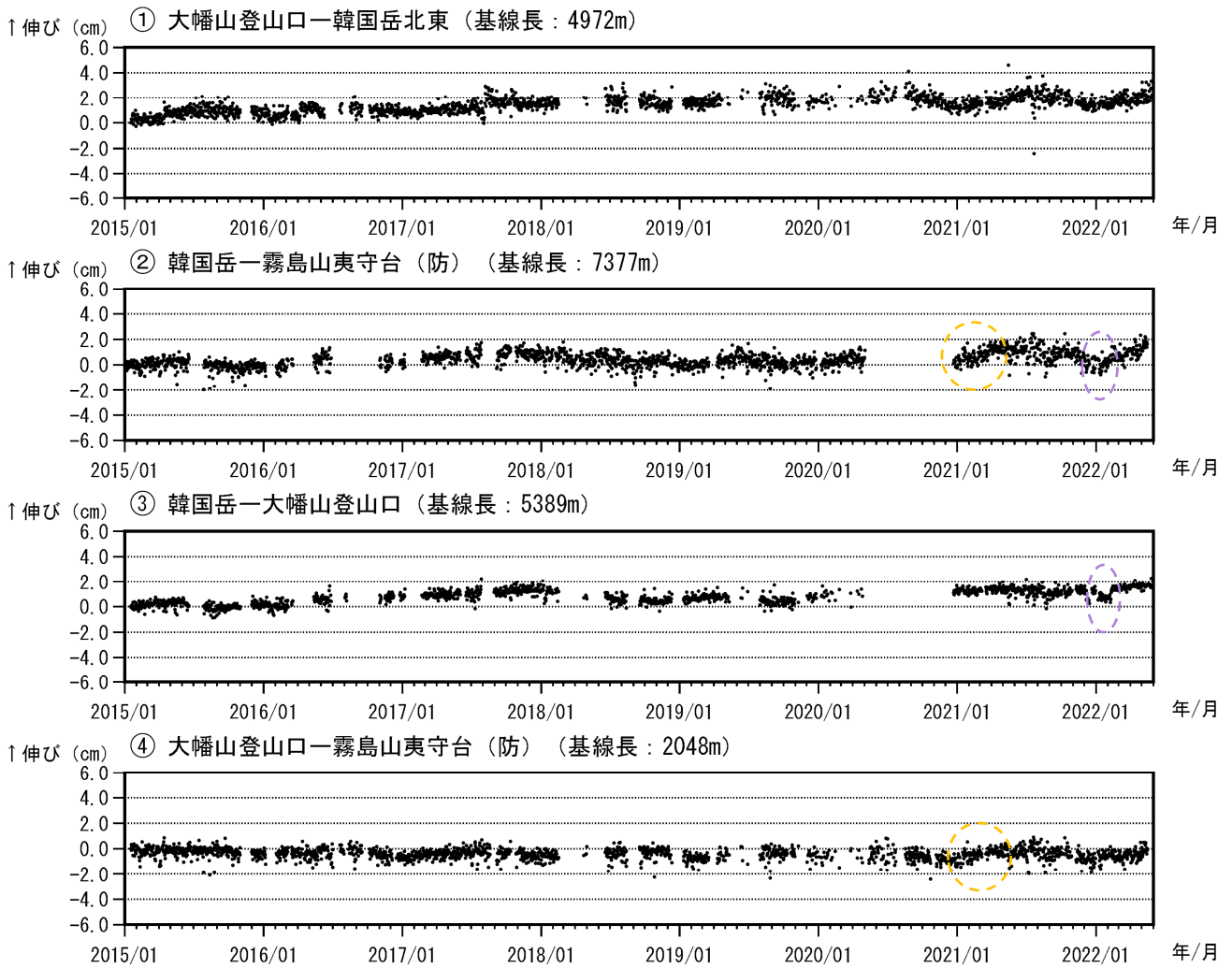
図6 霧島山（大幡池） GNSS 連続観測による基線長変化（2015年1月～2022年5月）
