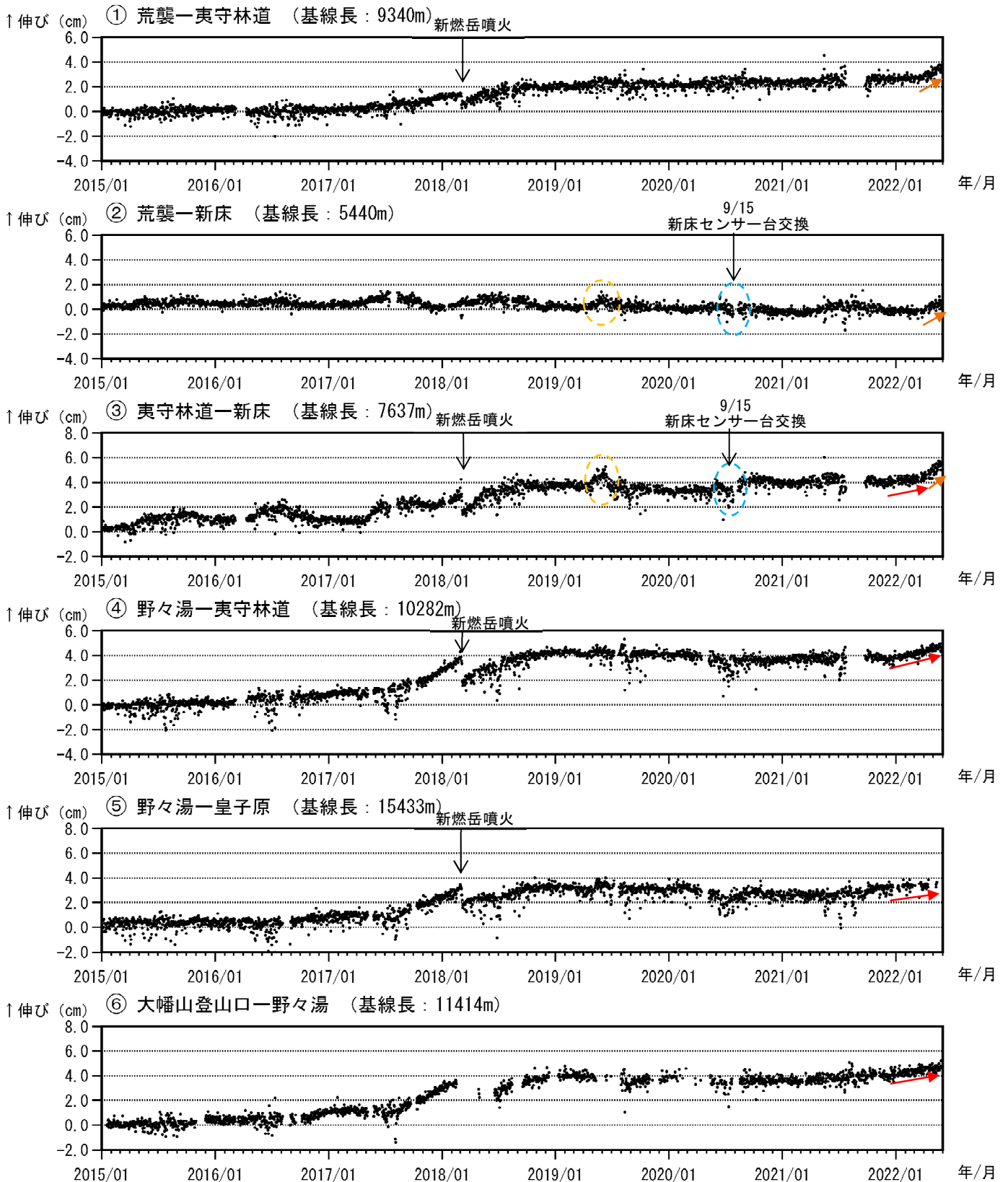
図7 霧島山（新燃岳） GNSS 連続観測による基線長変化（2015年1月～2022年5月）
