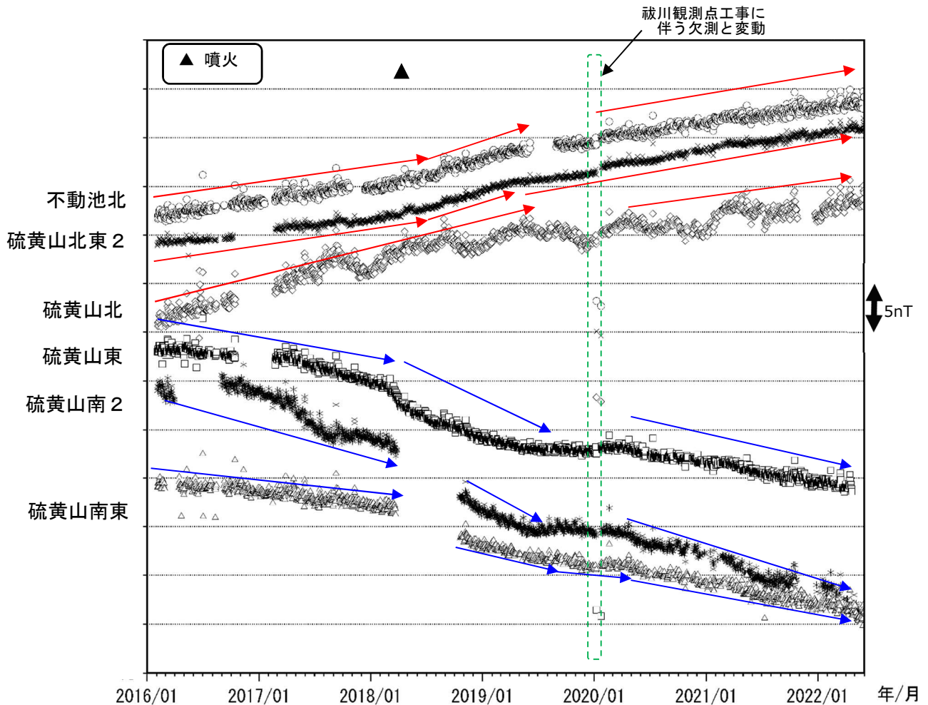
図 8-2 霧島山（えびの高原（硫黄山）周辺） 全磁力観測点で観測された全磁力変動（2016年1月～2022年5月）
