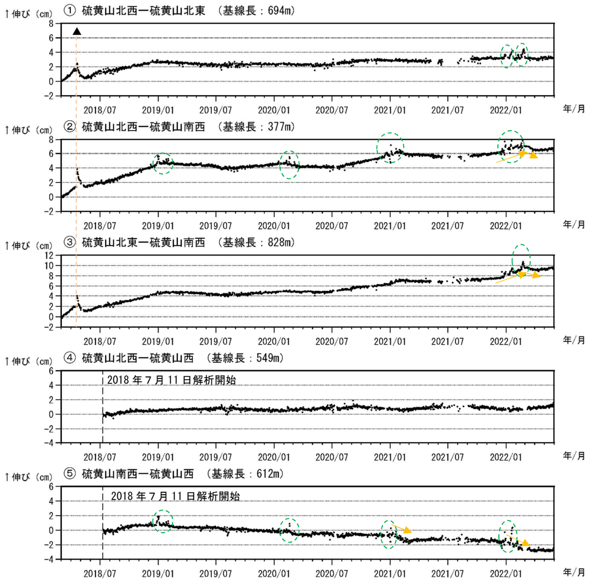
図6 霧島山（えびの高原（硫黄山）周辺） GNSS 連続観測による基線長変化 (2018年3月～2022年5月)
