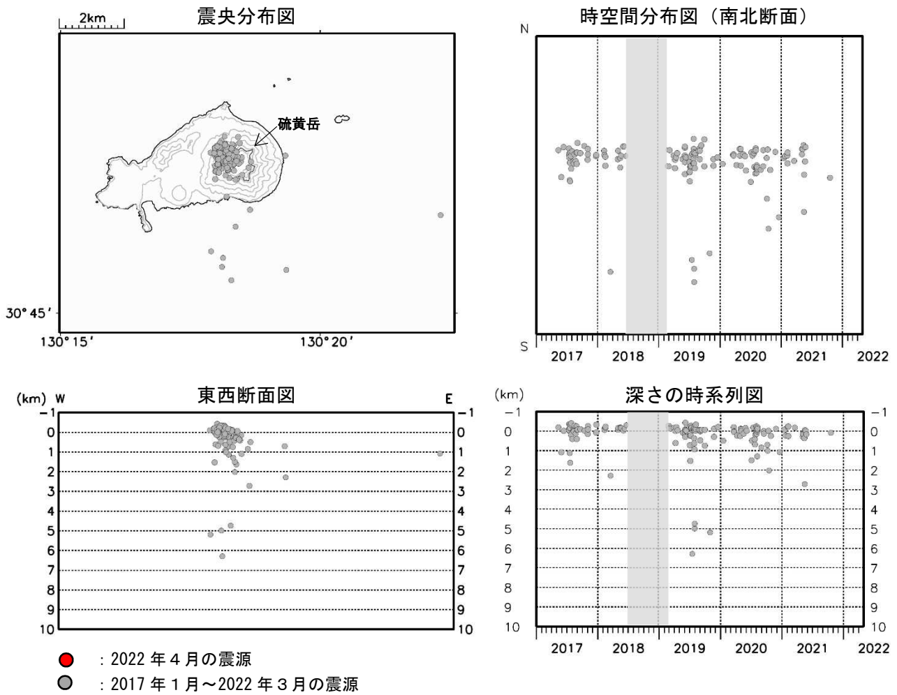
図5 薩摩硫黄島 火山性地震の震源分布図（2017年1月～2022年4月）
