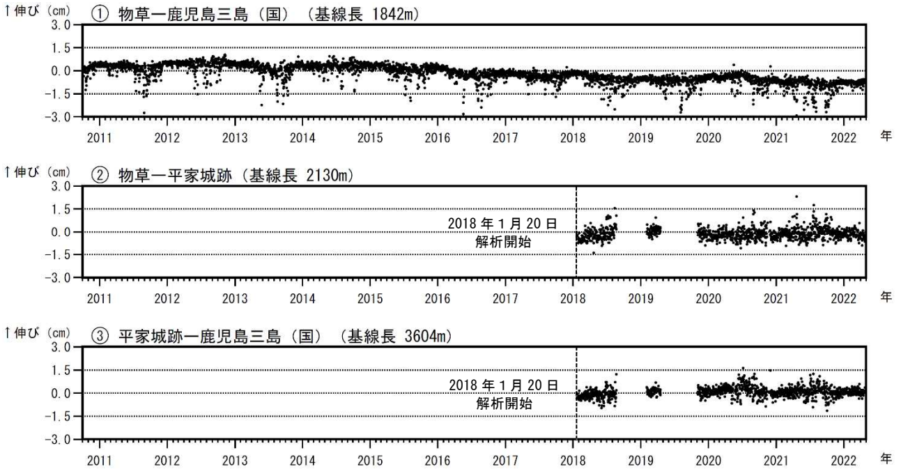
図6 薩摩硫黄島 GNSS連続観測による基線長変化 (2010年10月～2022年4月)
