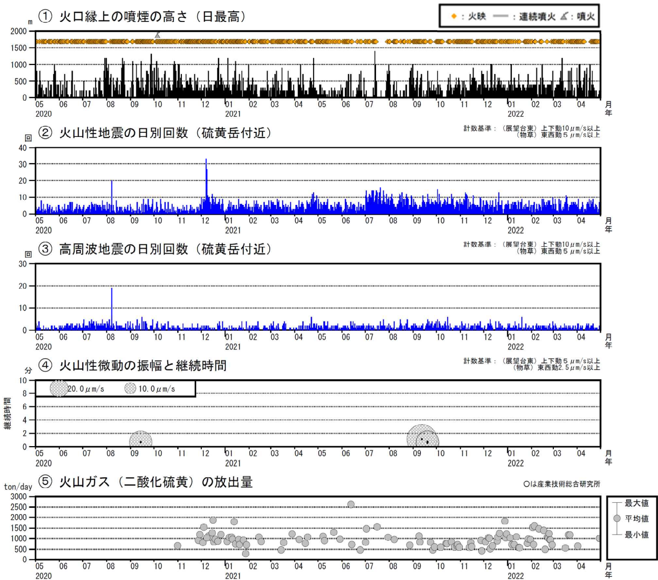
図4 薩摩硫黄島 火山活動経過図（2020年5月～2022年4月）
