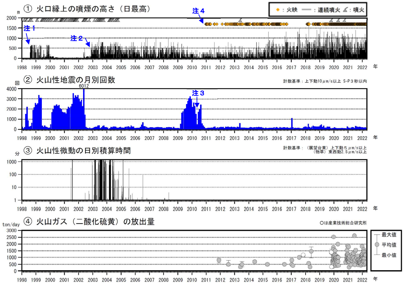
図3 薩摩硫黄島 火山活動経過図（1998年1月～2022年4月）
