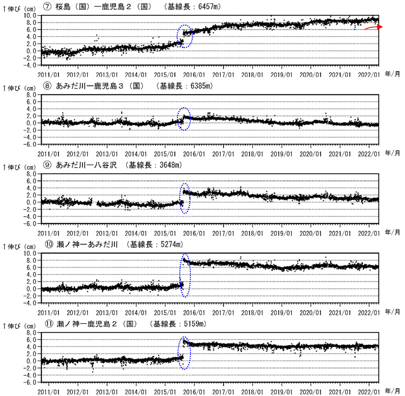
図 7-2 桜島 GNSS 連続観測による基線長変化（2010 年 10 月～2022 年 4 月）
