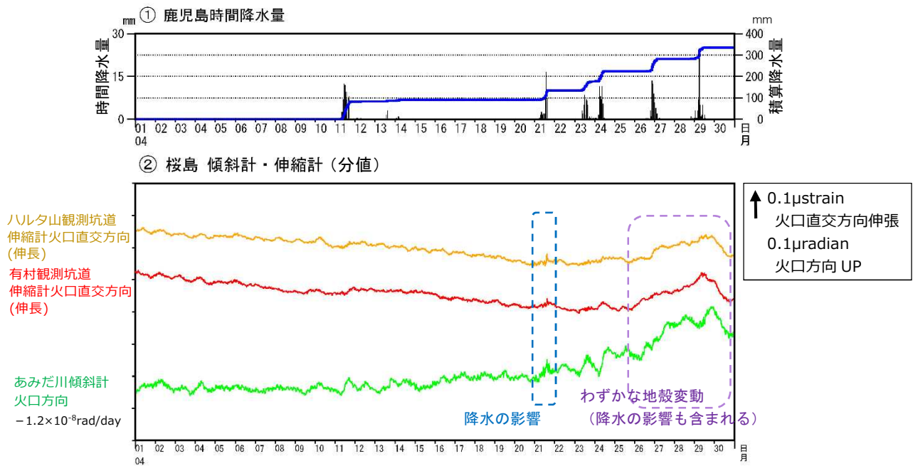
図6 桜島 傾斜計及び伸縮計による地殻変動の状況（2022年4月）
