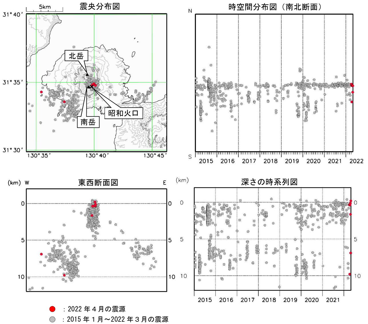
図2 桜島 震源分布図（2015年1月～2022年4月）
