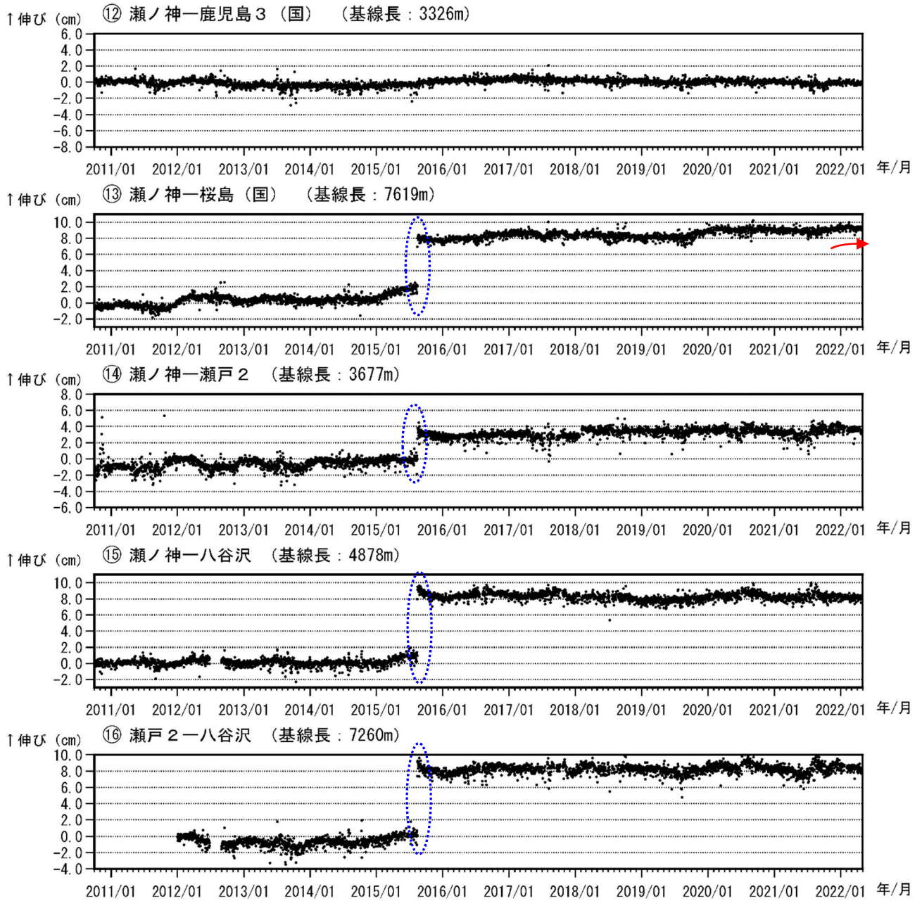
図 7-3 桜島 GNSS 連続観測による基線長変化 (2010 年 10 月～2022 年 4 月)
