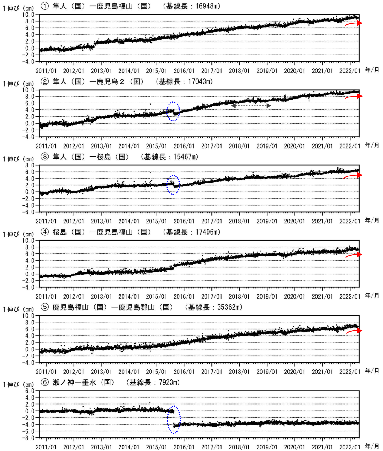
図 7-1 桜島 GNSS 連続観測による基線長変化（2010年10月～2022年4月）
