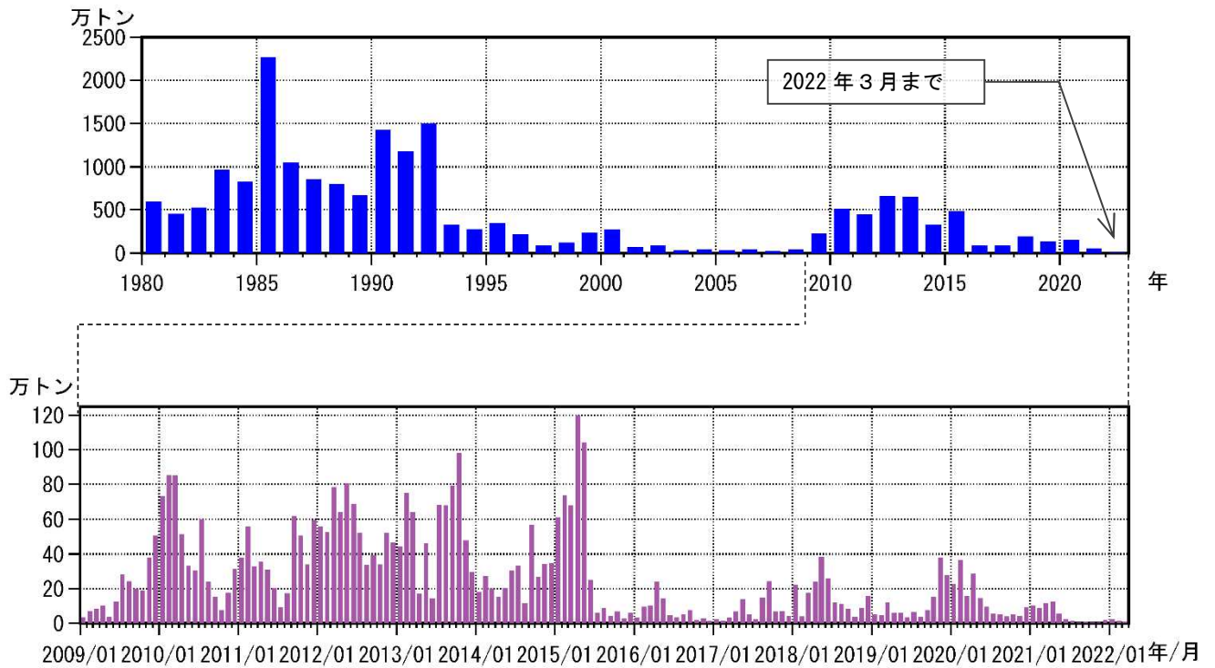
図4 桜島 鹿児島県が実施している降灰の観測データから推定した火山灰の総噴出量 （上段：1980年1月～2022年3月の年別値、下段：2009年1月～2022年3月の月別値）
