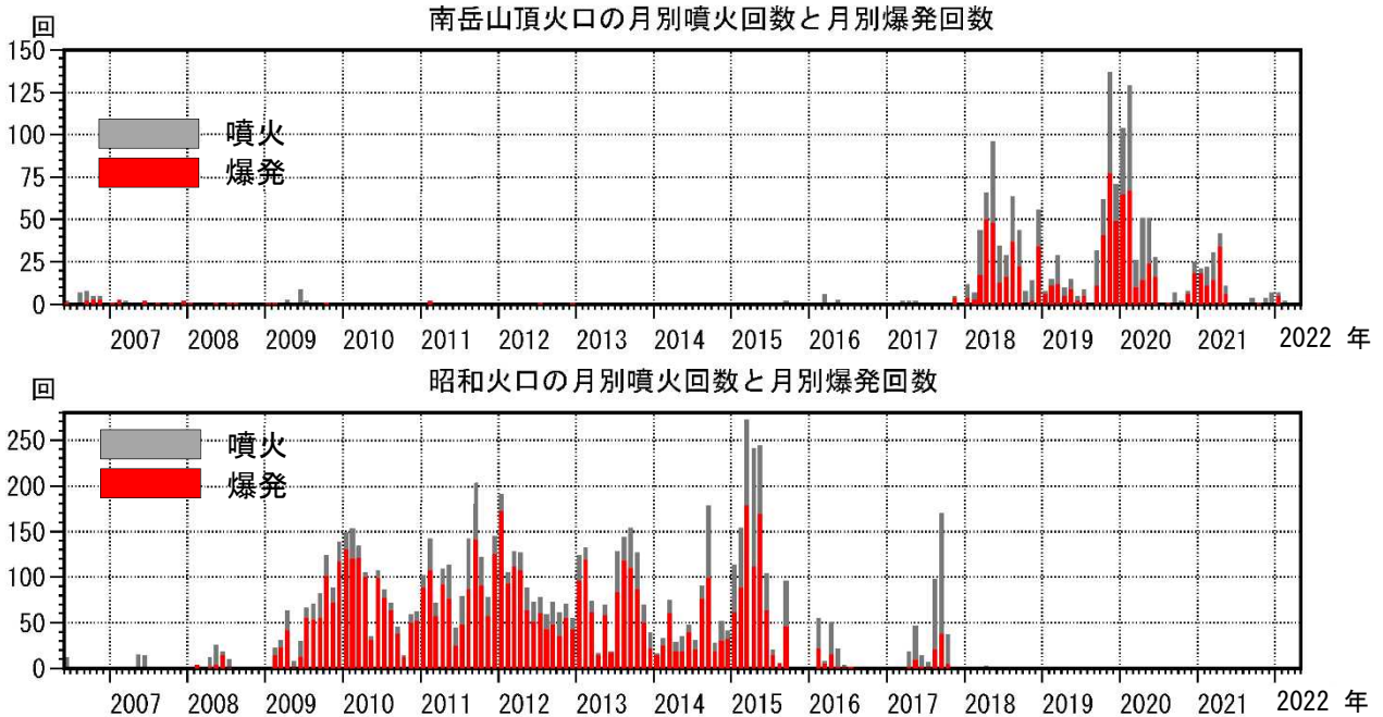
図3 桜島 南岳山頂火口（上図）と昭和火口（下図）の月別噴火回数と月別爆発回数 （2006年6月～2022年4月）
