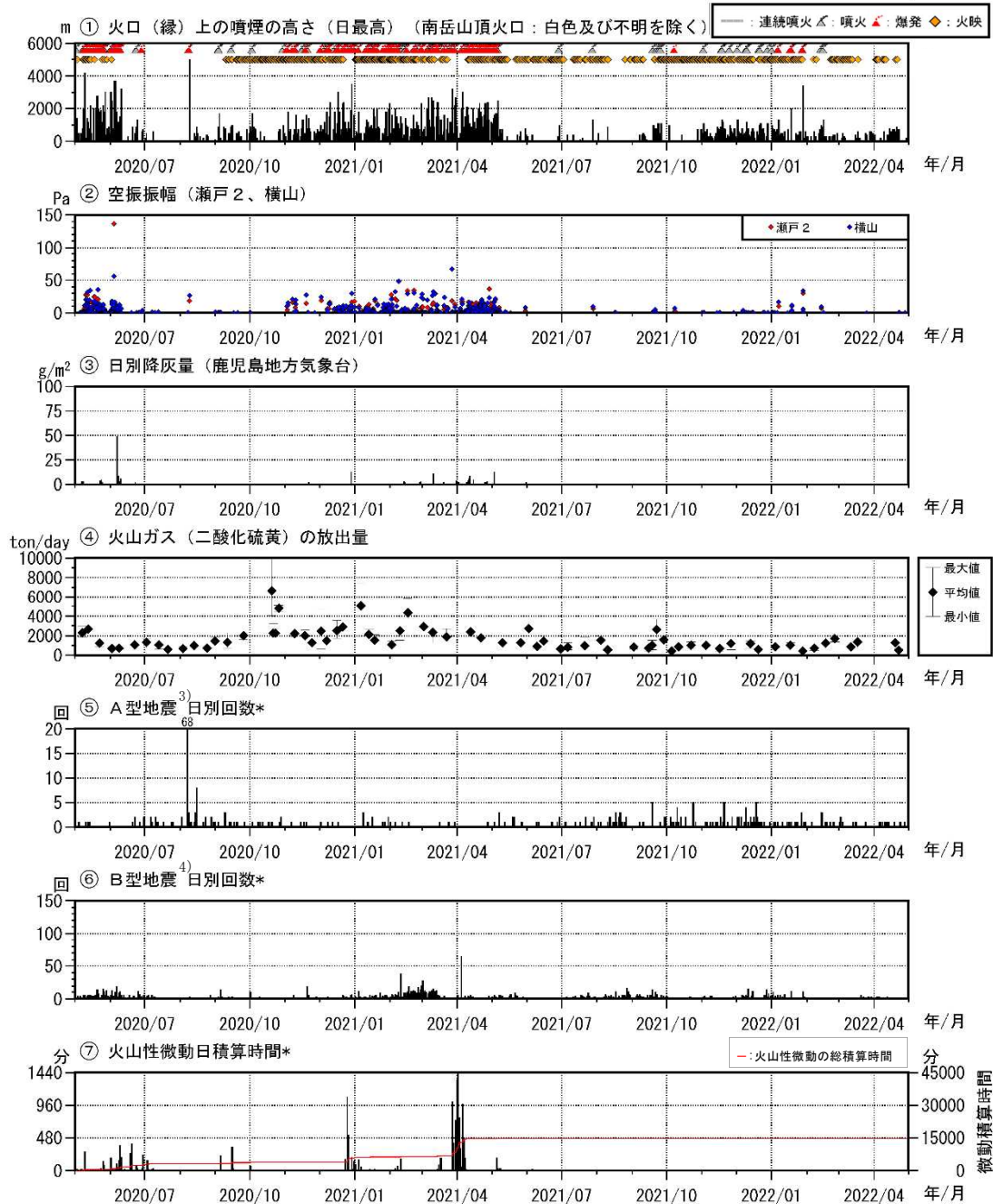
図5 桜島 最近2年間の活動経過図（2020年5月～2022年4月）
