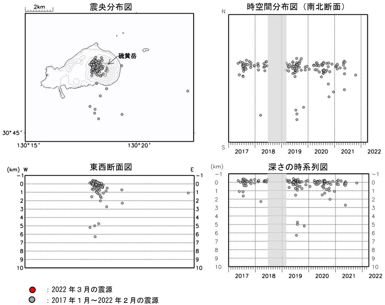
図5 薩摩硫黄島 火山性地震の震源分布図（2017年1月～2022年3月）
