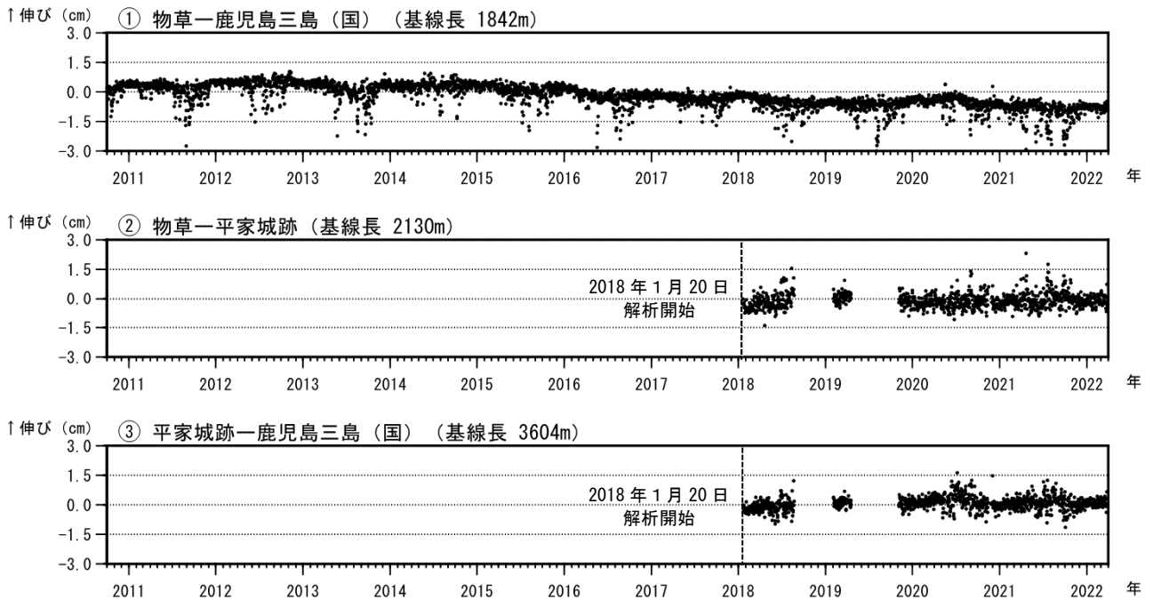
図6 薩摩硫黄島 GNSS連続観測による基線長変化 (2010年10月～2022年3月)
