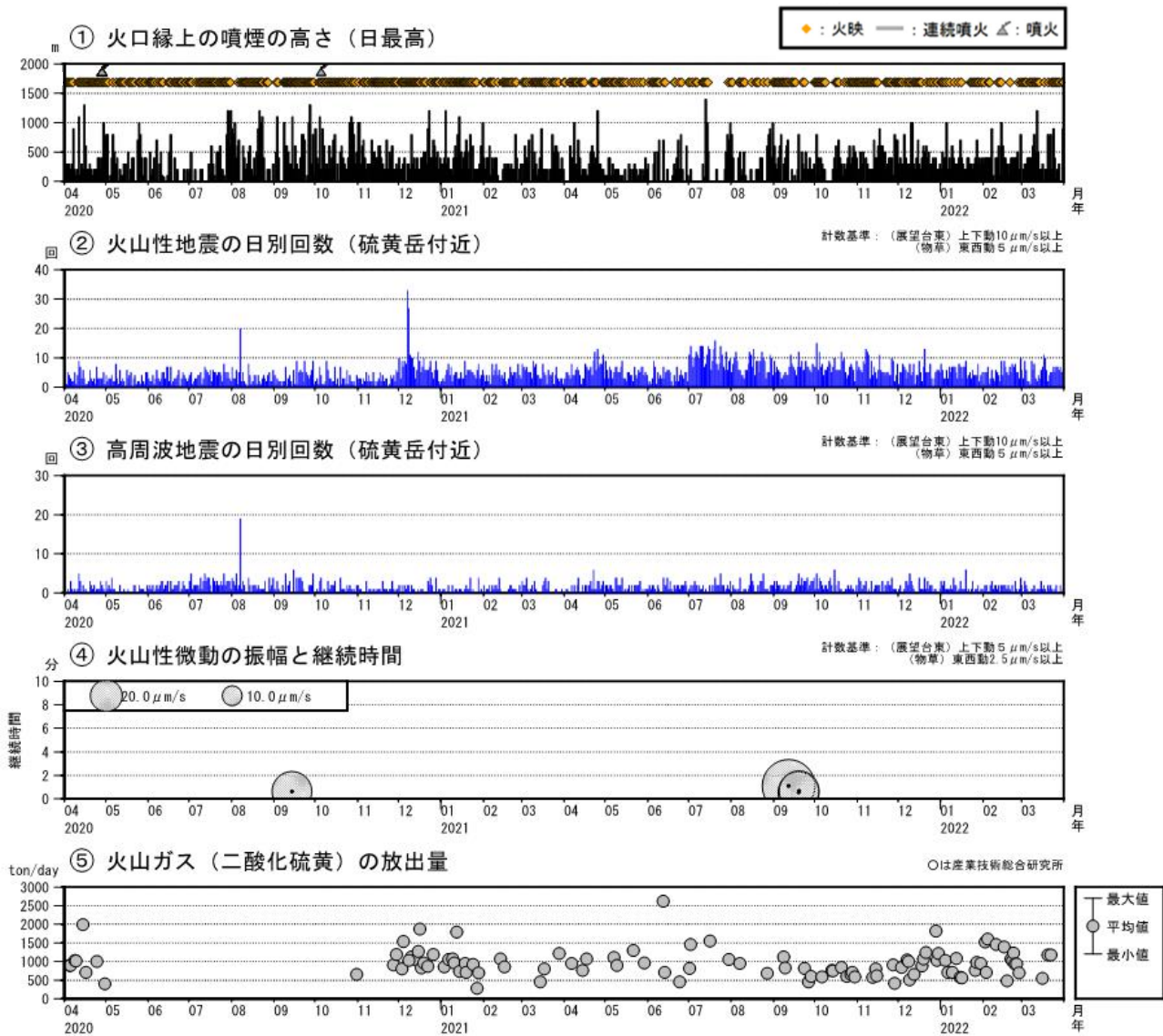
図4 薩摩硫黄島 火山活動経過図（2020年4月～2022年3月）
