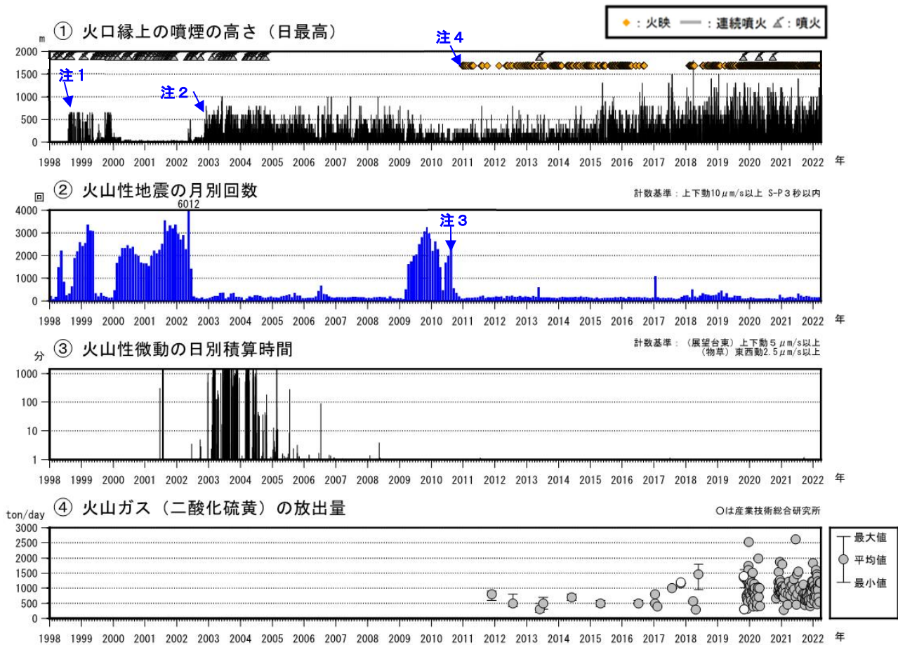
図3 薩摩硫黄島 火山活動経過図（1998年1月～2022年3月）
