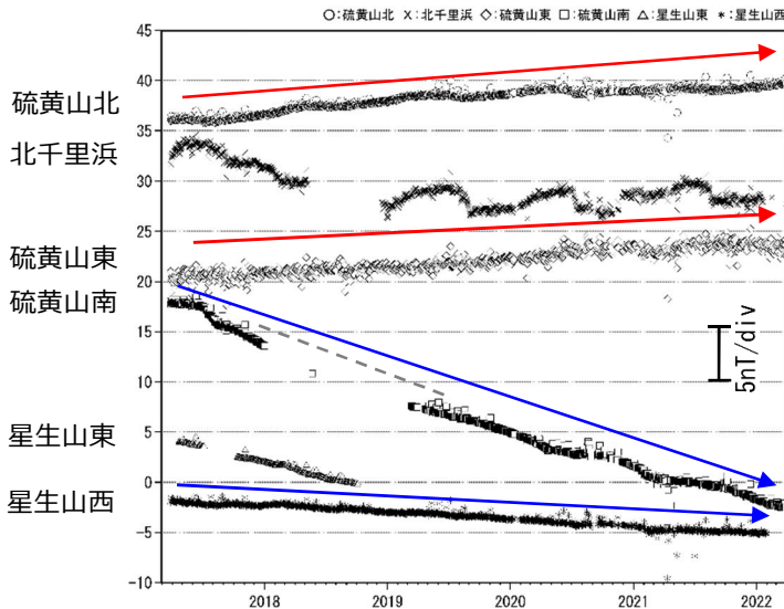
図 5-1 九重山 連続観測による全磁力の変化 (2017年3月～2022年3月)
