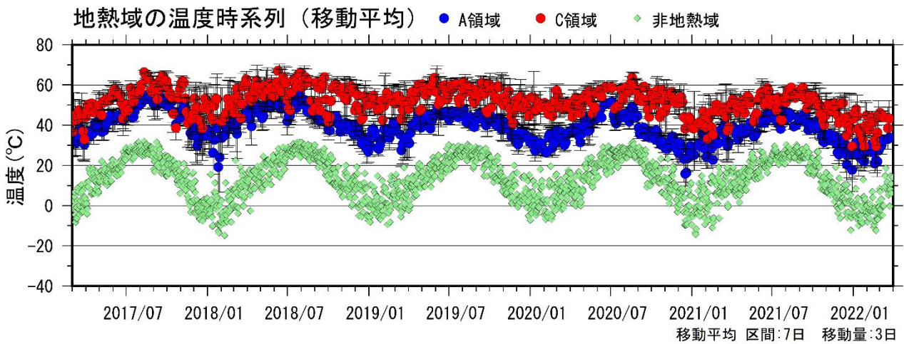
図 1-2 九重山 星生山北尾根の赤外熱映像装置による日別最高温度（2017年3月～2022年3月）
