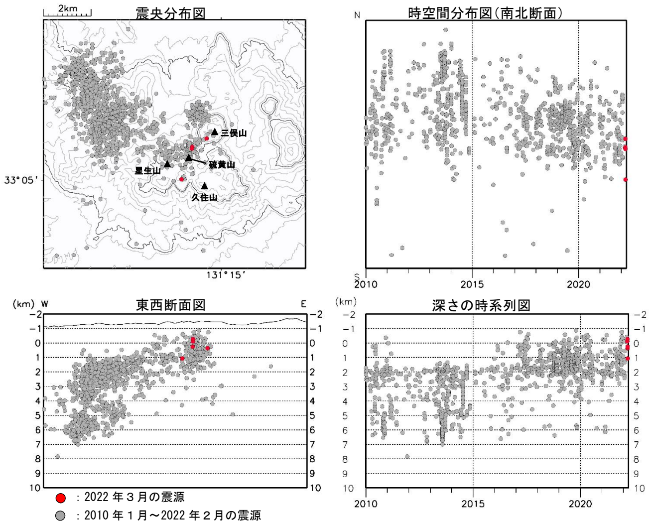
図4 九重山 震源分布図（2010年1月～2022年3月）
