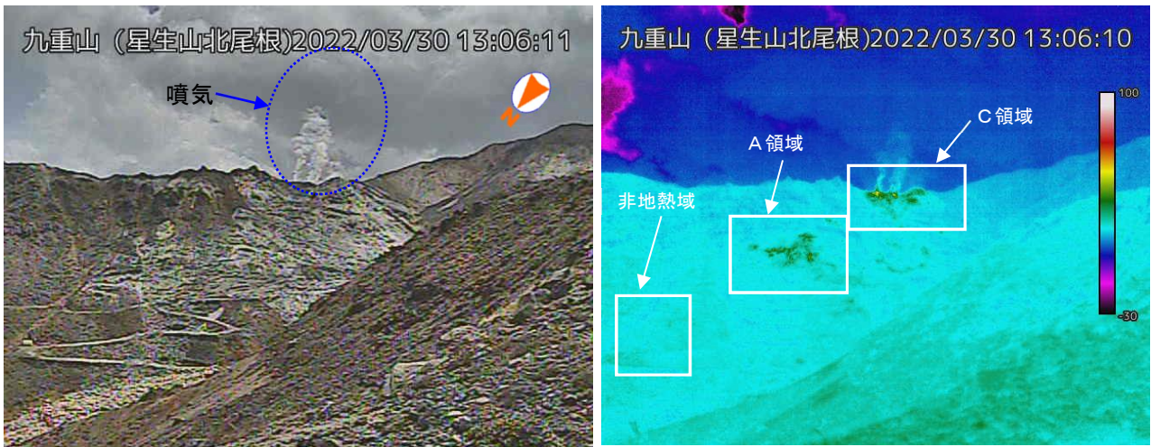
図 1-1 九重山 硫黄山の噴気及び地熱域の状況（3月30日 星生山北尾根監視カメラ）
