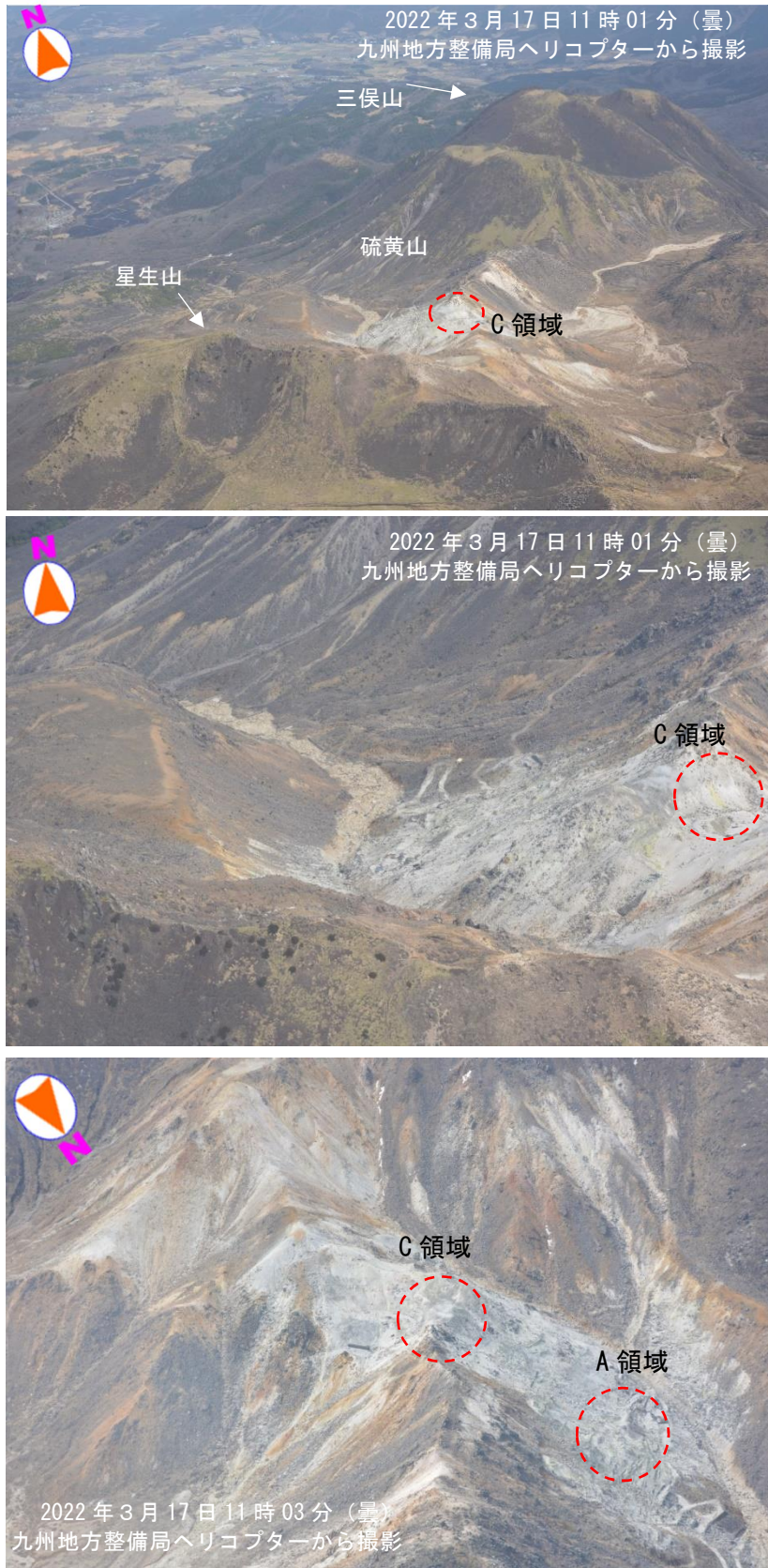
図 2-3 九重山 上空からの観測による硫黄山周辺及び硫黄山付近の状況 17日に九州地方整備局の協力により実施した上空からの観測では、硫黄山の噴気地帯（A領域、C領域）から白色の噴気が上がっているのを確認しました（赤破線部分）。
