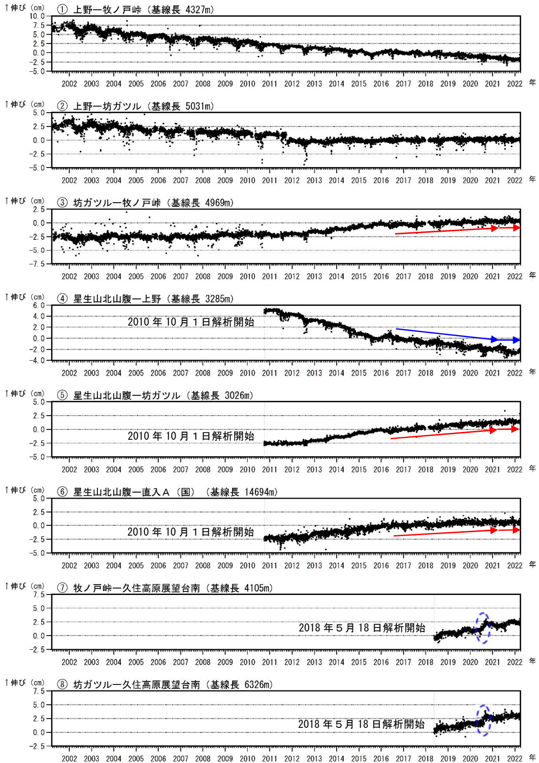
図6 九重山 GNSS連続観測による基線長変化（2001年4月～2022年3月）
