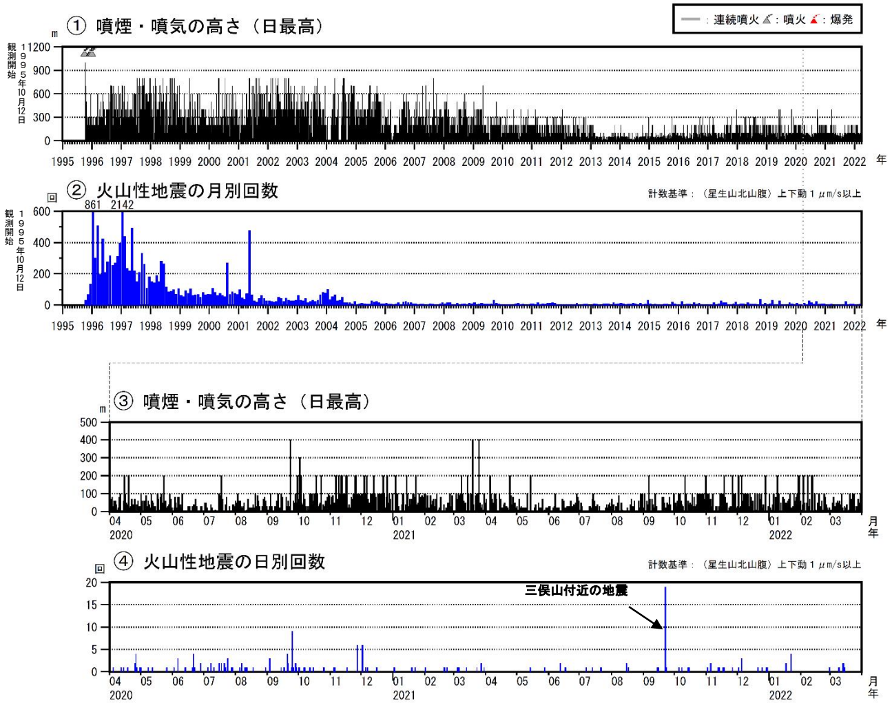
図3 九重山 火山活動経過図（1995年1月～2022年3月）
