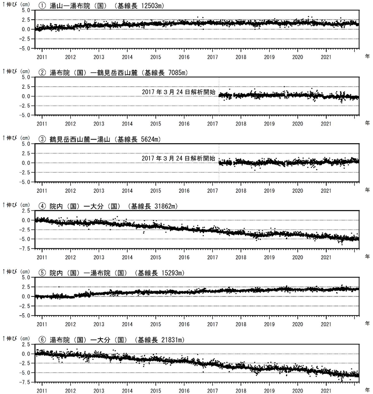
図4 鶴見岳・伽藍岳 GNSS連続観測による基線長変化（2010年10月～2022年2月）
