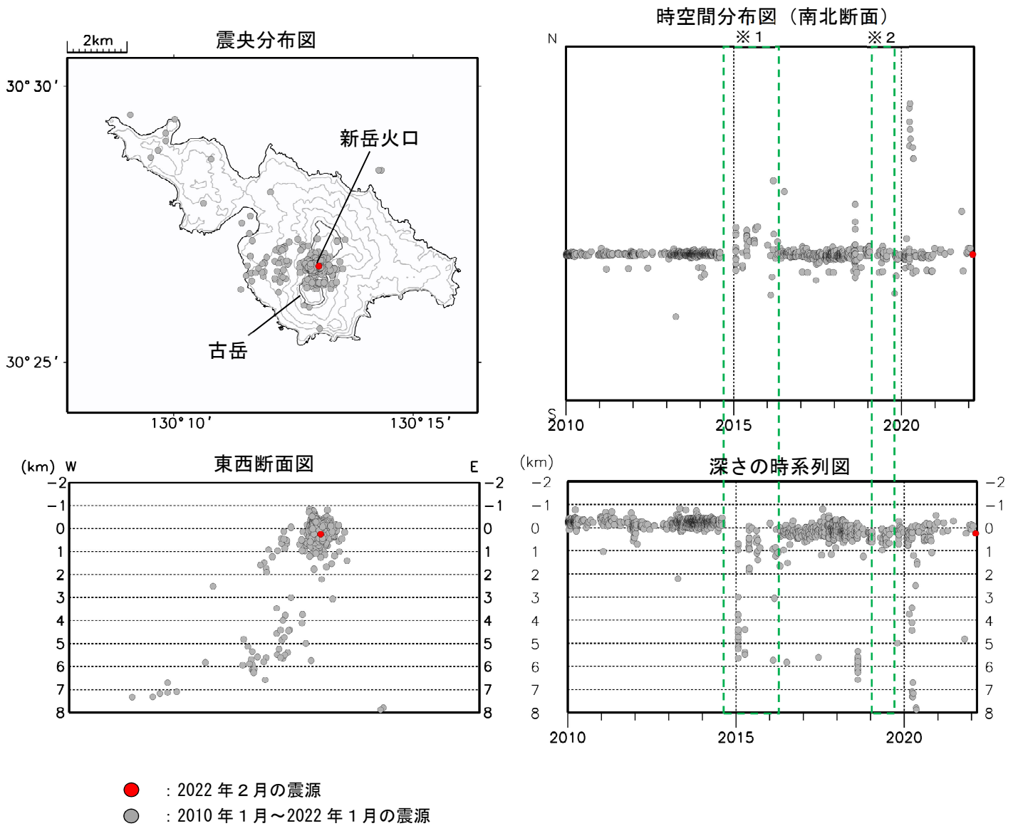
図7 口永良部島 震源分布図（2010年1月～2022年2月）
