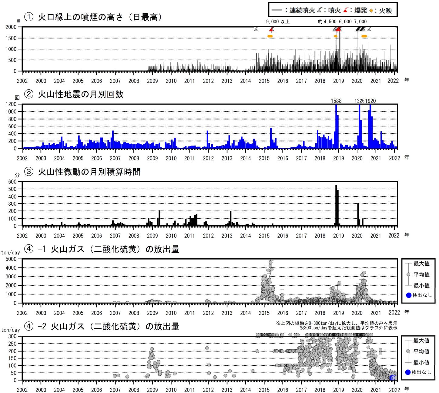
図5 口永良部島 火山活動経過図（2002年1月～2022年2月）
