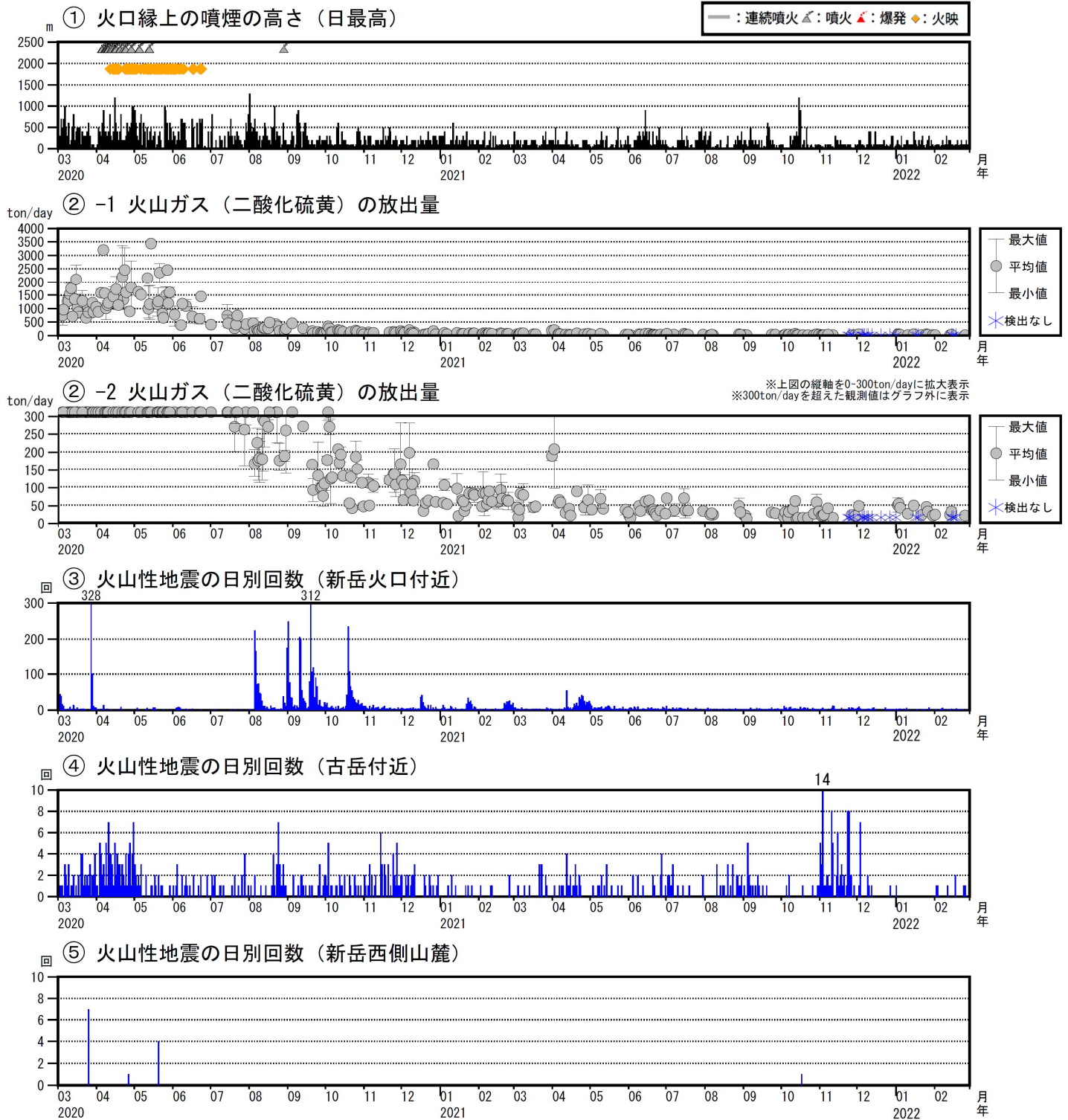
図6 口永良部島 最近の火山活動経過図（2020年3月～2022年2月）
