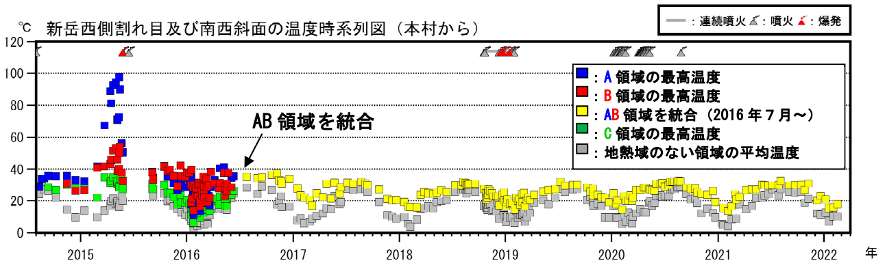
図3 口永良部島 新岳火口西側割れ目付近及び新岳南西側斜面の地熱域の温度時系列 (2014年8月～2022年2月)
