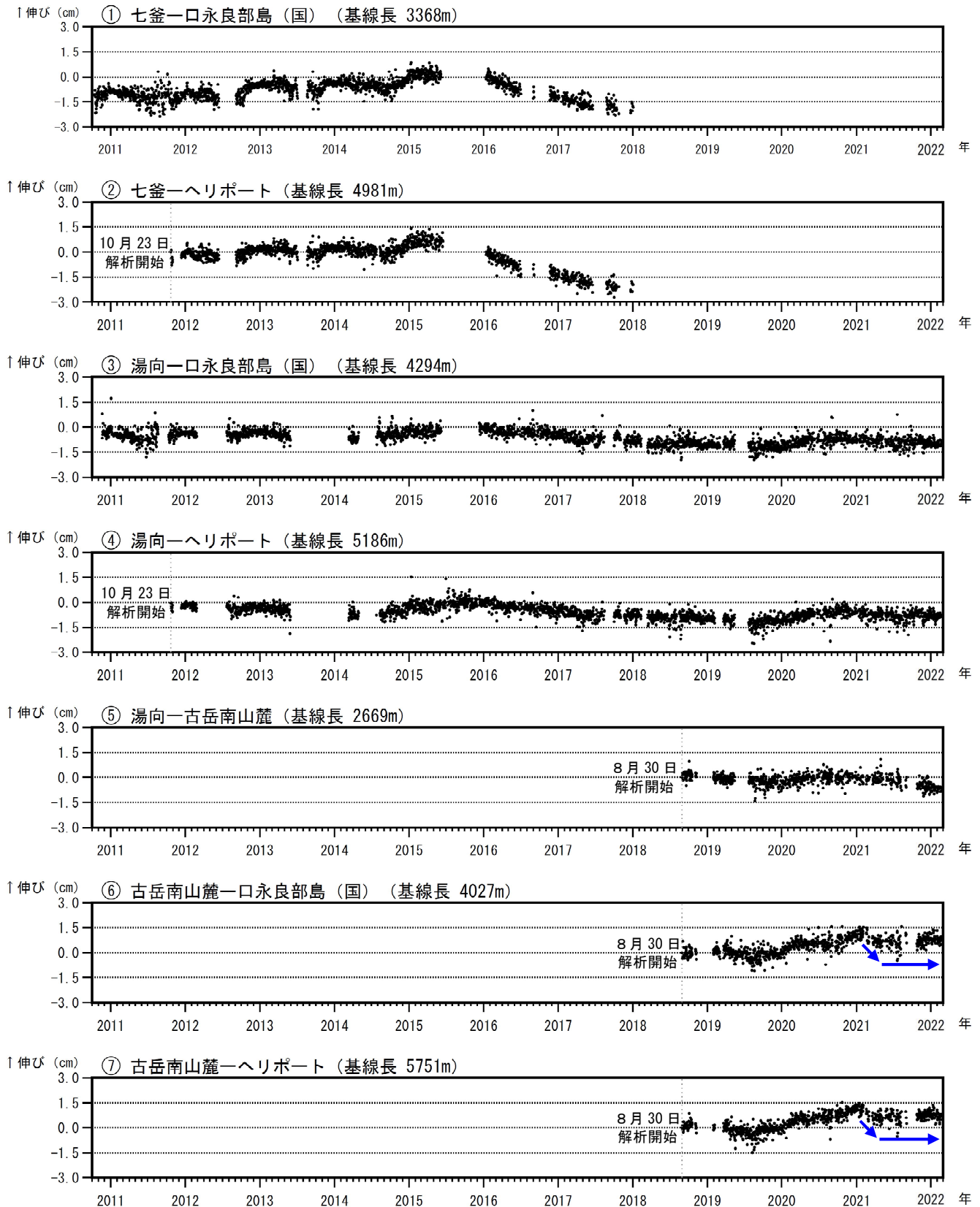
図8 口永良部島 GNSS 連続観測による基線長変化（2010年10月～2022年2月）
