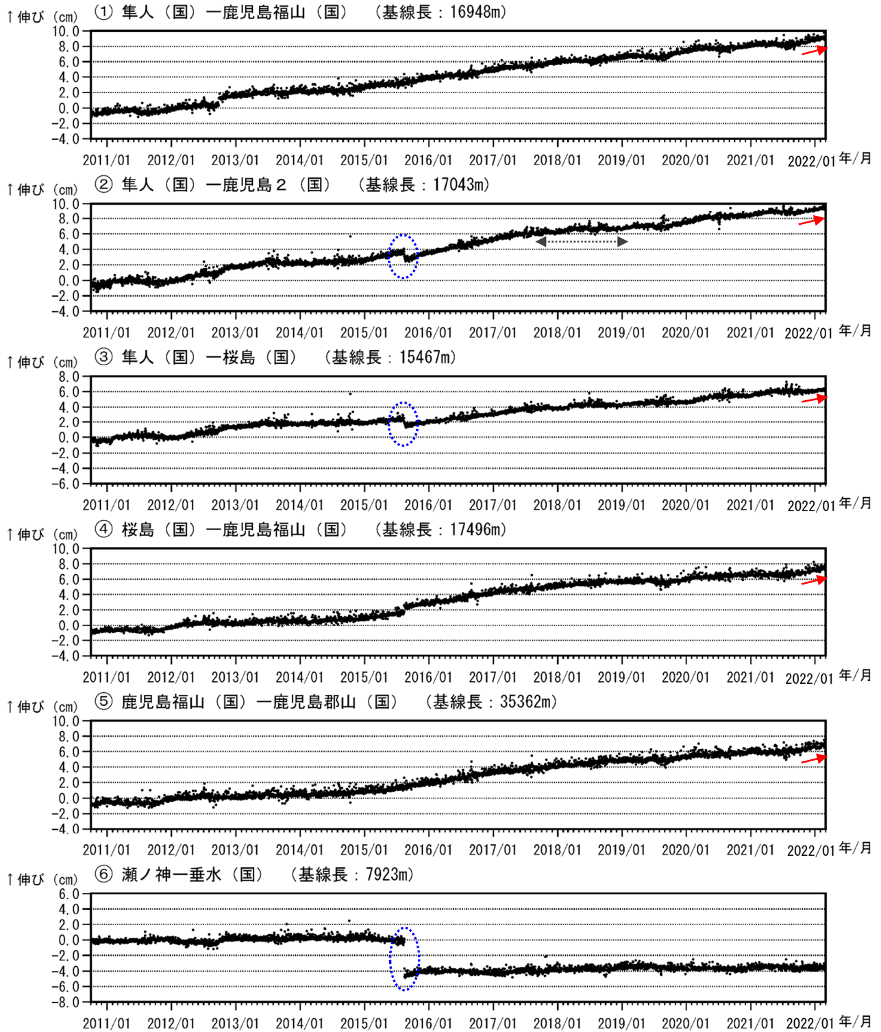
図9-1 桜島 GNSS 連続観測による基線長変化（2010年10月～2022年2月）
