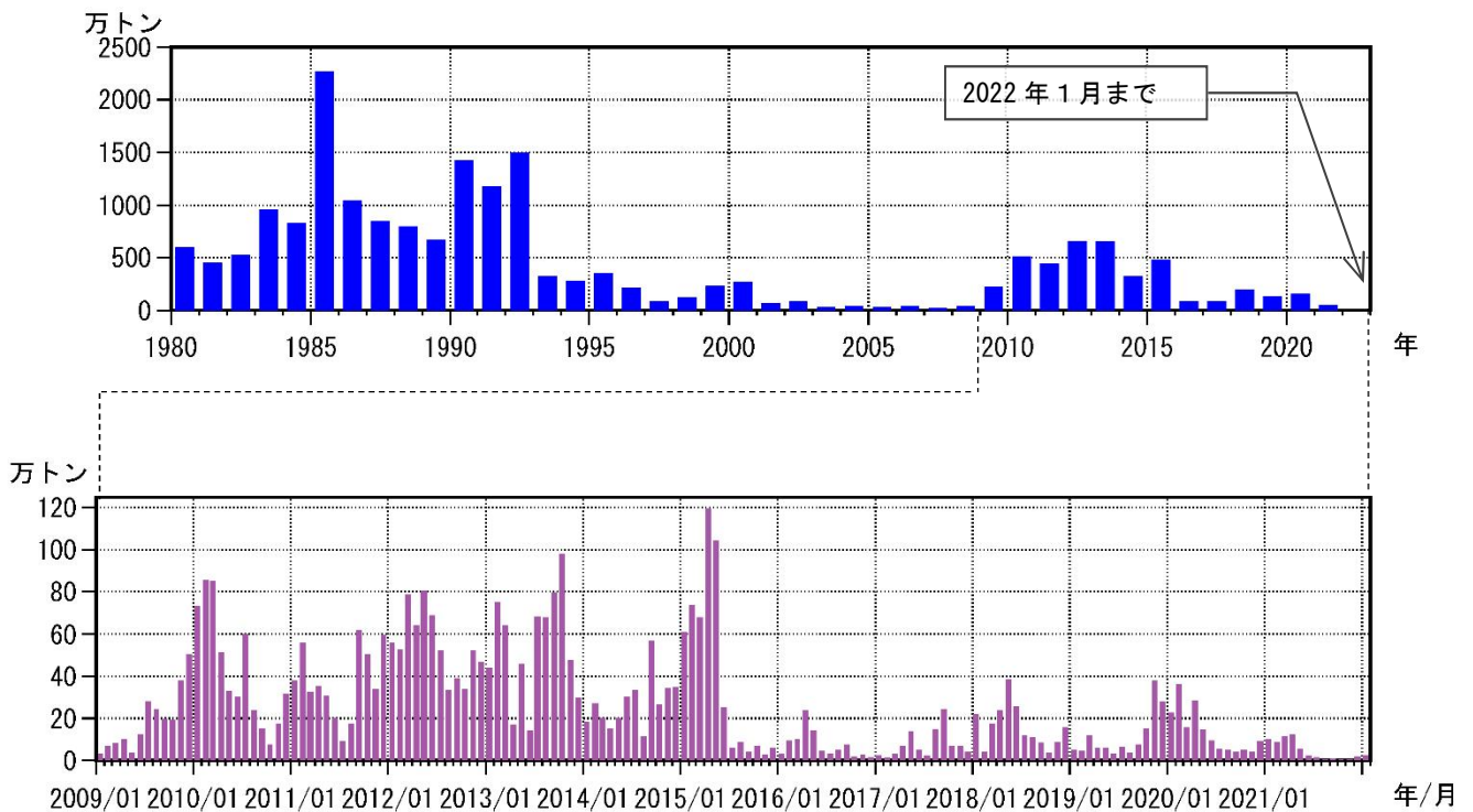
図6 桜島 鹿児島県が実施している降灰の観測データから推定した火山灰の総噴出量 （上段：1980年1月～2022年1月の年別値、下段：2009年1月～2022年1月の月別値）
