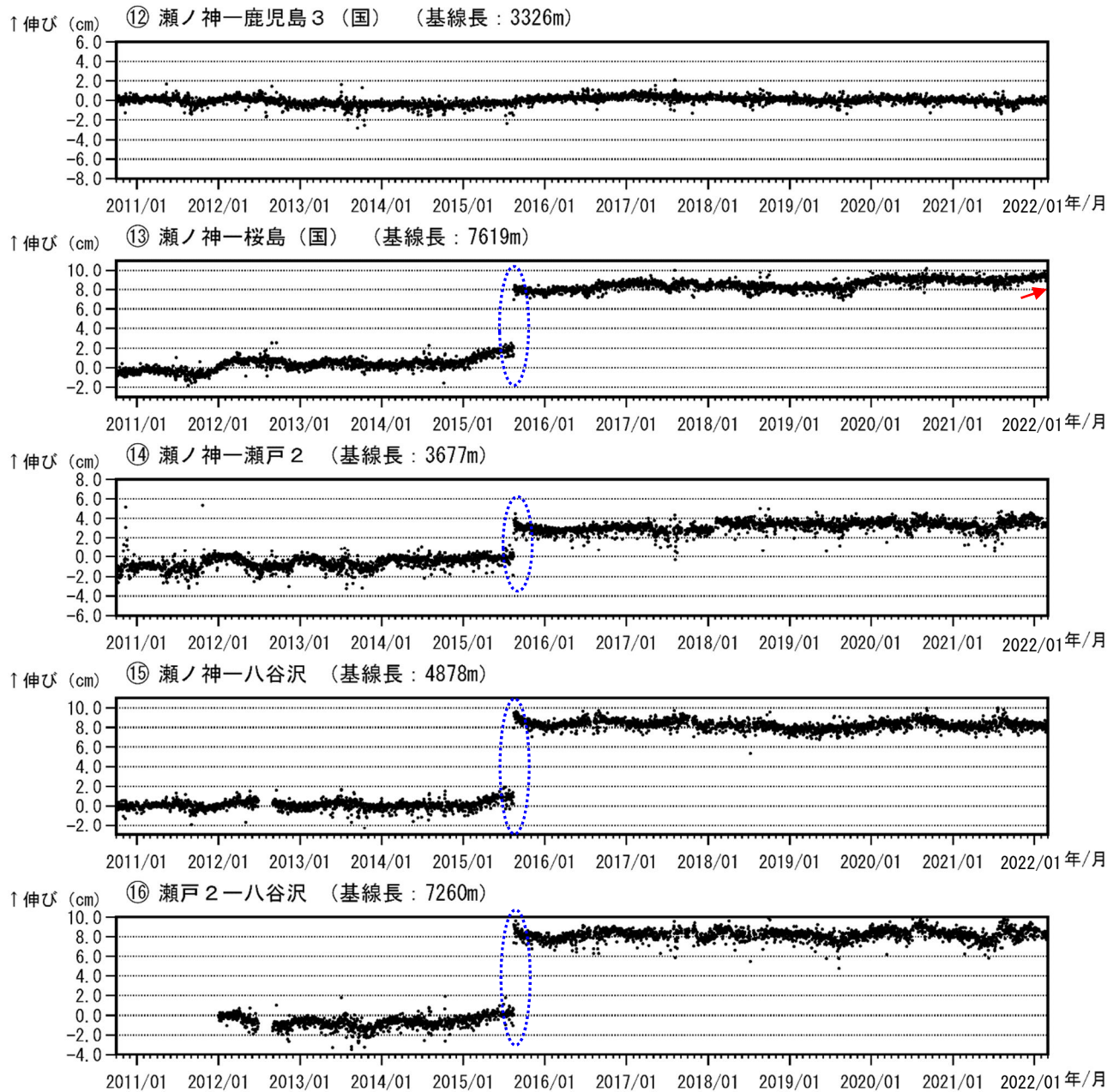
図 9-3 桜島 GNSS 連続観測による基線長変化 (2010 年 10 月～2022 年 2 月)
