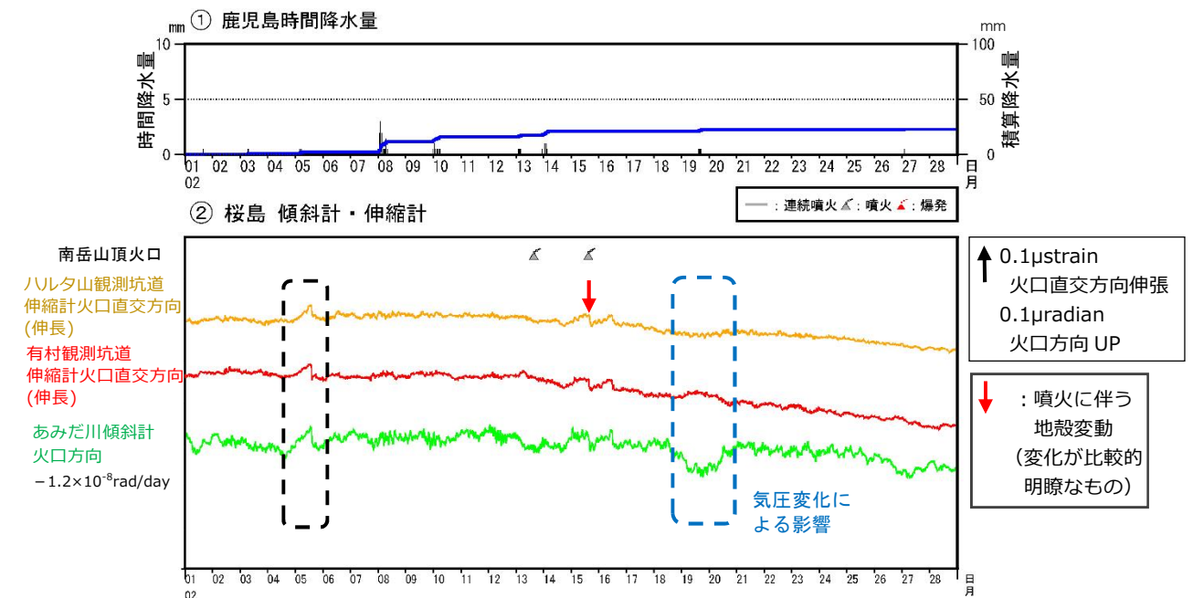
図 8-2 桜島 傾斜計及び伸縮計による地殻変動の状況（2022年2月）
