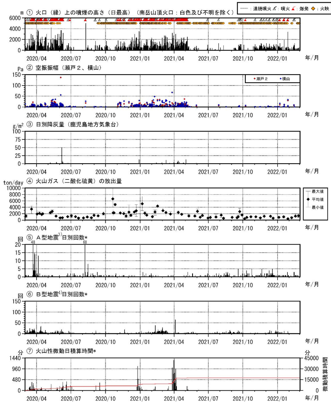
図7 桜島 最近2年間の活動経過図（2020年3月～2022年2月）
