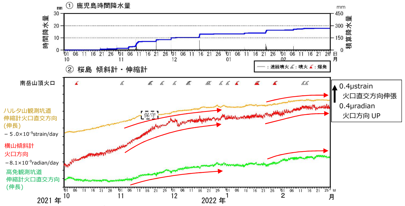
図 8-1 桜島 傾斜計及び伸縮計による地殻変動の状況（2021年10月～2022年2月）
