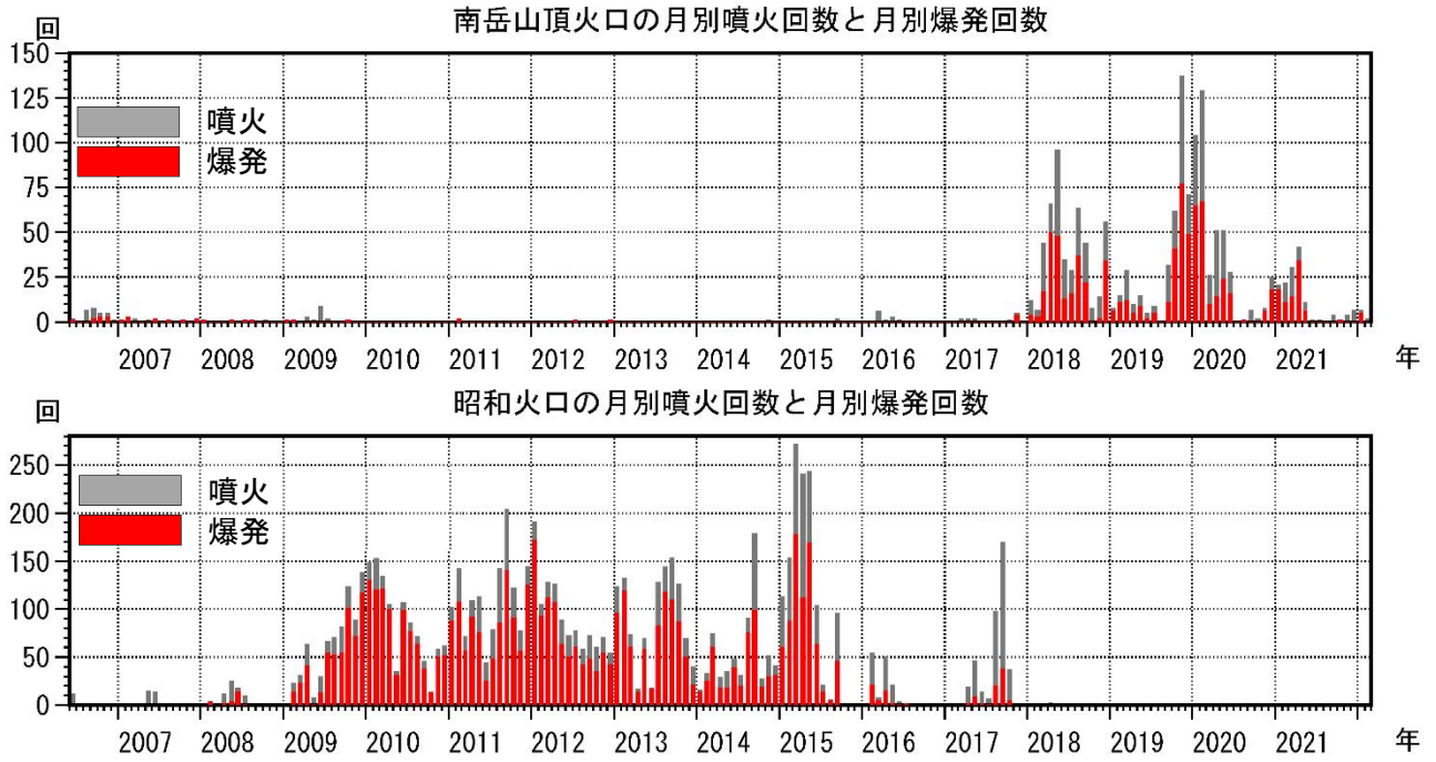
図5 桜島 南岳山頂火口（上図）と昭和火口（下図）の月別噴火回数と月別爆発回数 （2006年6月～2022年2月）
