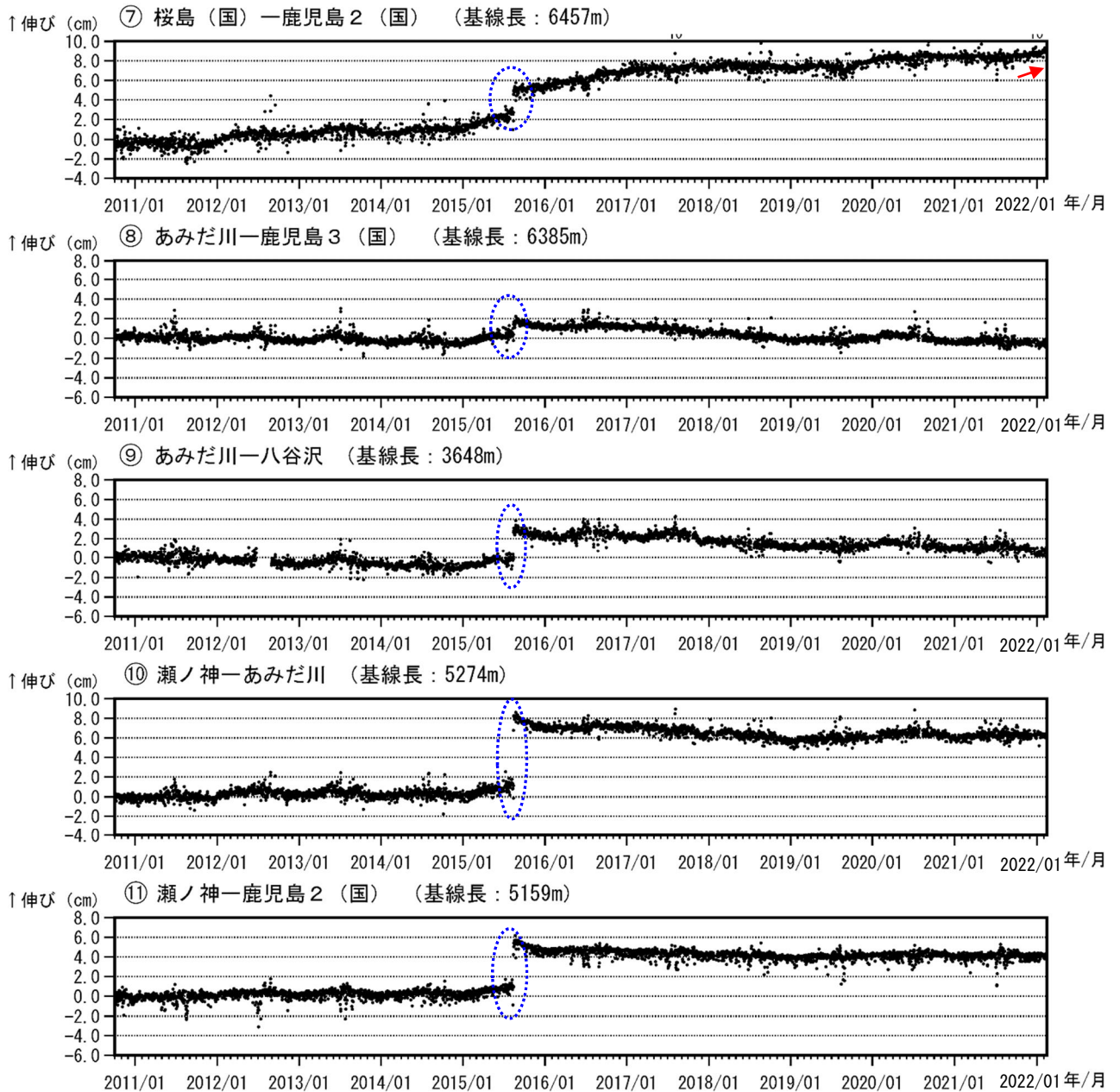
図 9-2 桜島 GNSS 連続観測による基線長変化（2010 年 10 月～2022 年 2 月）
