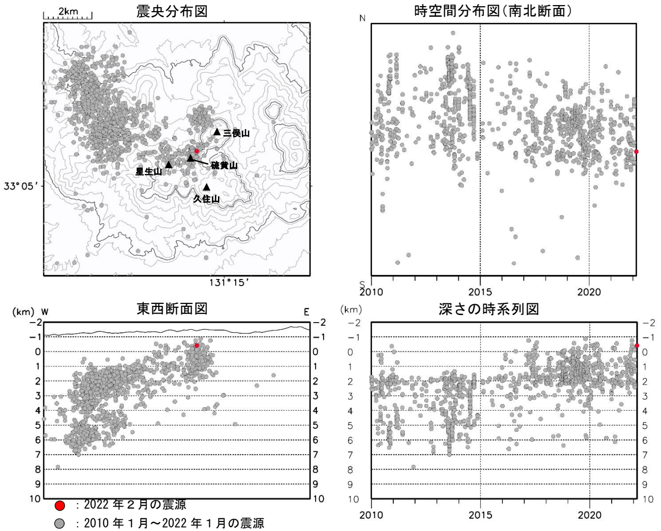
図3 九重山 震源分布図（2010年1月～2022年2月）
