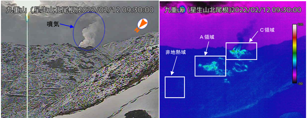
図 1-1 九重山 硫黄山の噴気及び地熱域の状況（2月12日 星生山北尾根監視カメラ）
