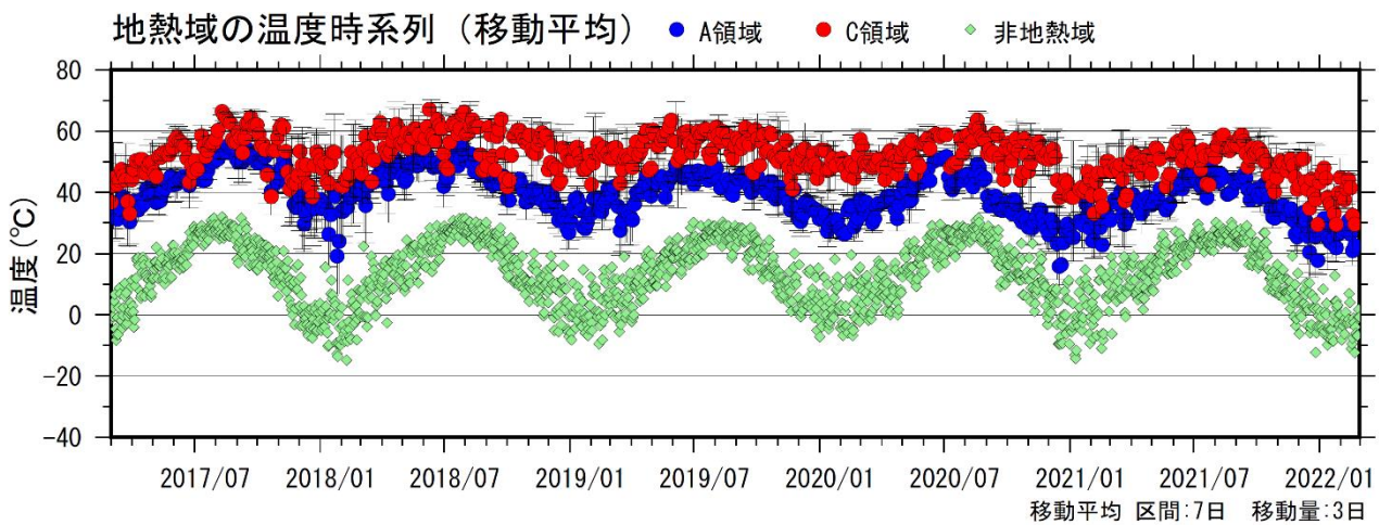
図 1-2 九重山 星生山北尾根の赤外熱映像装置による日別最高温度（2017年3月～2022年2月）
