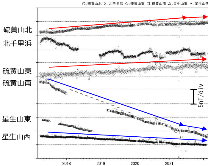
図 4-1 九重山 連続観測による全磁力の変化 (2017年3月～2022年2月)
