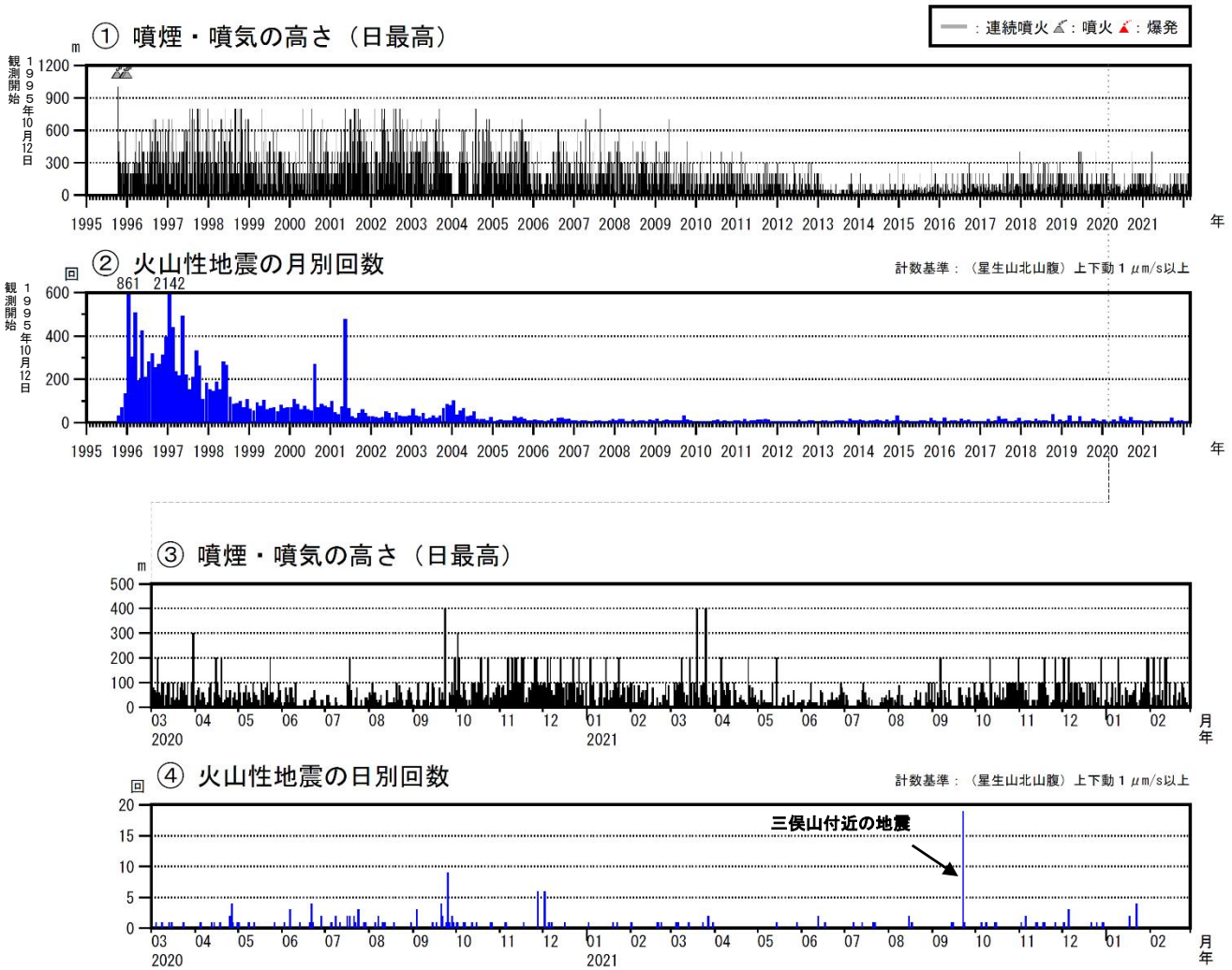
図2 九重山 火山活動経過図（1995年1月～2022年2月）
