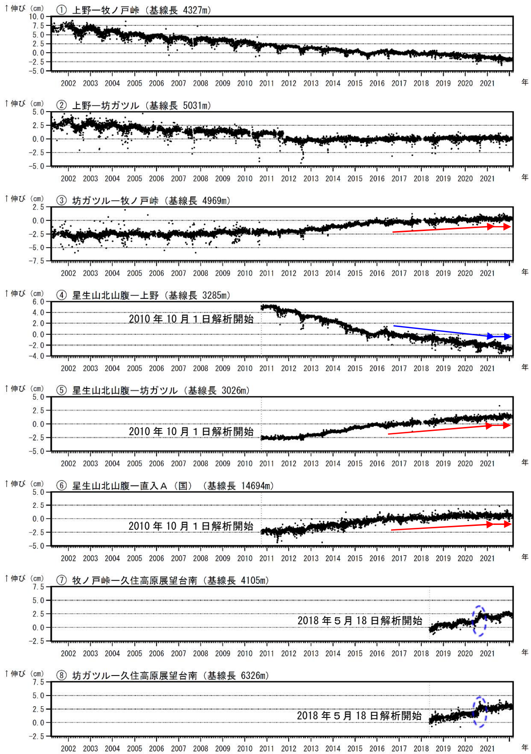
図5 九重山 GNSS 連続観測による基線長変化（2001年4月～2022年2月）
