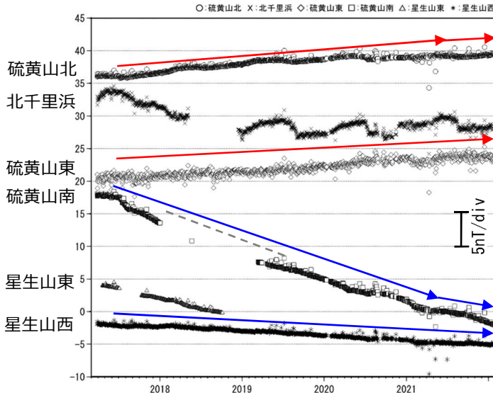
図 4-1 九重山 連続観測による全磁力の変化 (2017年3月～2022年1月)
