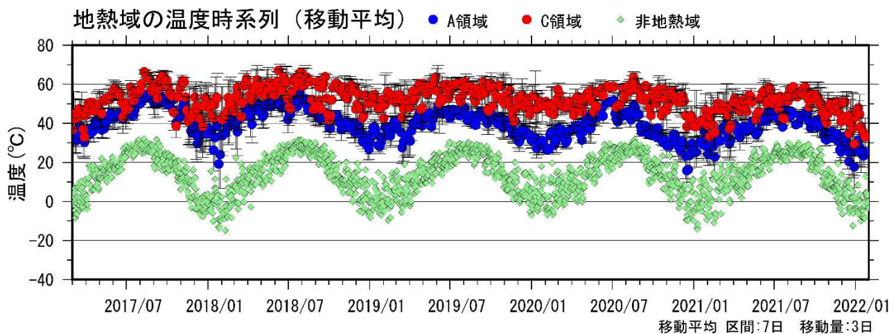
図 1-2 九重山 星生山北尾根の赤外熱映像装置による日別最高温度（2017年3月～2022年1月）
