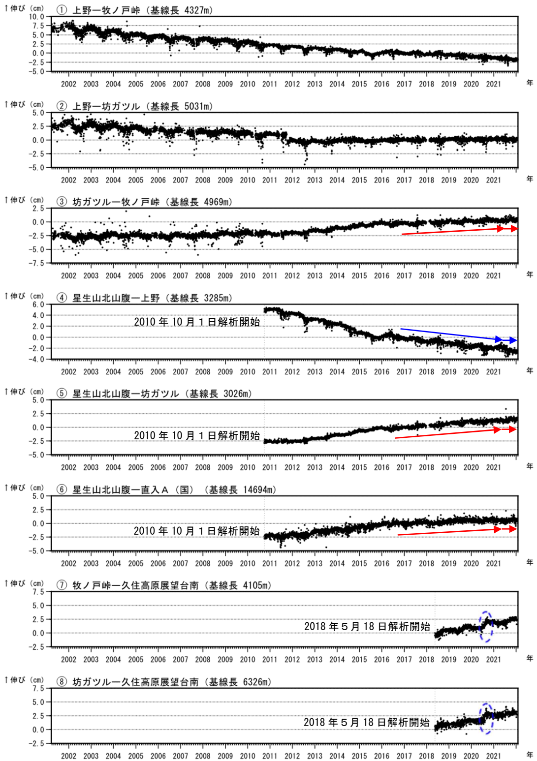
図5 九重山 GNSS 連続観測による基線長変化（2001年4月～2022年1月）
