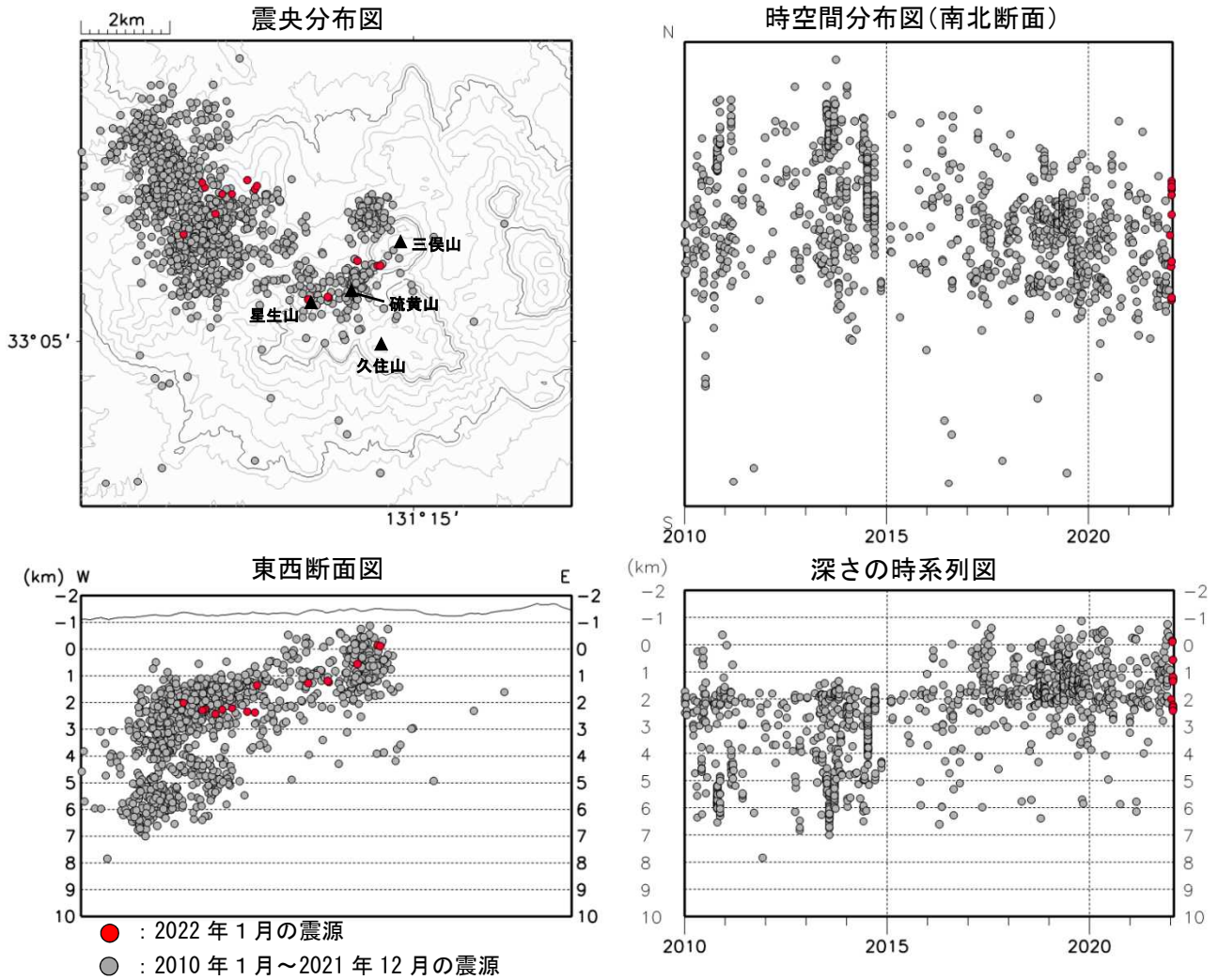
図3 九重山 震源分布図（2010年1月～2022年1月）
