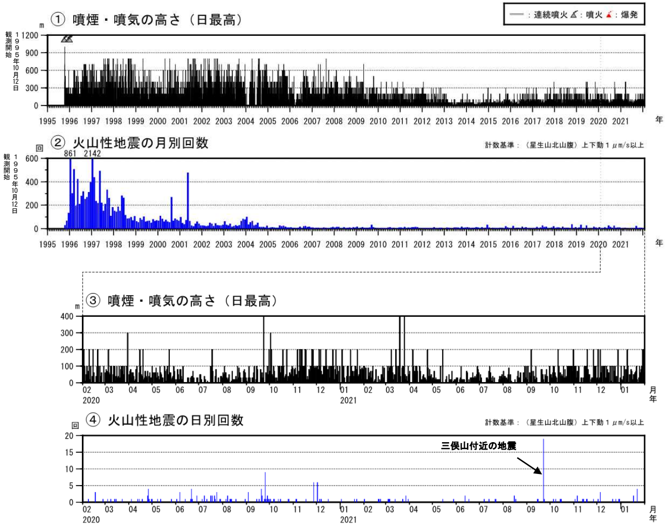
図2 九重山 火山活動経過図（1995年1月～2022年1月）
