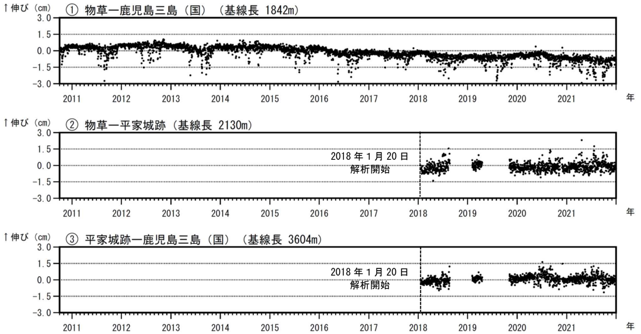
図6 薩摩硫黄島 GNSS連続観測による基線長変化 (2010年10月~2021年12月)
