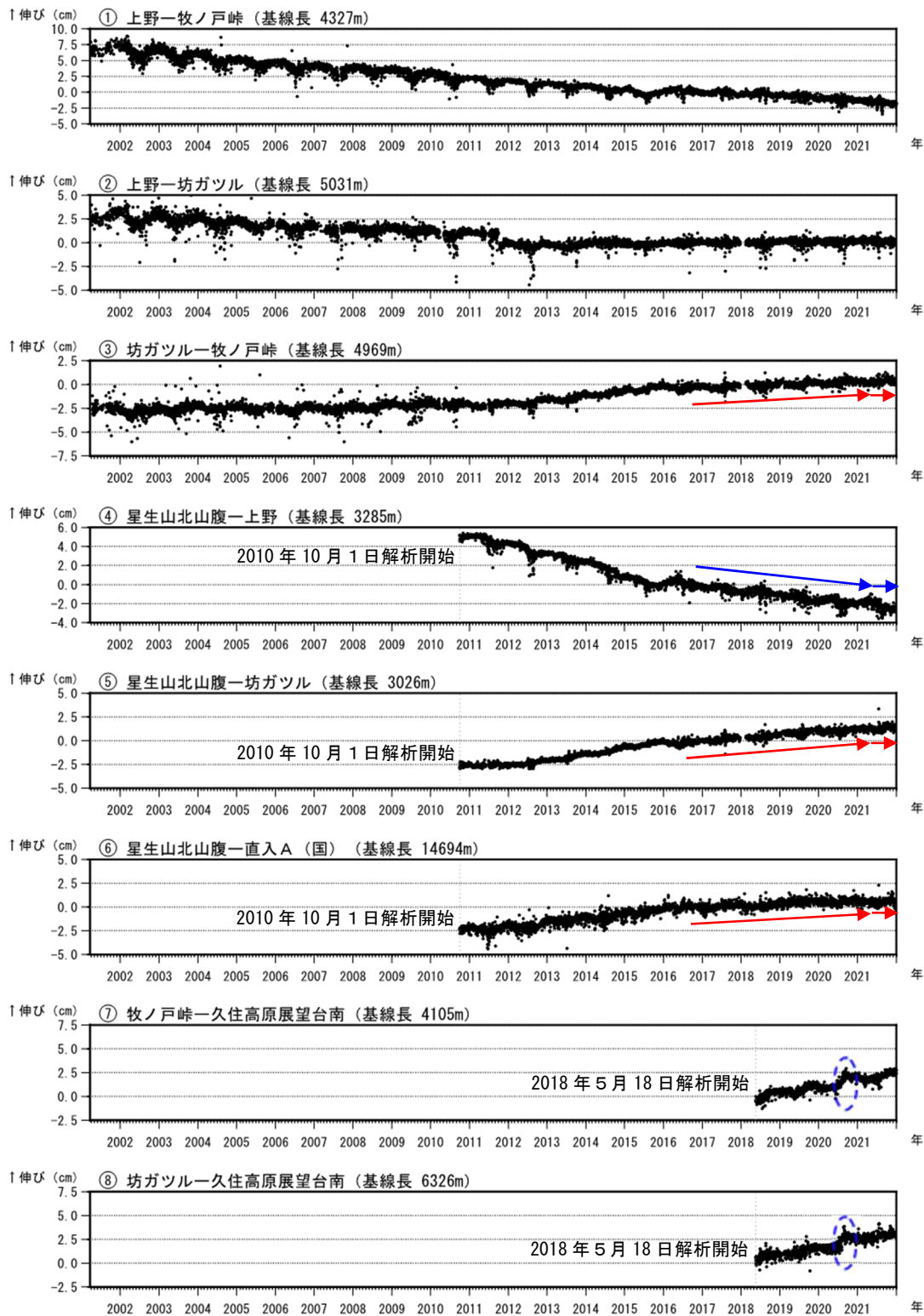
図6 九重山 GNSS 連続観測による基線長変化（2001年4月～2021年12月）
