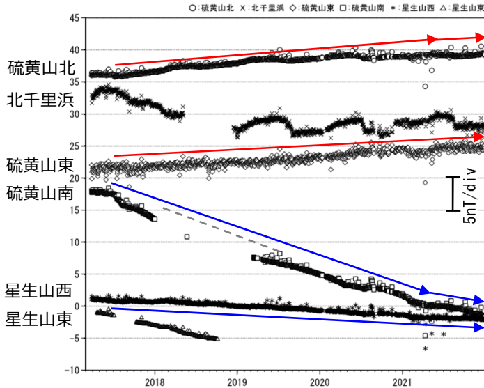
図 5-1 九重山 連続観測による全磁力の変化 (2017年3月～2021年12月)
