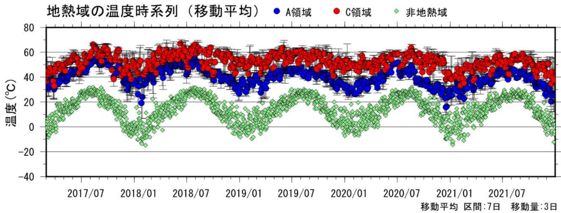
図 1-2 九重山 星生山北尾根の赤外熱映像装置による日別最高温度(2017年3月~2021年12月)
