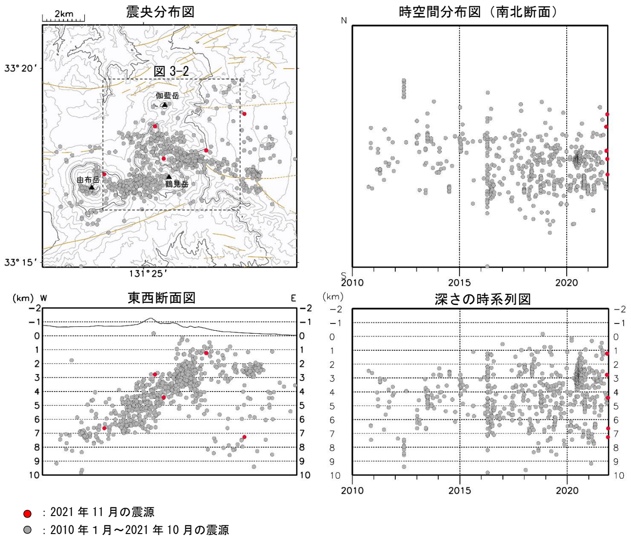
図3-1 鶴見岳・伽藍岳 震源分布図（2010年1月～2021年11月）
