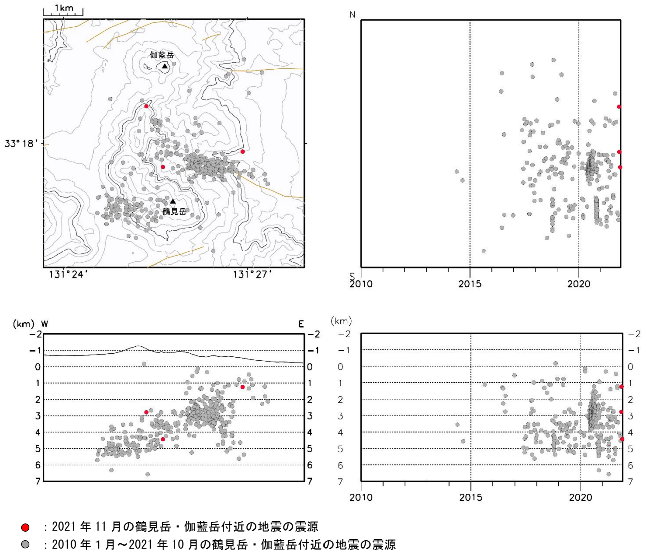
図 3-2 鶴見岳・伽藍岳 震源分布図（鶴見岳・伽藍岳付近の地震）（2010年1月～2021年11月）
