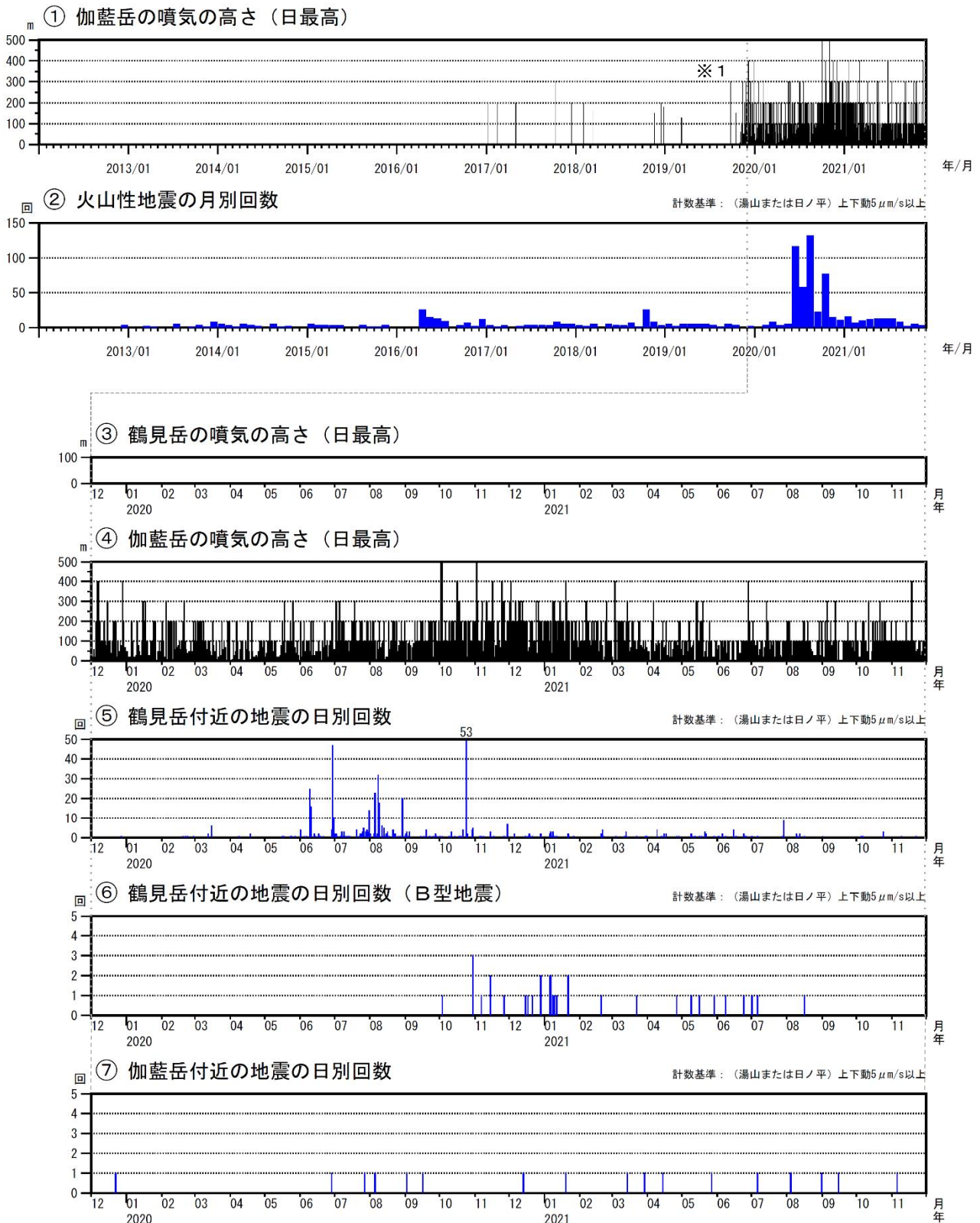
図2 鶴見岳・伽藍岳 火山活動経過図（2012年1月～2021年11月）
