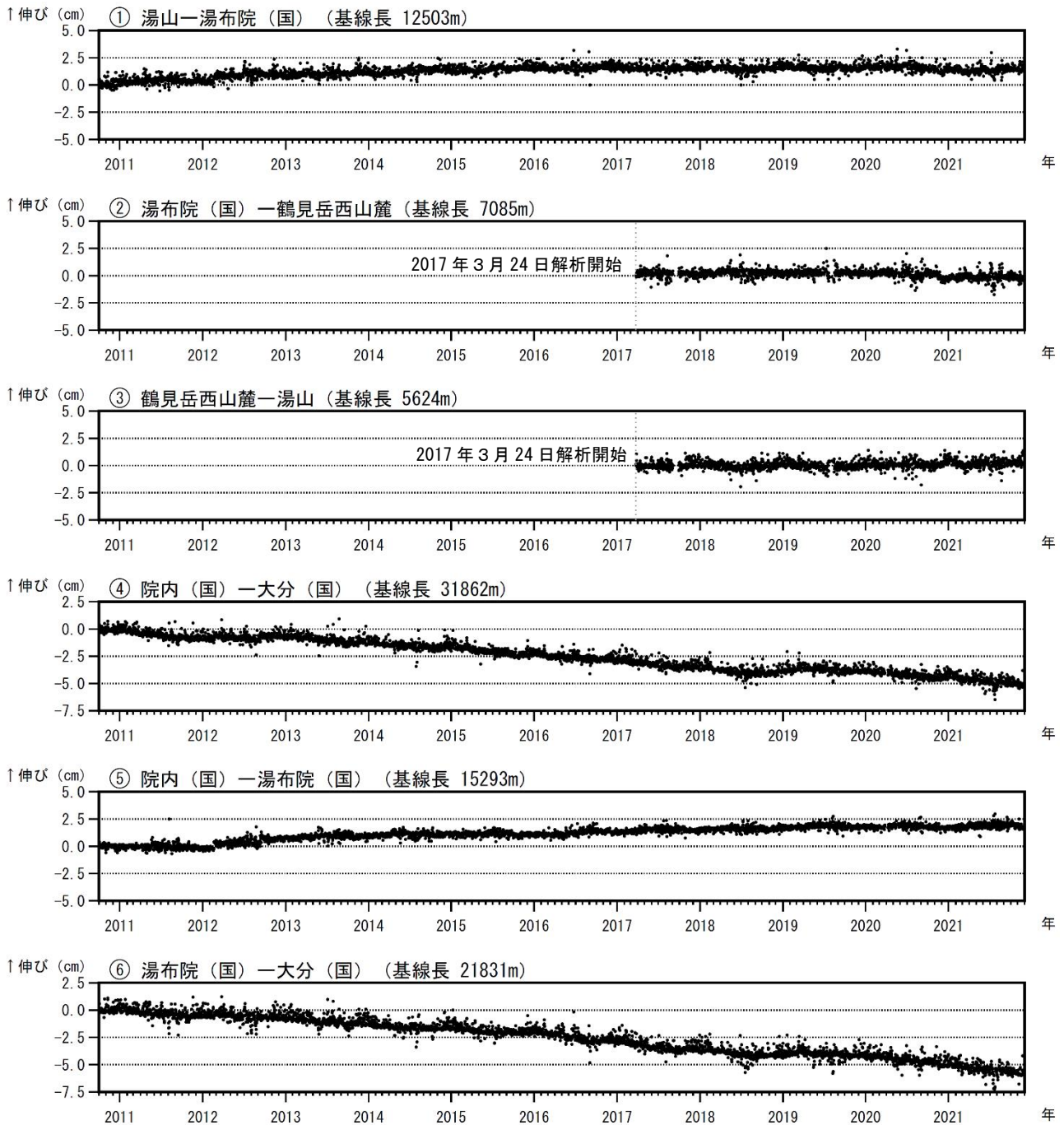
図4 鶴見岳・伽藍岳 GNSS連続観測による基線長変化（2010年10月～2021年11月）
