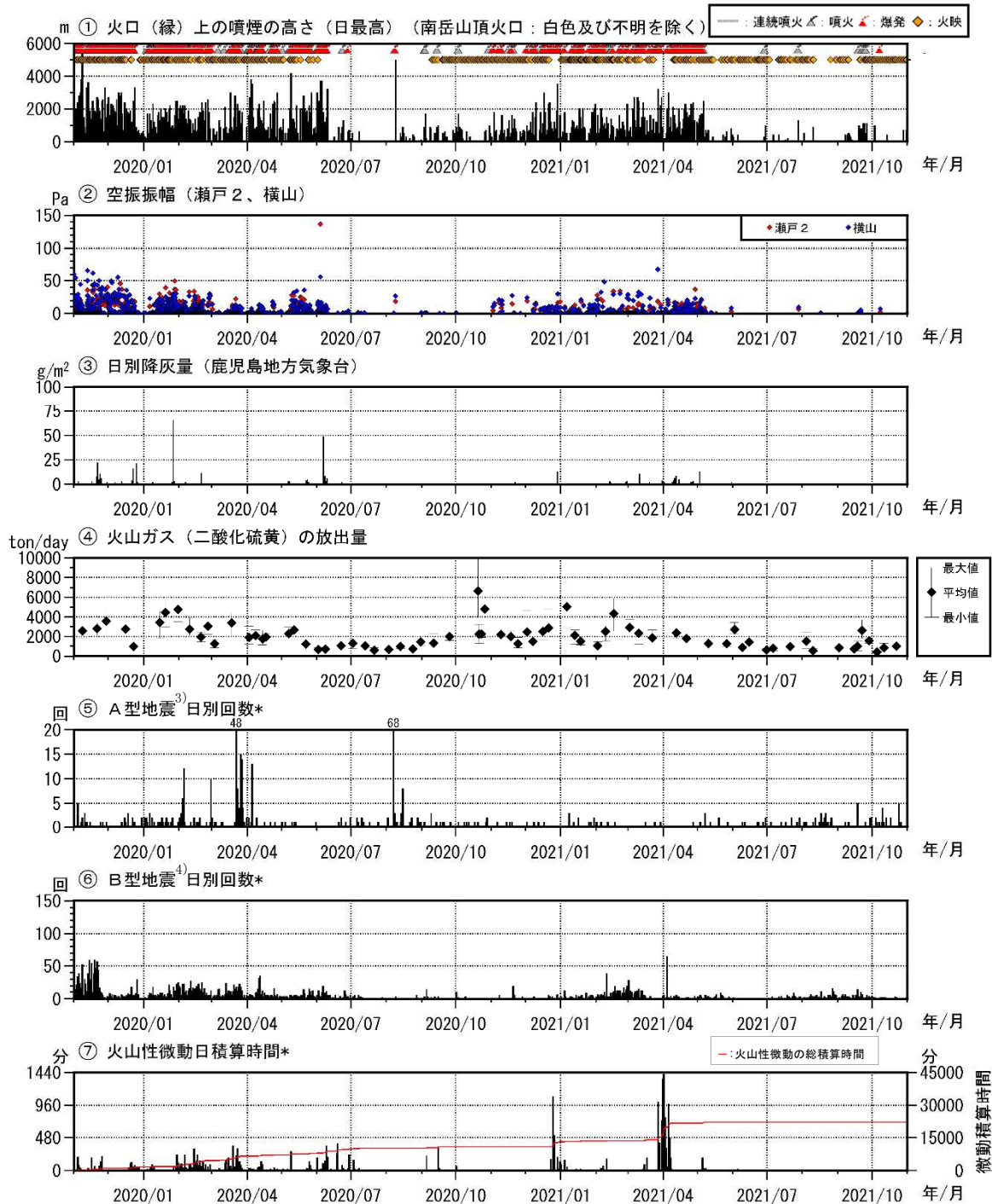
図7 桜島 最近2年間の活動経過図（2019年11月～2021年10月）
