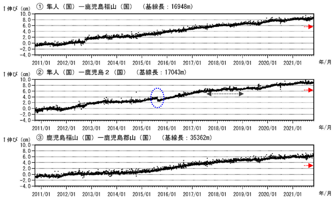
図9-1 桜島 GNSS 連続観測による基線長変化（2010年10月～2021年10月）
