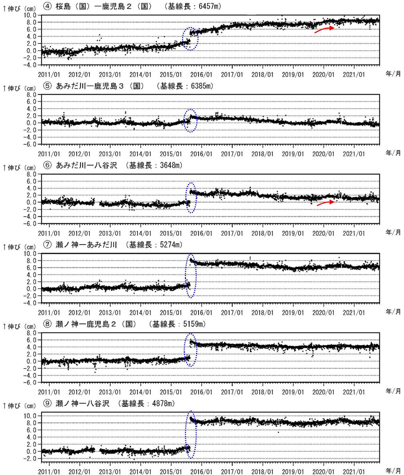
図 9-2 桜島 GNSS 連続観測による基線長変化（2010 年 10 月～2021 年 10 月）
