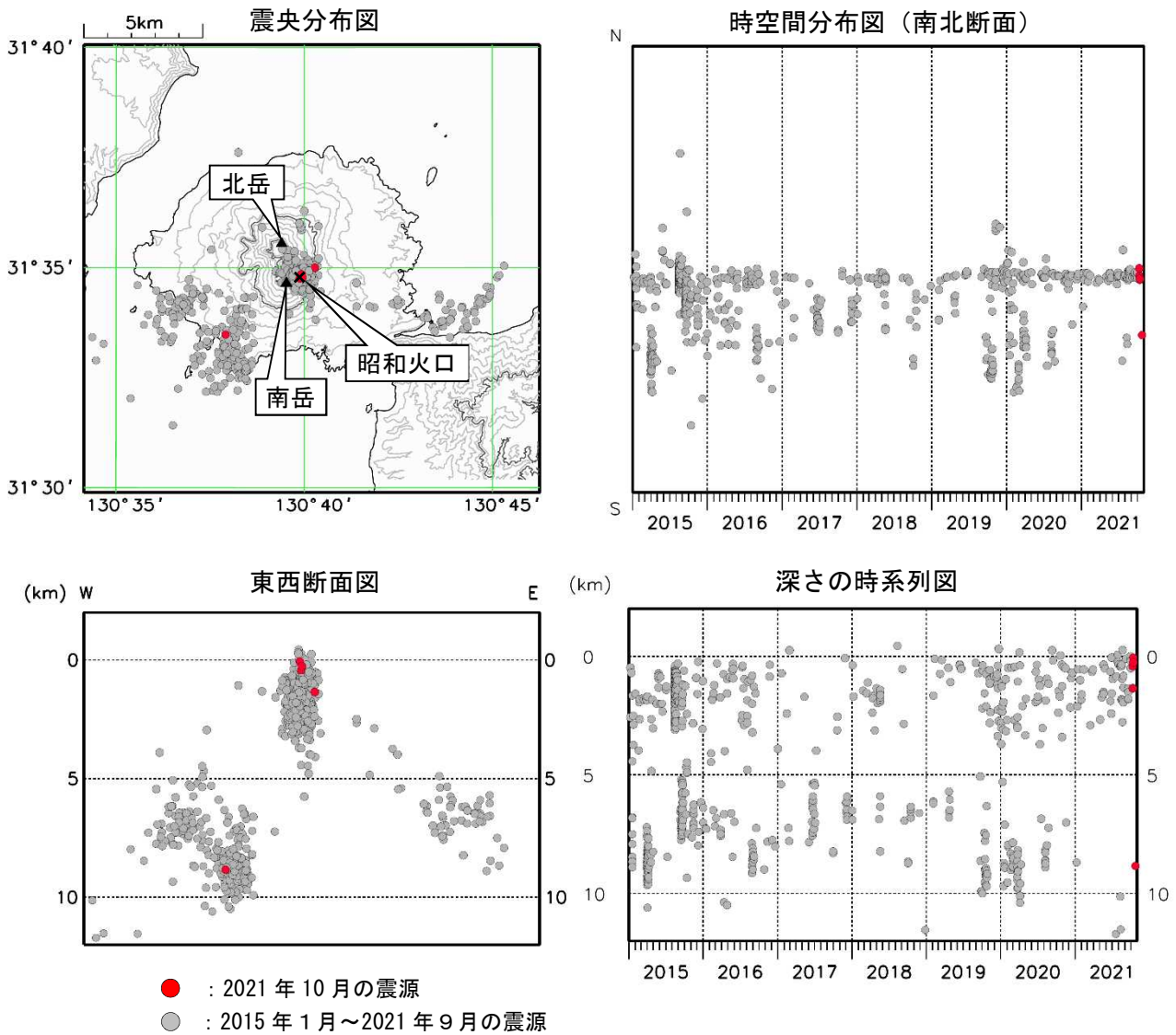
図4 桜島 震源分布図（2015年1月～2021年10月）
