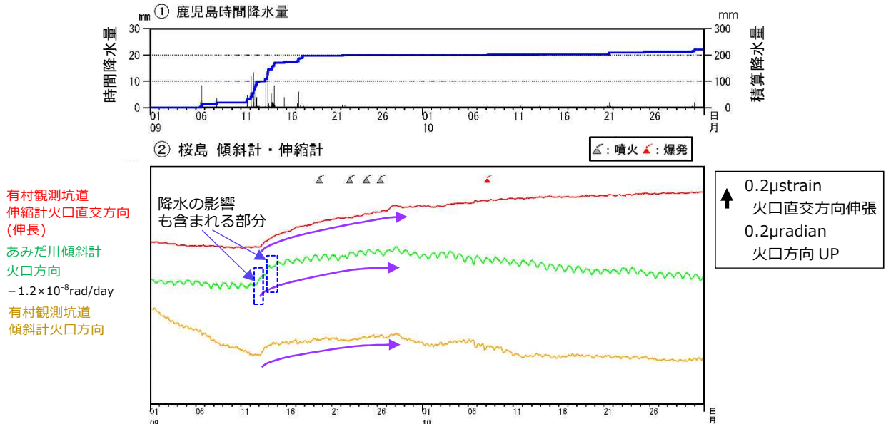
図8 桜島 傾斜計及び伸縮計による地殻変動の状況（2021年9～10月）
