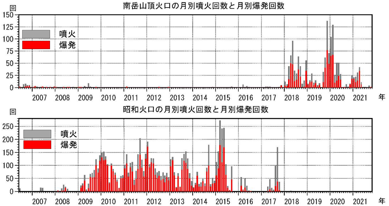
図5 桜島 南岳山頂火口（上図）と昭和火口（下図）の月別噴火回数と月別爆発回数 （2006年6月～2021年10月）
