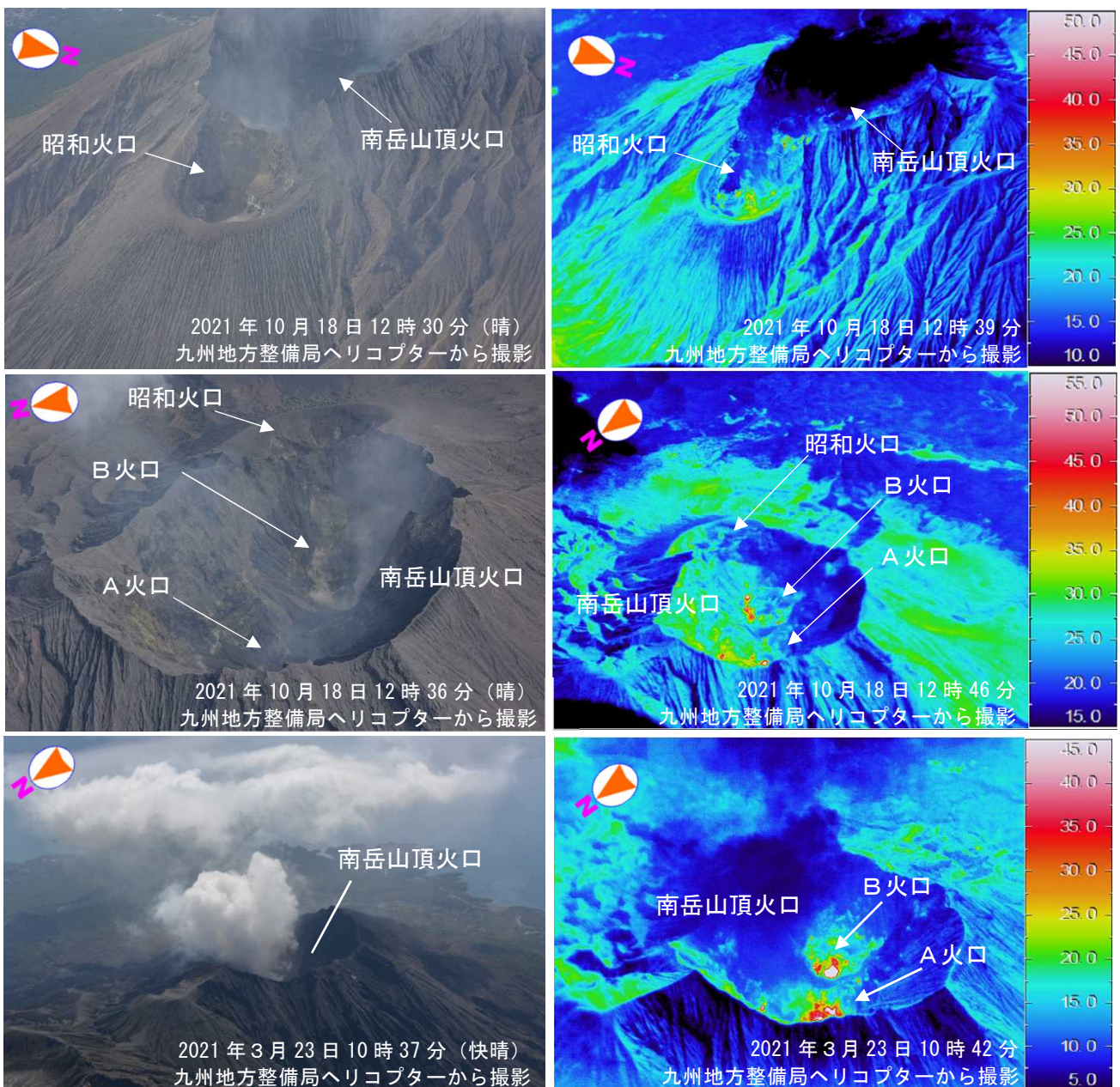
図3 桜島 上空から観測した南岳山頂火口及び昭和火口の状況
