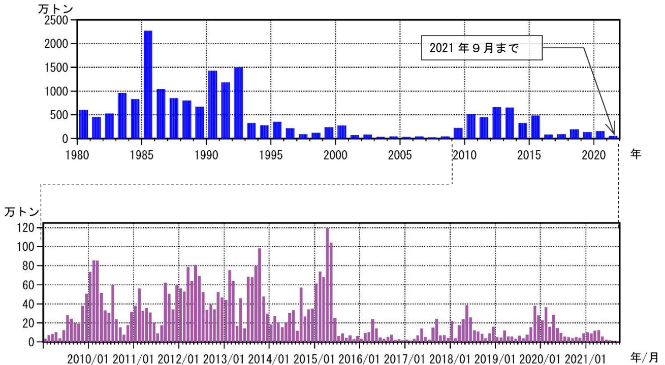
図6 桜島 鹿児島県が実施している降灰の観測データから推定した火山灰の総噴出量 （上段：1980年1月～2021年9月の年別値、下段：2009年1月～2021年9月の月別値）
