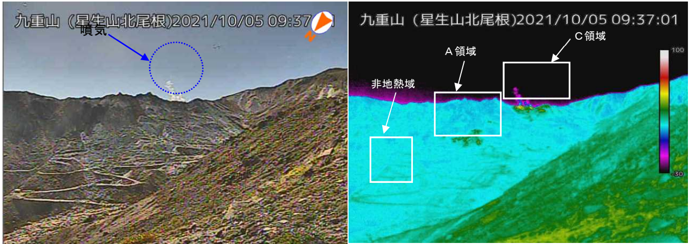
図 1-1 九重山 硫黄山の噴気及び地熱域の状況（10月5日 星生山北尾根監視カメラ）
