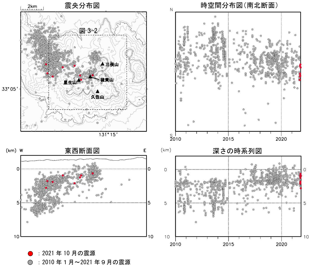
図3-1 九重山 震源分布図（2010年1月～2021年10月）
