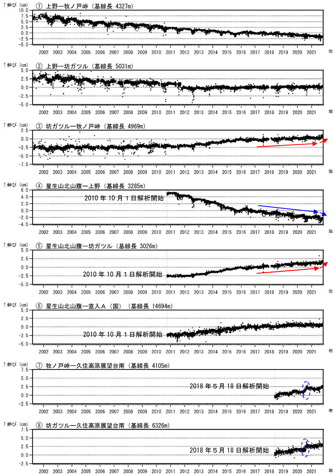
図5 九重山 GNSS 連続観測による基線長変化（2001年4月～2021年10月）
