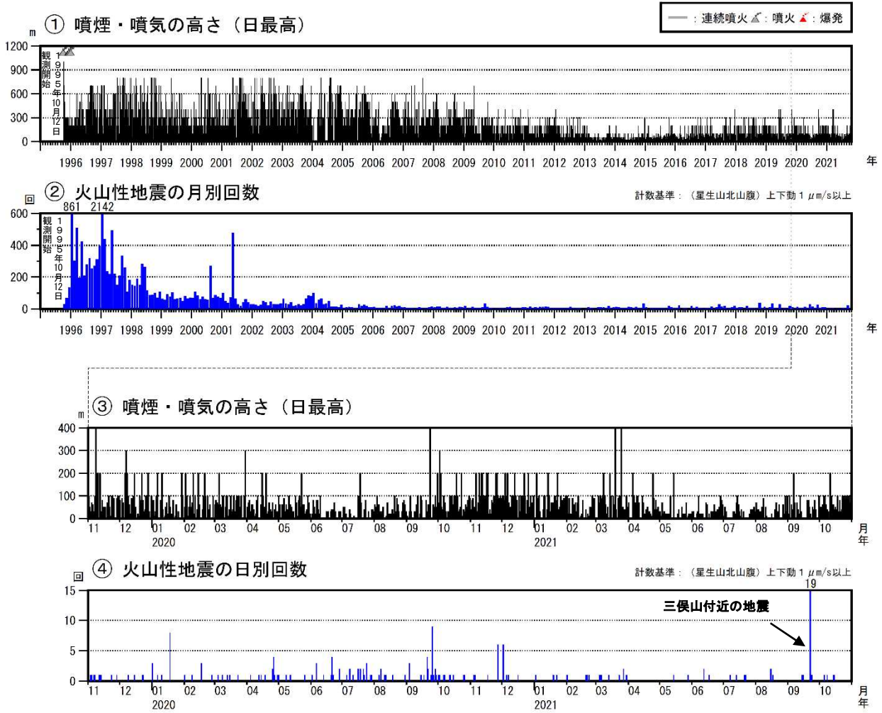
図2 九重山 火山活動経過図（1995年1月～2021年10月）
