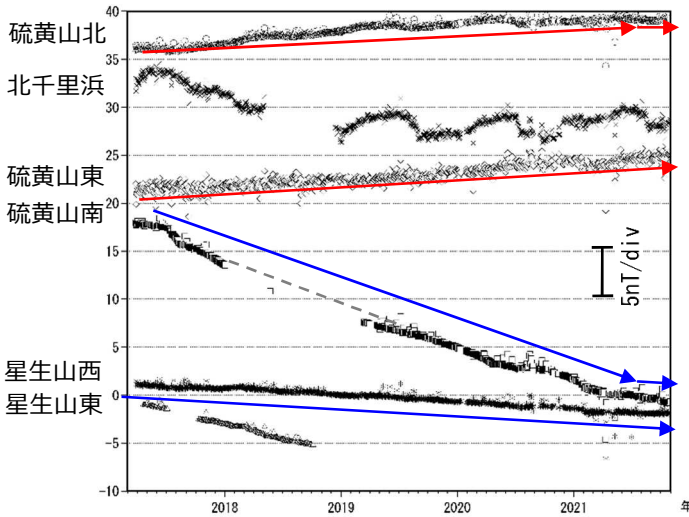
図 4-1 九重山 連続観測による全磁力の変化 (2017年3月～2021年10月)
