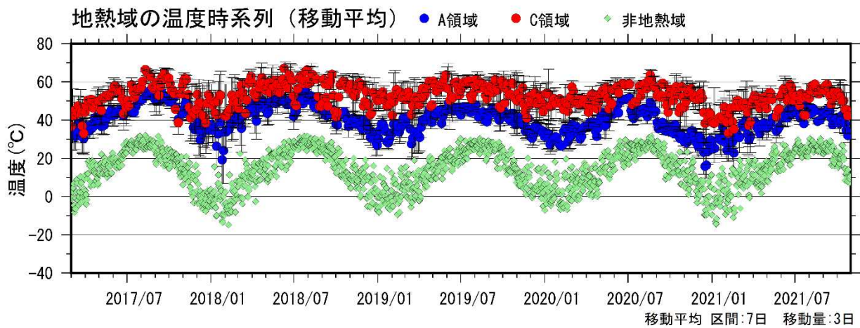
図 1-2 九重山 星生山北尾根の赤外熱映像装置による日別最高温度（2017年3月～2021年10月）
