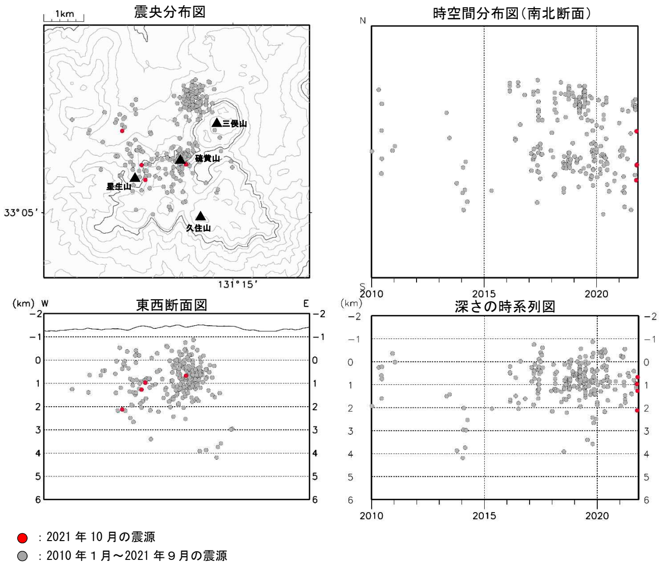
図3-2 九重山 震源分布図（硫黄山付近）（2010年1月～2021年10月）
