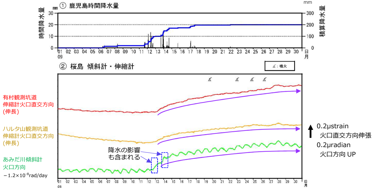
図6 桜島 傾斜計及び伸縮計による地殻変動の状況（2021年9月）
