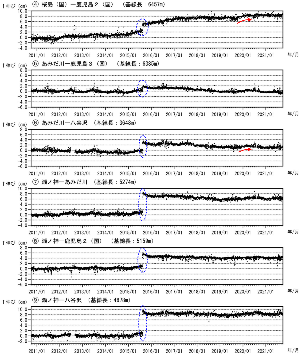
図7-2 桜島 GNSS連続観測による基線長変化（2010年10月～2021年9月）
