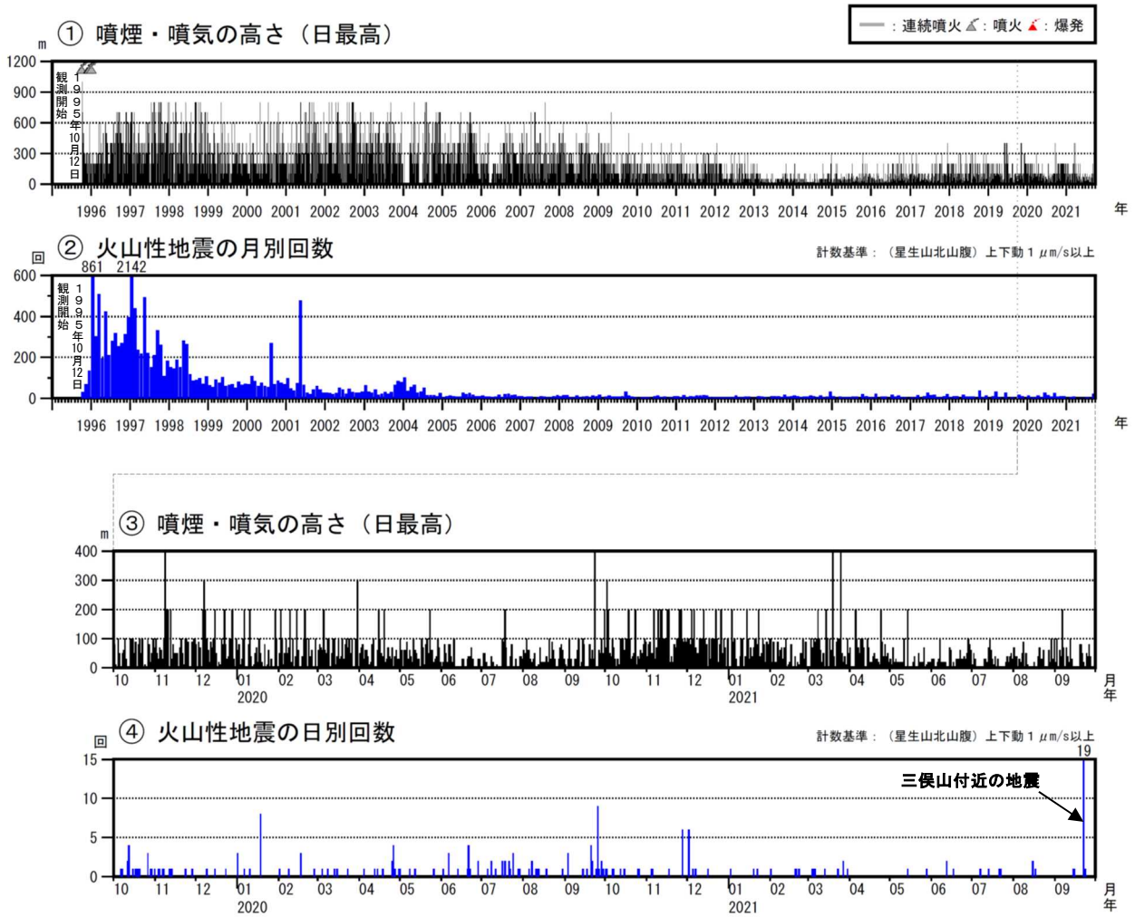
図2 九重山 火山活動経過図（1995年1月～2021年9月）
