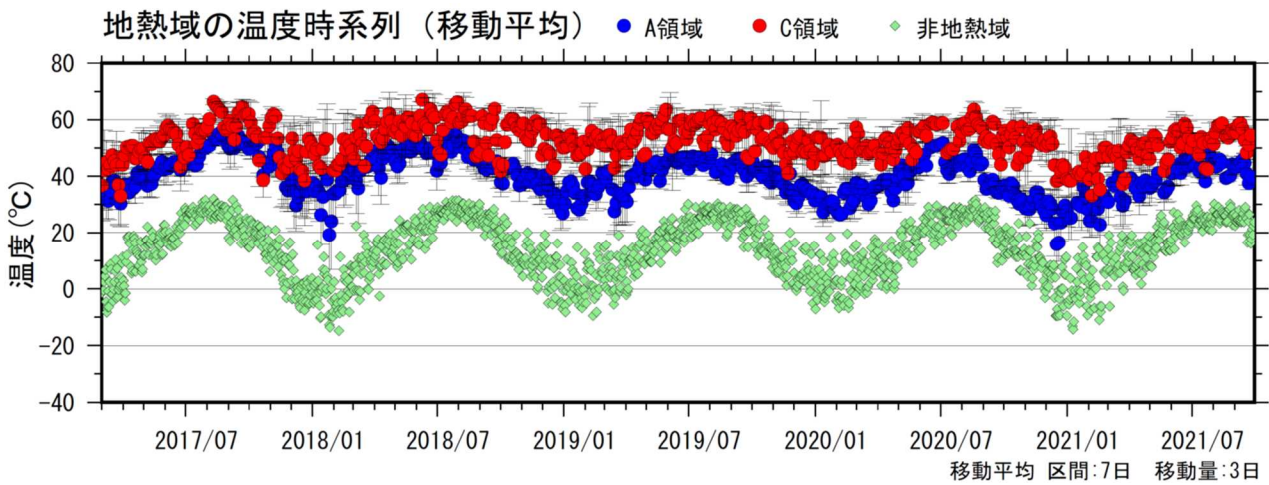
図 1-2 九重山 星生山北尾根の赤外熱映像装置による日別最高温度（2017年3月～2021年9月）
