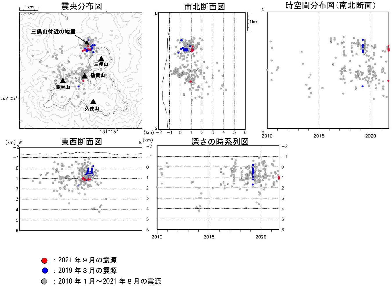
図 3-2 九重山 震源分布図（硫黄山付近）（2010年1月～2021年9月）
