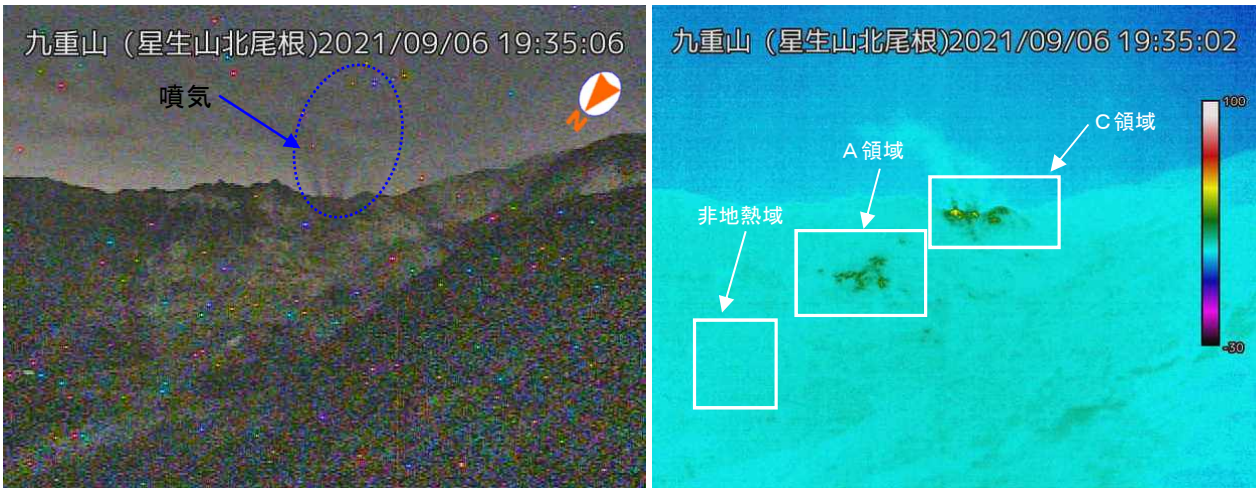
図 1-1 九重山 硫黄山の噴気及び地熱域の状況（9月6日 星生山北尾根監視カメラ）
