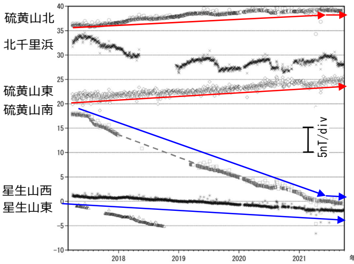
図 5-1 九重山 連続観測による全磁力の変化 (2017年3月～2021年9月)
