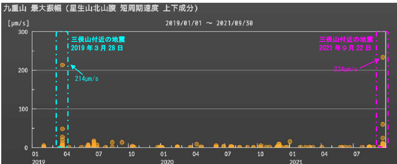
図 4-2 九重山 三俣山付近の火山性地震の最大振幅（星生山北山腹観測点 上下動成分）（2019年1月～2021年9月）
