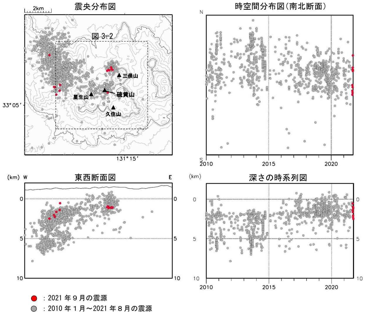
図 3-1 九重山 震源分布図（2010年1月～2021年9月）
