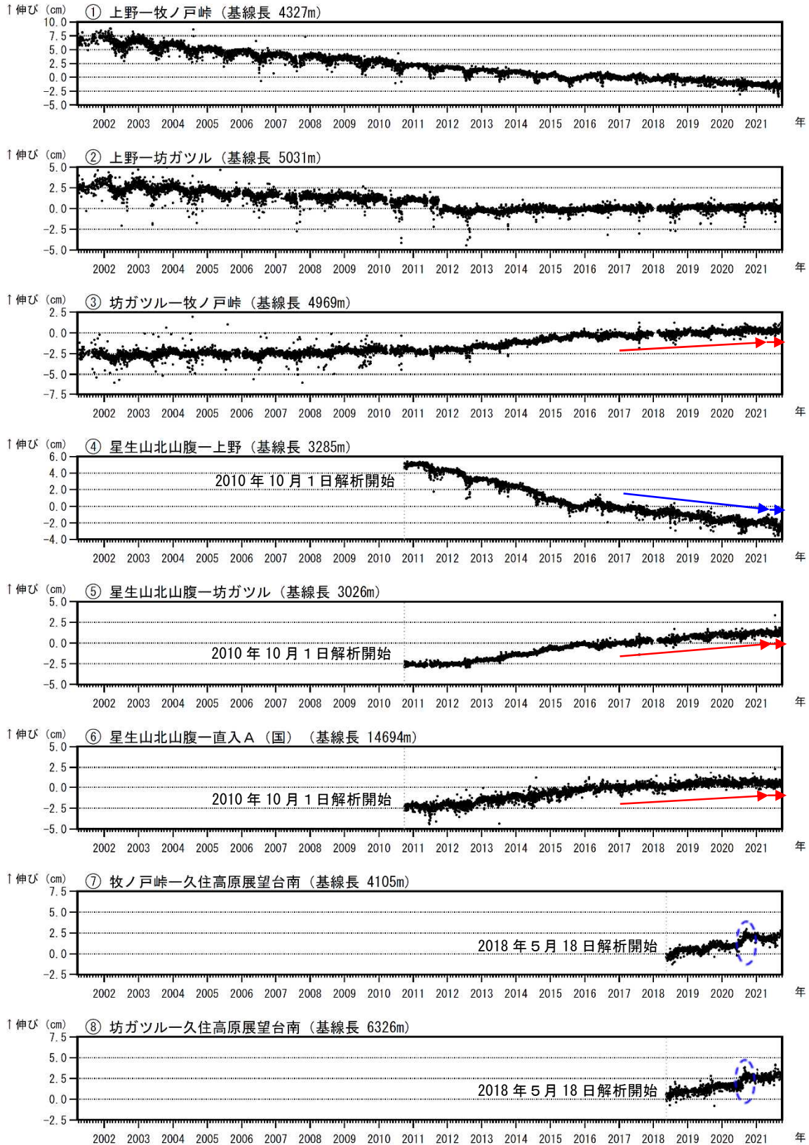
図6 九重山 GNSS連続観測による基線長変化（2001年4月～2021年9月）
