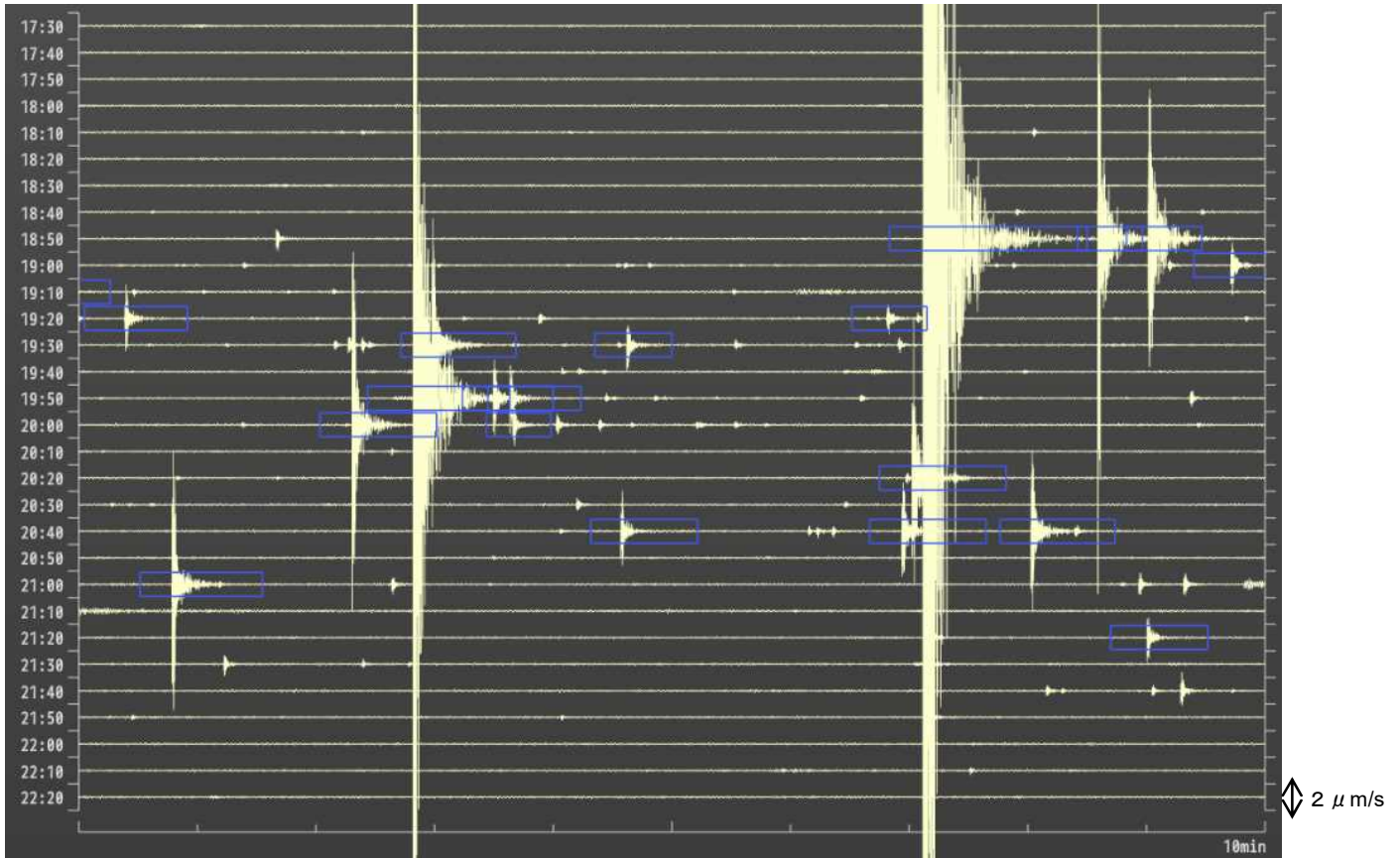
図 4-1 九重山 三俣山付近の火山性地震の最大振幅（星生山北山腹観測点 上下動成分）（2021年9月22日17時30分～22時30分）
