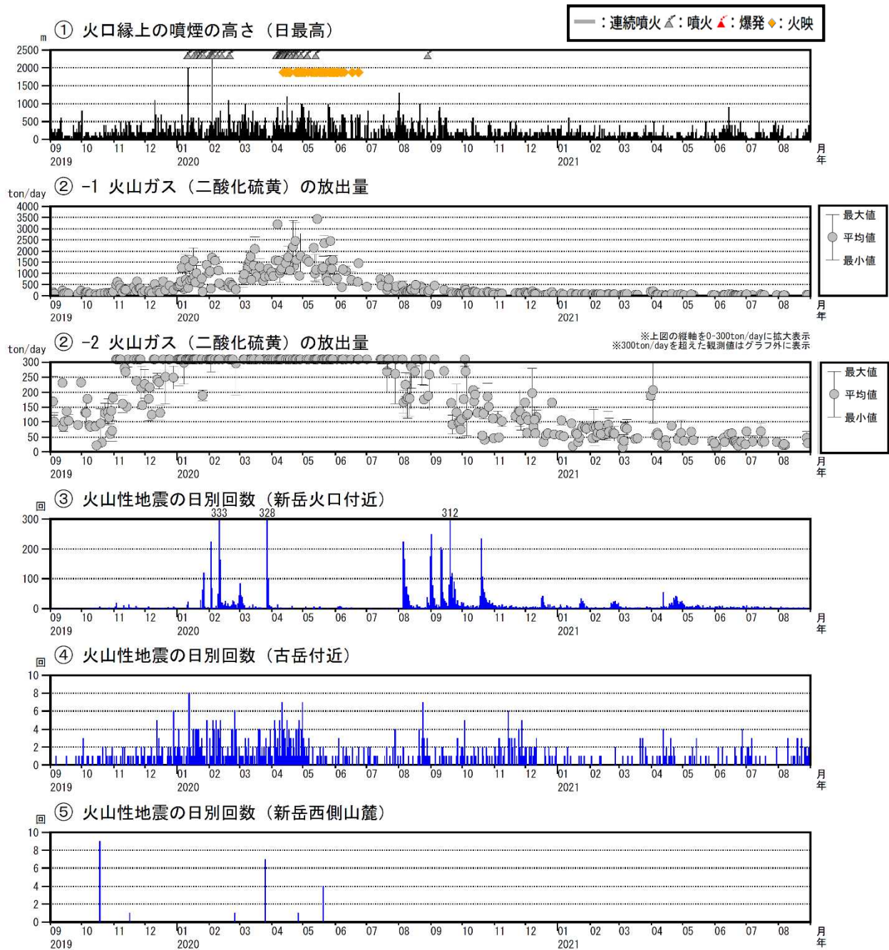
図6 口永良部島 最近の火山活動経過図（2019年9月～2021年8月）
