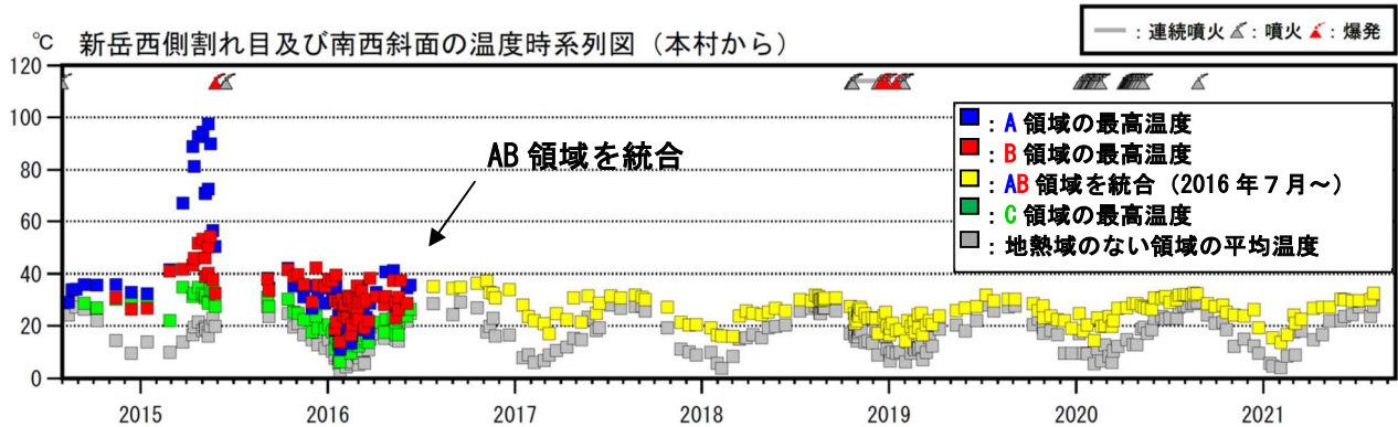
図3 口永良部島 新岳西斜面及び新岳南西側斜面の地熱域の温度時系列(2014年8月～2021年8月)
