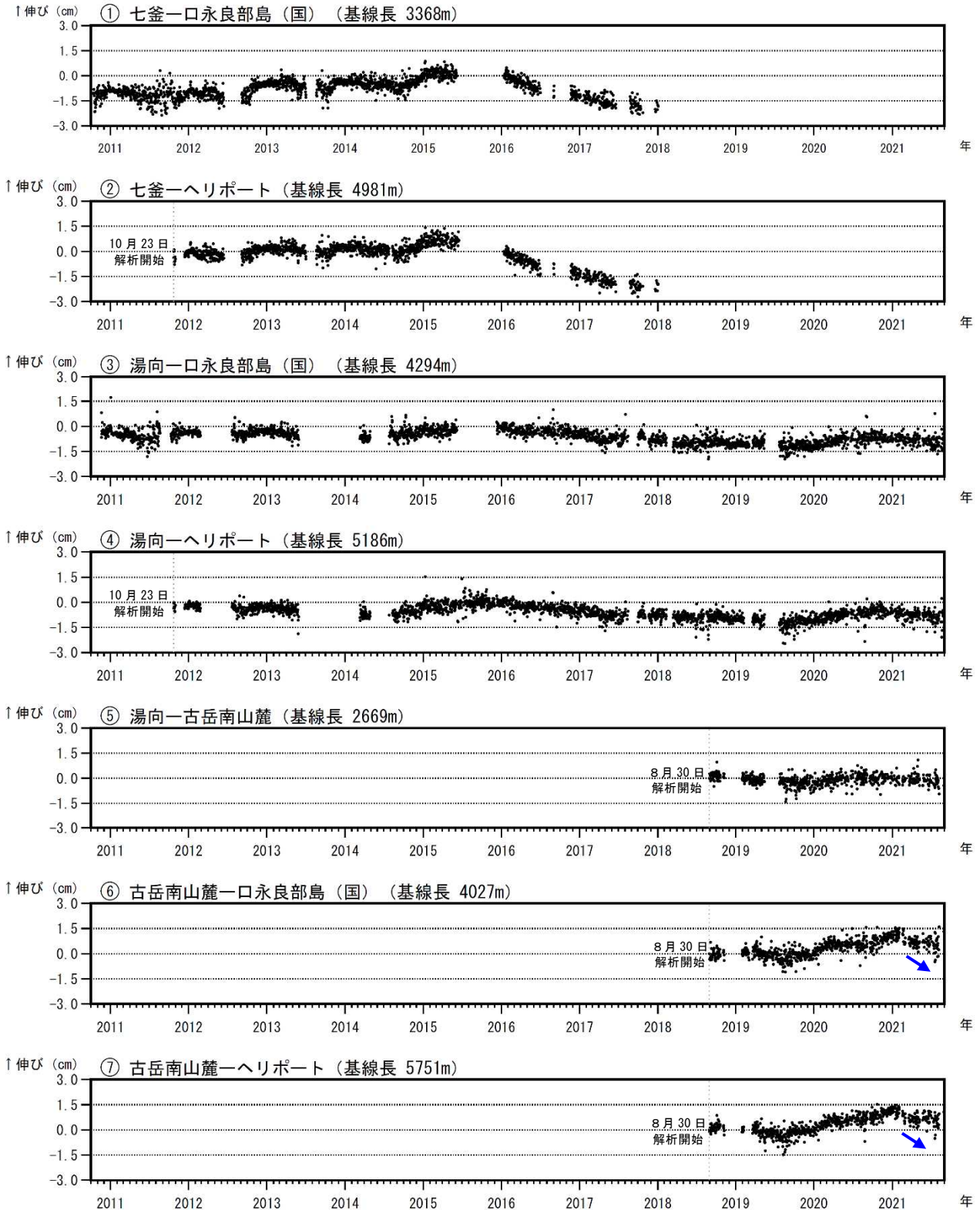
図8 口永良部島 GNSS 連続観測による基線長変化（2010年10月～2021年8月）
