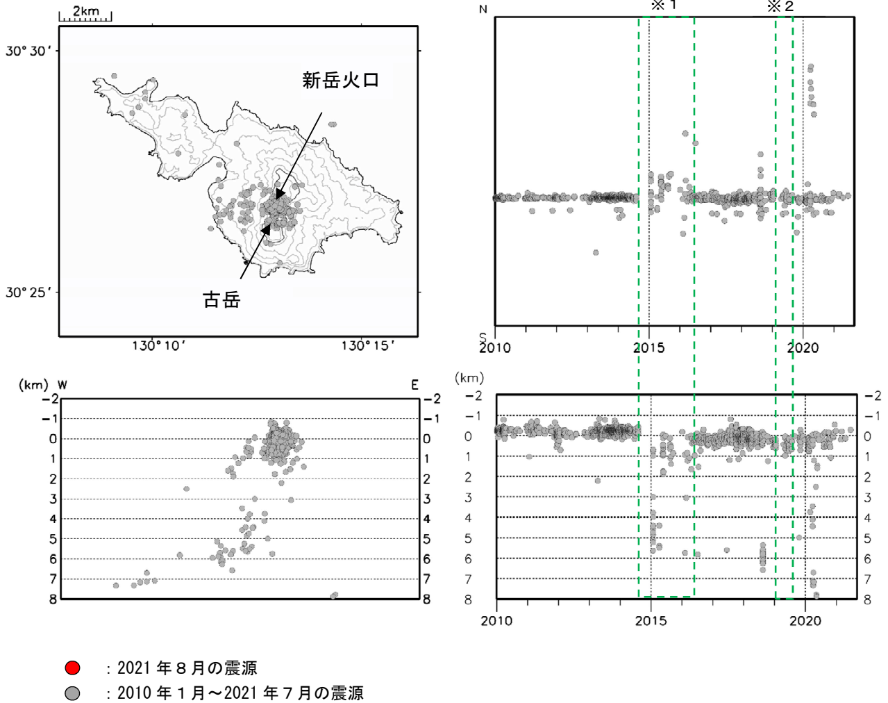
図7 口永良部島 震源分布図（2010年1月～2021年8月）
