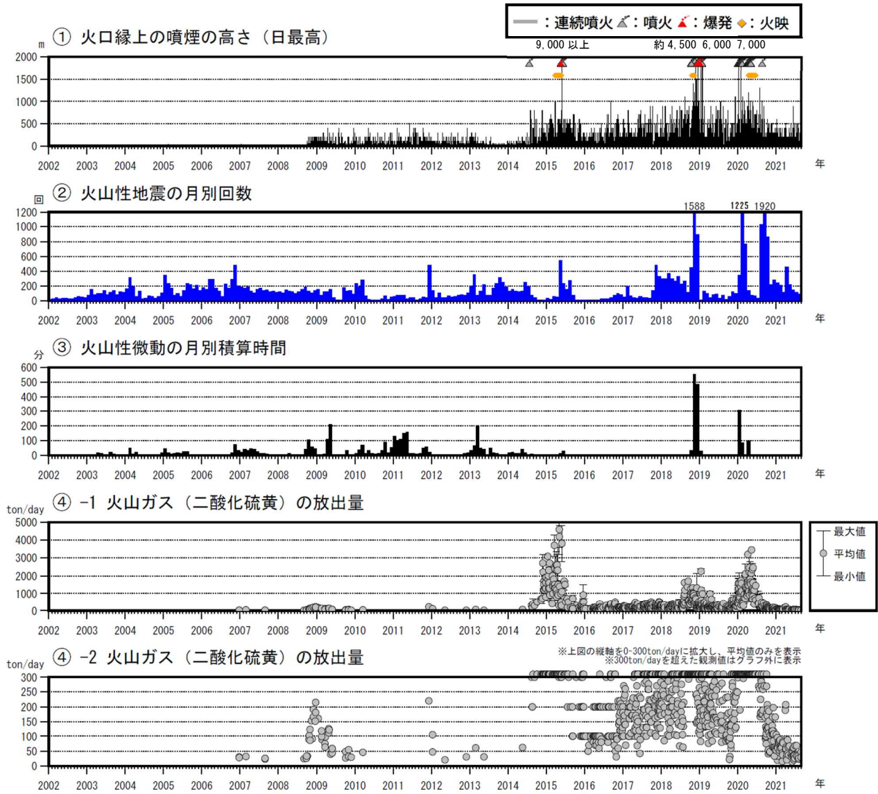
図5 口永良部島 火山活動経過図（2002年1月～2021年8月）
