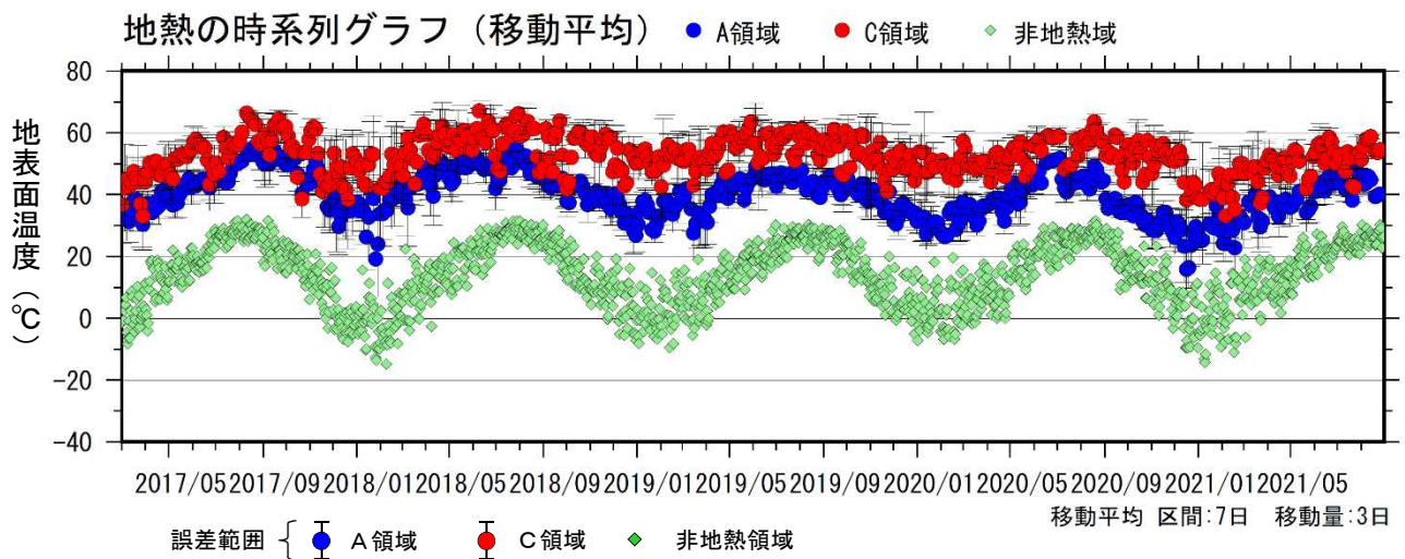
図 1-2 九重山 星生山北尾根の赤外熱映像装置による日別最高温度（2017年3月～2021年8月）
