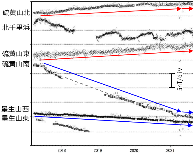
図 4-1 九重山 連続観測による全磁力の変化 (2017年3月～2021年8月)
