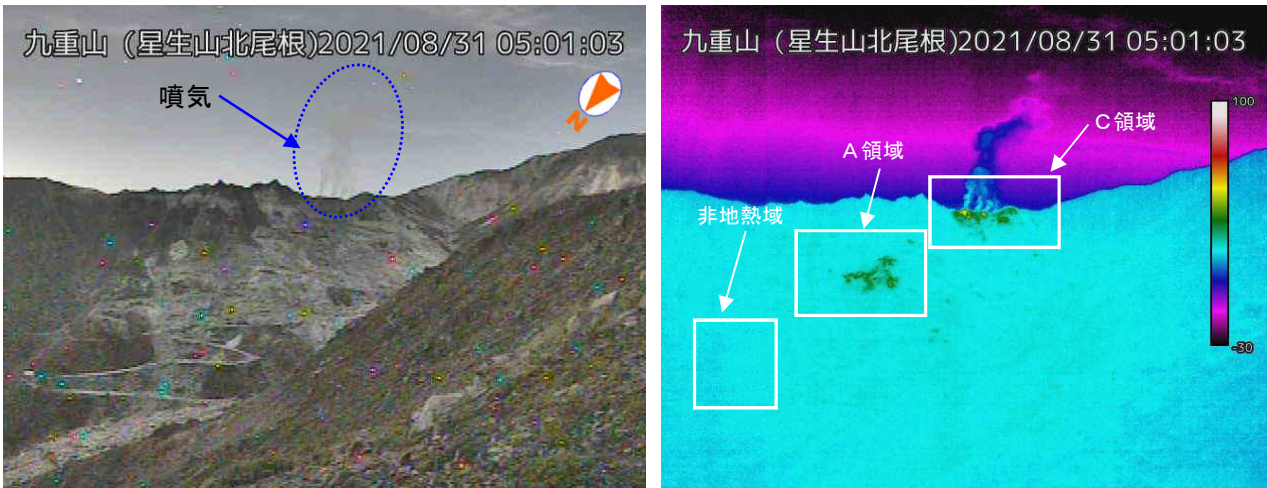
図 1-1 九重山 硫黄山の噴気及び地熱域の状況（8月31日 星生山北尾根監視カメラ）
