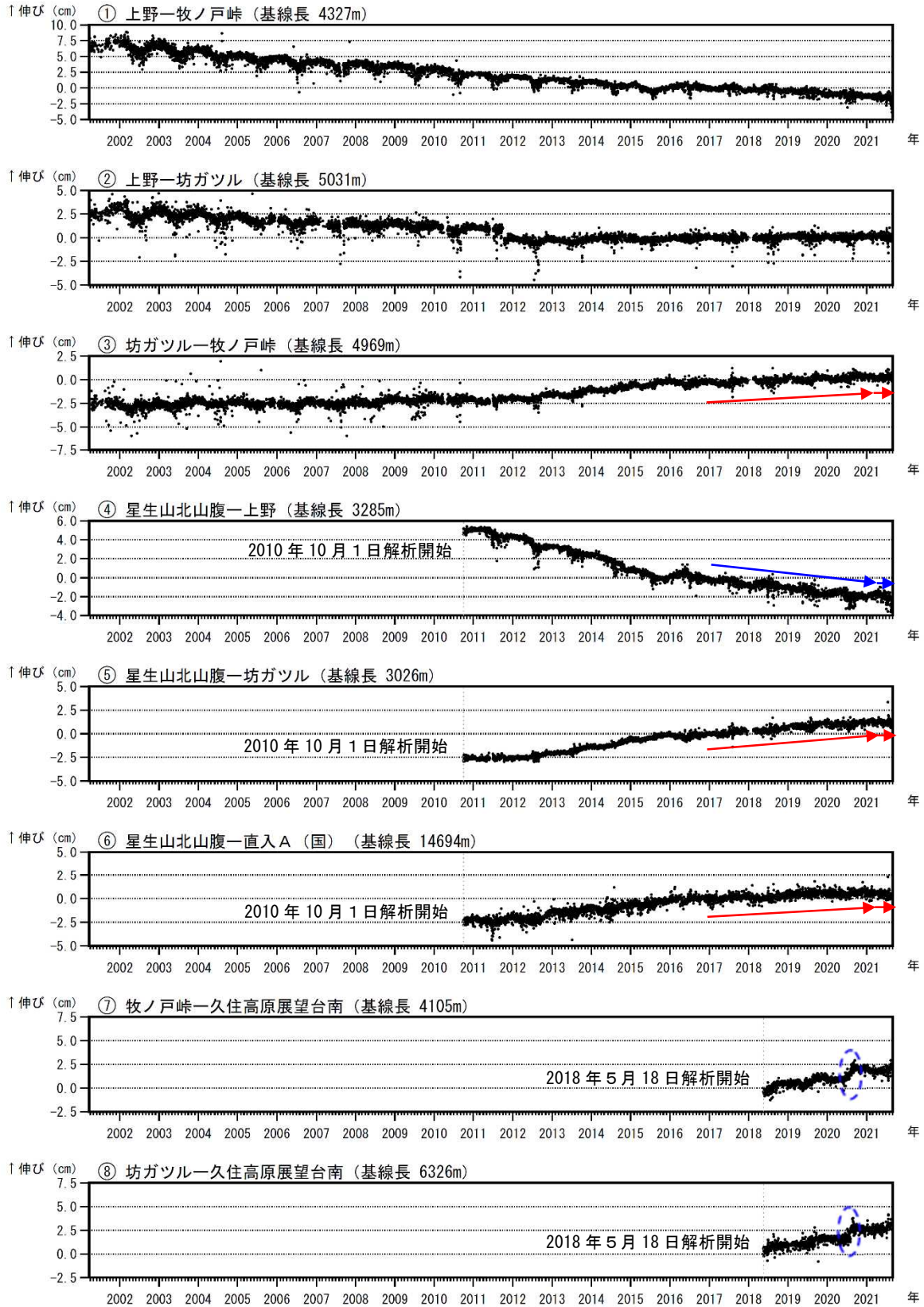
図5 九重山 GNSS連続観測による基線長変化（2001年4月～2021年8月）
