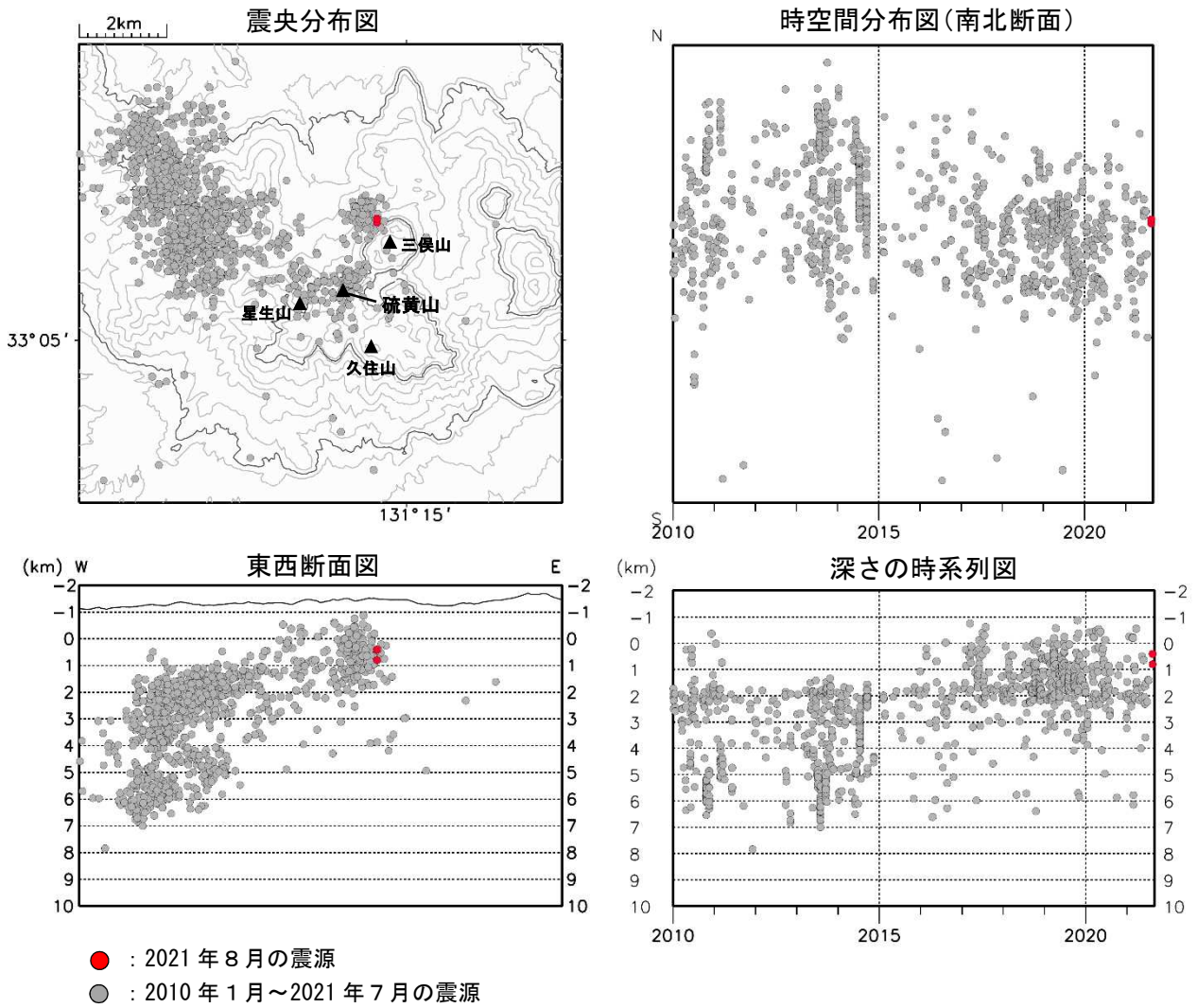
図3 九重山 震源分布図（2010年1月～2021年8月）
