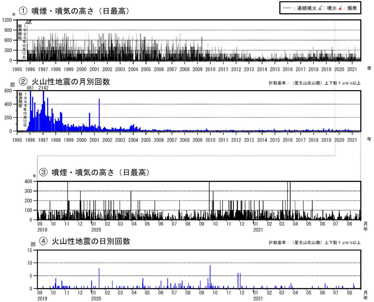
図2 九重山 火山活動経過図（1995年1月～2021年8月）
