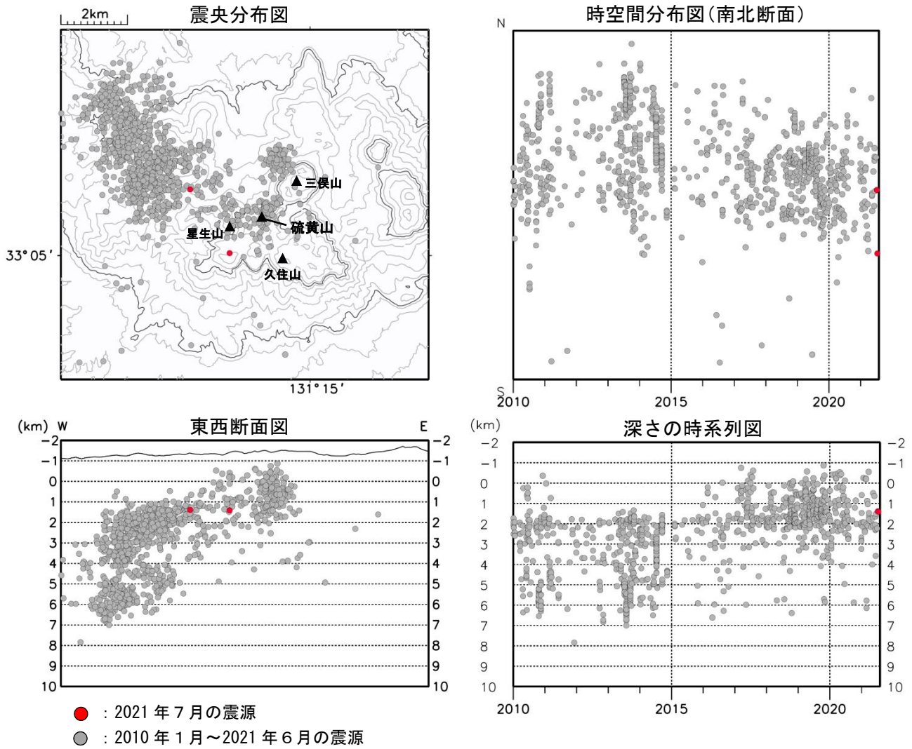
図3 九重山 震源分布図（2010年1月～2021年7月）
