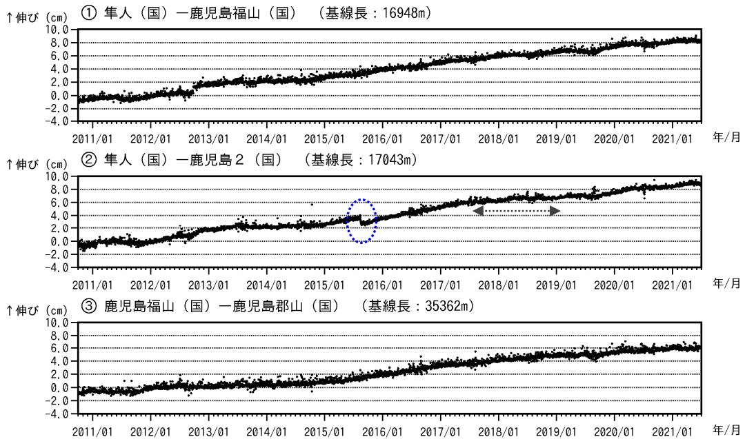
図7-1 桜島 GNSS 連続観測による基線長変化（2010年10月～2021年6月）
