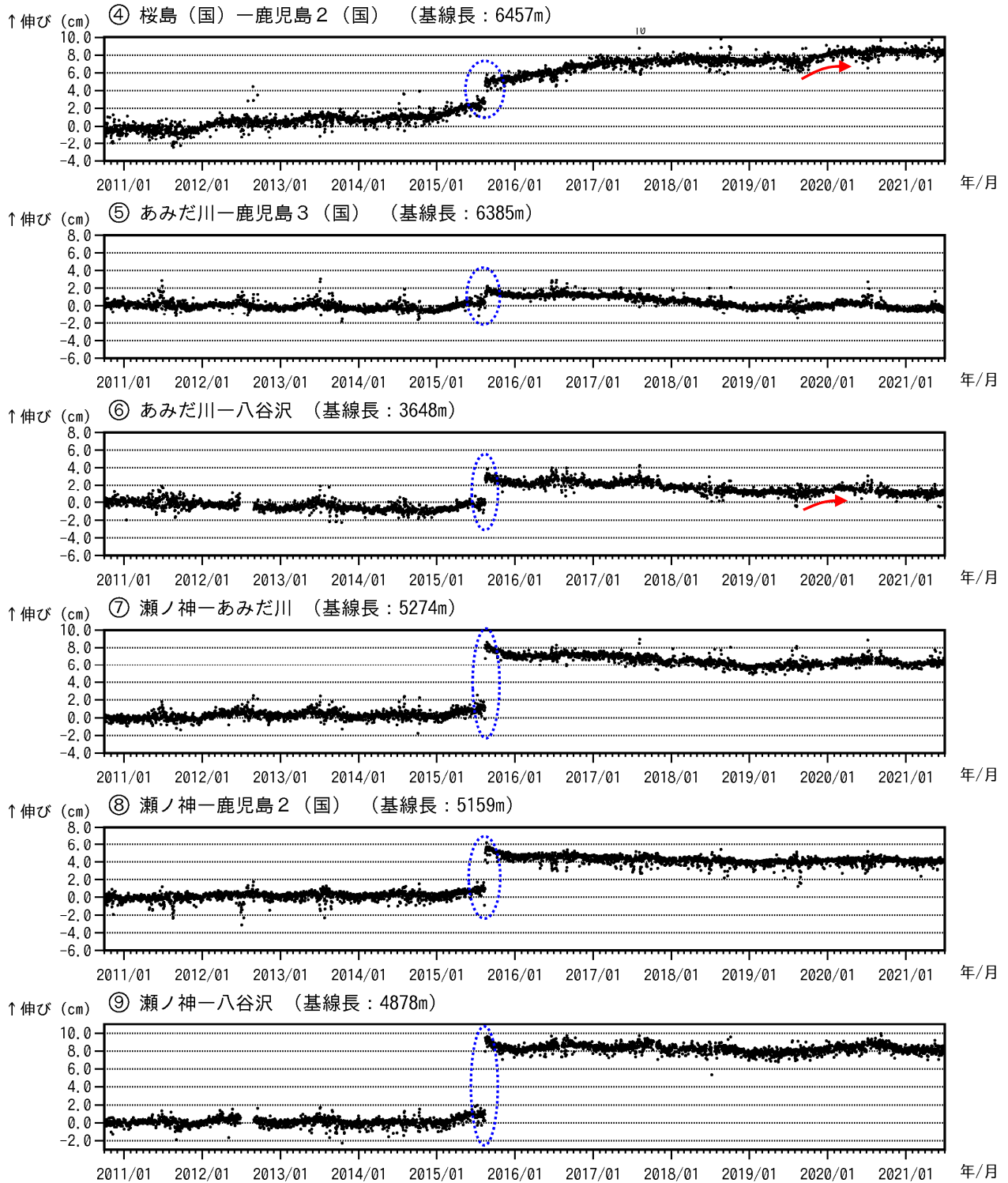
図7-2 桜島 GNSS 連続観測による基線長変化（2010年10月～2021年6月）
