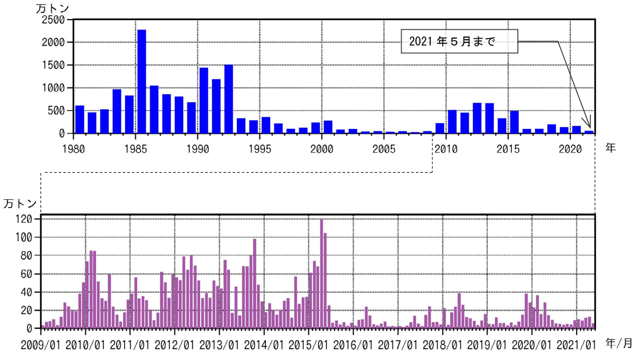
図4 桜島 鹿児島県が実施している降灰の観測データから推定した火山灰の総噴出量 （上段：1980年1月～2021年5月の年別値、下段：2009年1月～2021年5月の月別値）
