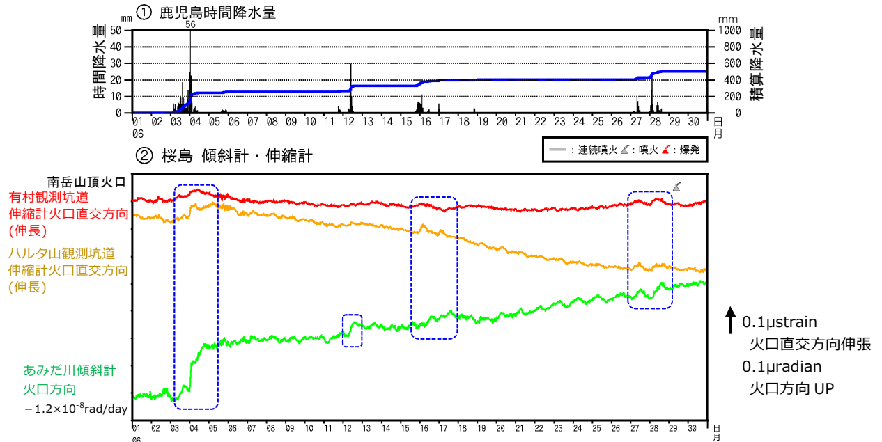
図6 桜島 傾斜計及び伸縮計による地殻変動の状況（2021年6月）
