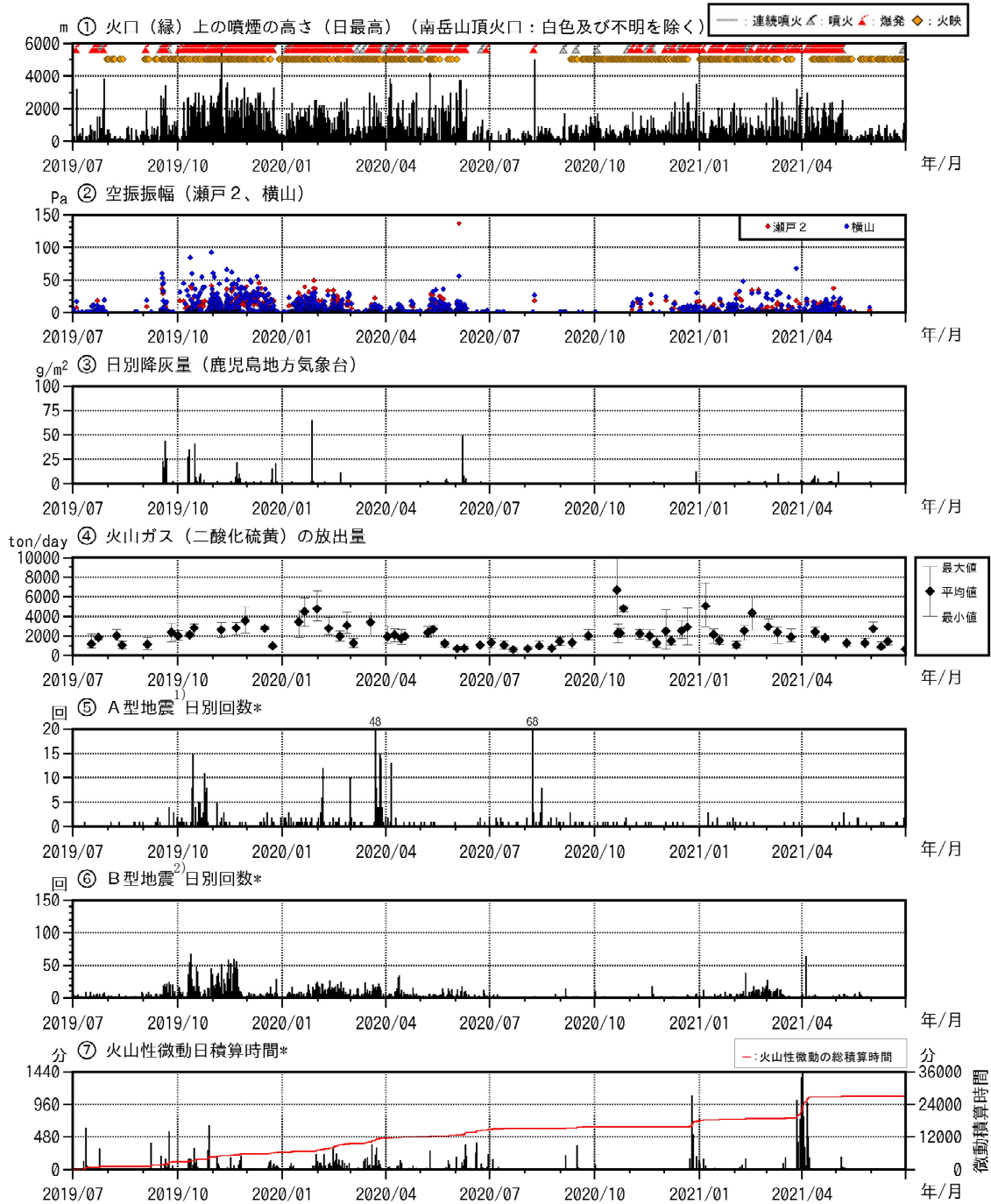
図5 桜島 最近2年間の活動経過図（2019年7月～2021年6月）
