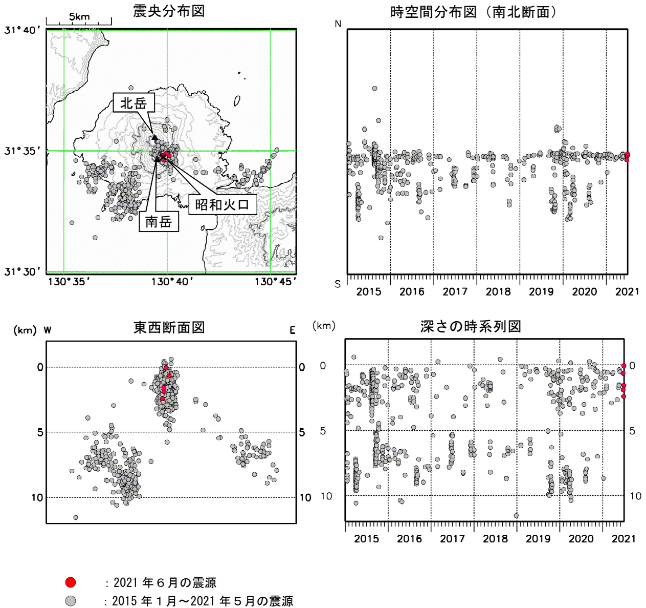
図2 桜島 震源分布図（2015年1月～2021年6月）
