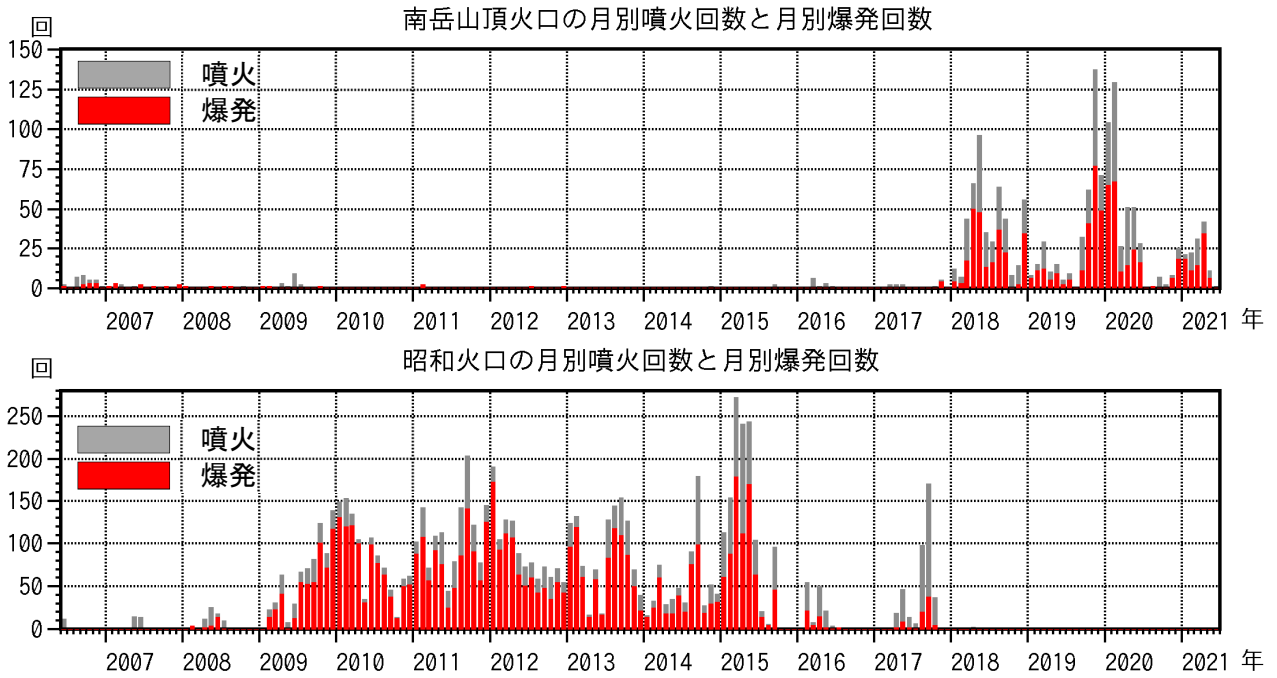
図3 桜島 南岳山頂火口（上図）と昭和火口（下図）の月別噴火回数と月別爆発回数 （2006年6月～2021年6月）
