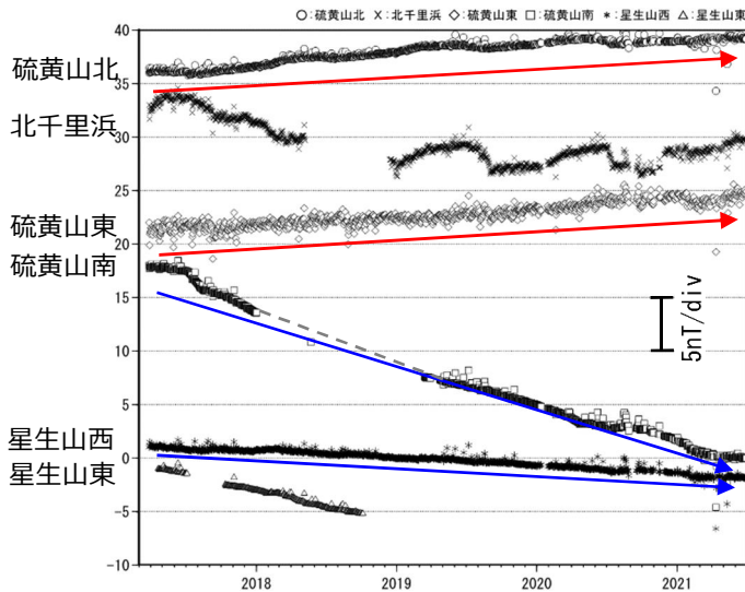
全磁力連続観測（2017年3月～2021年6月）
