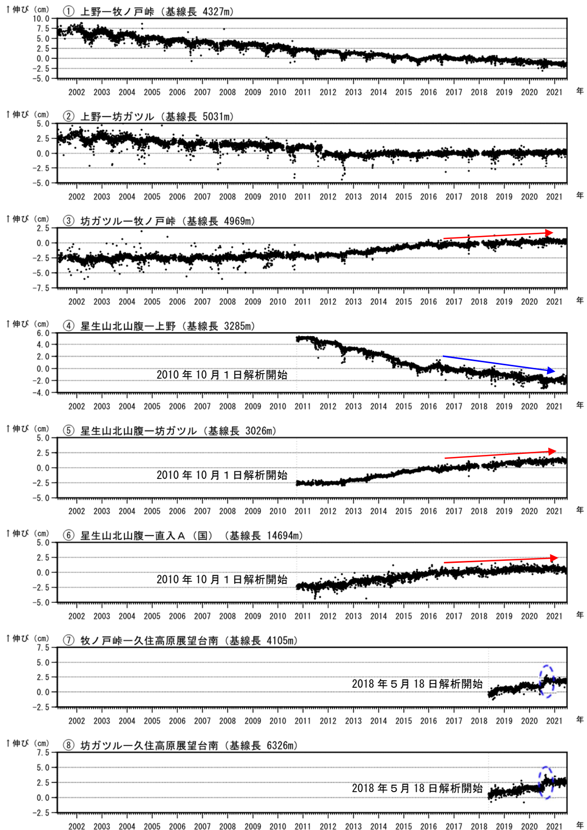
図5 九重山 GNSS連続観測による基線長変化（2001年4月～2021年6月）
