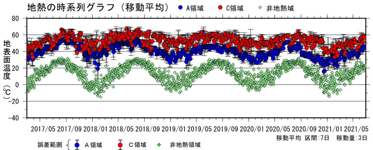
図 1-2 九重山 星生山北尾根の赤外熱映像装置による日別最高温度（2017年3月～2021年6月）
