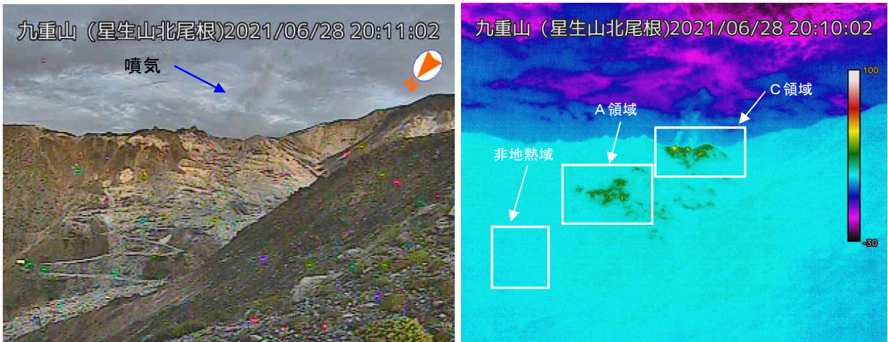
図 1-1 九重山 硫黄山の噴気および地熱域の状況（6月28日 星生山北尾根監視カメラ）
