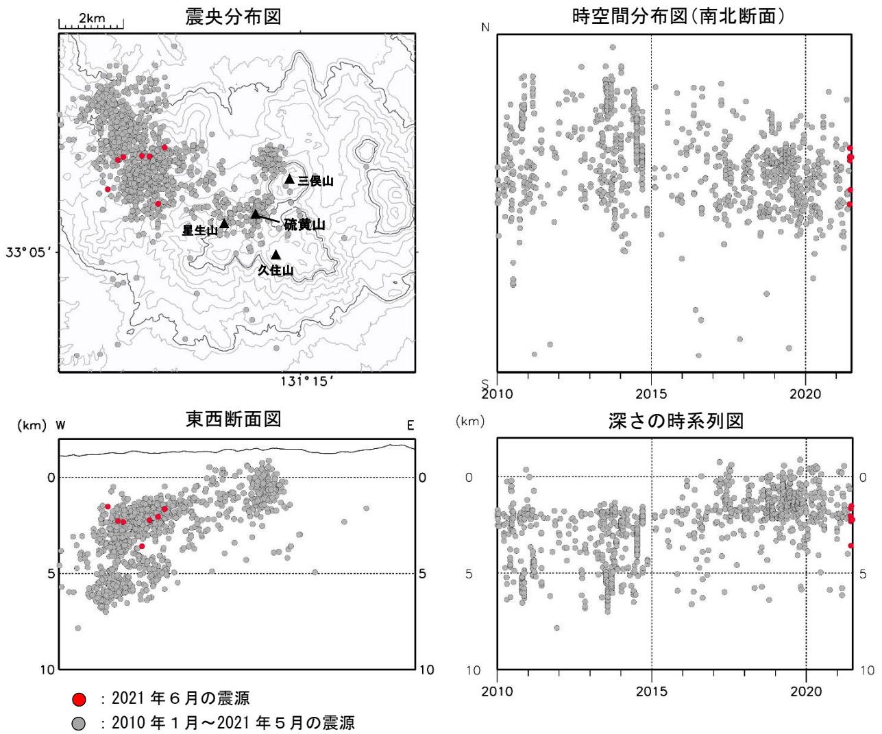
図3 九重山 震源分布図（2010 年 1 月～2021 年 6 月）
