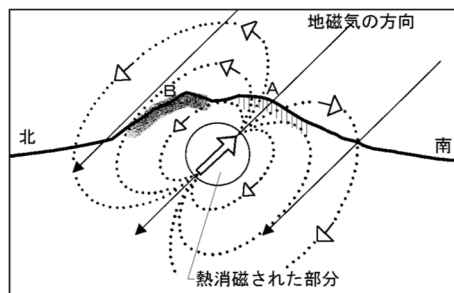
図 4-3 熱消磁に伴う全磁力変化のモデル
