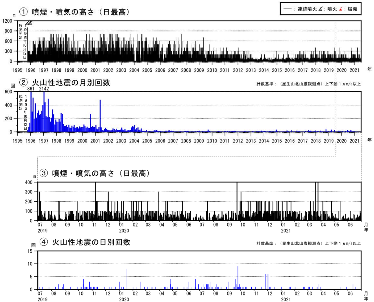
図2 九重山 火山活動経過図（1995年1月～2021年6月）
