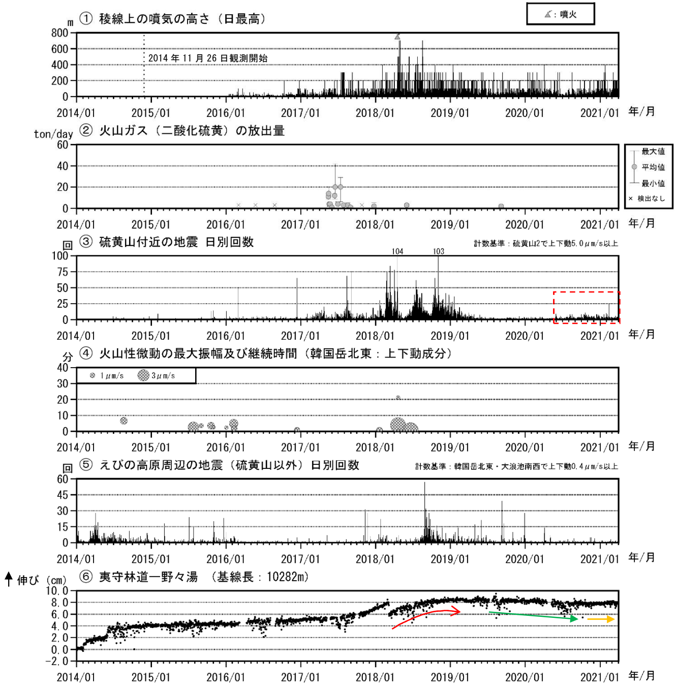
図7 霧島山（えびの高原（硫黄山）周辺） 火山活動経過図（2014年1月～2021年3月）
