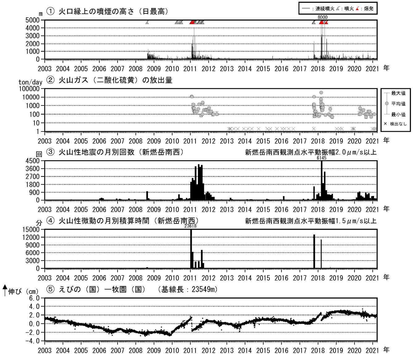
図4 霧島山（新燃岳） 火山活動経過図（2003年1月～2021年3月）
