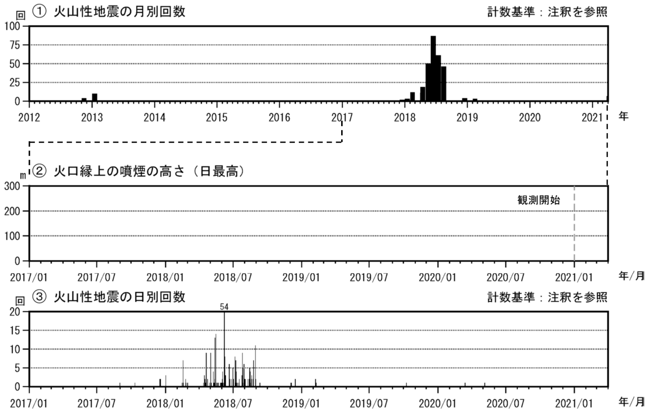
図4 霧島山（大幡池） 火山活動経過図（2012年1月～2021年3月）
