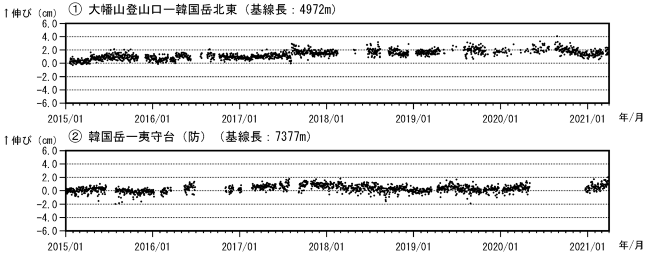
図6 霧島山（大幡池） GNSS 連続観測による基線長変化（2015年1月～2021年3月）
