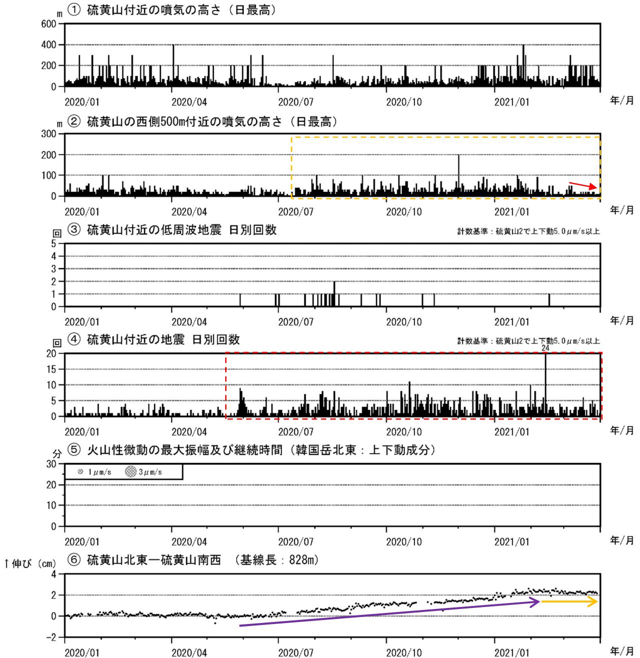
図6 霧島山（えびの高原（硫黄山）周辺） 火山活動経過図（2020年1月～2021年3月）
