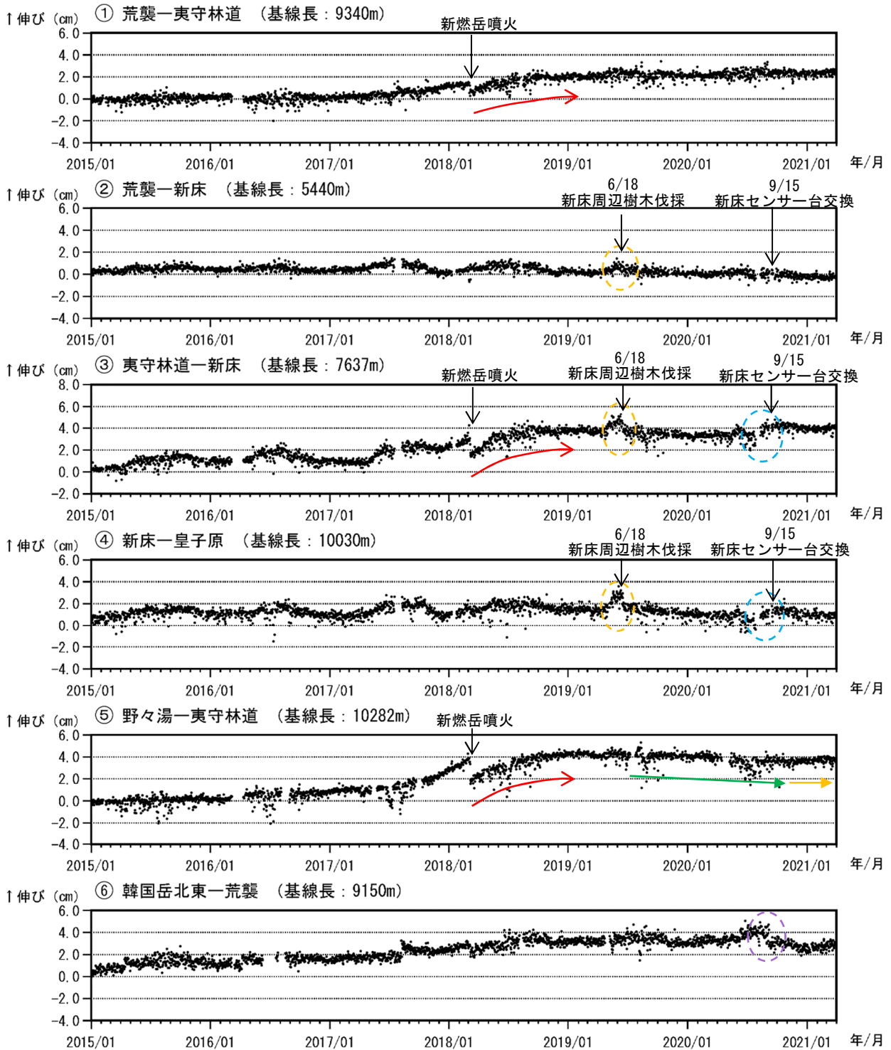
図 8-1 霧島山（新燃岳）GNSS 連続観測による基線長変化（2015 年 1 月～2021 年 3 月）
