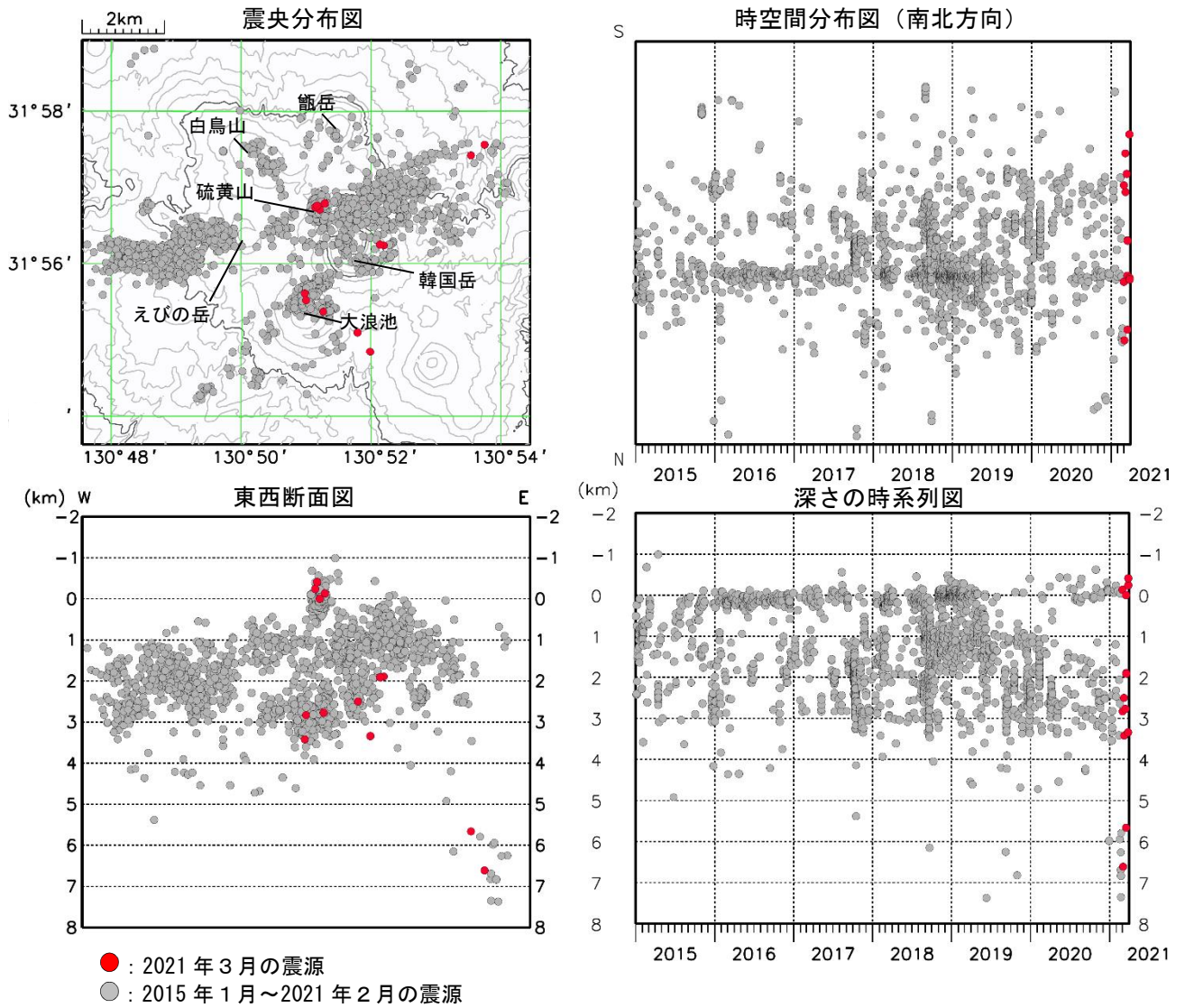
図5 霧島山（えびの高原（硫黄山）周辺） 震源分布図（2015年1月～2021年3月）
