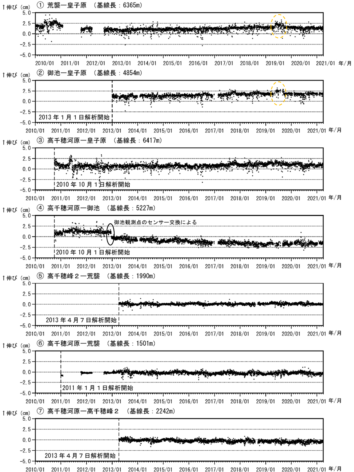
図4 霧島山（御鉢） GNSS 連続観測による基線長変化（2010年1月～2021年3月）
