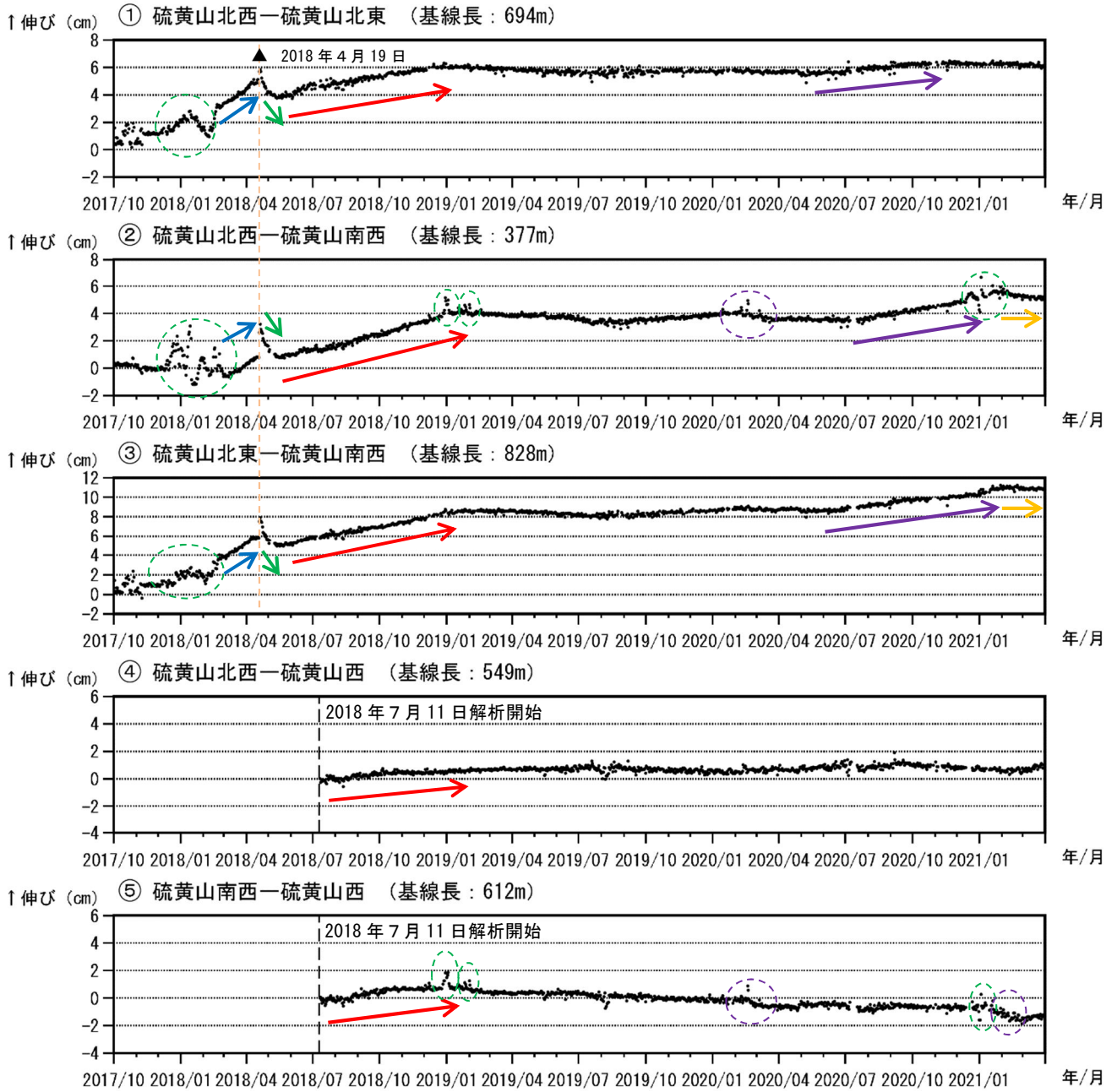
図8 霧島山（えびの高原（硫黄山）周辺） GNSS 連続観測による基線長変化 (2017年10月～2021年3月)
