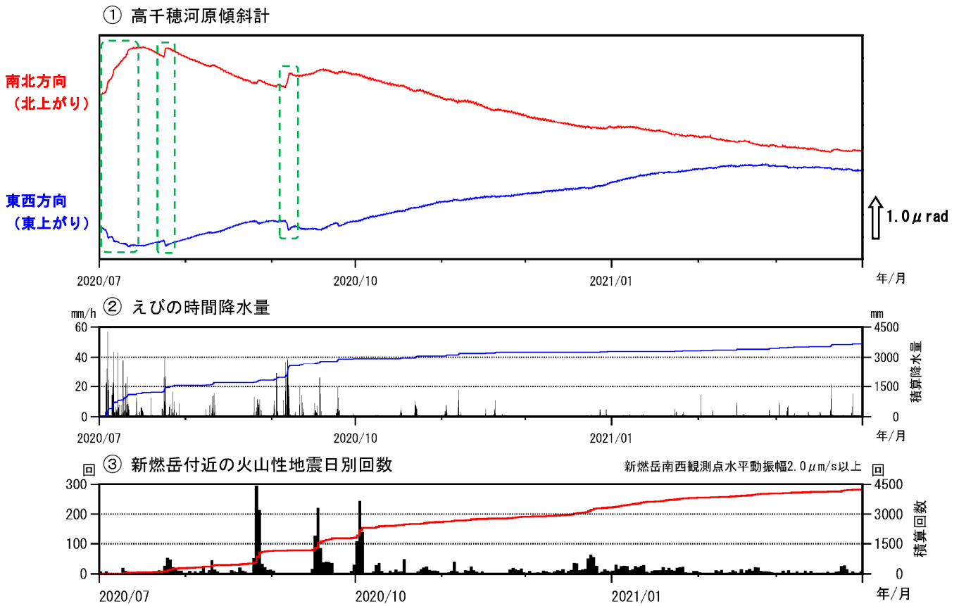
図6 霧島山（新燃岳） 高千穂河原観測点の傾斜変動の状況（2020年7月～2021年3月）
