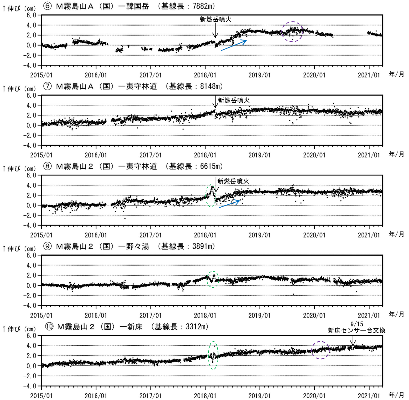
図 9-2 霧島山（えびの高原（硫黄山）周辺） GNSS 連続観測による基線長変化 (2015年1月～2021年3月)
