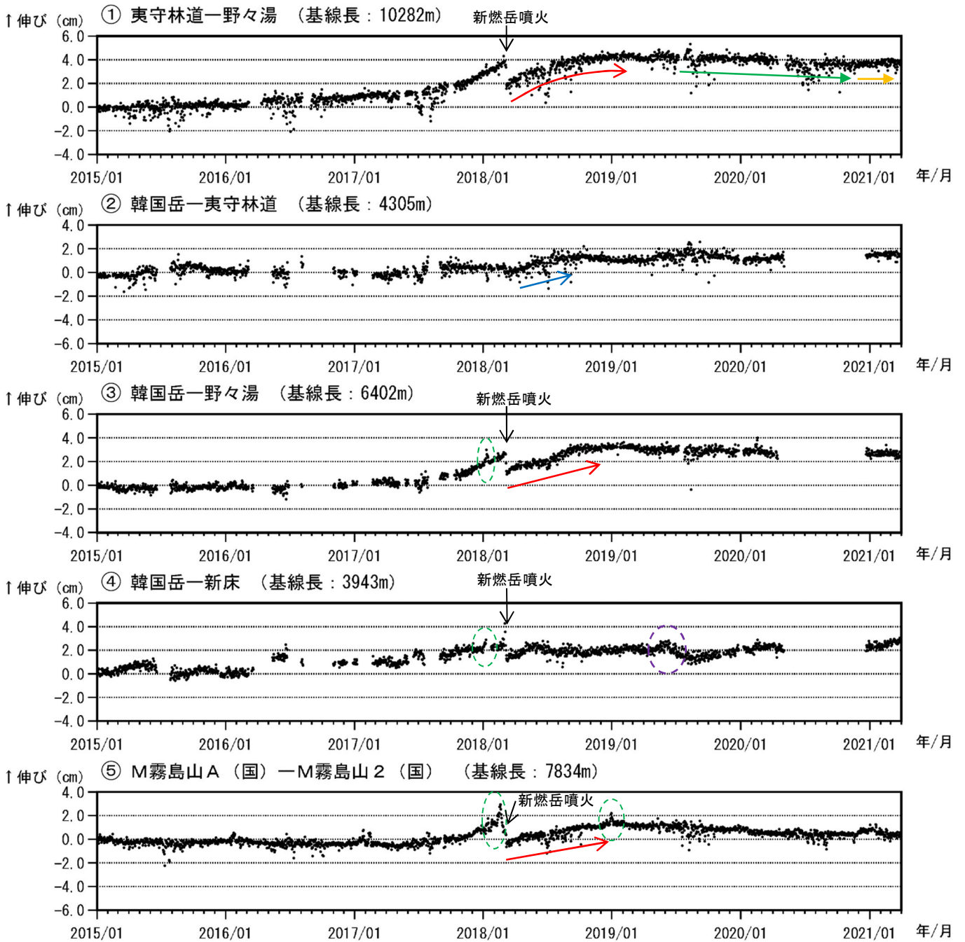
図 9-1 霧島山（えびの高原（硫黄山）周辺） GNSS 連続観測による基線長変化 (2015年1月～2021年3月)
