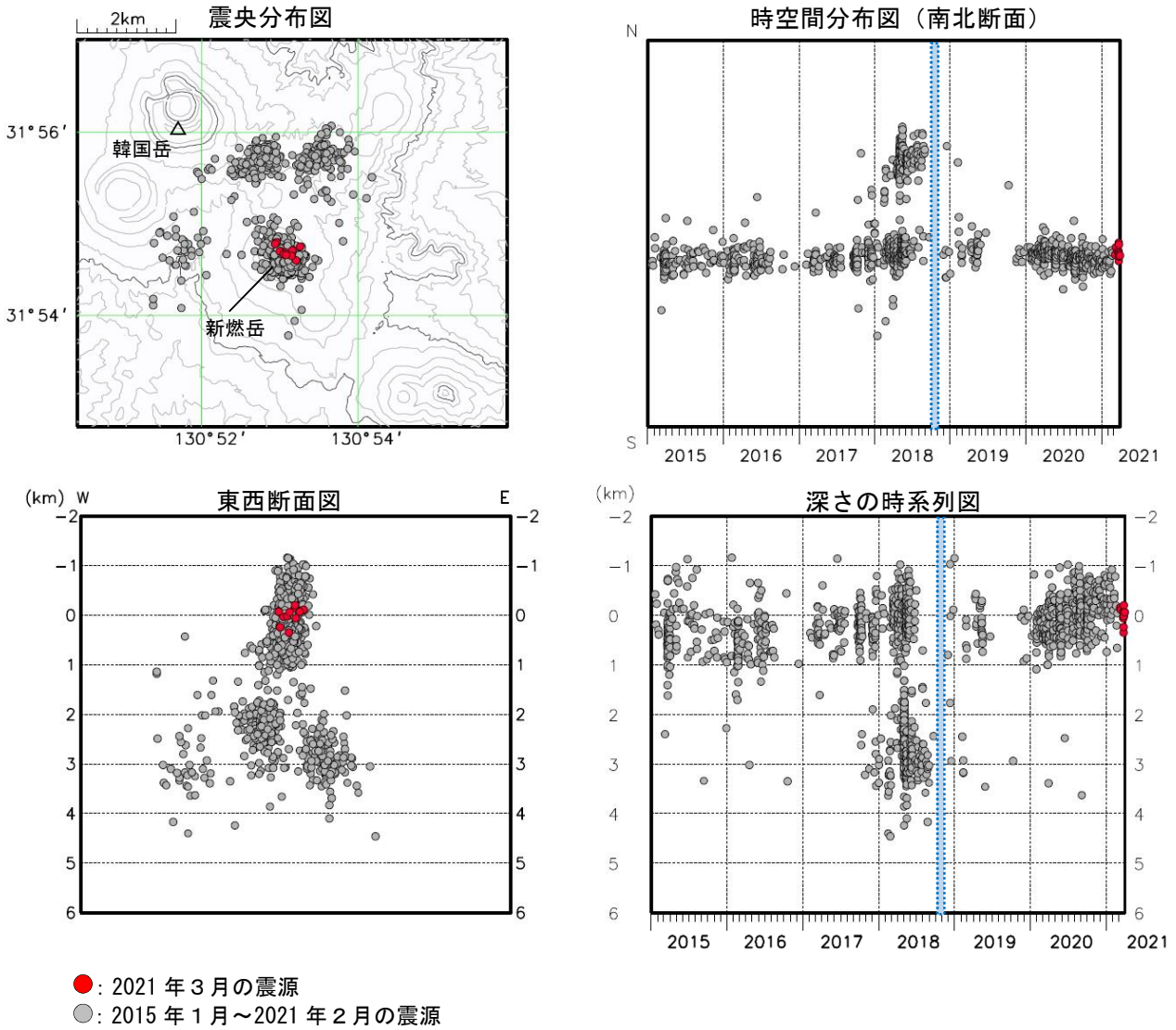
図7 霧島山（新燃岳） 震源分布図（2015年1月～2021年3月）
