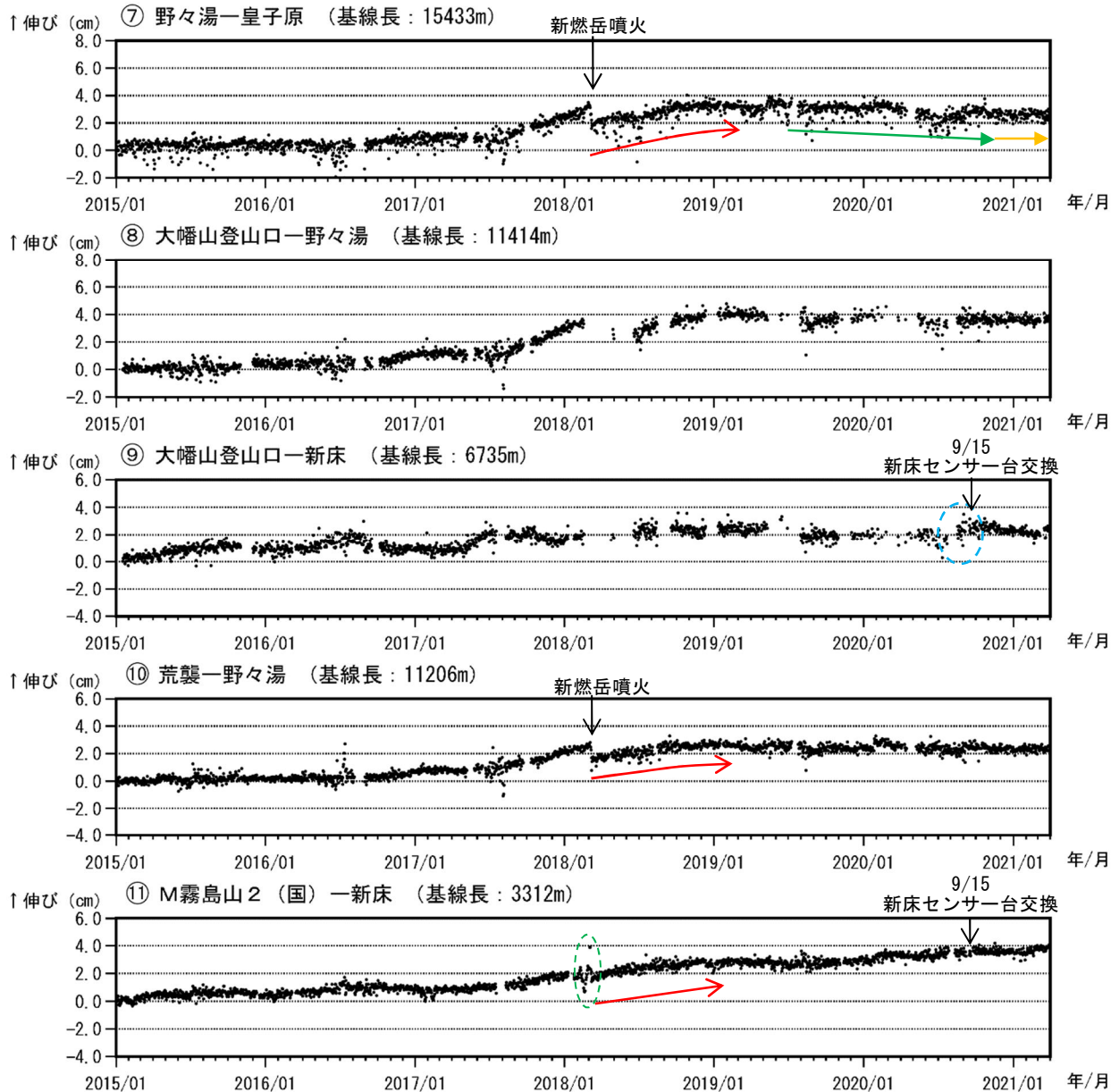
図 8-2 霧島山（新燃岳） GNSS 連続観測による基線長変化（2015 年 1 月～2021 年 3 月）
