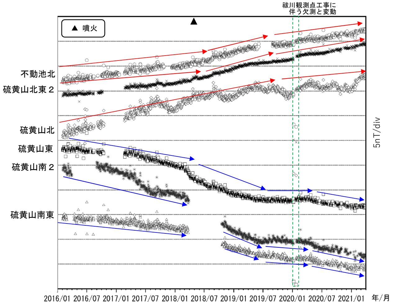
図13 霧島山（えびの高原（硫黄山）周辺） 全磁力観測点で観測された全磁力変動（2016年1月～2021年3月）
