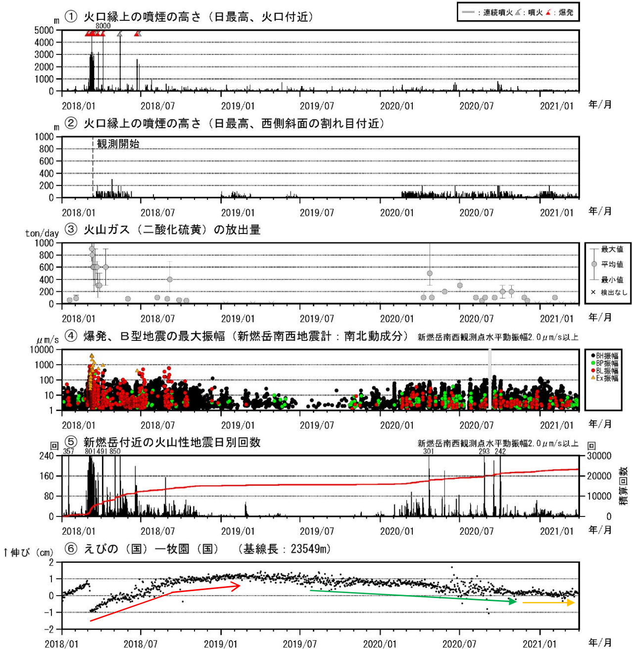
図5 霧島山（新燃岳） 火山活動経過図（2018年1月～2021年3月）
