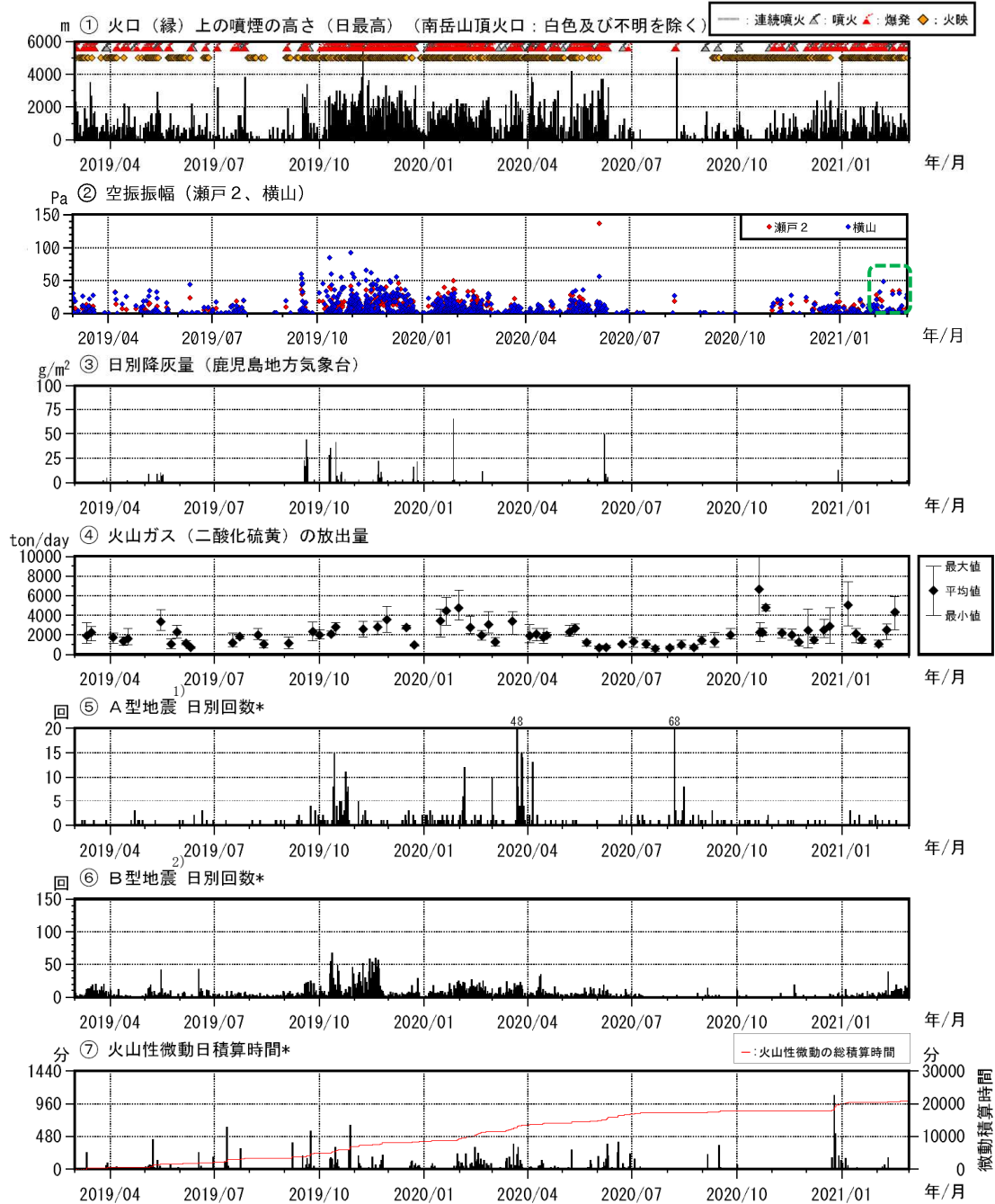
図4 桜島 最近2年間の活動経過図（2019年3月～2021年2月）
