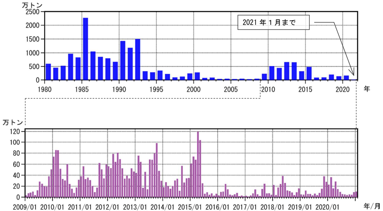
図8 桜島 鹿児島県が実施している降灰の観測データから推定した火山灰の総噴出量 (上段：1980年1月～2021年1月の年別値、下段：2009年1月～2021年1月の月別値)
