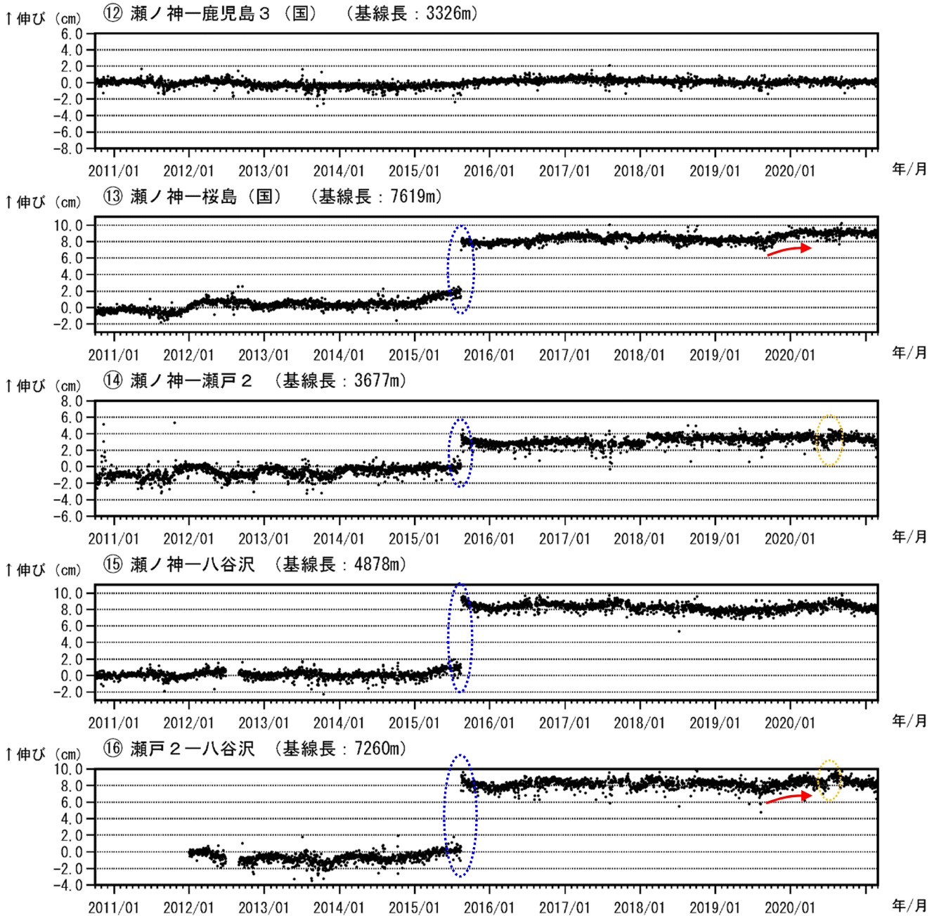
図 6-3 桜島 GNSS 連続観測による基線長変化（2010 年 10 月～2021 年 2 月）
