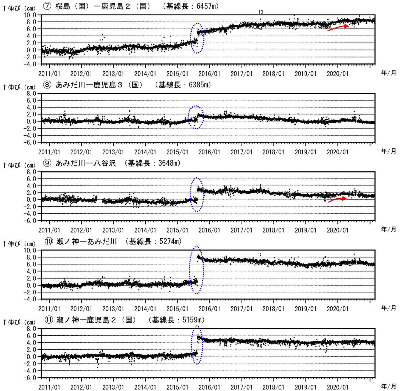
図 6-2 桜島 GNSS 連続観測による基線長変化 (2010 年 10 月～2021 年 2 月)
