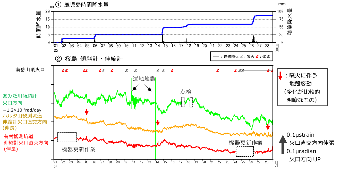
図5 桜島 傾斜計及び伸縮計による地殻変動の状況（2021年2月）
