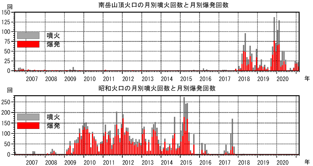
図 3-2 桜島 南岳山頂火口（上図）と昭和火口（下図）の月別噴火回数と月別爆発回数 （2006年6月～2021年2月）
