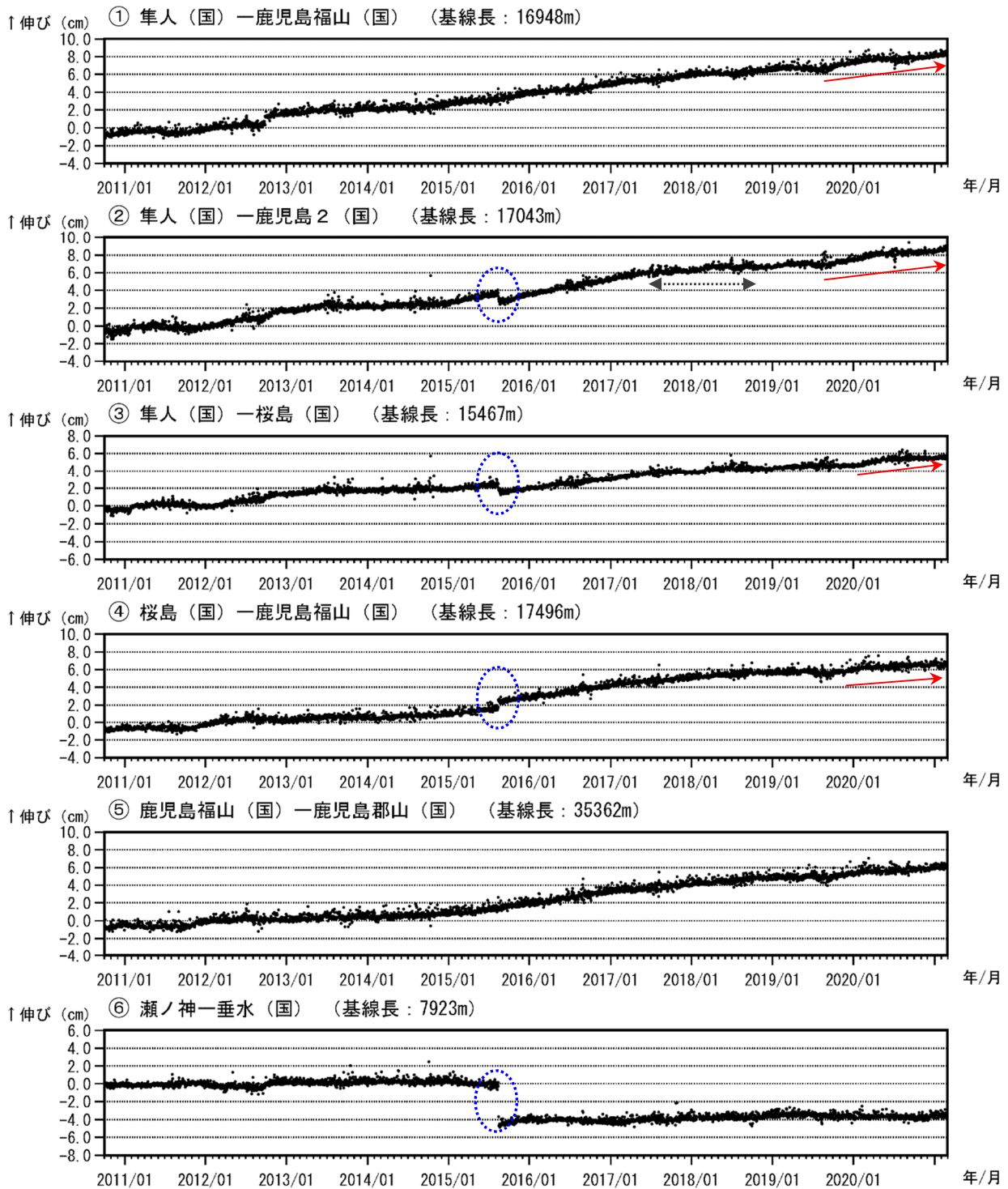
図 6-1 桜島 GNSS 連続観測による基線長変化（2010年10月～2021年2月）
