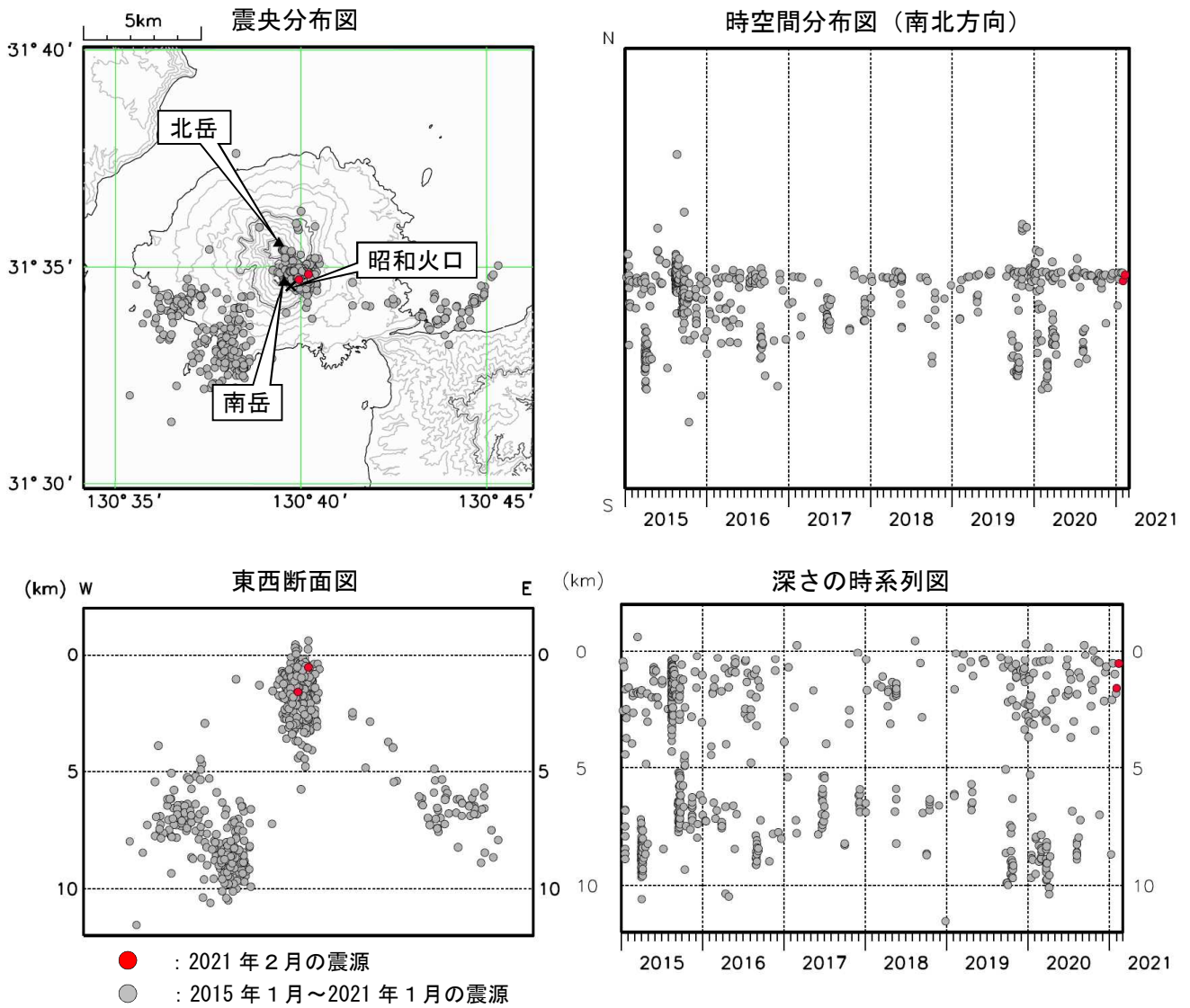
図2 桜島 震源分布図（2015年1月～2021年2月）
