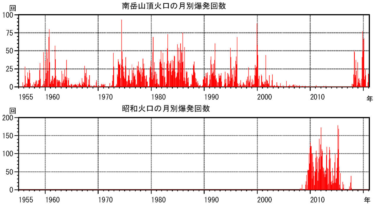
図 3-1 桜島 南岳山頂火口（上図）と昭和火口（下図）の月別爆発回数 （1955年1月～2021年2月）
