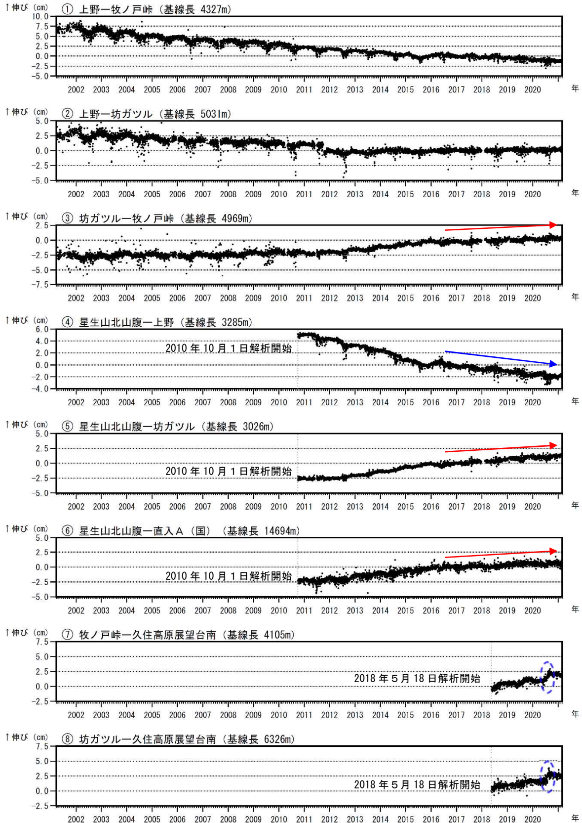
図8 九重山 GNSS連続観測による基線長変化（2001年4月～2021年2月）
