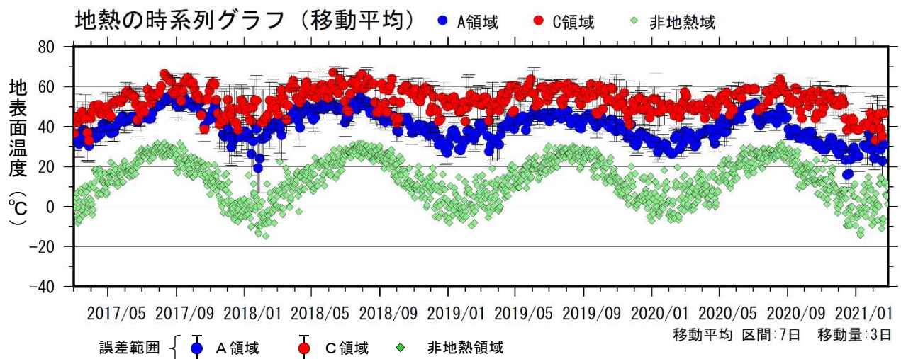
図2-2 九重山 星生山北尾根の赤外熱映像装置による日別最高温度（2017年3月～2021年2月）
