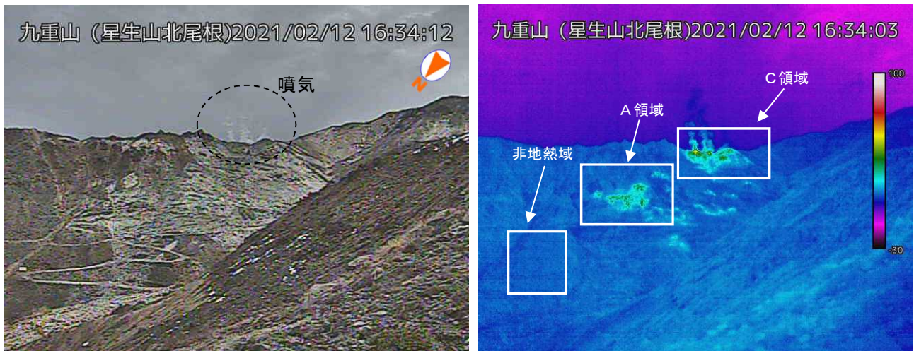
図2-1 九重山 噴気および地熱域の状況（2月12日 星生山北尾根監視カメラによる）
