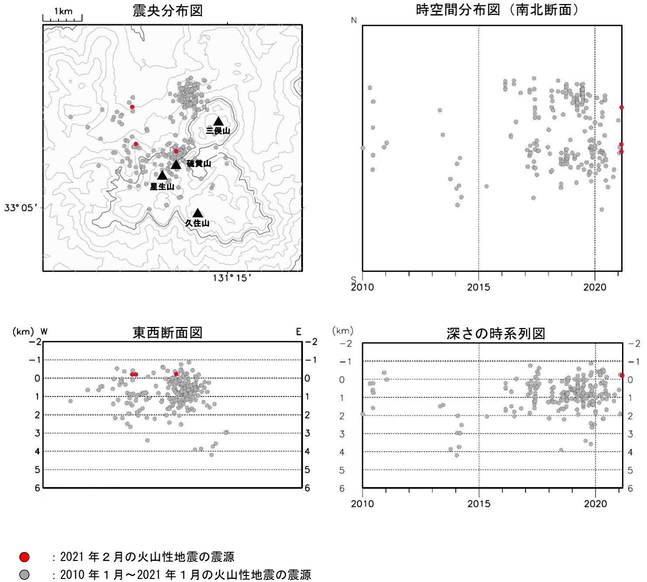
図 4-2 九重山 震源分布図（硫黄山付近の火山性地震）（2010年1月～2021年2月）
