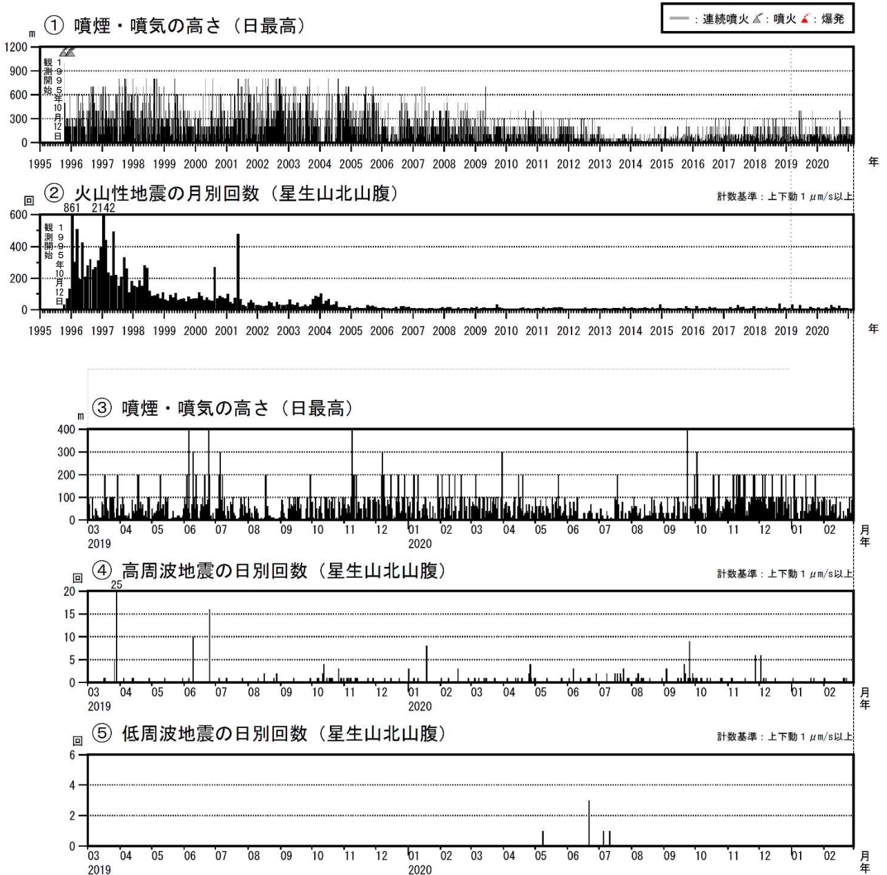
図3 九重山 火山活動経過図（1995年1月～2021年2月）
