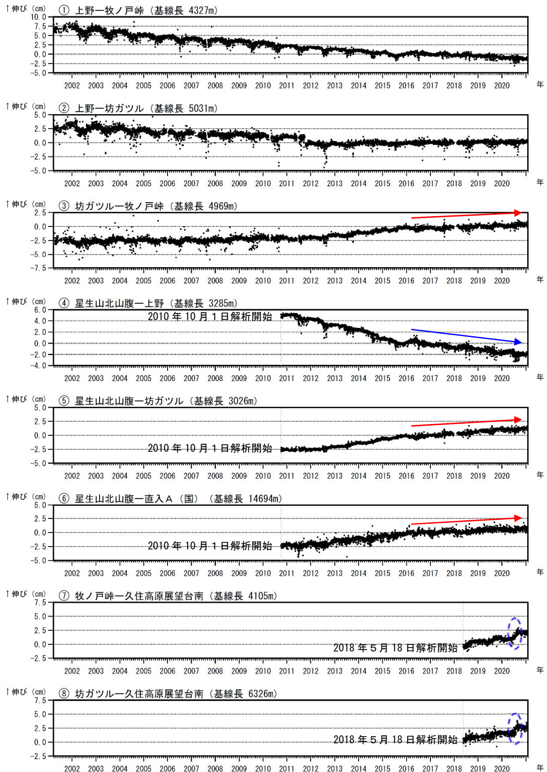
図8 九重山 GNSS連続観測による基線長変化（2001年4月～2021年1月）
