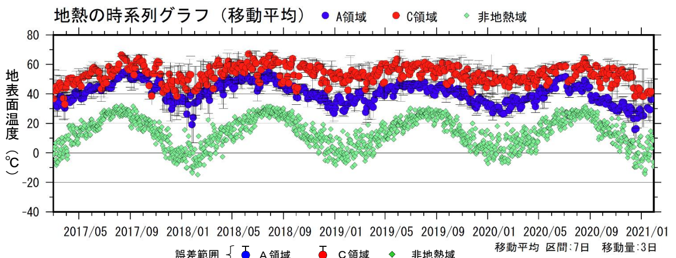
図2-2 九重山 星生山北尾根の赤外熱映像装置による日別最高温度（2017年3月～2021年1月）
