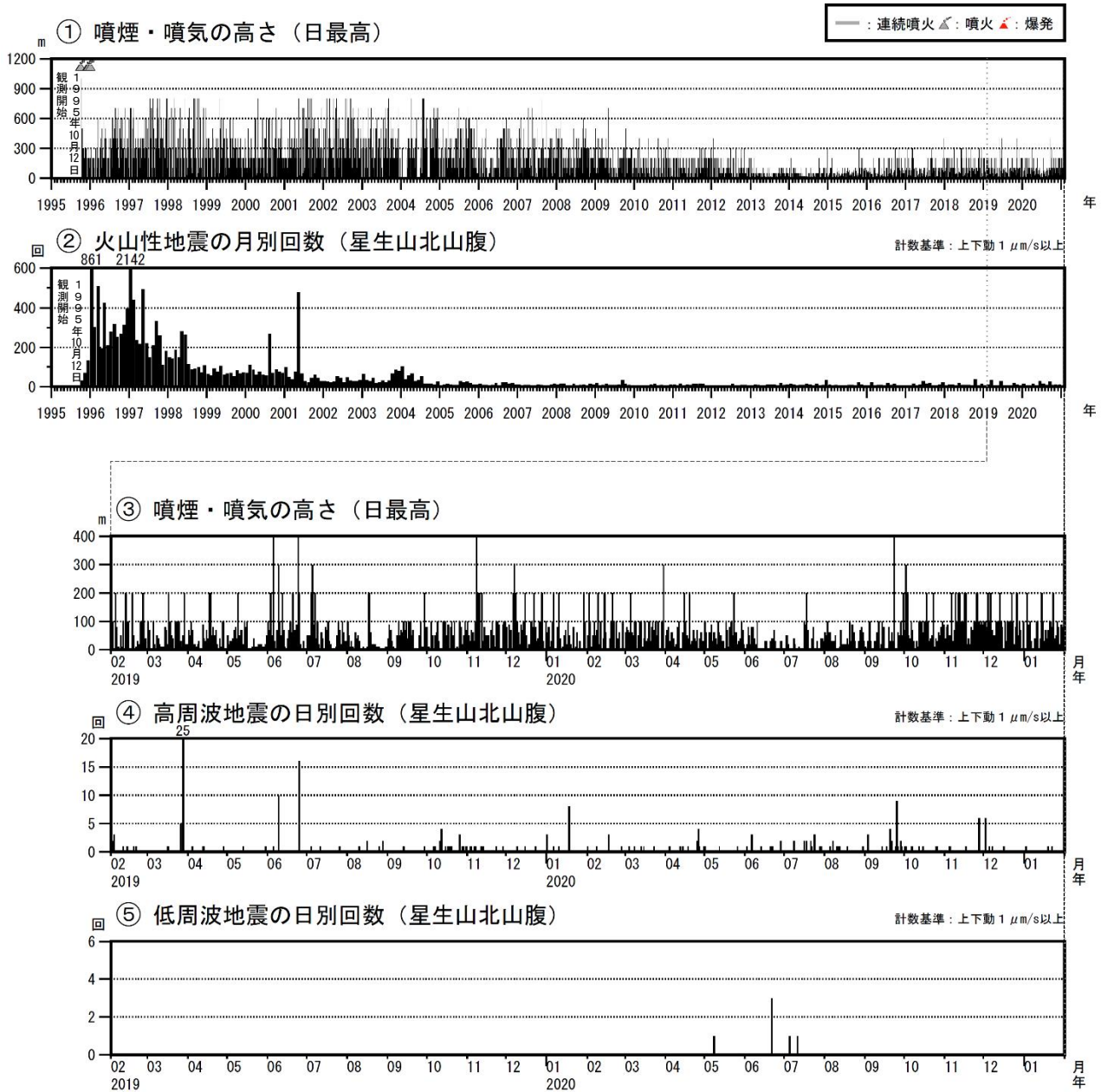
図3 九重山 火山活動経過図（1995年1月～2021年1月）
