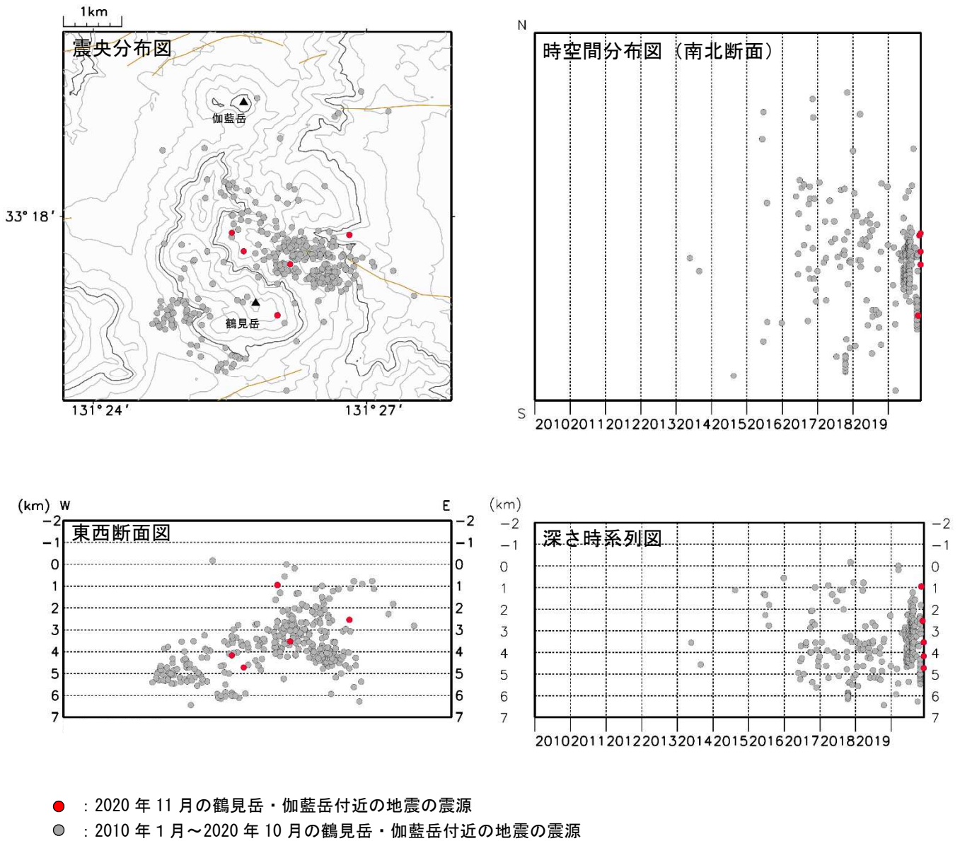
図 3-2 鶴見岳・伽藍岳 震源分布図（鶴見岳・伽藍岳付近の地震）（2010年1月～2020年11月）
