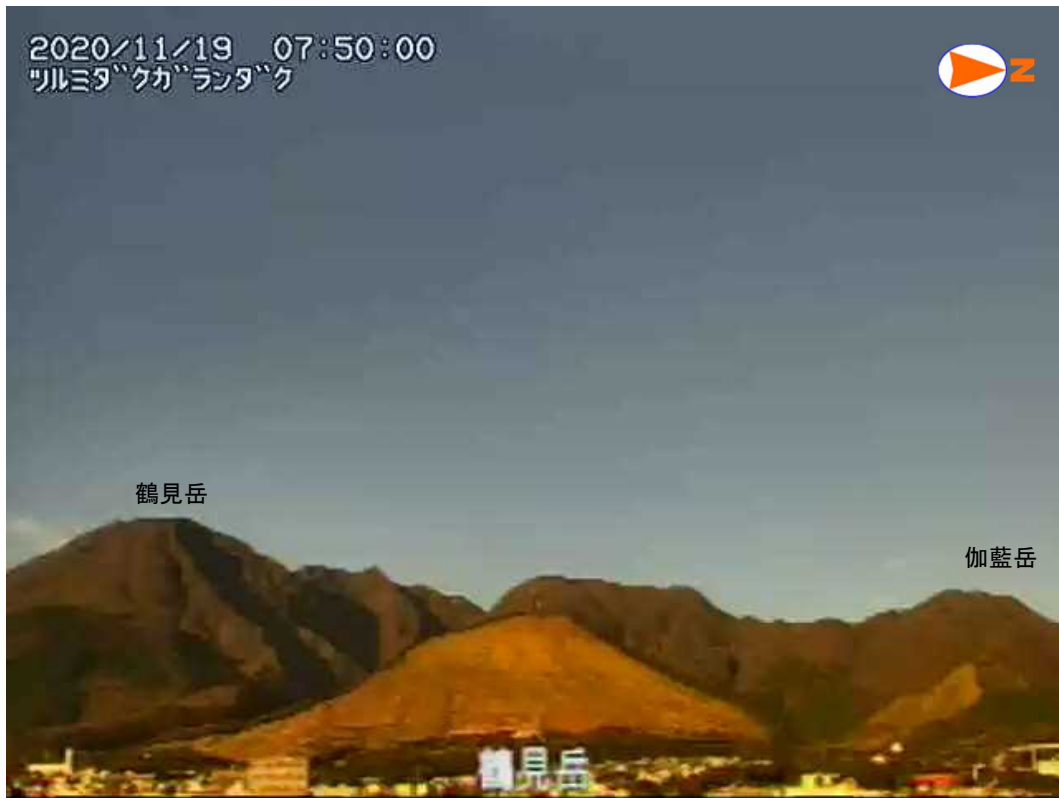
図 1-1 鶴見岳・伽藍岳 噴気の状態（11月19日、大分県監視カメラによる）
