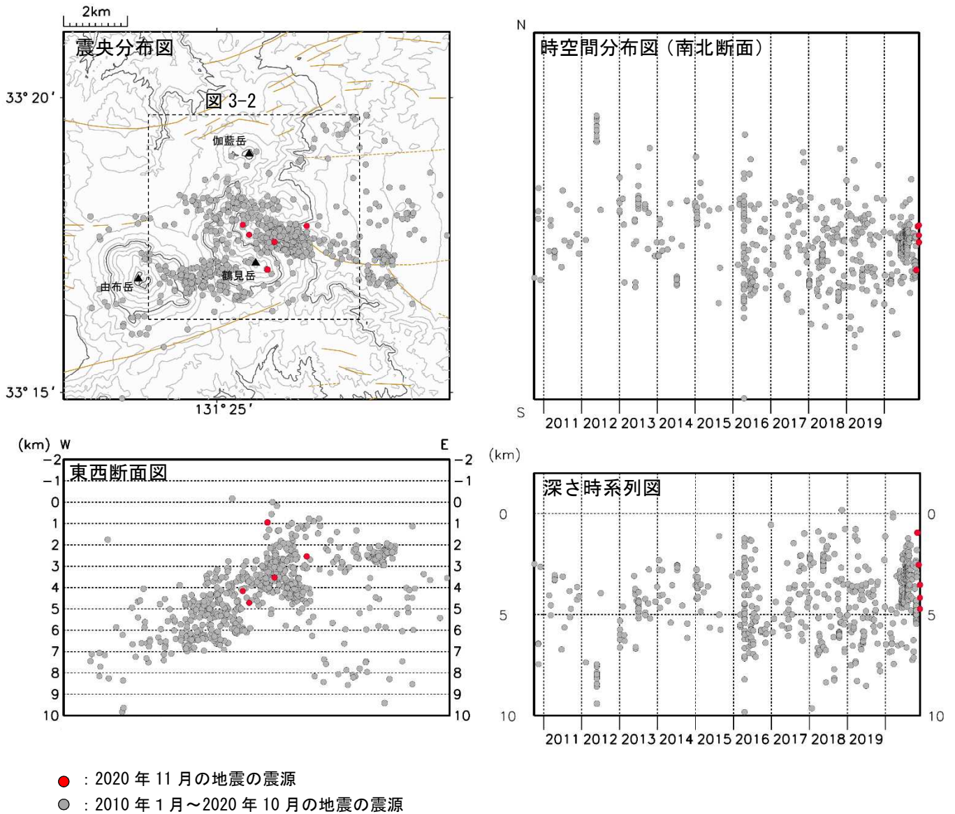
図 3-1 鶴見岳・加藍岳 震源分布図（広域）（2010年1月～2020年11月）
