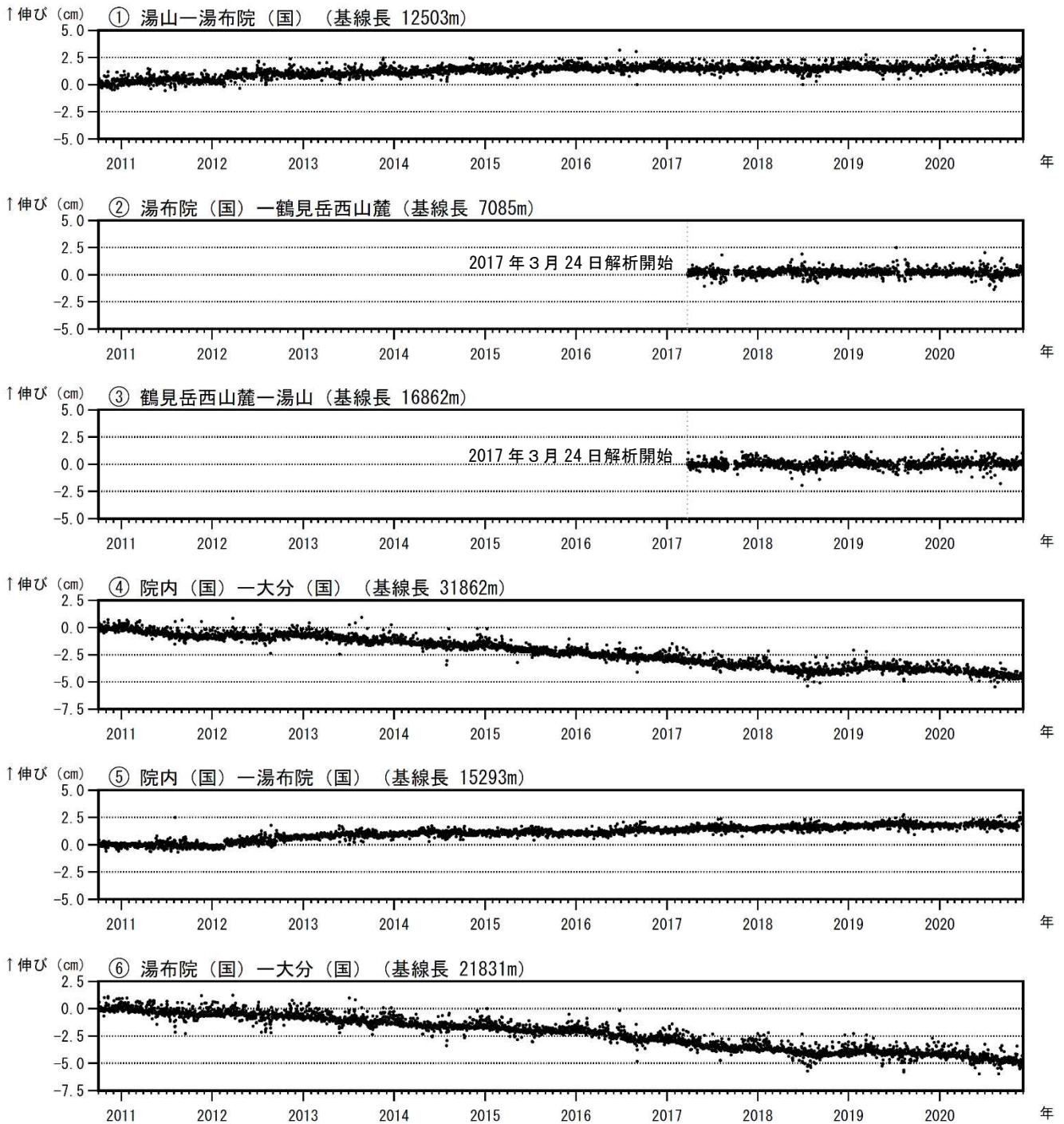
図4 鶴見岳・伽藍岳 GNSS連続観測による基線長変化（2010年10月～2020年11月）
