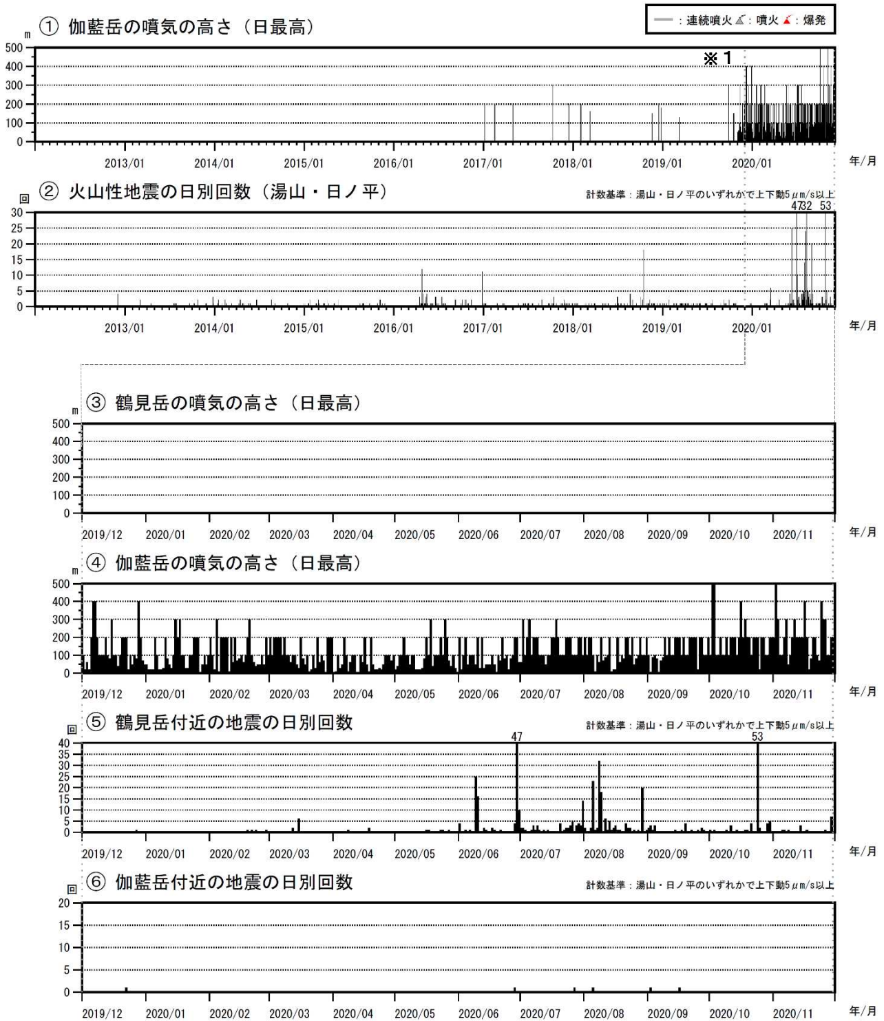
図2 鶴見岳・伽藍岳 火山活動経過図（2012年1月～2020年11月）
