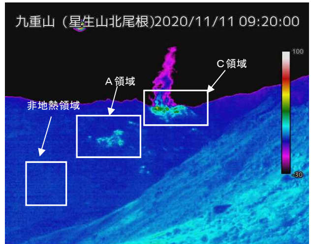
図2-1 九重山 噴気および地熱域の状況 (11月11日 星生山北尾根監視カメラ (左) 及び赤外熱映像装置による (右))
