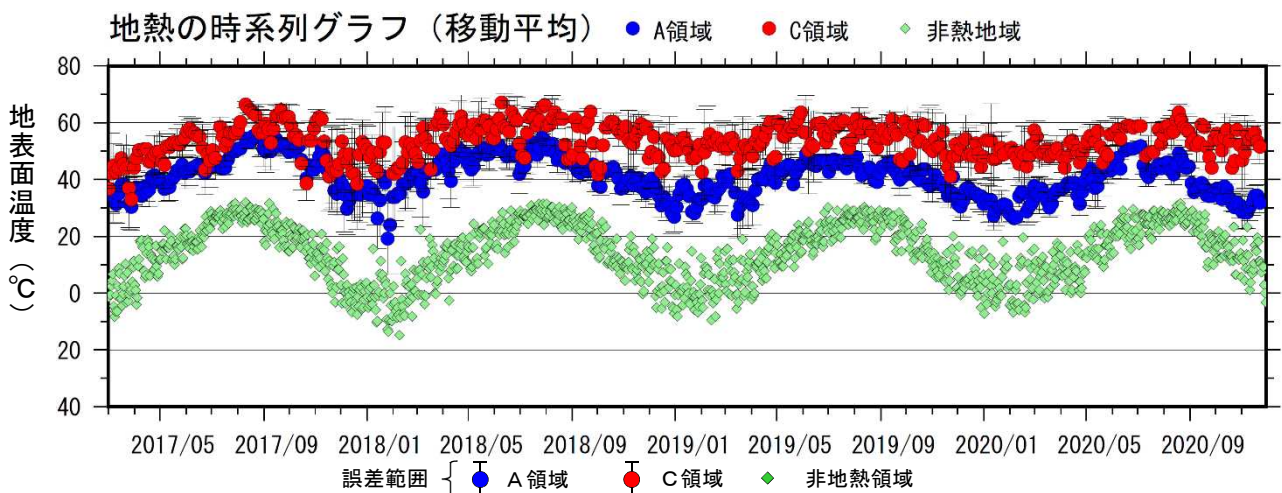
図2-2 九重山 星生山北尾根の赤外熱映像装置による日別最高温度(2017年3月~2020年11月) A領域、C領域ともに非地熱領域と比べて地表面温度が高い状態が続いています。
