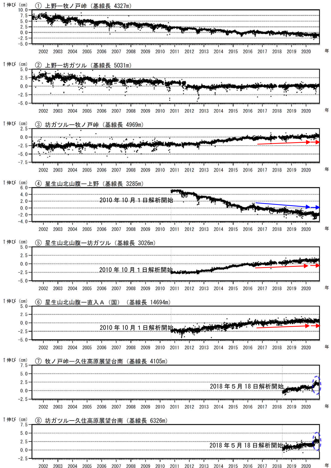
図8 九重山 GNSS連続観測による基線長変化（2001年4月～2020年11月）
