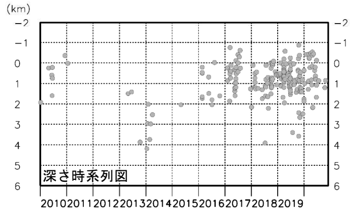
図4-2 九重山 震源分布図（硫黄山付近の火山性地震）（2010年1月～2020年11月）
