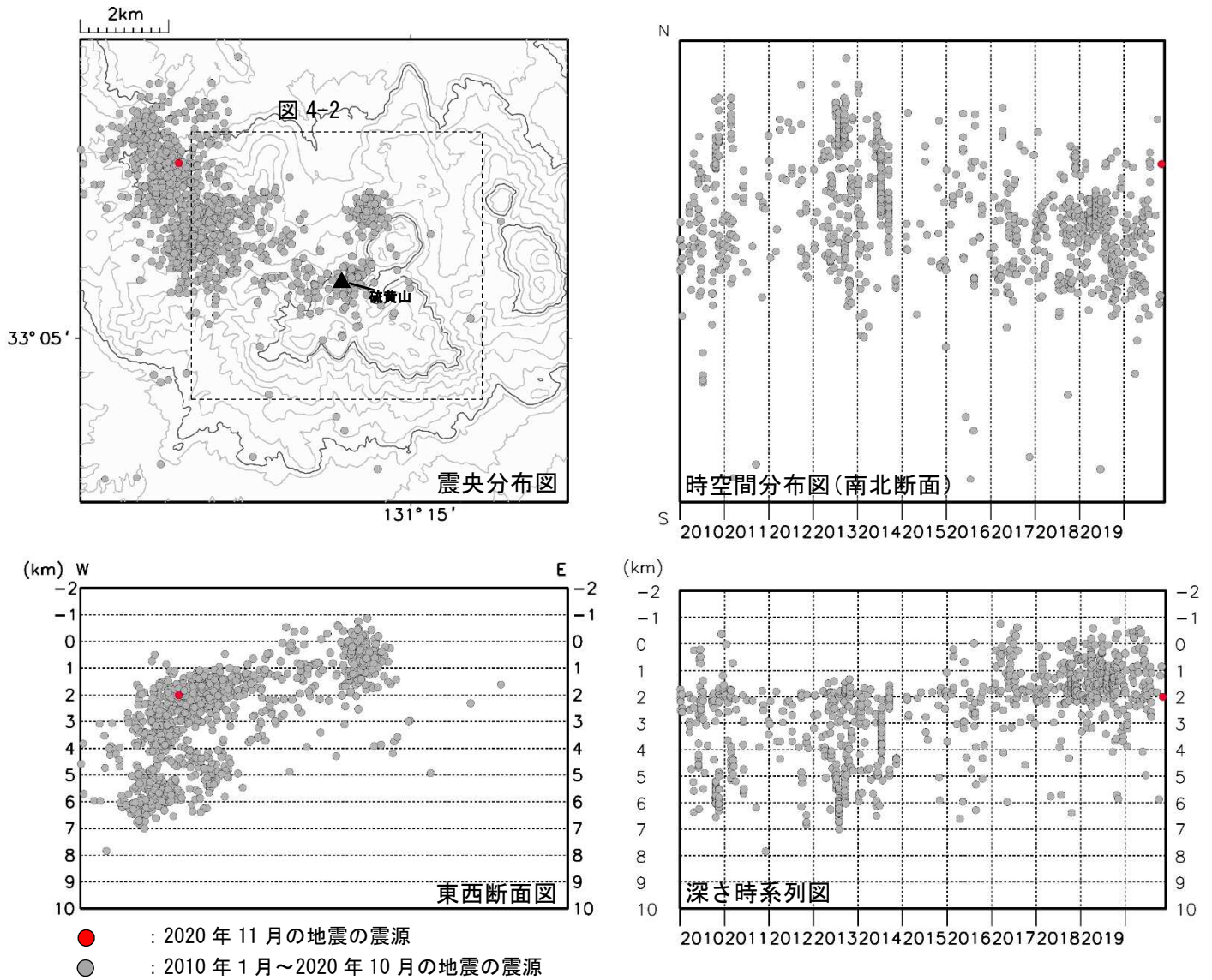
図 4-1 九重山 震源分布図（広域）（2010年1月～2020年11月）
