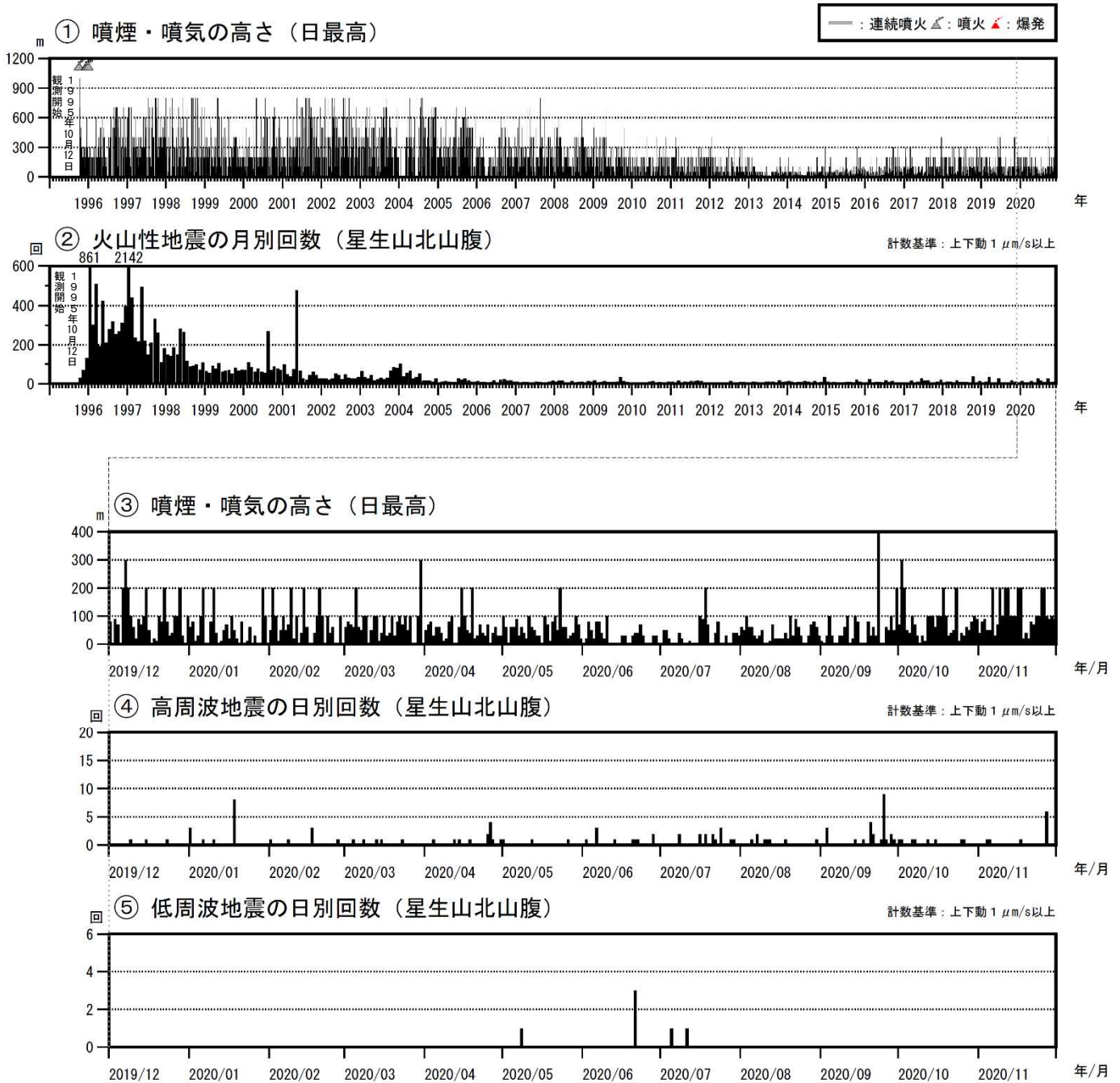
図3 九重山 火山活動経過図（1995年1月～2020年11月）
