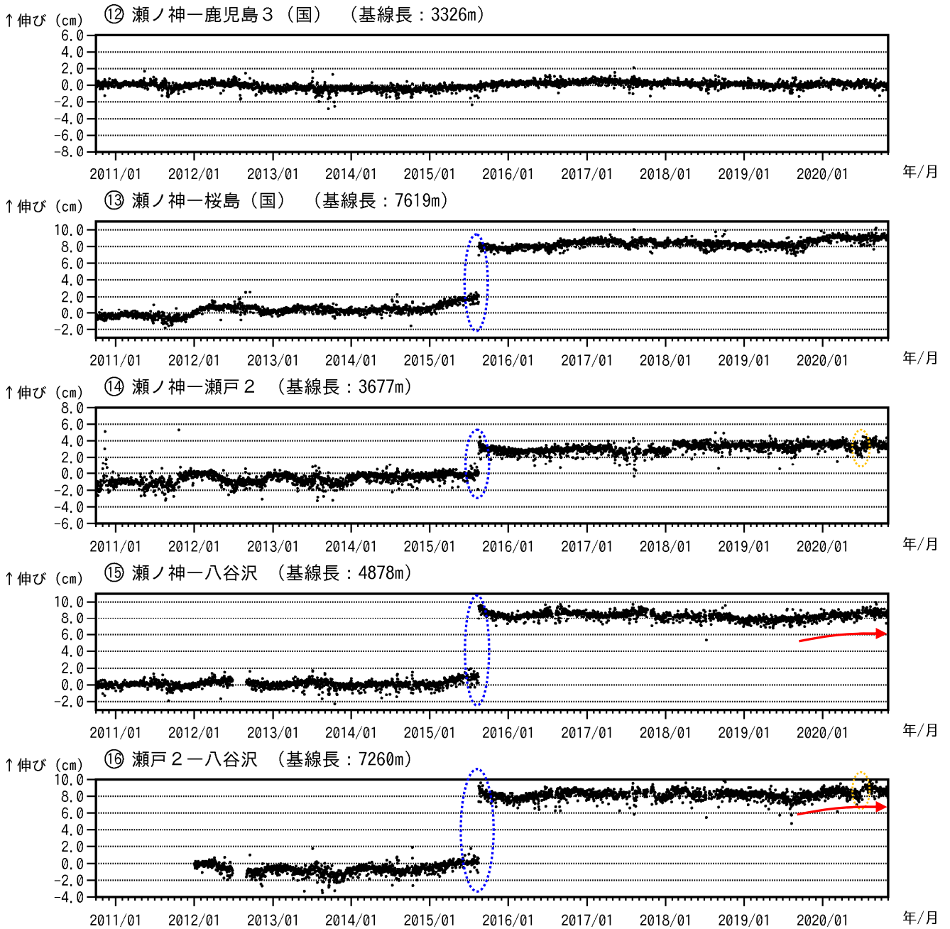
図 8-3 桜島 GNSS 連続観測による基線長変化 (2010 年 10 月～2020 年 10 月)
