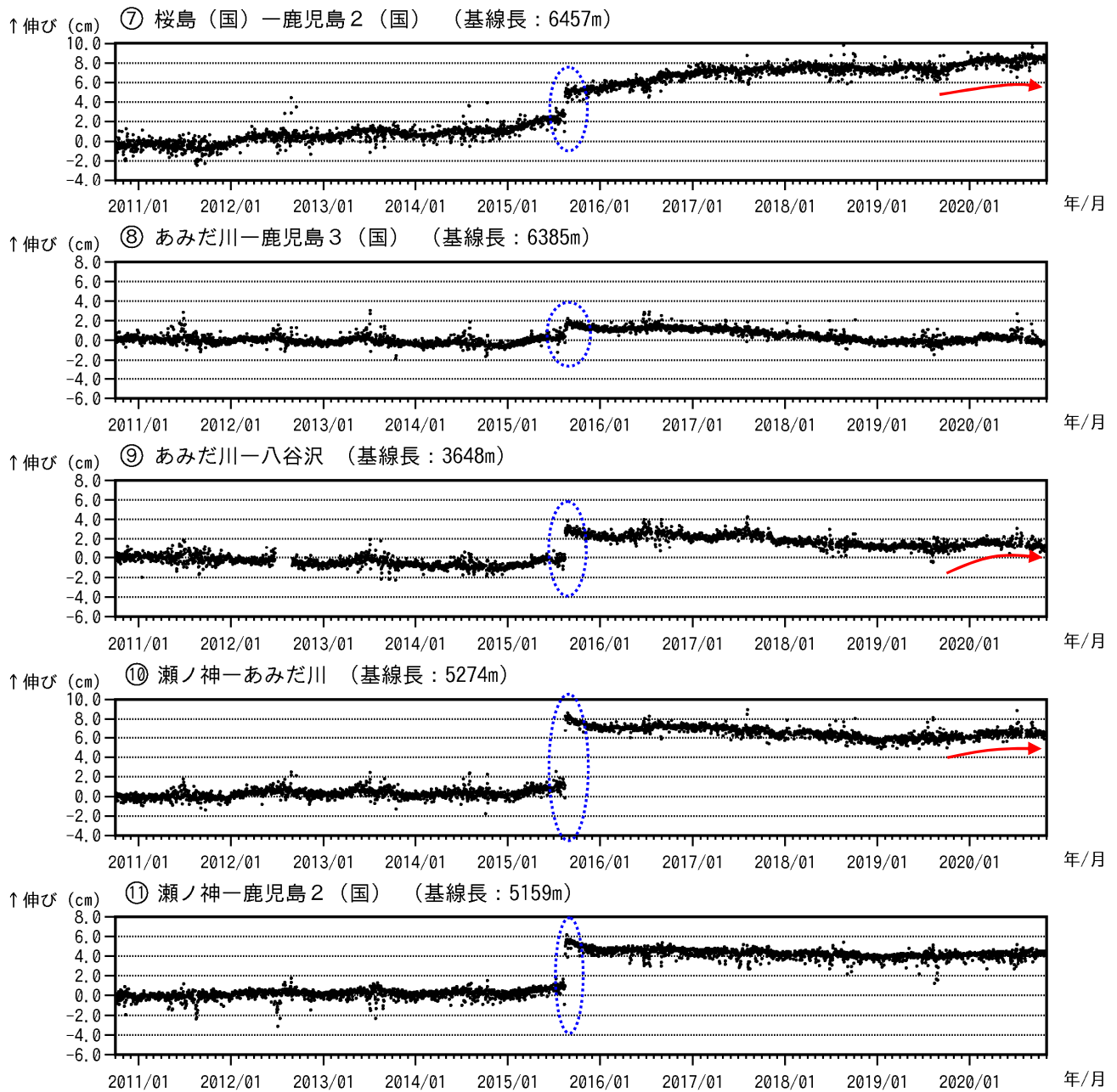
図 8-2 桜島 GNSS 連続観測による基線長変化 (2010 年 10 月～2020 年 10 月)
