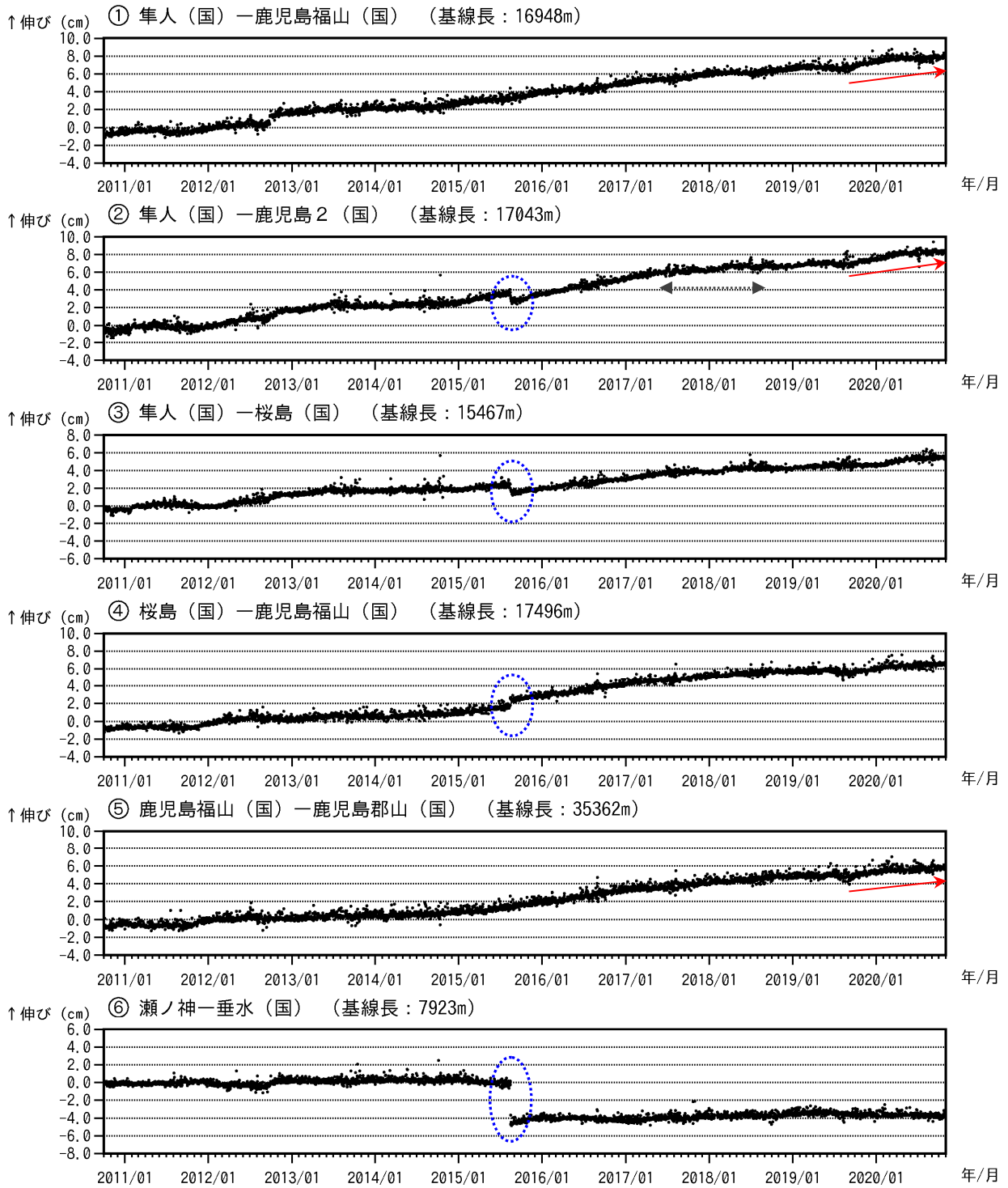
図 8-1 桜島 GNSS 連続観測による基線長変化 (2010 年 10 月～2020 年 10 月)
