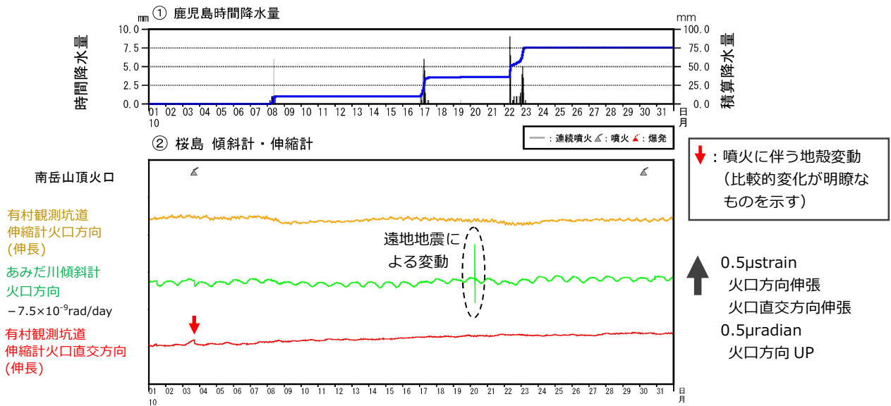
図7 桜島 傾斜計及び伸縮計による地殻変動の状況（2020年10月1日～10月31日）
