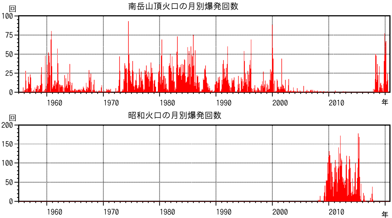
図 5-1 桜島 南岳山頂火口（上図）と昭和火口（下図）の月別爆発回数 （1955年1月～2020年10月）
