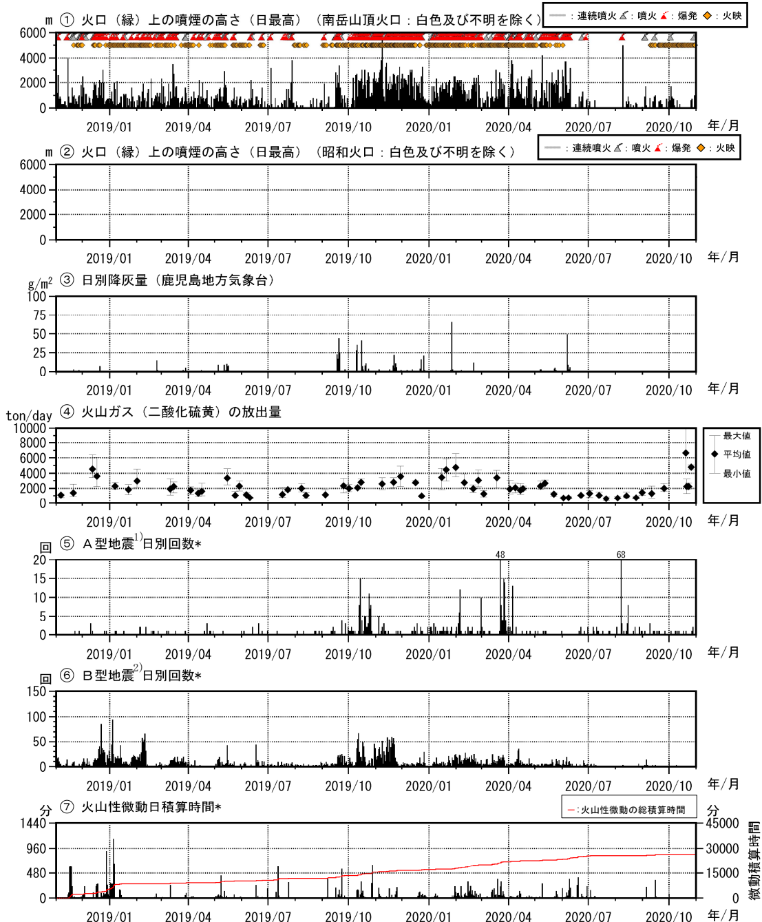
図6 桜島 最近2年間の活動経過図（2018年11月～2020年10月）
