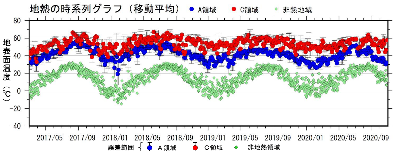
図2-2 九重山 星生山北尾根の赤外熱映像装置による日別最高温度(2017年3月~2020年10月) A領域、C領域ともに非地熱領域と比べて地表面温度が高い状態が続いています。
