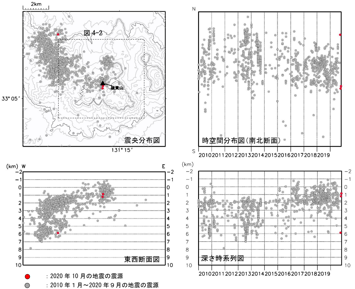
図4-1 九重山 震源分布図（広域）（2010年1月～2020年10月）
