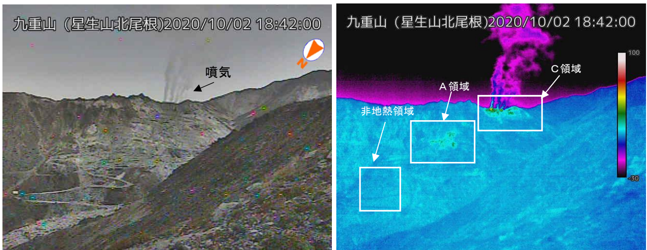
図2-1 九重山 噴気および地熱域の状況 (10月2日 星生山北尾根監視カメラ (左) 及び赤外熱映像装置による (右))
