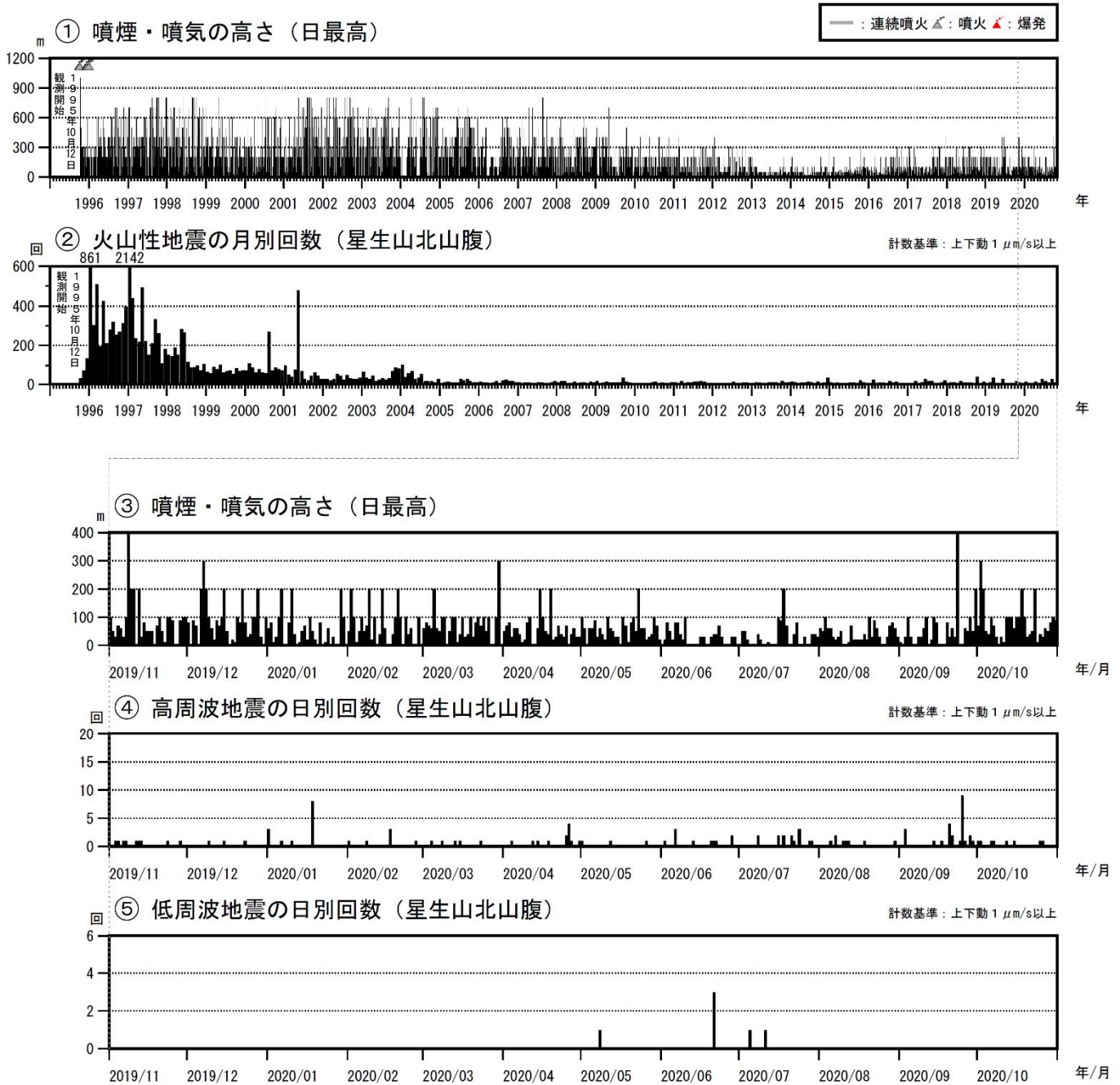
図3 九重山 火山活動経過図（1995年1月～2020年10月）
