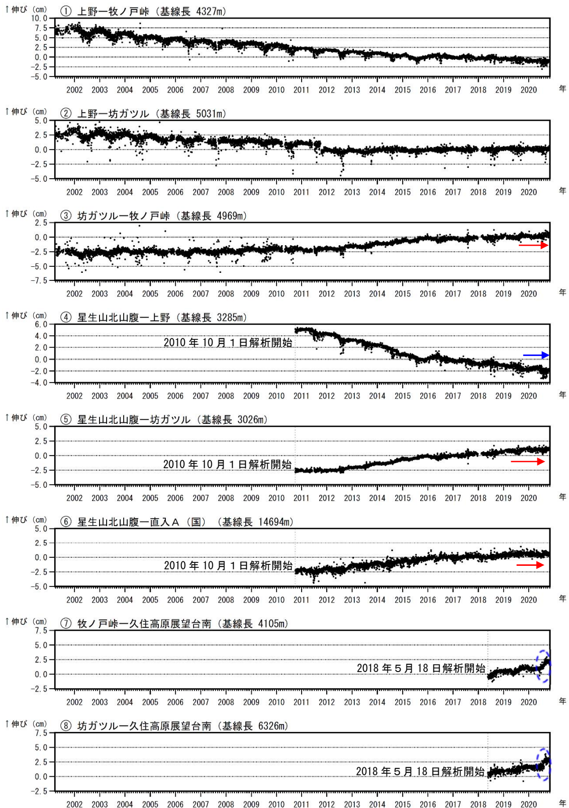
図8 九重山 GNSS連続観測による基線長変化（2001年4月～2020年10月）
