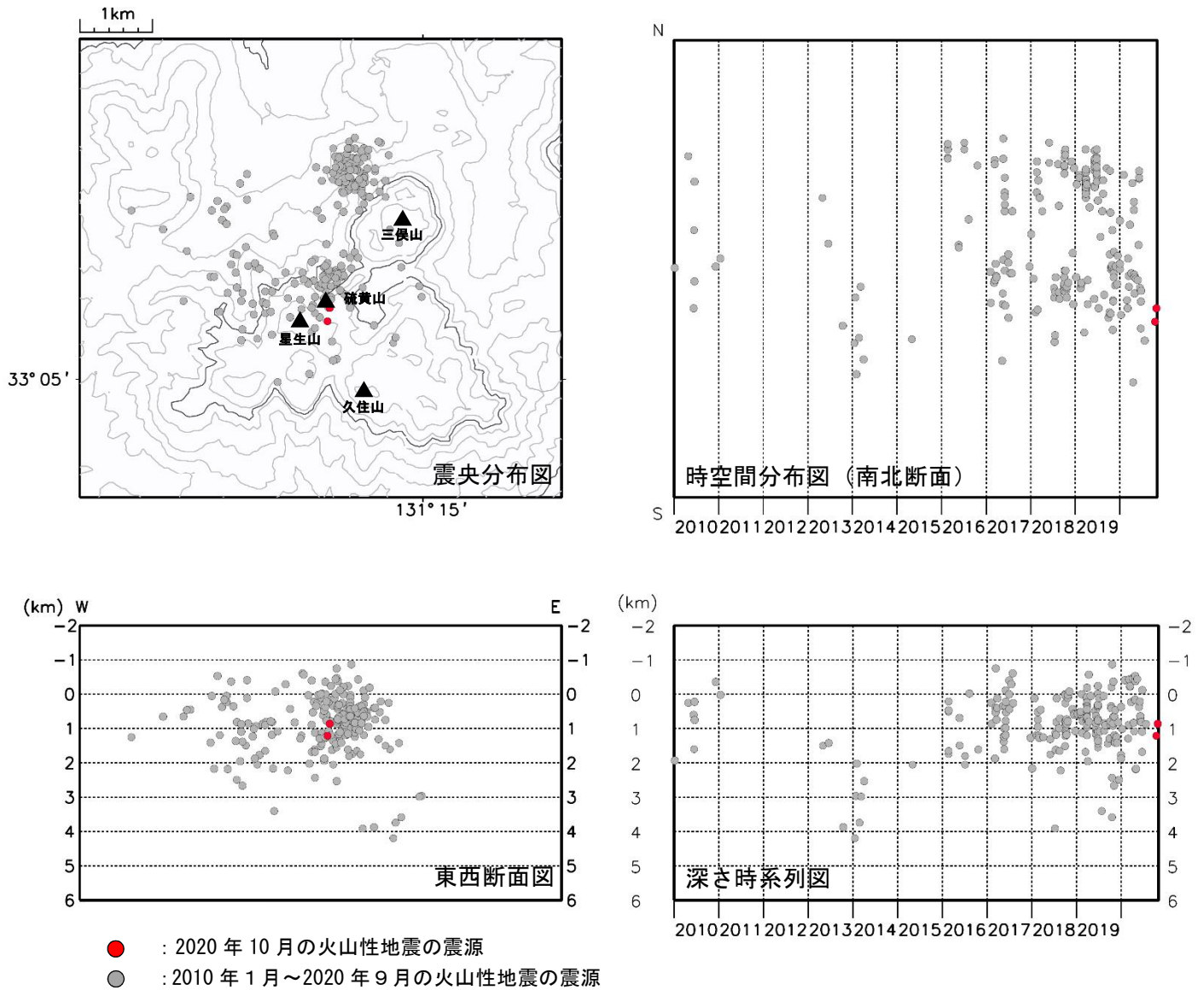
図 4-2 九重山 震源分布図（硫黄山付近の火山性地震）（2010年1月～2020年10月）
