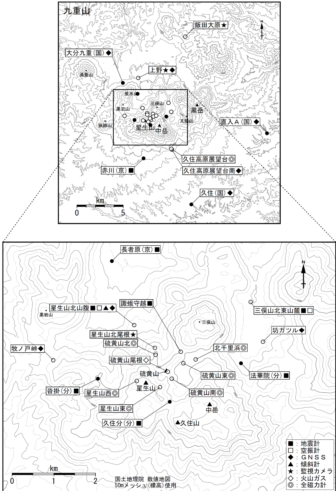
図10 九重山 観測点配置図
