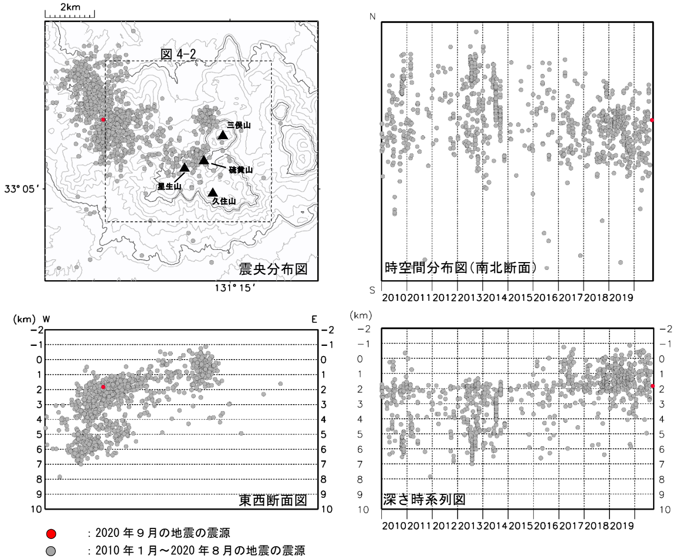
図 4-1 九重山 震源分布図（広域）（2010年1月～2020年9月）
