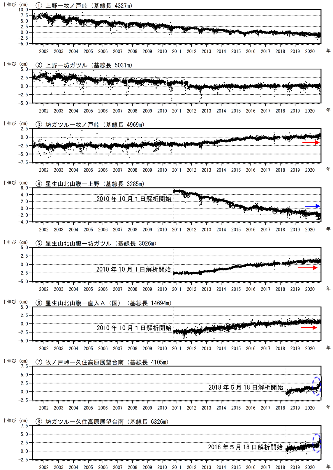
図8 九重山 GNSS連続観測による基線長変化（2001年4月～2020年9月）
