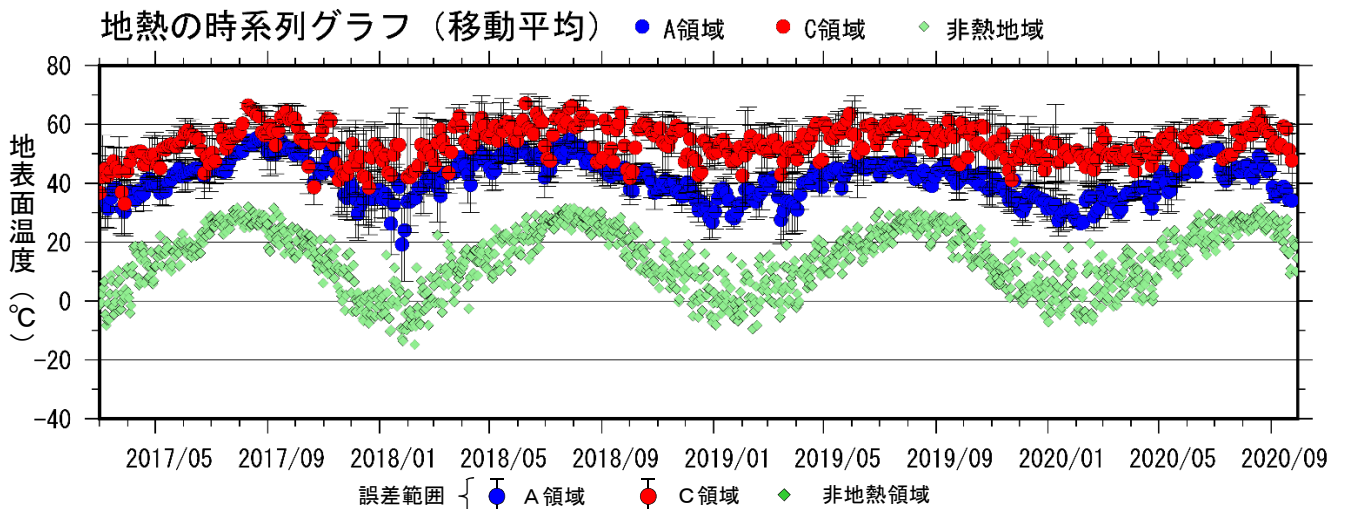
図2-2 九重山 星生山北尾根の赤外熱映像装置による日別最高温度（2017年3月～2020年9月） A領域、C領域ともに非地熱領域と比べて地表面温度が高い状態が続いています。
