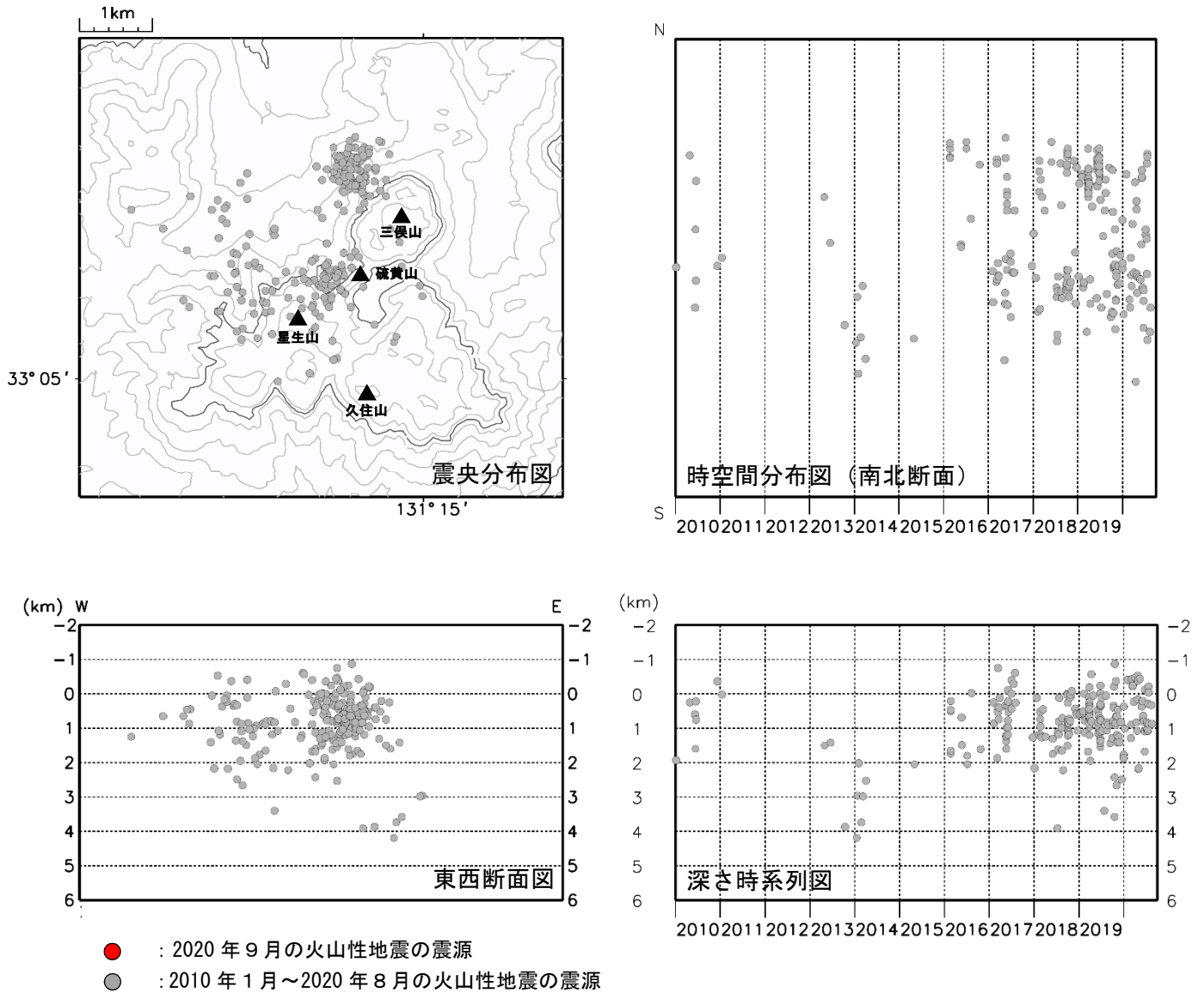
図 4-2 九重山 震源分布図（硫黄山付近の火山性地震）（2010年1月～2020年9月）
