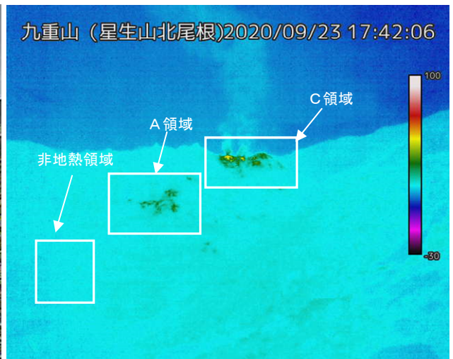
図2-1 九重山 噴気および地熱域の状況 （9月23日 星生山北尾根監視カメラ（左）及び赤外熱映像装置による（右））
