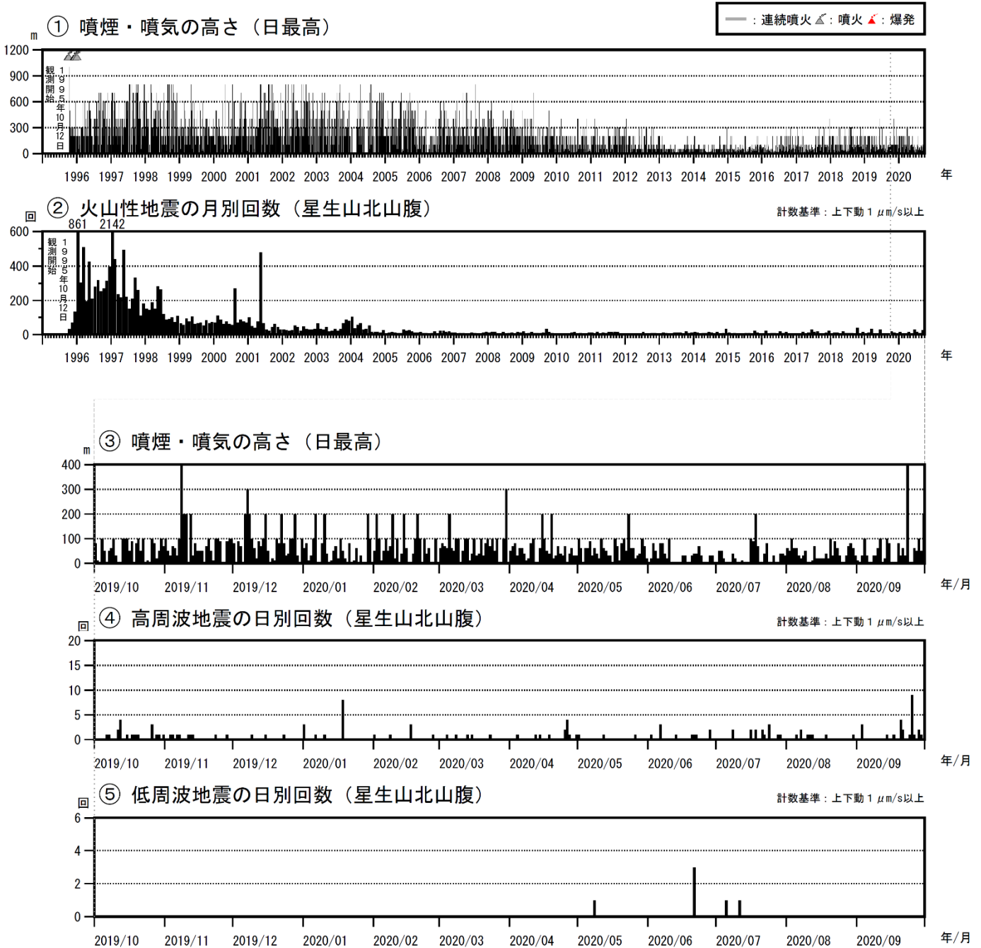
図3 九重山 火山活動経過図（1995年1月～2020年9月）
