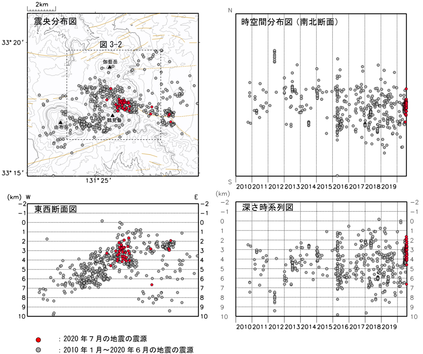
図3-1 鶴見岳・伽藍岳 震源分布図（広域）（2010年1月～2020年7月）
