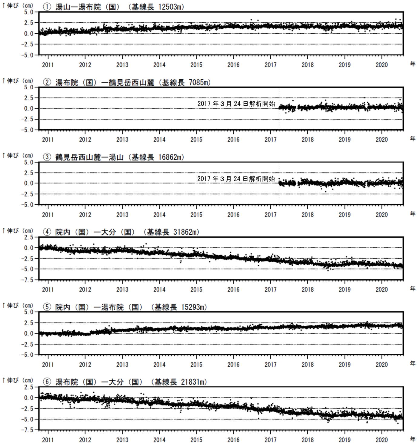
図4 鶴見岳・伽藍岳 GNSS連続観測による基線長変化（2010年10月～2020年7月）
