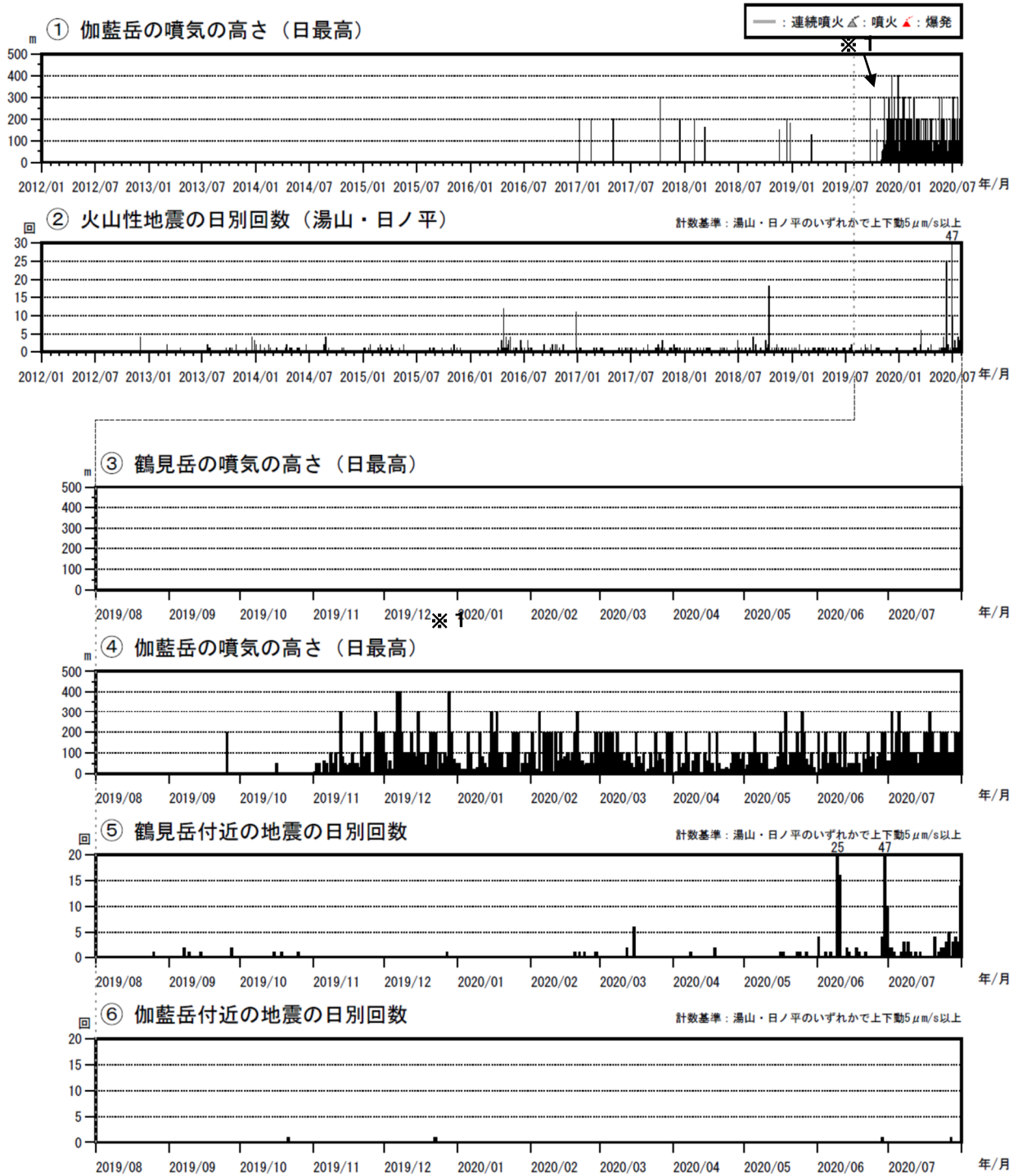
図2 鶴見岳・伽藍岳 火山活動経過図（2012年1月～2020年7月）
