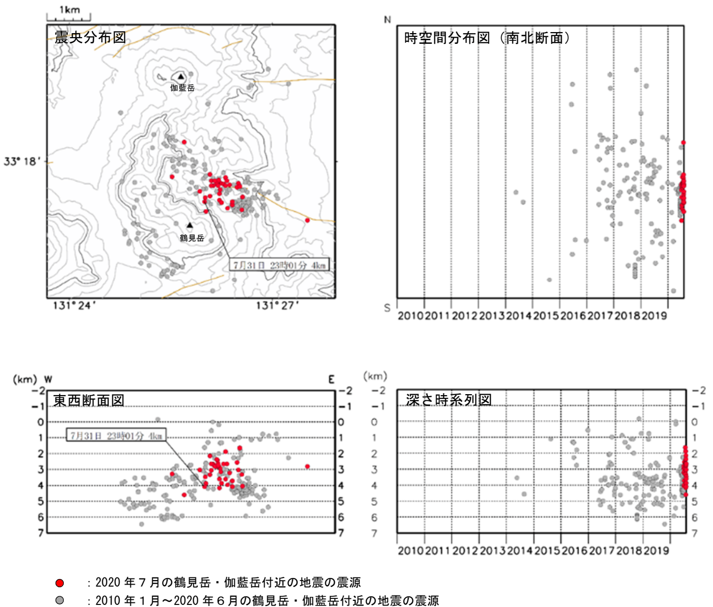
図 3-2 鶴見岳・伽藍岳 震源分布図（鶴見岳・伽藍岳付近の地震）（2010年1月～2020年7月）
