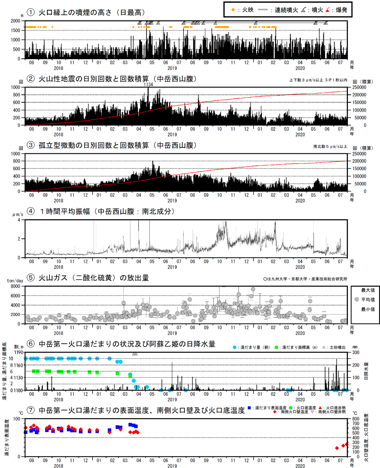
図8 阿蘇山 火山活動経過図（2018年8月～2020年7月）
