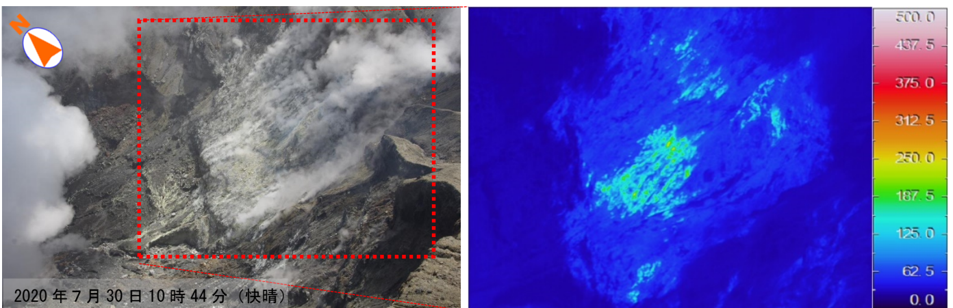
図7 阿蘇山 中岳第一火口内南側火口壁（中岳第一火口の南西側から観測）
