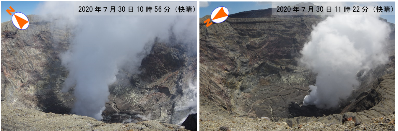
図5 阿蘇山 噴煙の状況
