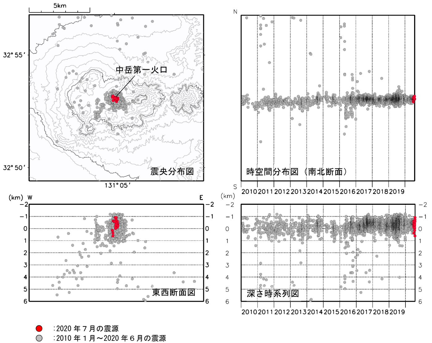
図11 阿蘇山 火山性地震の震源分布（2010年1月～2020年7月）
