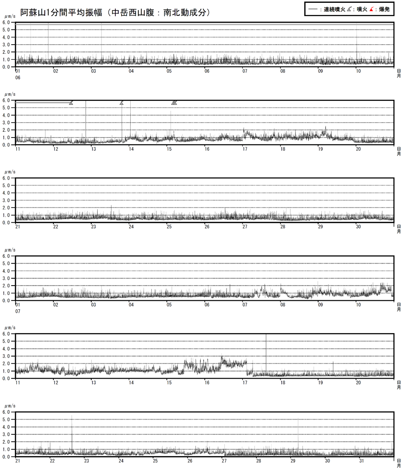
図10 阿蘇山 1分間平均振幅の時間変化（中岳西山腹観測点南北動成分、2020年6月～7月）
