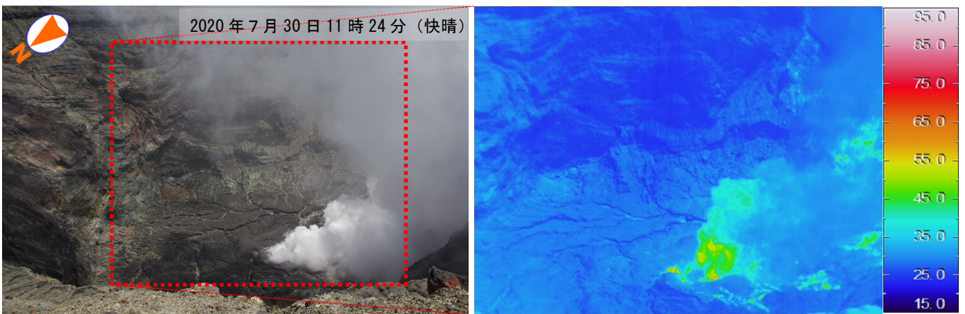
図6 阿蘇山 中岳第一火口内191火孔の状況（中岳第一火口の北西側から観測）
