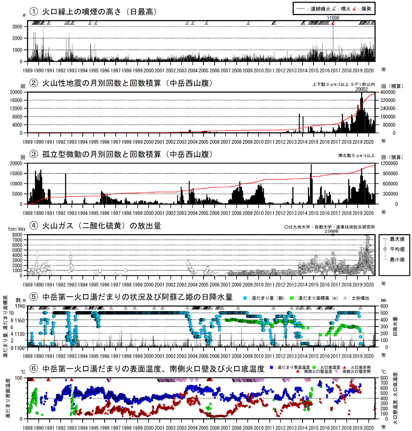
図9 阿蘇山 火山活動経過図（1989年1月～2020年7月）
