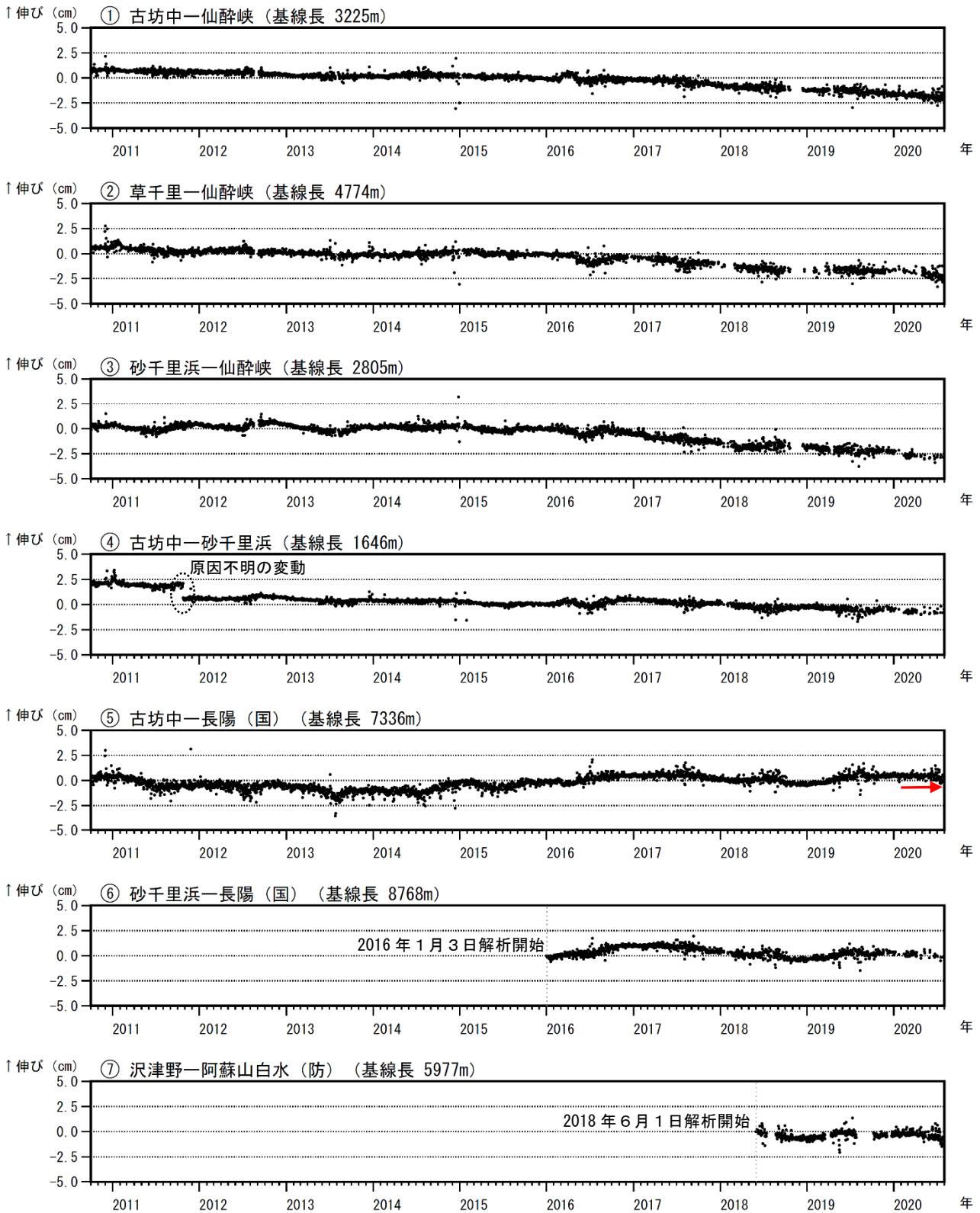
図 12 阿蘇山 GNSS 観測による基線長変化（2010年10月～2020年7月）
