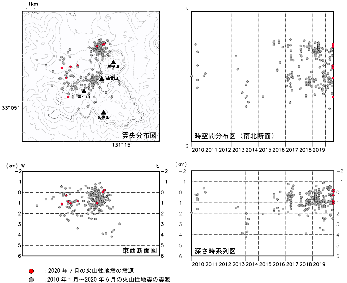
図 4-2 九重山 震源分布図（硫黄山付近の火山性地震）（2010年1月～2020年7月）
