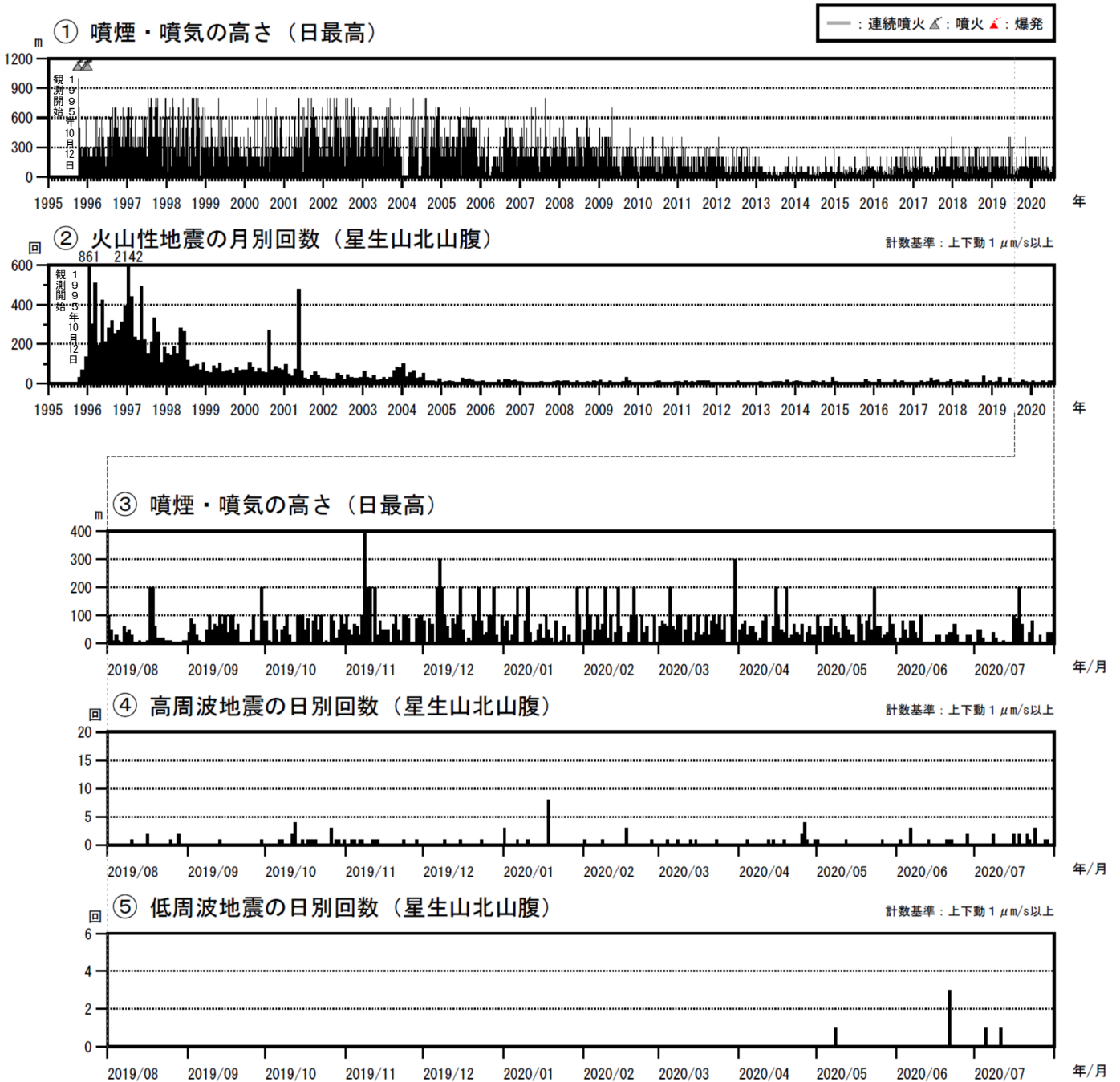
図3 九重山 火山活動経過図（1995年1月～2020年7月）
