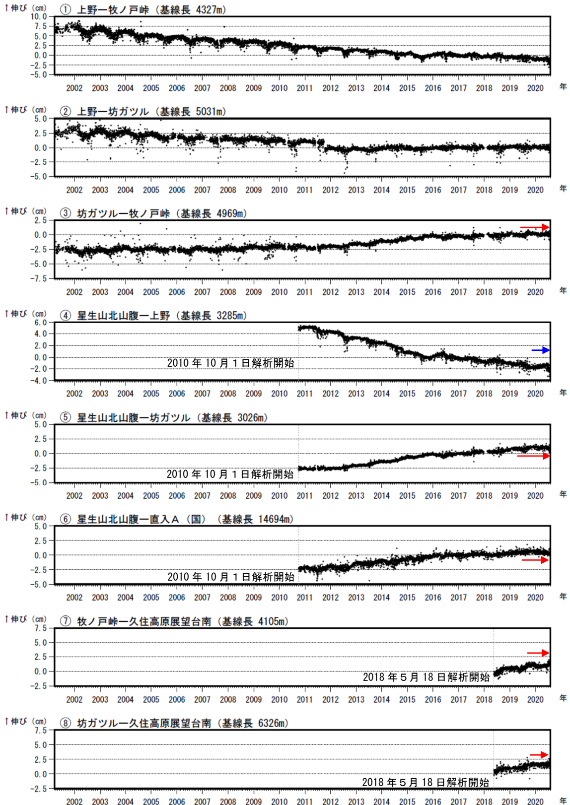
図8 九重山 GNSS連続観測による基線長変化（2001年4月～2020年7月）
