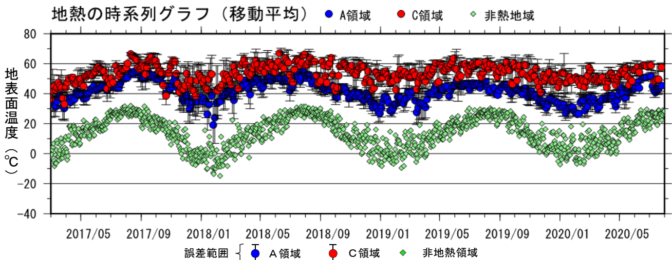
図2-2 九重山 星生山北尾根の赤外熱映像装置による日別最高温度（2017年3月～2020年7月） A領域、C領域ともに非地熱領域と比べて地表面温度が高い状態が続いています。
