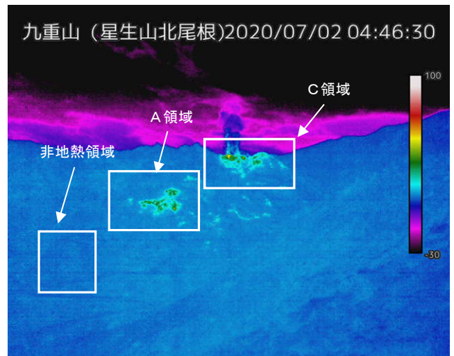
図2-1 九重山 噴気および地熱域の状況 （7月2日 星生山北尾根監視カメラ（左）及び赤外熱映像装置による（右））
