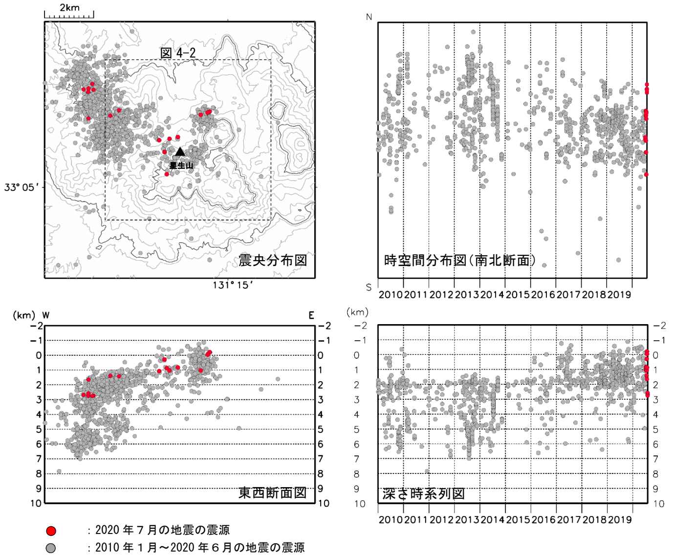
図 4-1 九重山 震源分布図（広域）（2010年1月～2020年7月）
