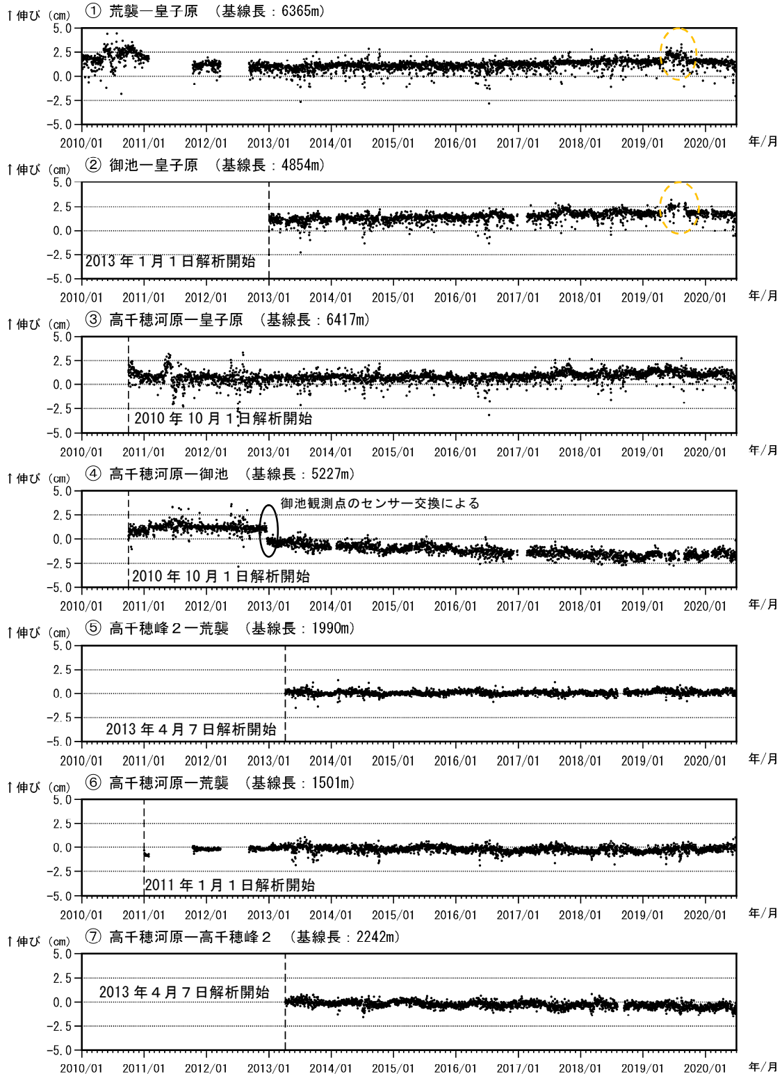
図4 霧島山（御鉢） GNSS連続観測による基線長変化（2010年1月～2020年6月）
