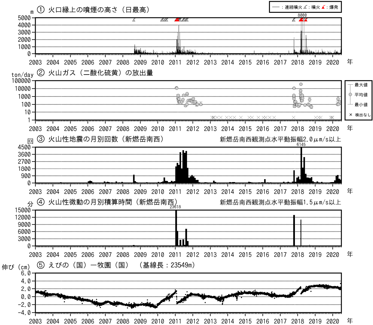
図3 霧島山（新燃岳） 火山活動経過図（2003年1月～2020年6月）
