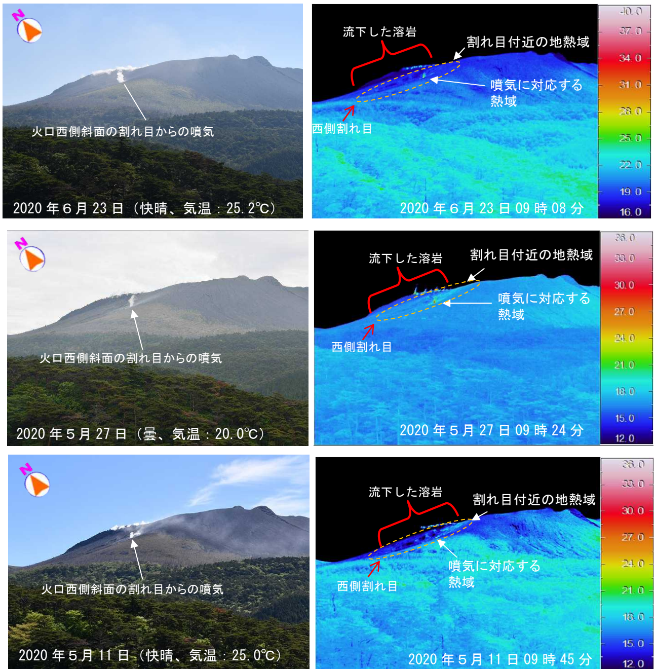
図2 霧島山（新燃岳） 新燃岳南西側斜面の状況（6月23日、新湯温泉付近から観測） 流下した溶岩の上部及び火口西側斜面の割れ目で、前回（5月27日）の観測と同様に噴気を確認しました。また、割れ目付近では引き続き地熱域を確認しました。
