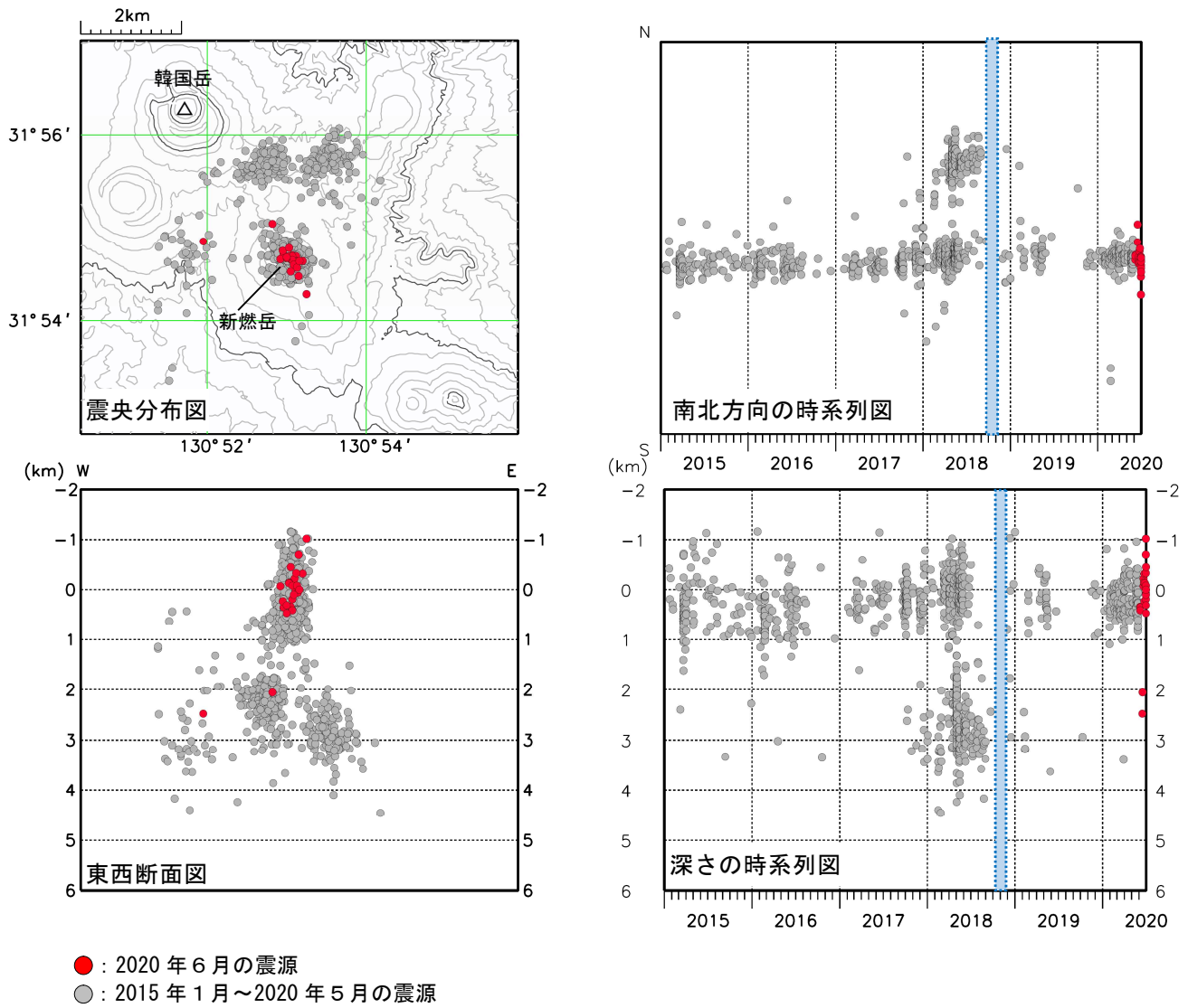
図7 霧島山（新燃岳） 震源分布図（2015年1月～2020年6月）
