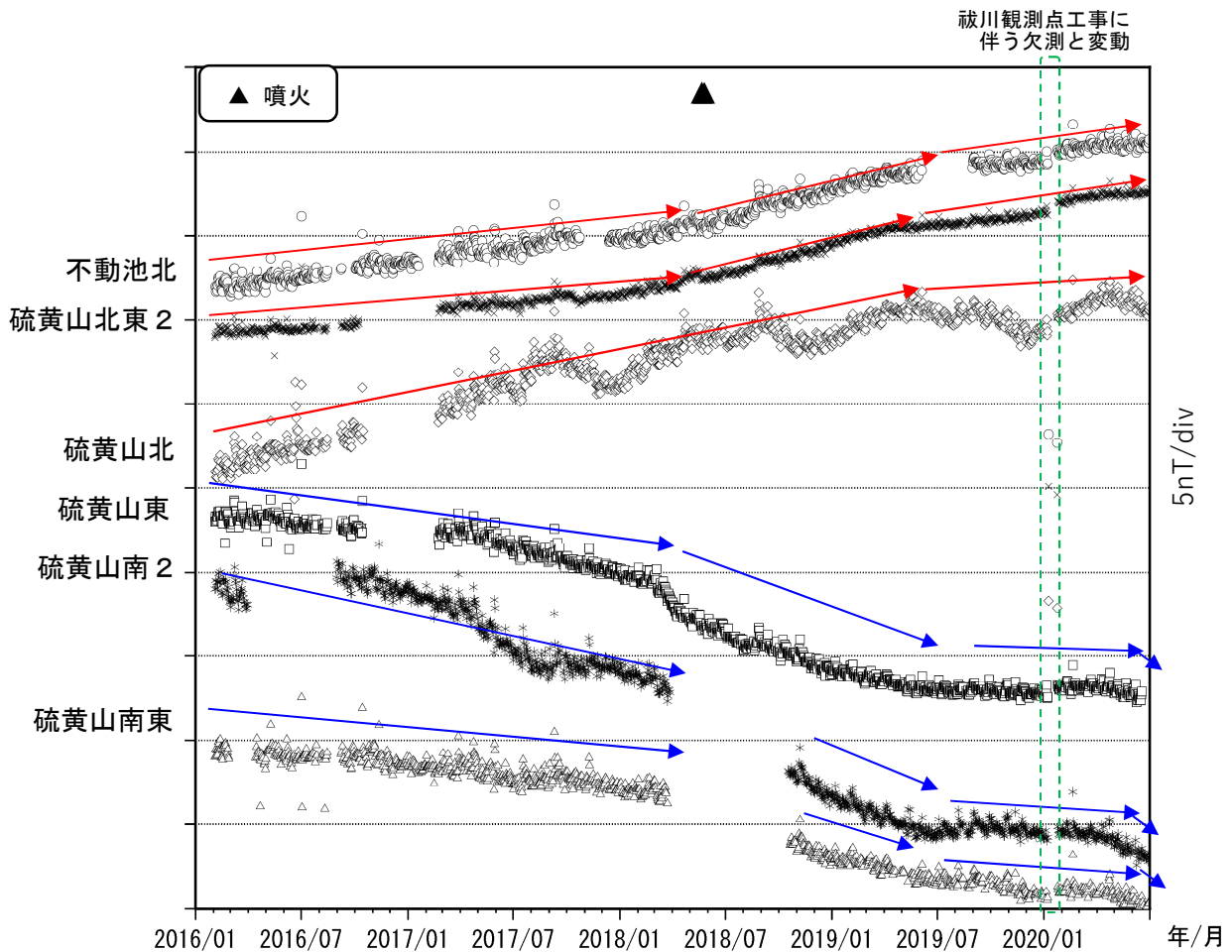
図 12 霧島山（えびの高原（硫黄山）周辺） 全磁力観測点で観測された全磁力変動（2016年2月～2020年6月）
