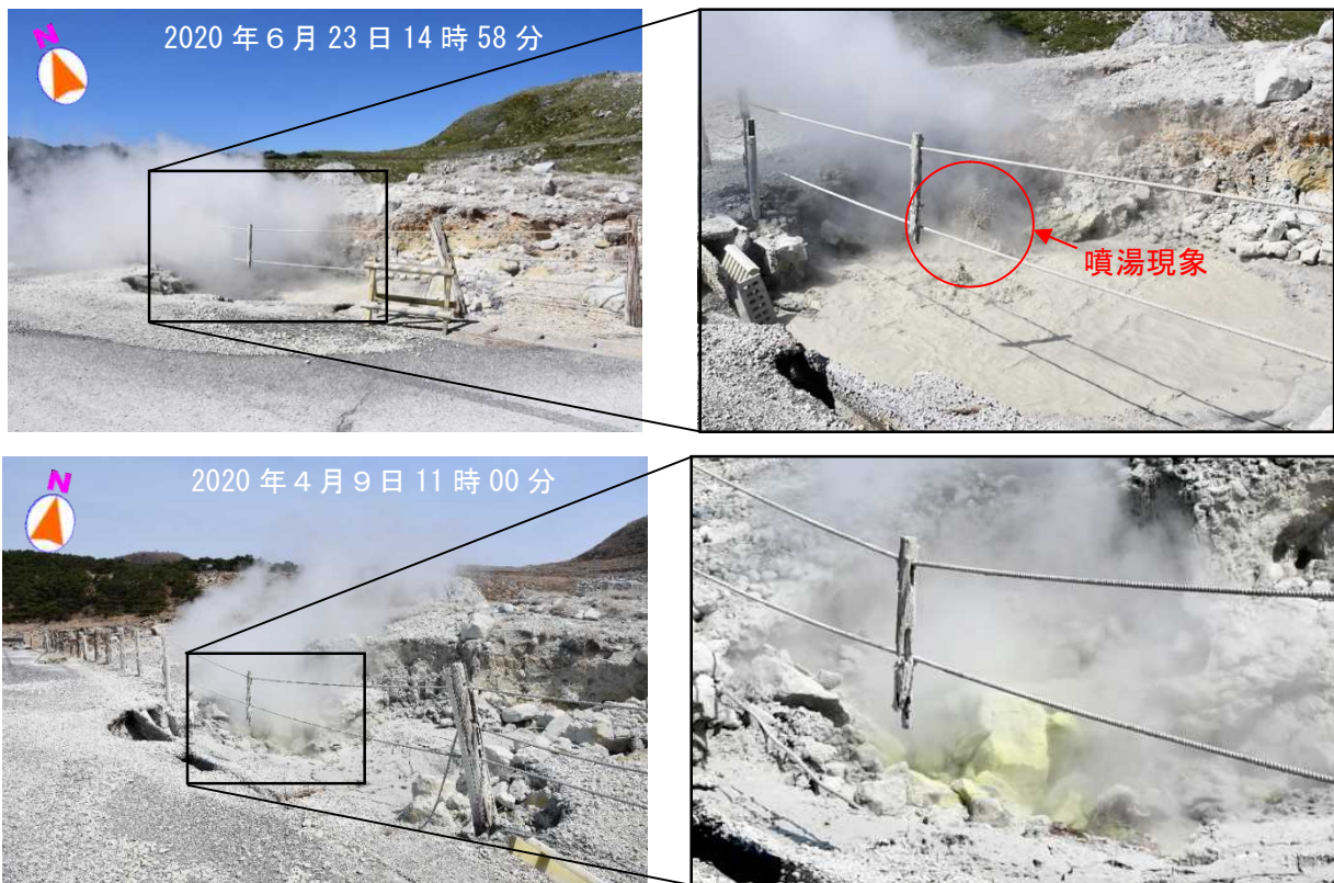
図 2-2 霧島山（えびの高原（硫黄山）周辺） 硫黄山西側 500mの噴気の状態
