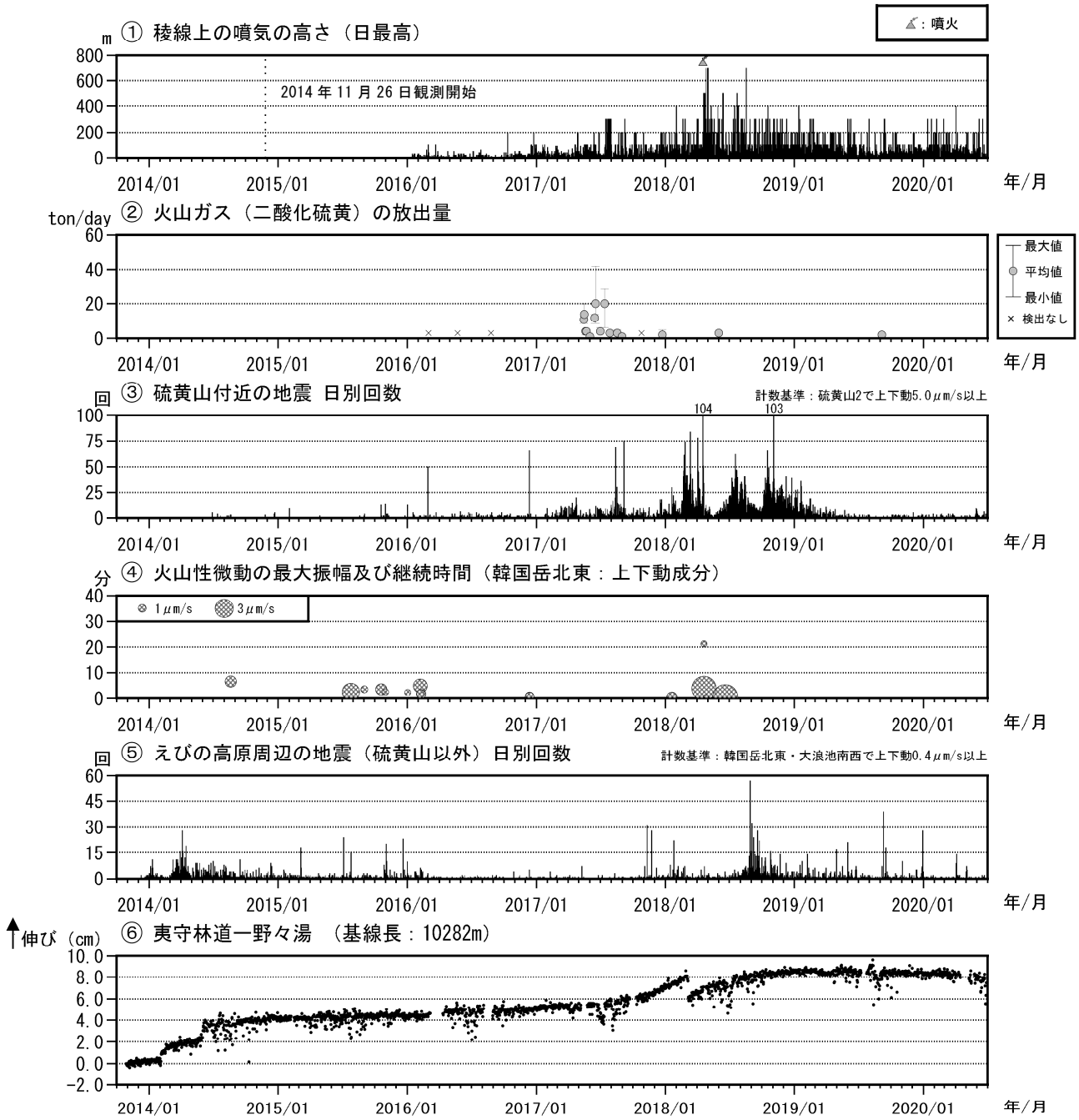
図6 霧島山（えびの高原（硫黄山）周辺）火山活動経過図（2014年1月～2020年6月）
