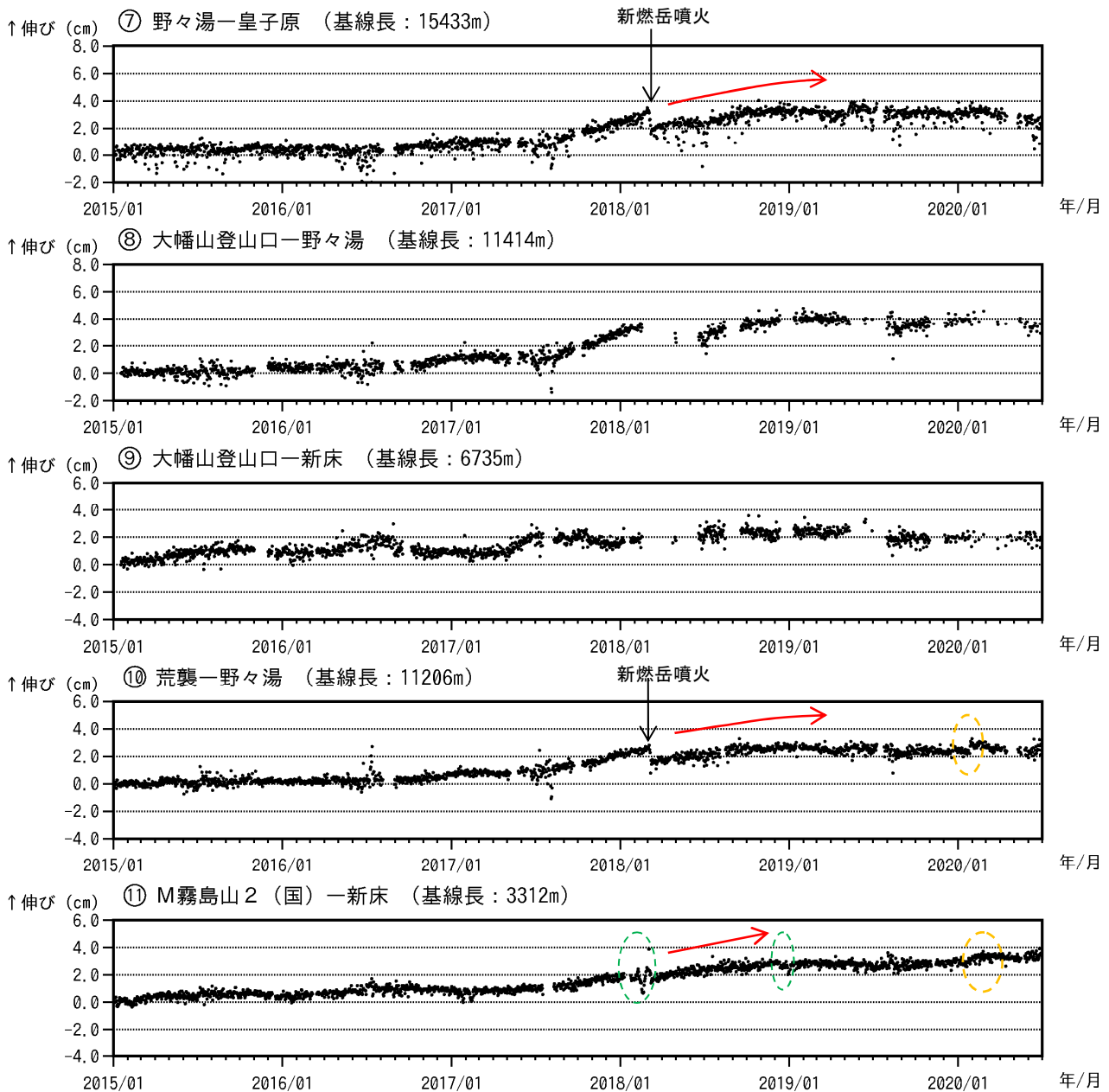
図 8-2 霧島山（新燃岳） GNSS 連続観測による基線長変化（2015 年 1 月～2020 年 6 月）
