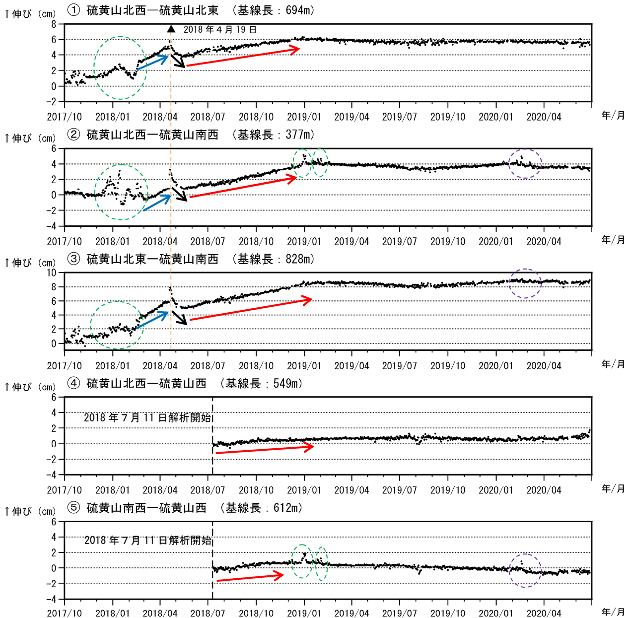
図7 霧島山（えびの高原（硫黄山）周辺） GNSS 連続観測による基線長変化 （2017年10月～2020年6月）
