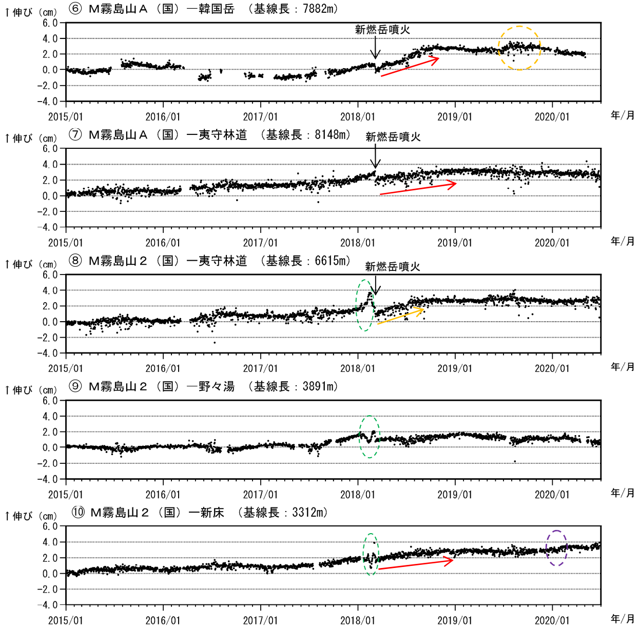
図 8-2 霧島山（えびの高原（硫黄山）周辺） GNSS 連続観測による基線長変化 (2015年1月～2020年6月)
