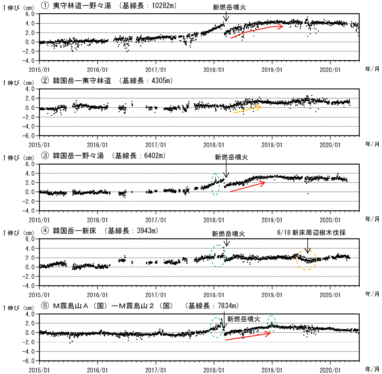
図 8-1 霧島山 (えびの高原 (硫黄山) 周辺) GNSS 連続観測による基線長変化 (2015年1月~2020年6月)
