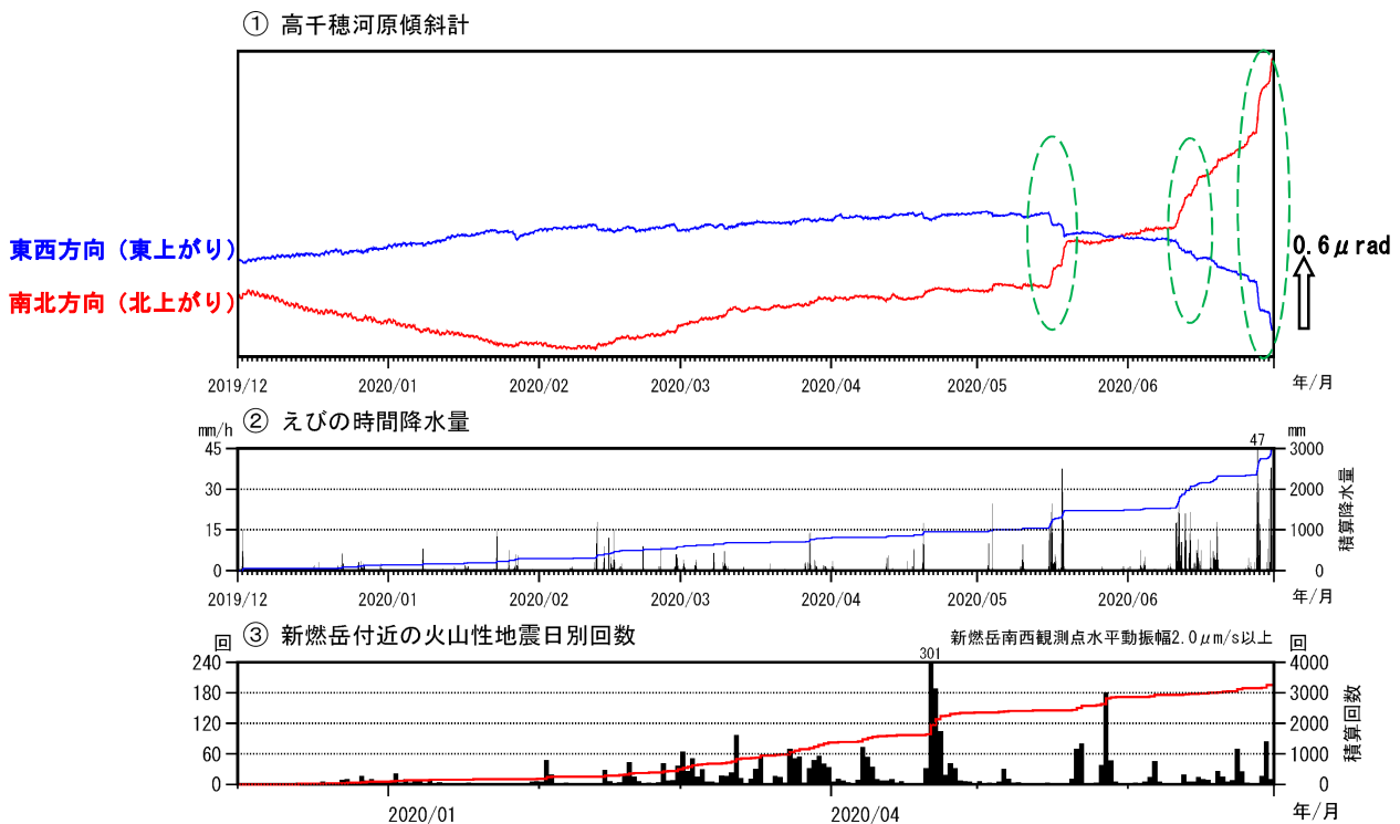
図6 霧島山（新燃岳） 高千穂河原観測点の傾斜変動の状況（2019年12月～2020年6月）
