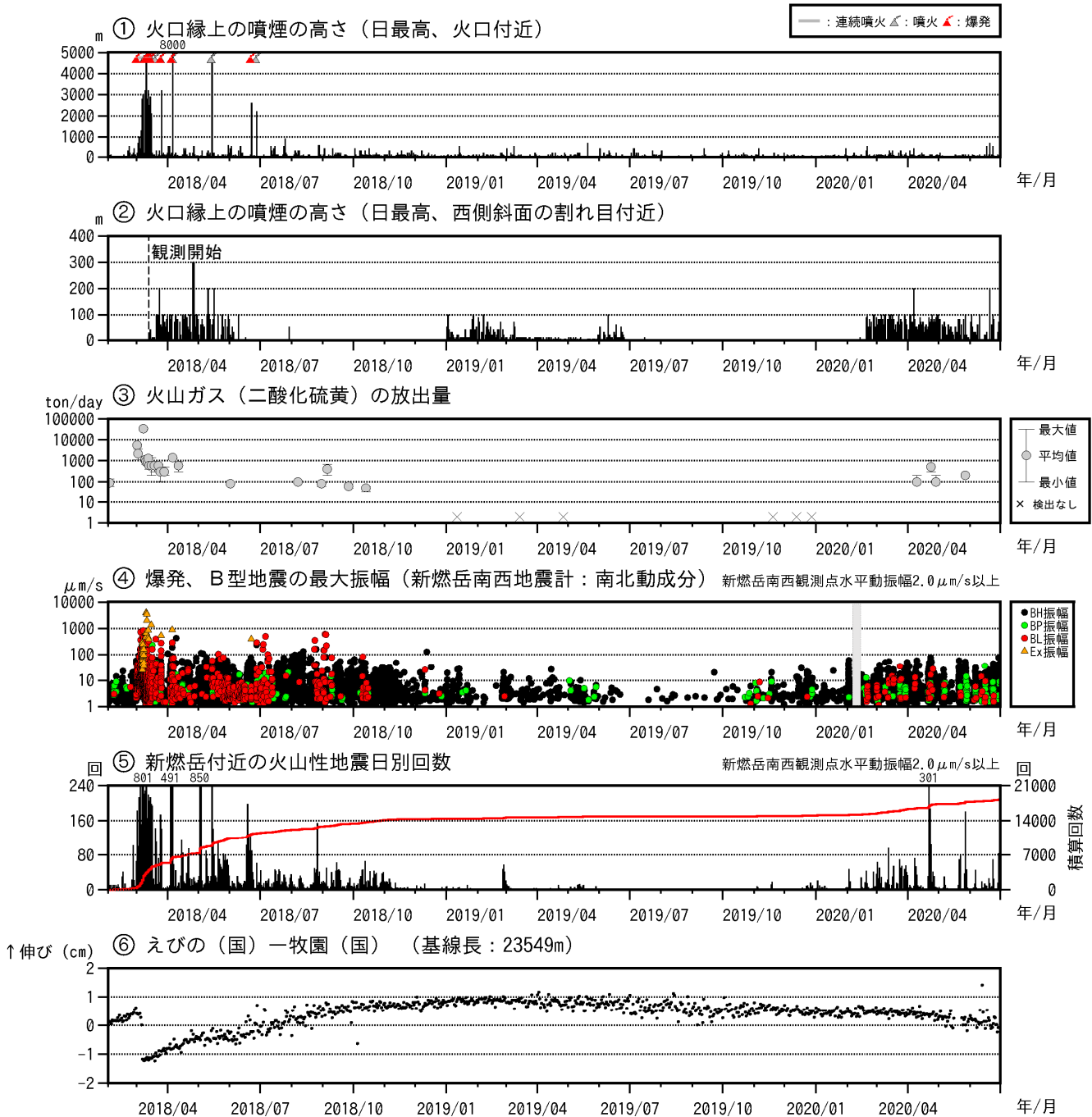
図4 霧島山（新燃岳） 火山活動経過図（2018年2月～2020年6月）
