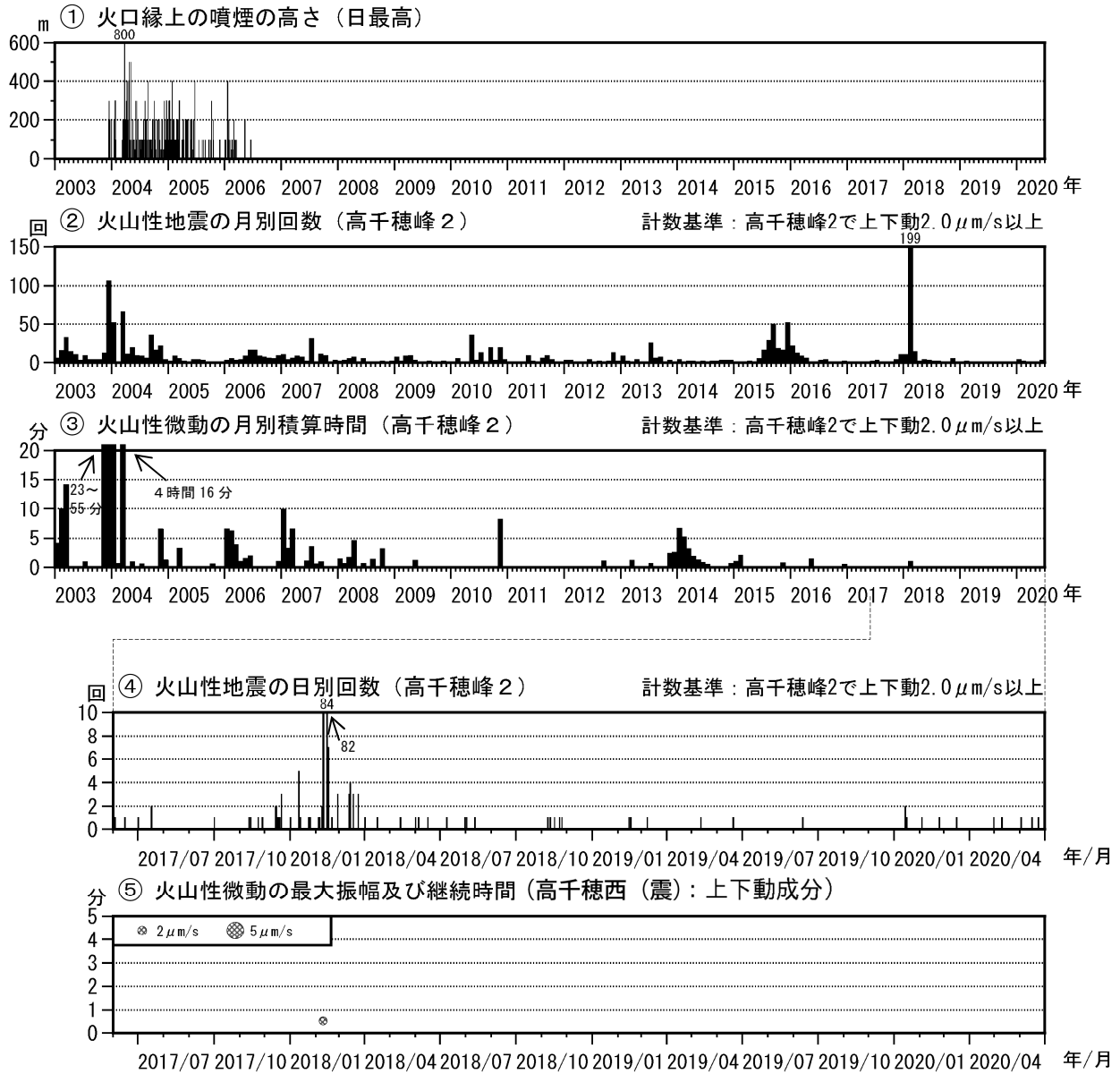
図2 霧島山（御鉢） 火山活動経過図（2003年1月～2020年6月）
