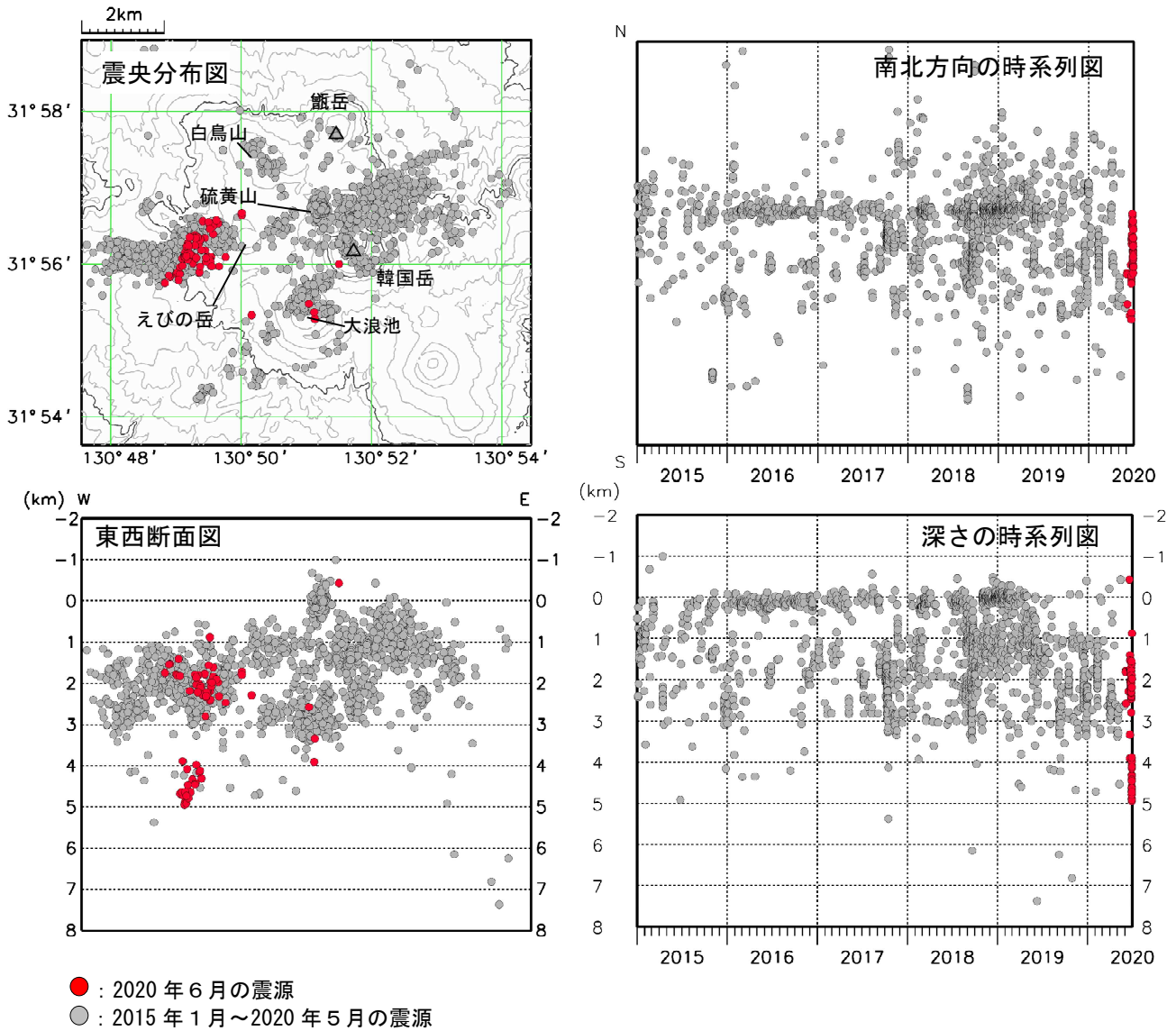
図4 霧島山（えびの高原（硫黄山）周辺） 震源分布図（2015年1月～2020年6月）
