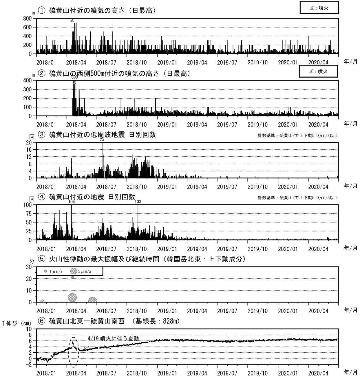
図5 霧島山（えびの高原（硫黄山）周辺） 火山活動経過図（2018年1月～2020年6月）
