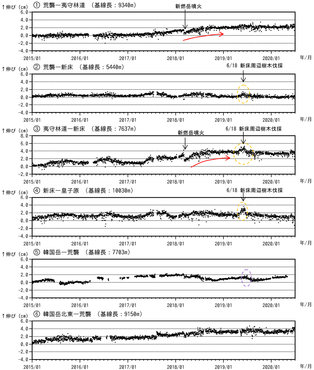
図 8-1 霧島山（新燃岳） GNSS 連続観測による基線長変化（2015 年 1 月～2020 年 6 月）
