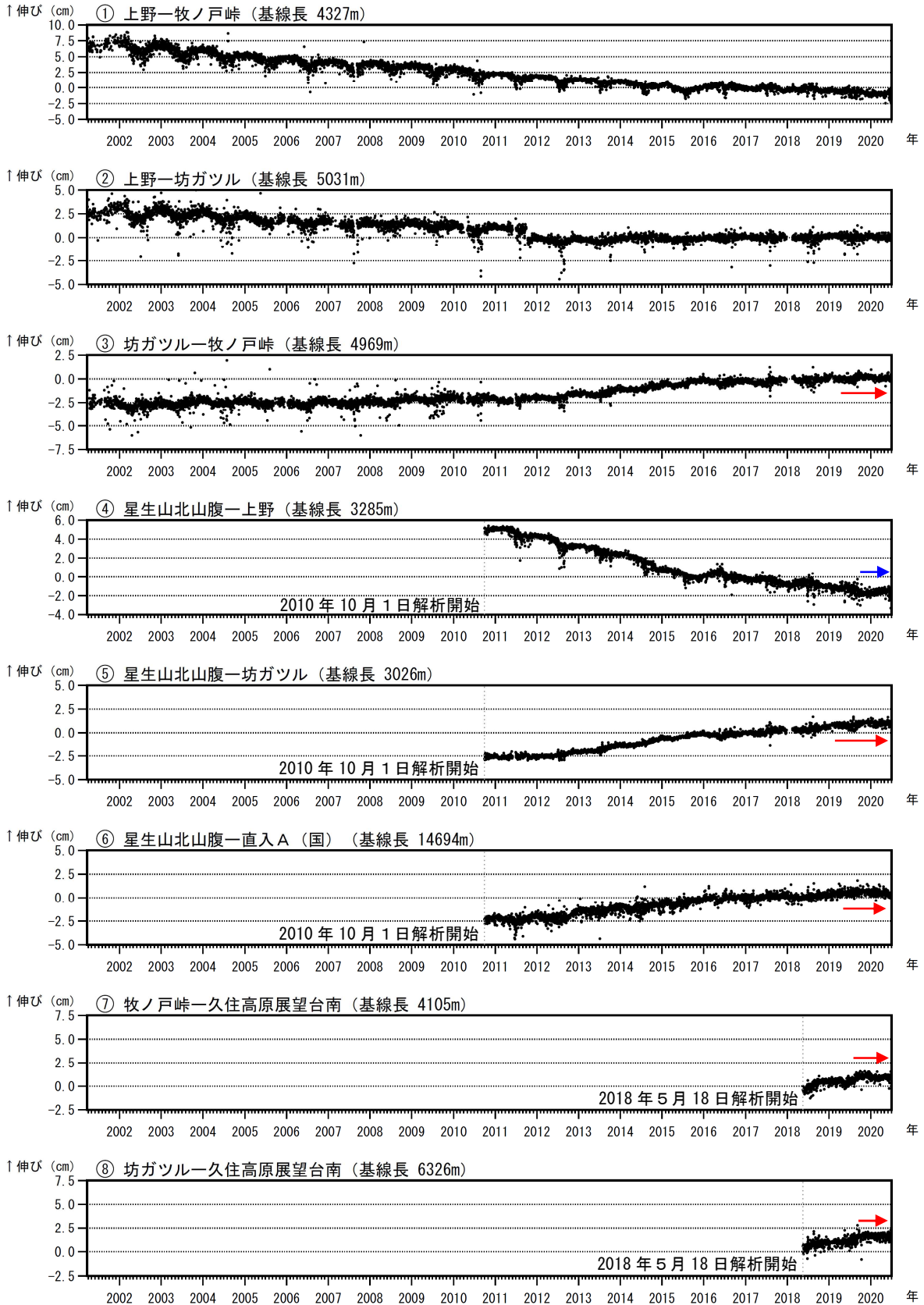
図8 九重山 GNSS連続観測による基線長変化（2001年4月～2020年6月）
