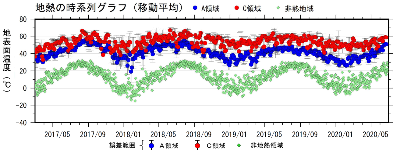
図2-2 九重山 星生山北尾根の赤外熱映像装置による日別最高温度（2017年3月～2020年6月） A領域、C領域ともに非地熱領域と比べて地表面温度が高い状態が続いています。
