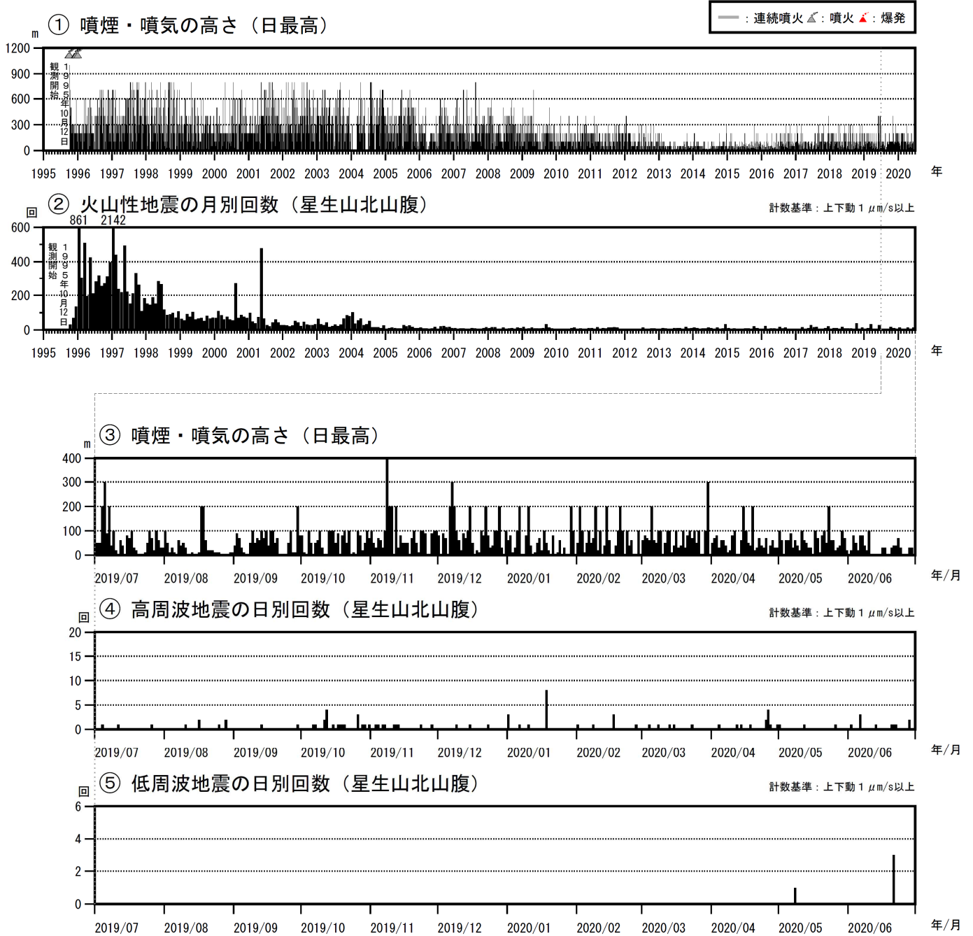
図3 九重山 火山活動経過図（1995年1月～2020年6月）
