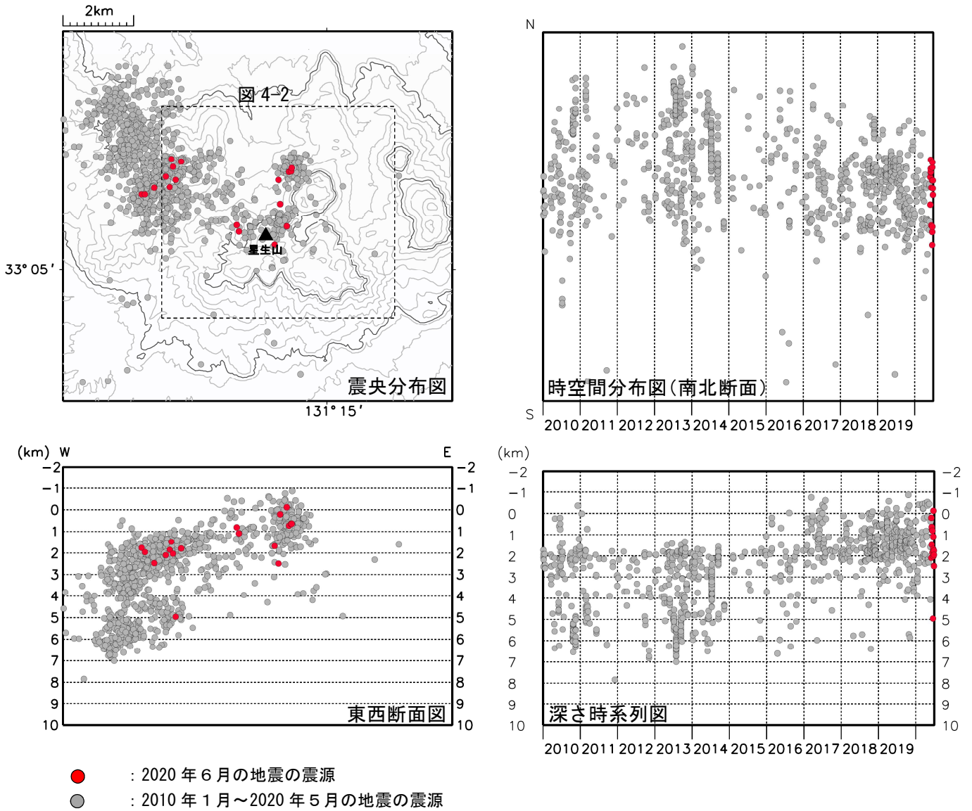
図 4-1 九重山 震源分布図（広域）（2010年1月～2020年6月）
