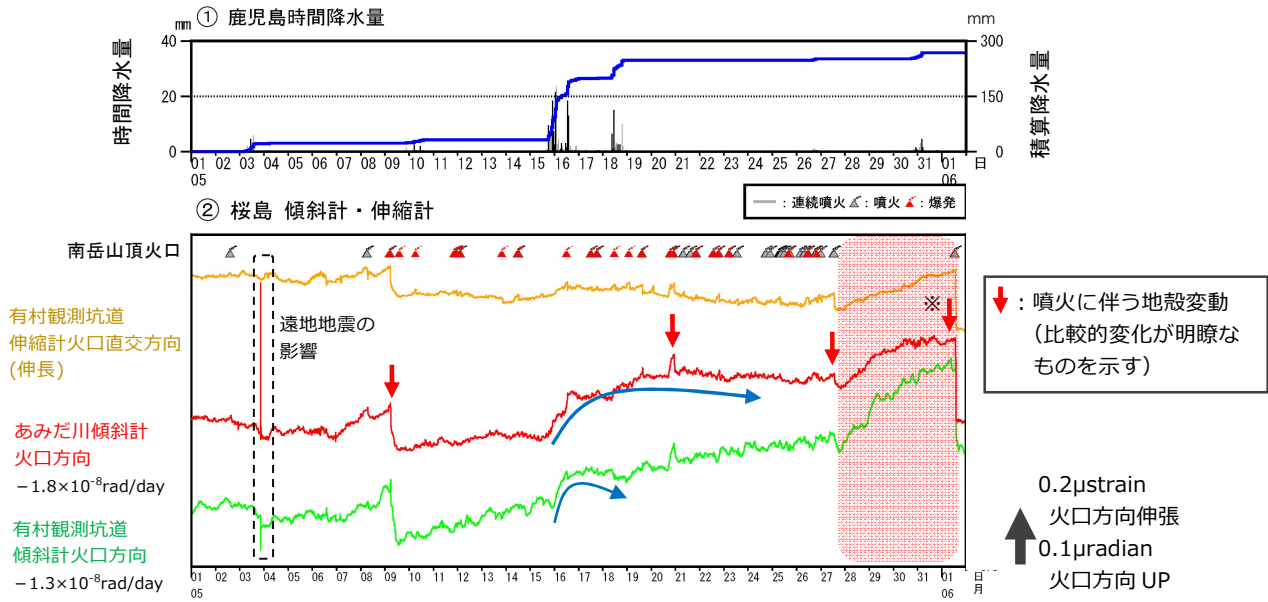
図5 桜島 傾斜計及び伸縮計による地殻変動の状況（2020年5月）
