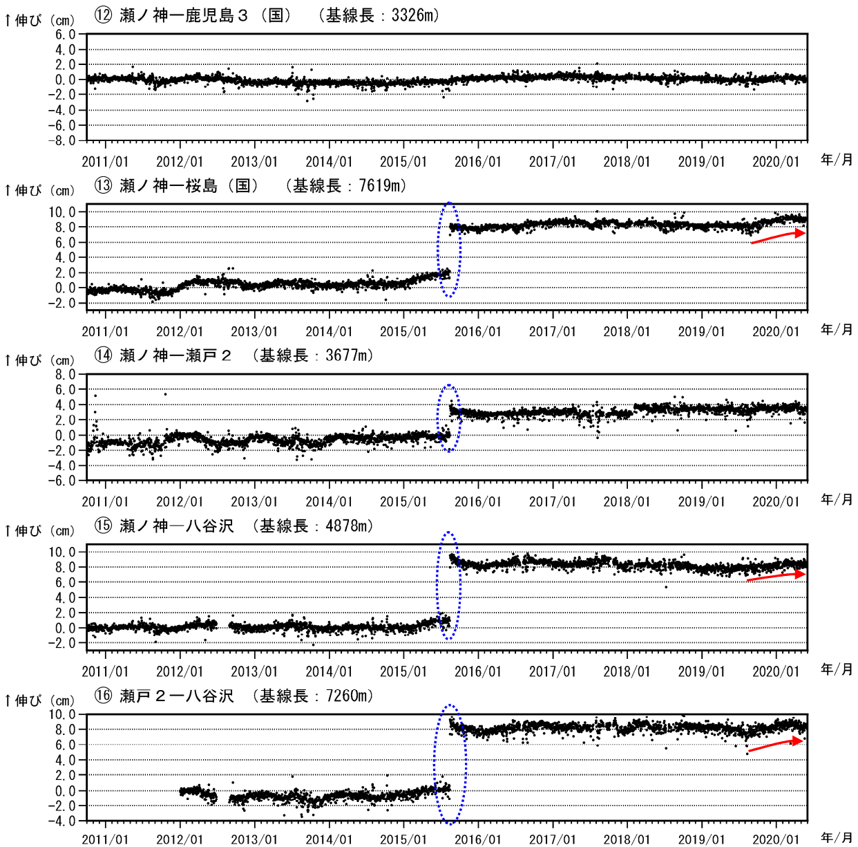
図 6-3 桜島 GNSS 連続観測による基線長変化（2010 年 10 月～2020 年 5 月）
