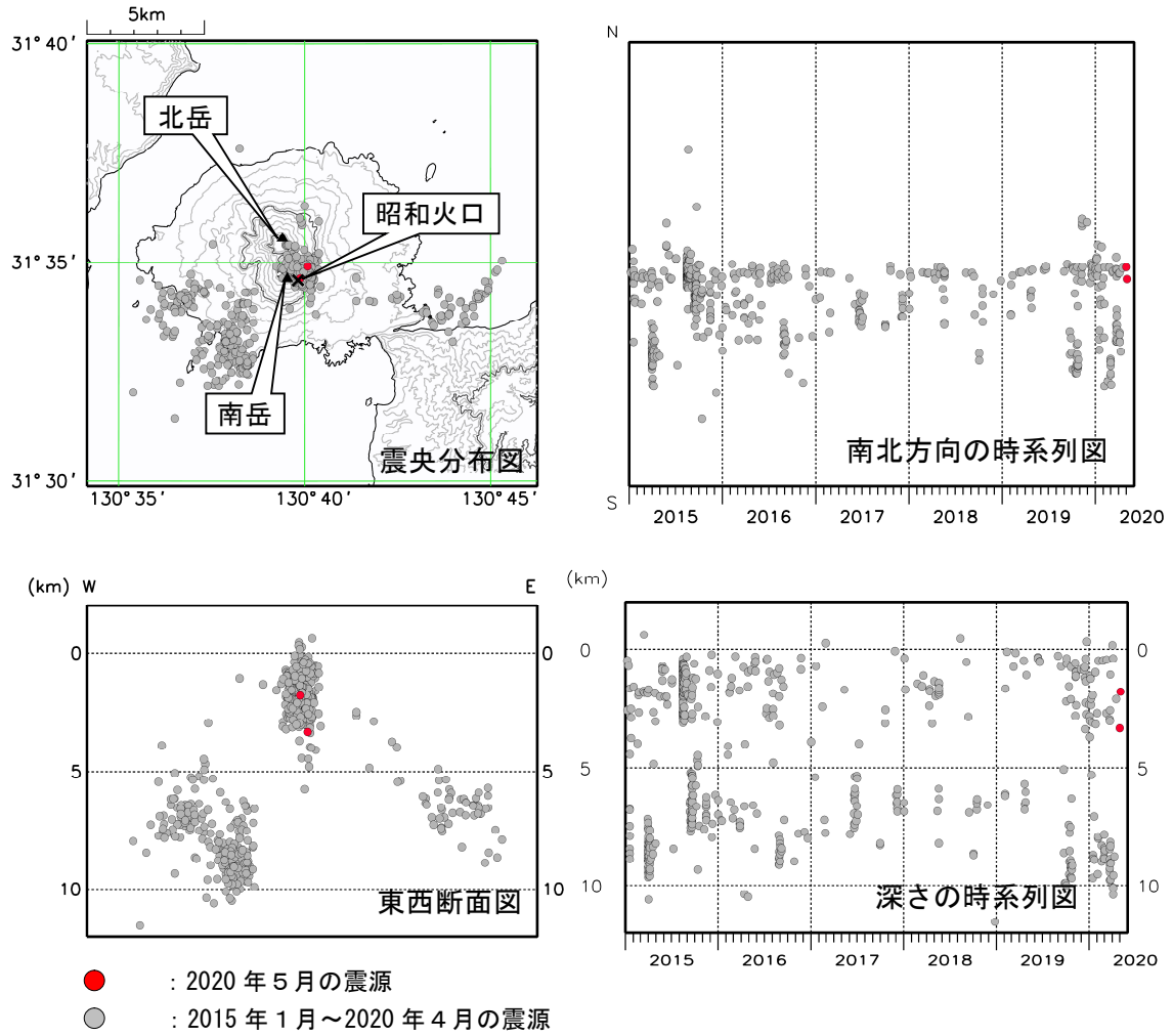
図2 桜島 震源分布図（2015年1月～2020年5月）
