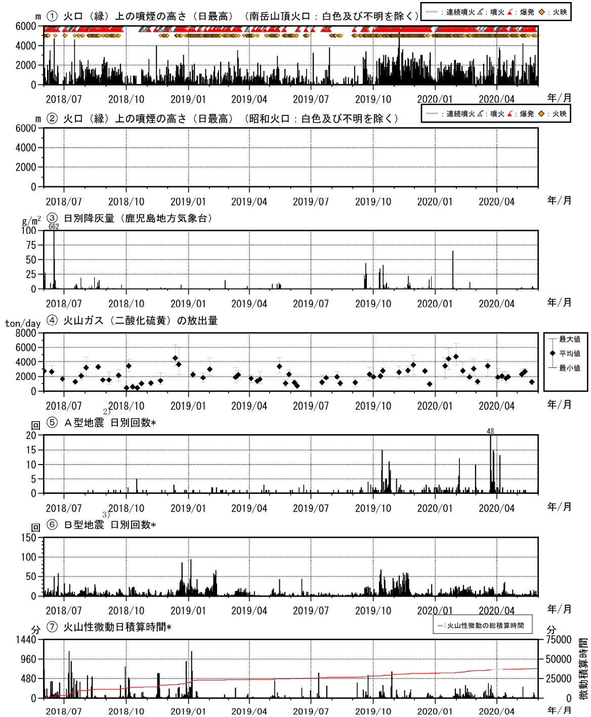
図4 桜島 最近2年間の活動経過図（2018年6月～2020年5月）
