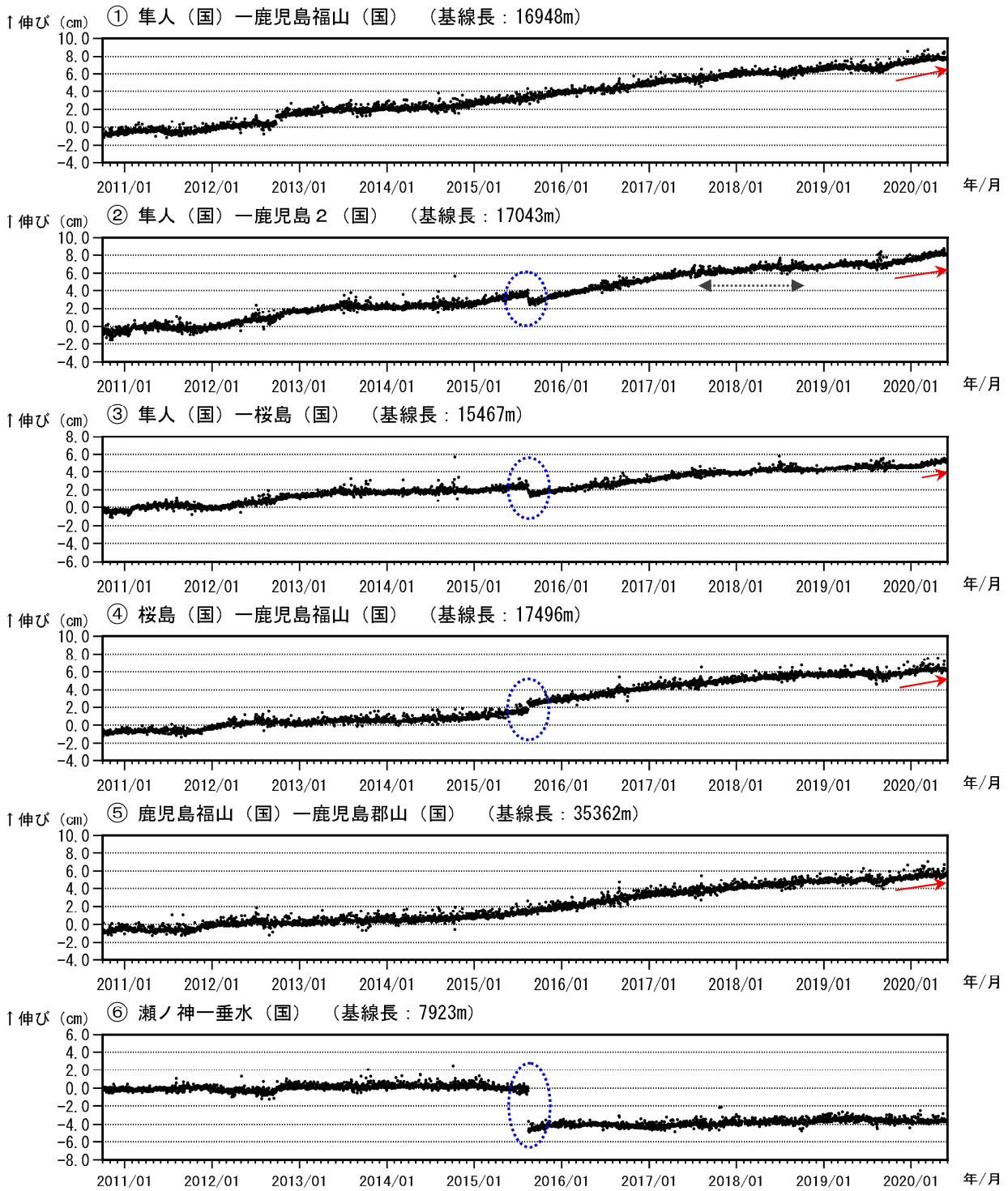
図 6-1 桜島 GNSS 連続観測による基線長変化（2010 年 10 月～2020 年 5 月）
