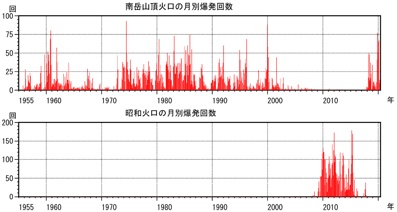
図 3-1 桜島 南岳山頂火口（上図）と昭和火口（下図）の月別爆発回数 （1955年1月～2020年5月）
