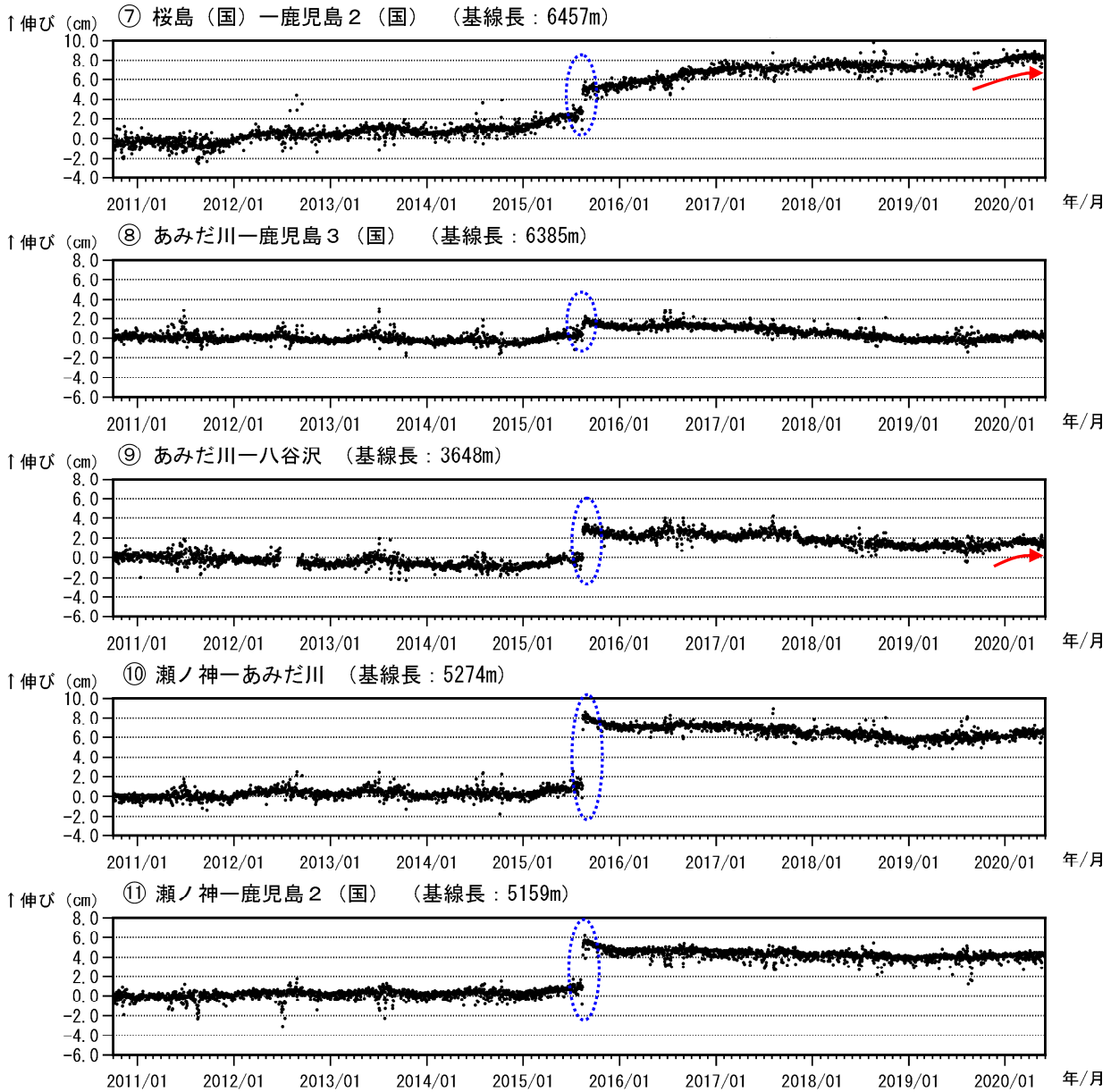
図 6-2 桜島 GNSS 連続観測による基線長変化（2010 年 10 月～2020 年 5 月）
