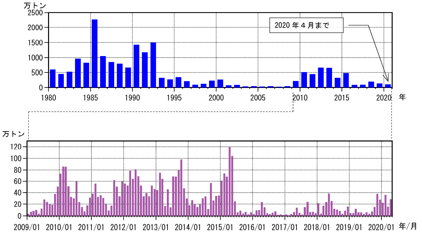
図8 桜島 鹿児島県が実施している降灰の観測データから推定した火山灰の総噴出量 (上段：1980年1月～2020年4月の年別値、下段：2009年1月～2020年4月の月別値)
