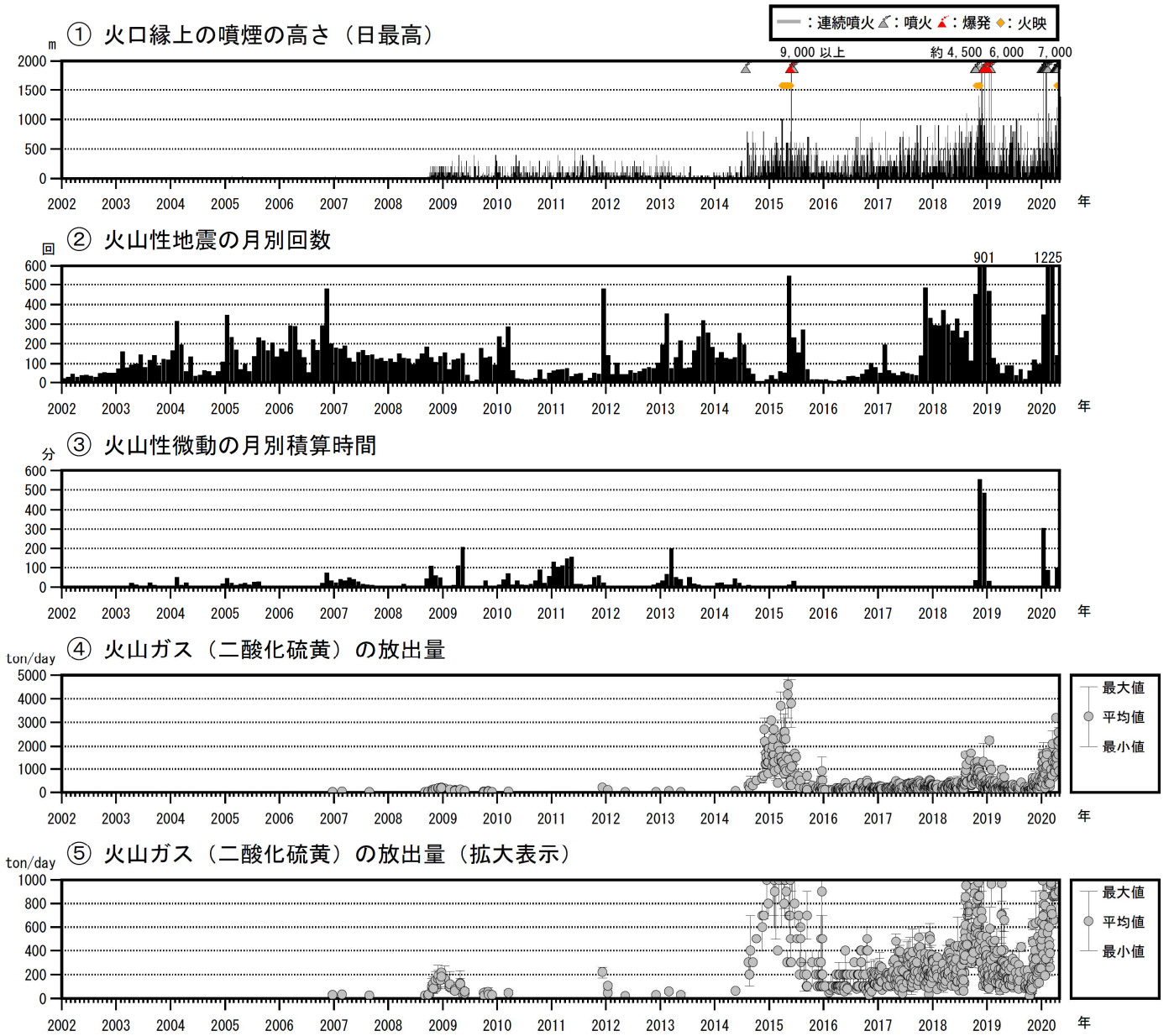
図6 口永良部島 火山活動経過図（2002年1月～2020年4月）
