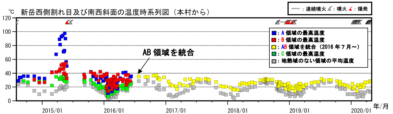
図4 口永良部島 新岳西斜面及び新岳南西側斜面の地熱域の温度時系列（2014年8月～2020年4月）
