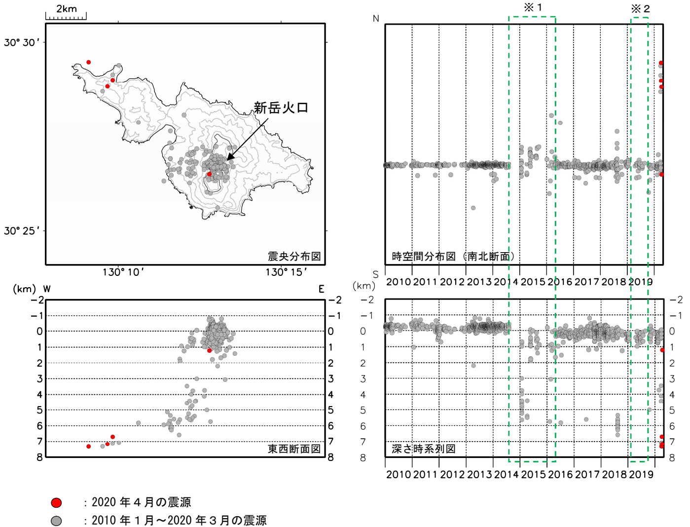
図8 口永良部島 震源分布図（2010年1月～2020年4月）
