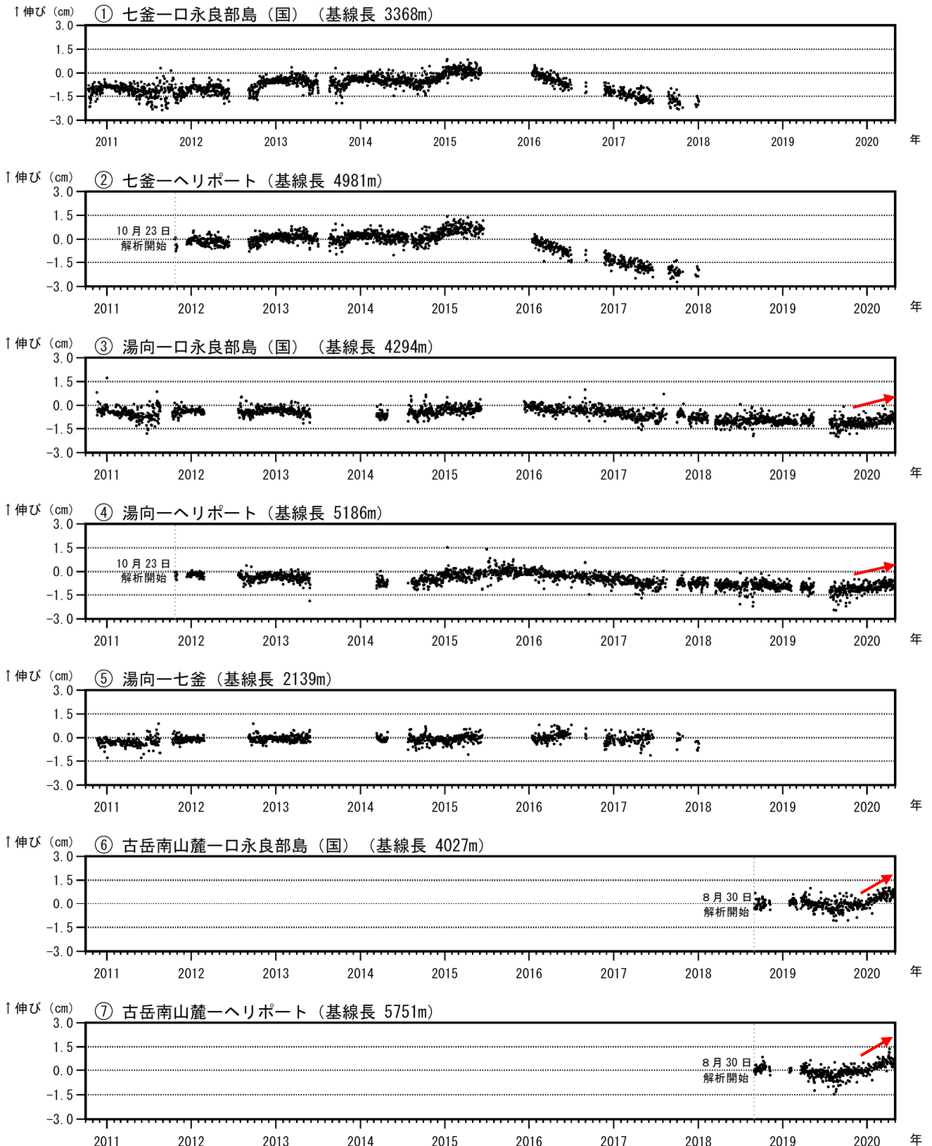
図9 口永良部島 GNSS 連続観測による基線長変化（2010年10月～2020年4月）
