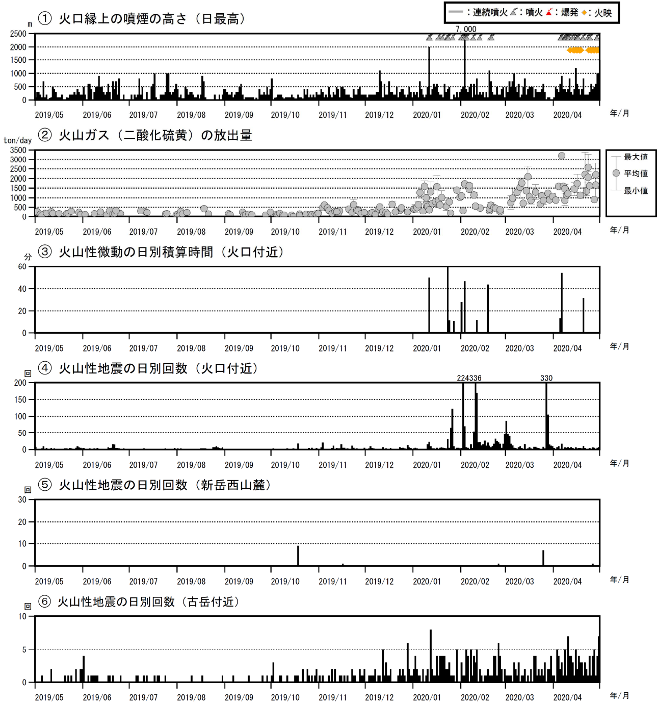
図7 口永良部島 最近の火山活動経過図（2019年5月～2020年4月）
