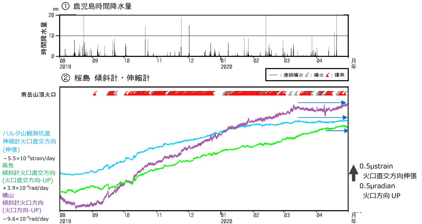
図 5-1 桜島 傾斜計及び伸縮計による地殻変動の状況（2019年8月～2020年4月）
