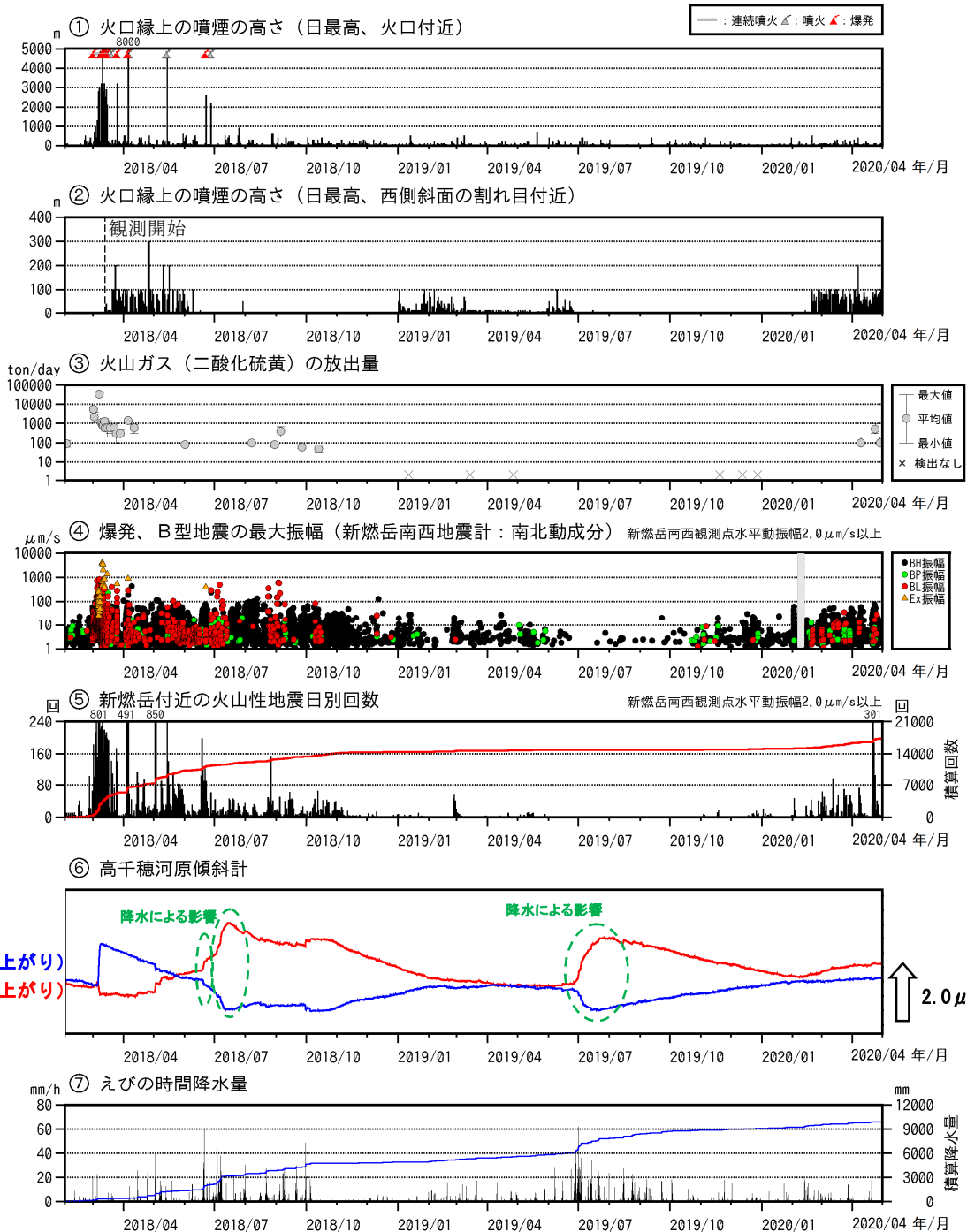
図5 霧島山（新燃岳） 火山活動経過図（2018年2月～2020年4月）
