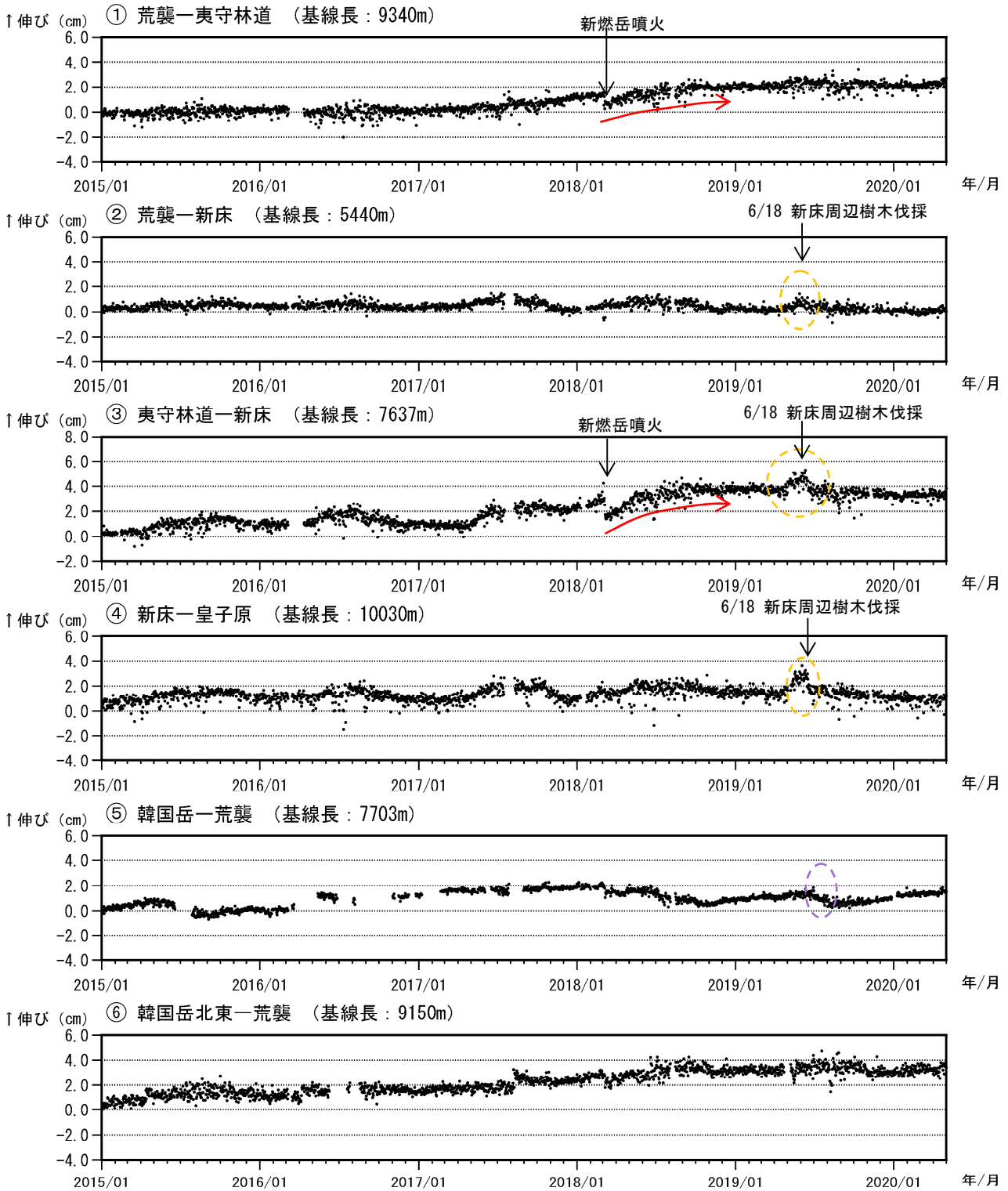
図 7-1 霧島山（新燃岳） GNSS 連続観測による基線長変化（2015 年 1 月～2020 年 4 月）
