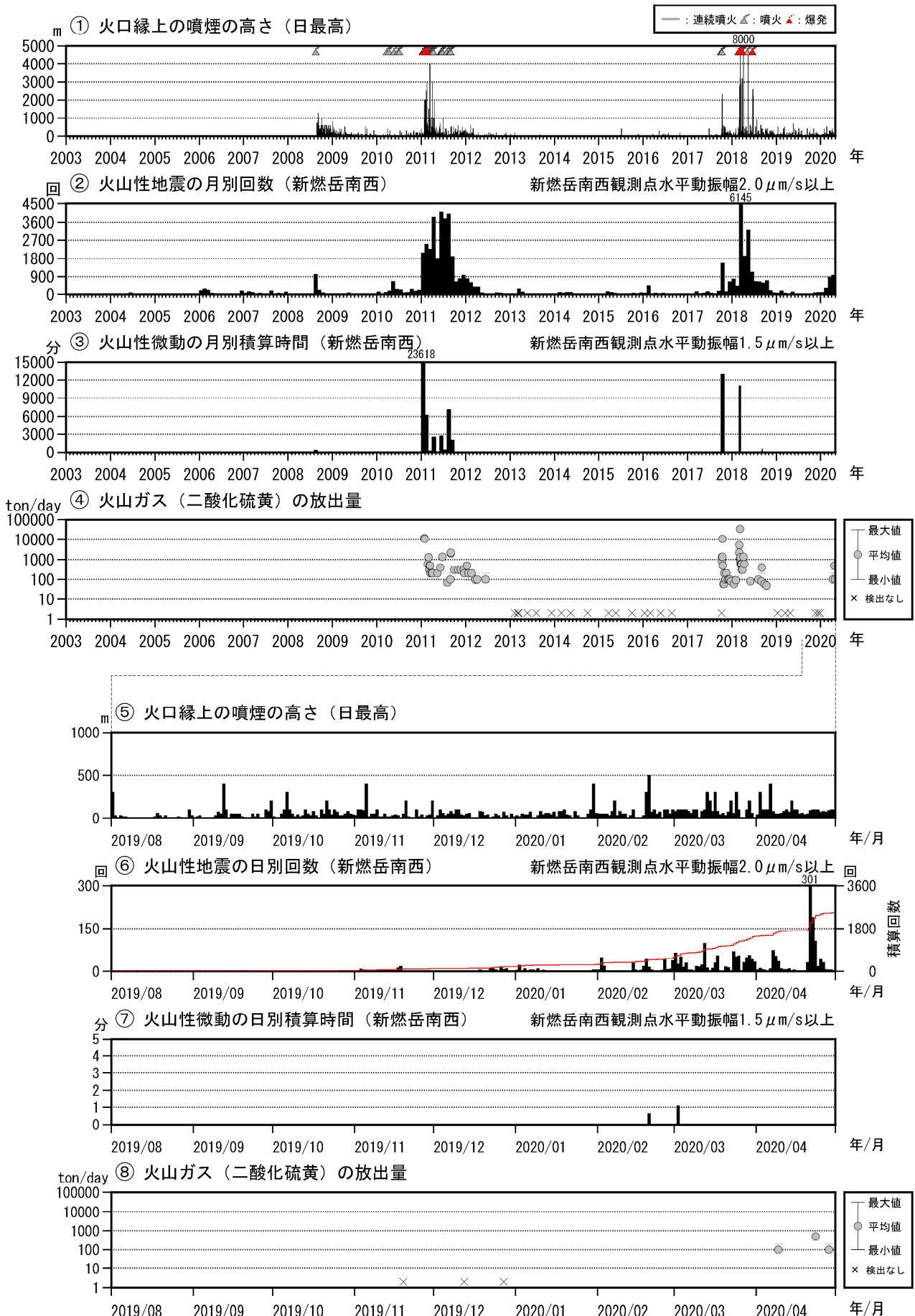
図4 霧島山（新燃岳）火山活動経過図（2003年1月～2020年4月）
