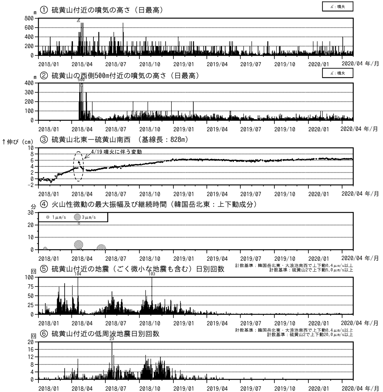
図5 霧島山（えびの高原（硫黄山）周辺） 火山活動経過図（2018年1月～2020年4月）
