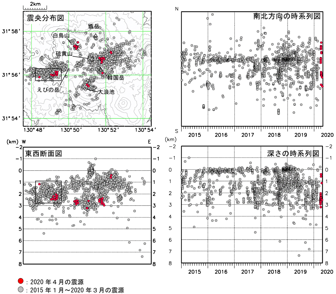
図4 霧島山（えびの高原（硫黄山）周辺） 震源分布図（2015年1月～2020年4月）
