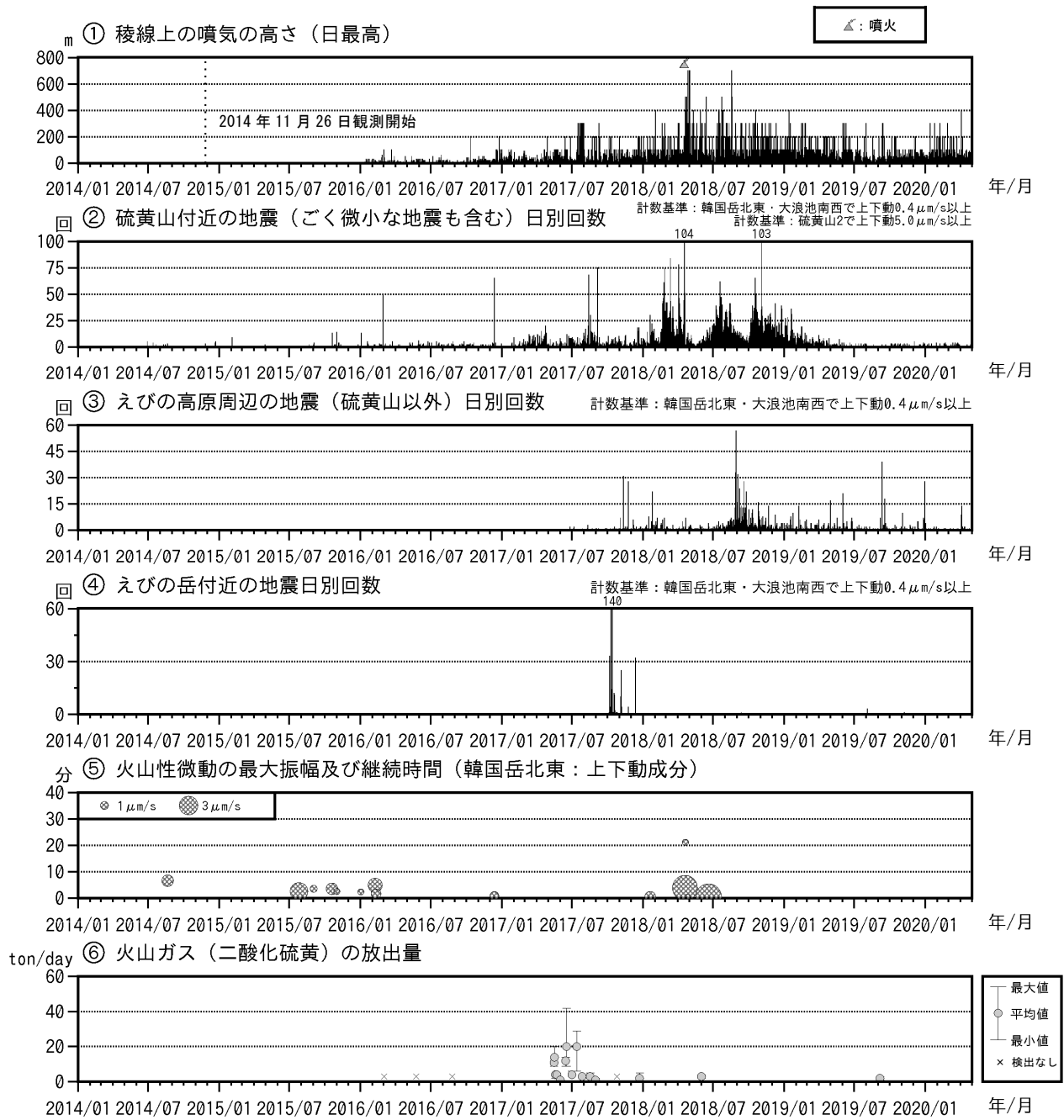
図6 霧島山（えびの高原（硫黄山）周辺） 火山活動経過図（2014年1月～2020年4月）
