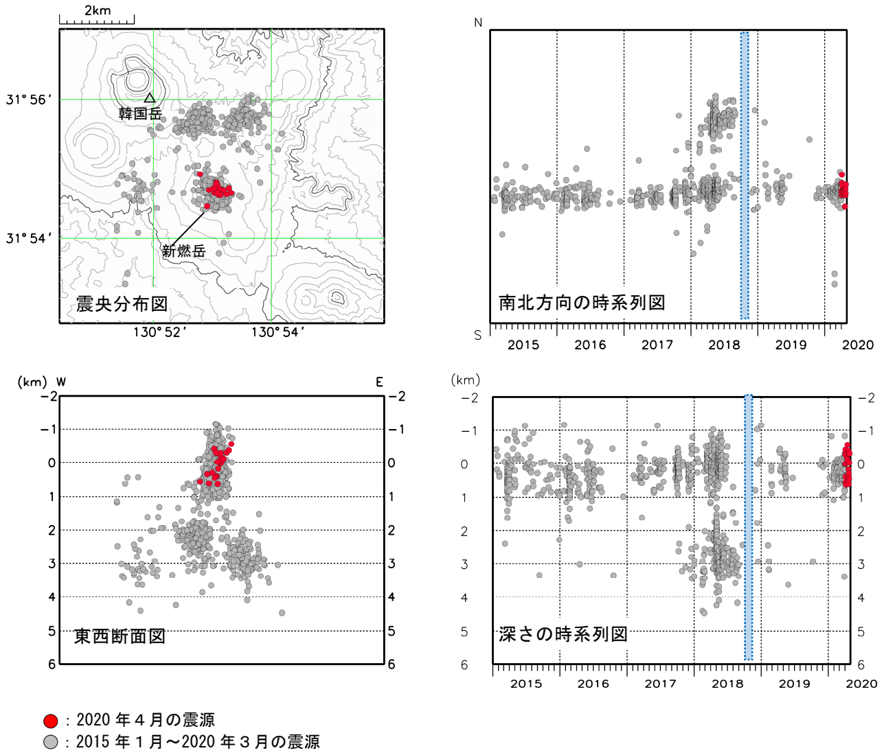
図6 霧島山（新燃岳） 震源分布図（2015年1月～2020年4月）
