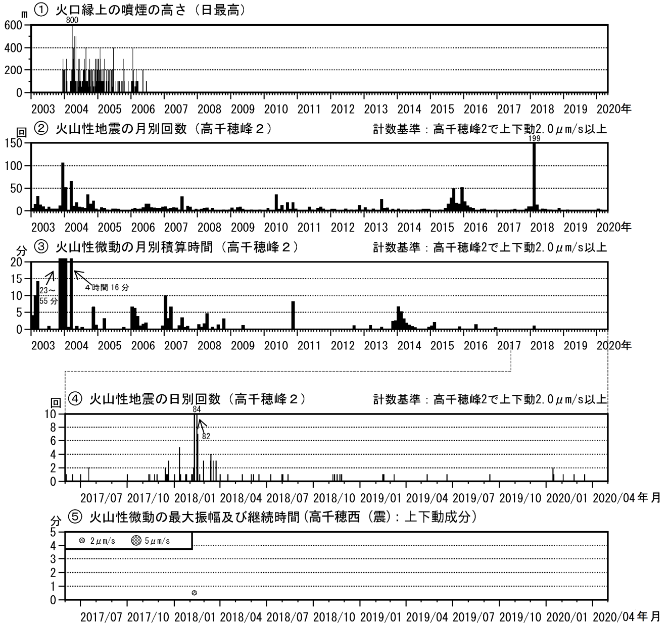
図2 霧島山（御鉢） 火山活動経過図（2003年1月～2020年4月）
