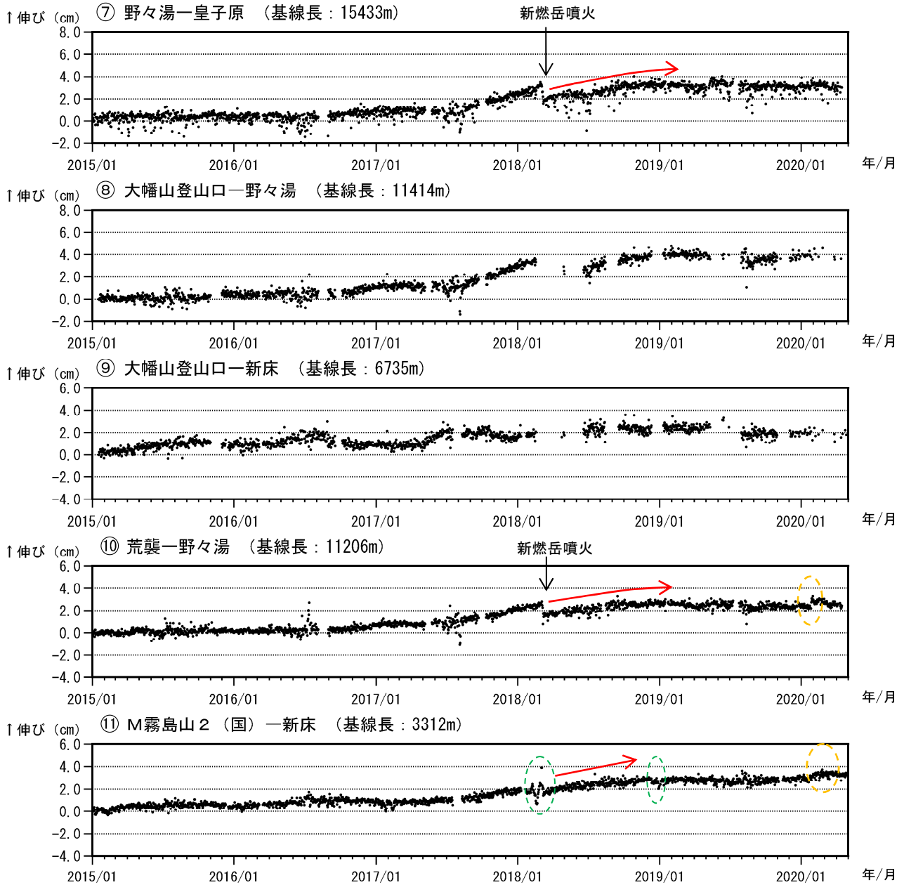
図 7-2 霧島山（新燃岳） GNSS 連続観測による基線長変化（2015 年 1 月～2020 年 4 月）
