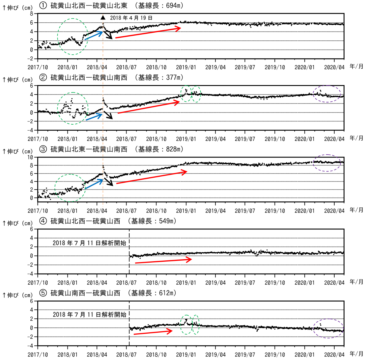
図7 霧島山（えびの高原（硫黄山）周辺） GNSS 連続観測による基線長変化 (2017年10月～2020年4月)
