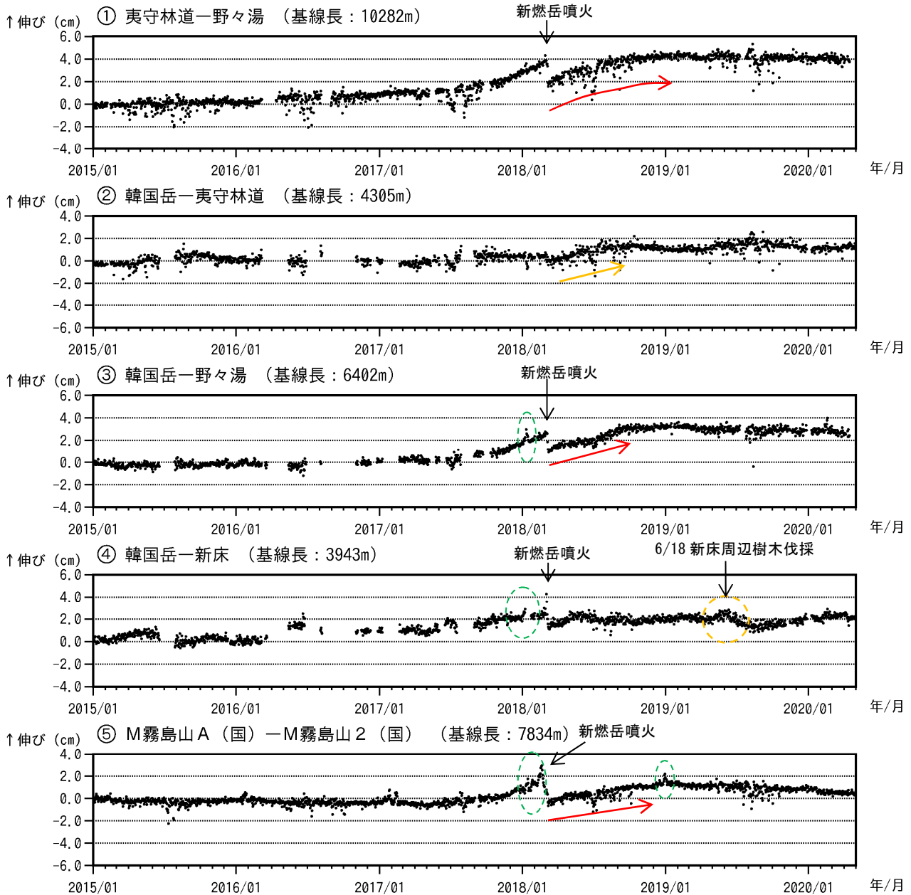
図 8-1 霧島山（えびの高原（硫黄山）周辺） GNSS 連続観測による基線長変化 (2015年1月～2020年4月)
