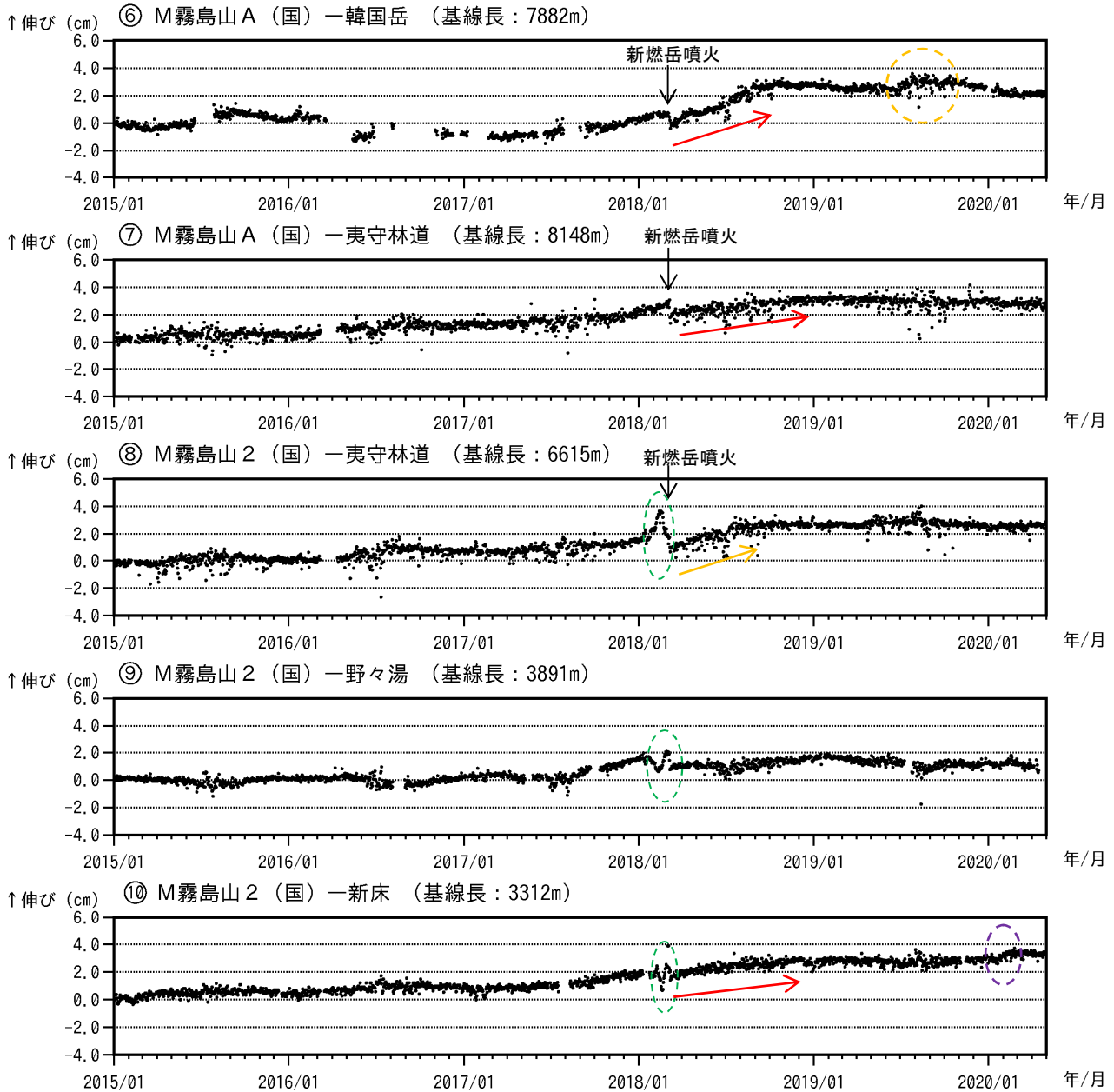
図 8-2 霧島山（えびの高原（硫黄山）周辺） GNSS 連続観測による基線長変化 (2015年1月～2020年4月)
