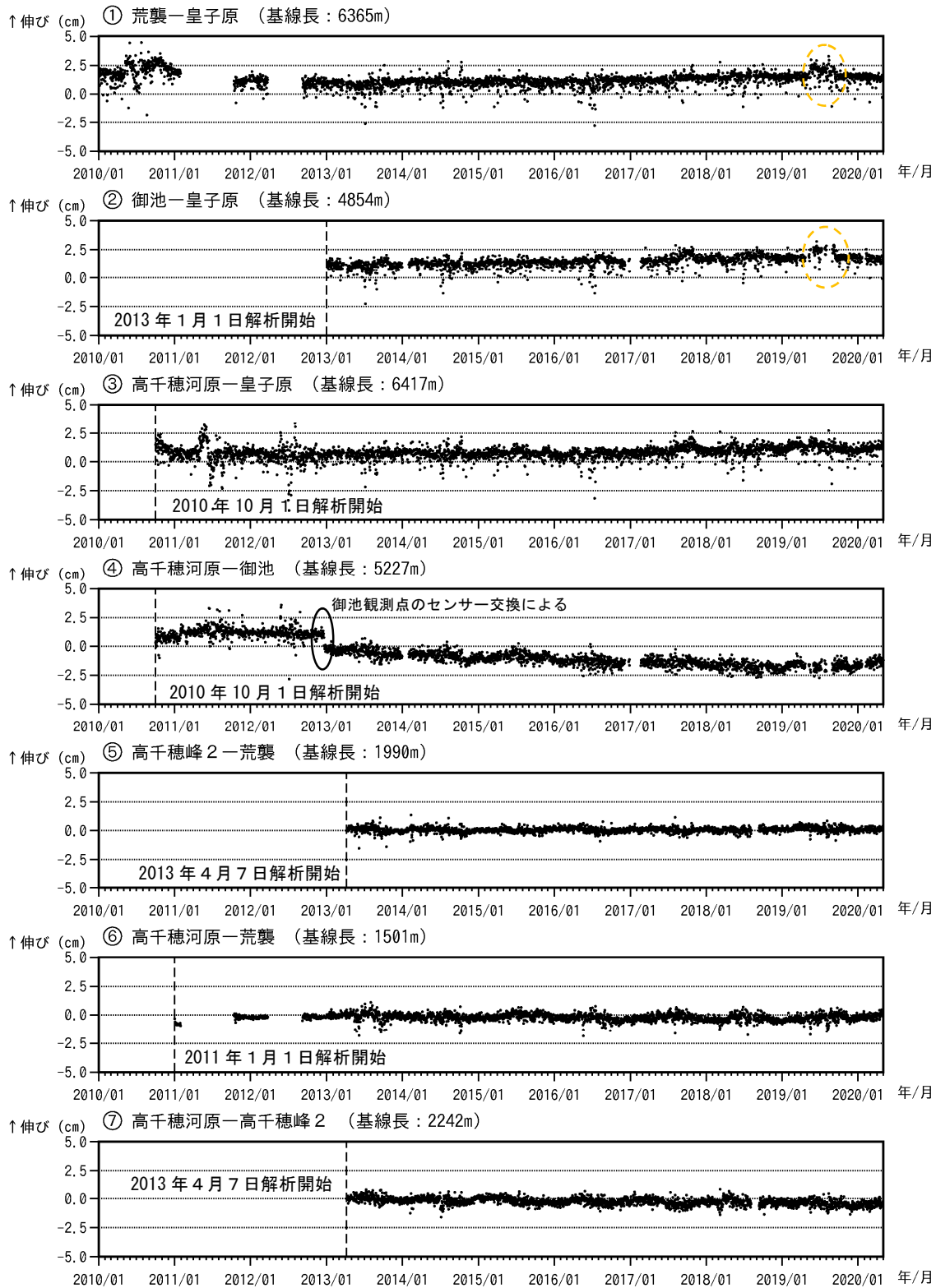
図4 霧島山（御鉢） GNSS連続観測による基線長変化（2010年1月～2020年4月）
