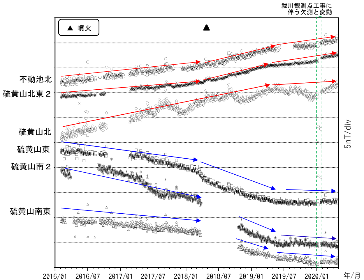
図 12 霧島山（えびの高原（硫黄山）周辺） 全磁力観測点で観測された全磁力変動 （2016年2月～2020年4月）
