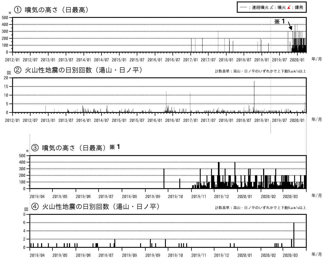
図2 鶴見岳・伽藍岳 火山活動経過図（2012年1月～2020年3月）
