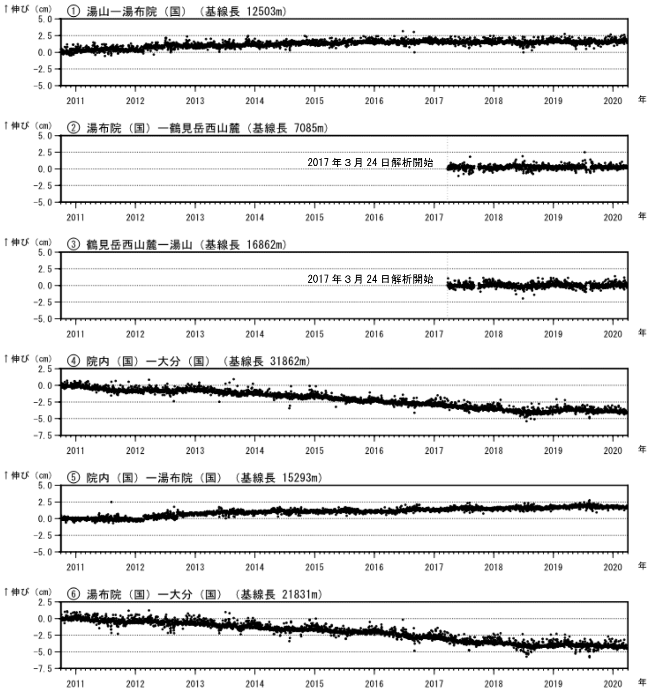
図4 鶴見岳・伽藍岳 GNSS連続観測による基線長変化（2010年10月～2020年3月）
