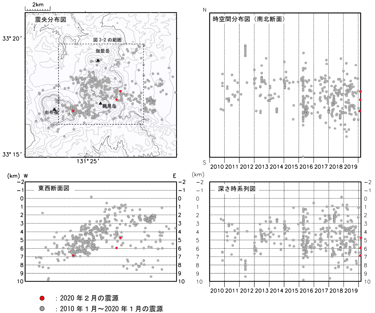
図3-1 鶴見岳・伽藍岳 震源分布図（広域）（2010年1月～2020年2月）
