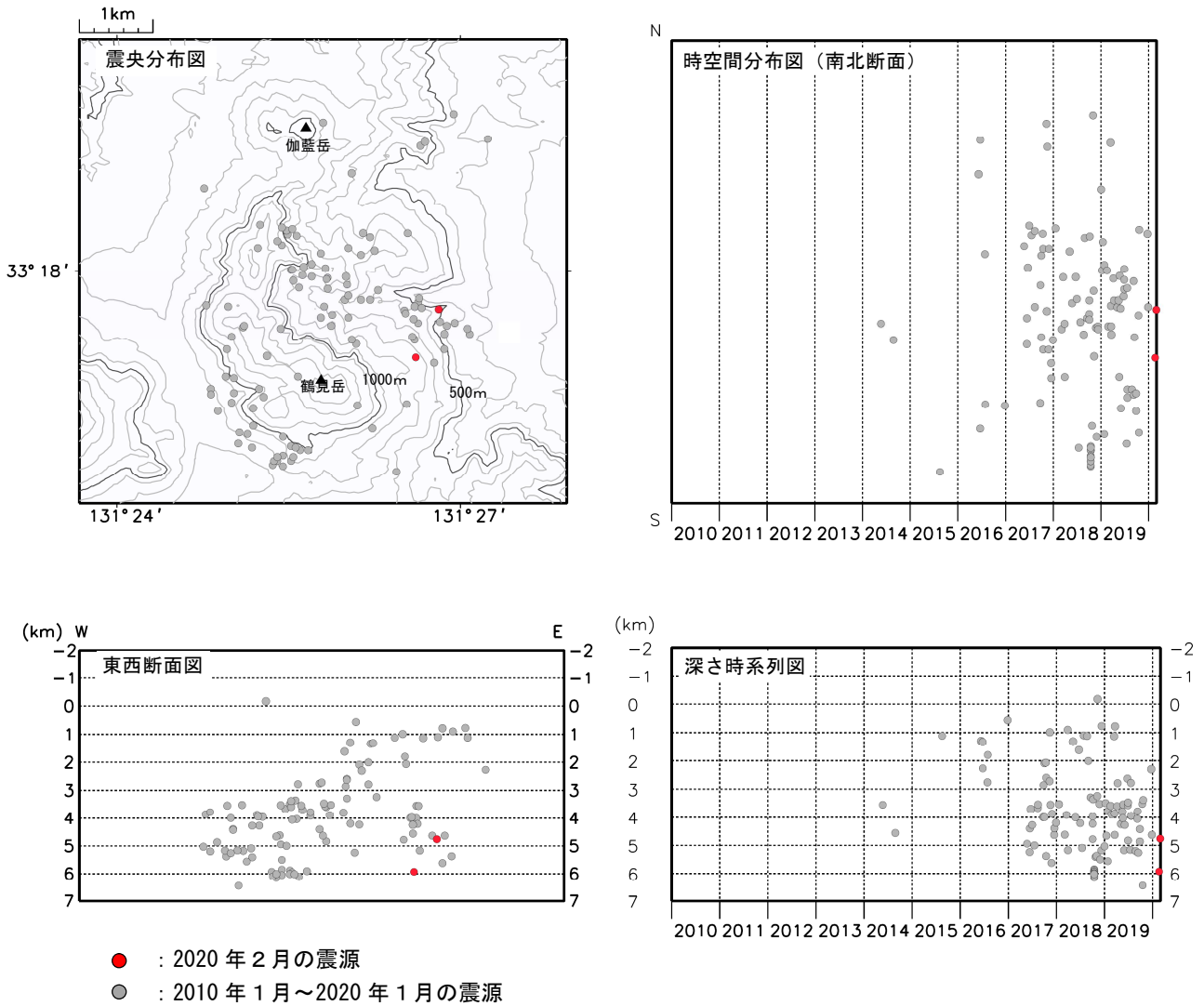
図 3-2 鶴見岳・伽藍岳 震源分布図（鶴見岳・伽藍岳付近の火山性地震） （2010年1月～2020年2月）
