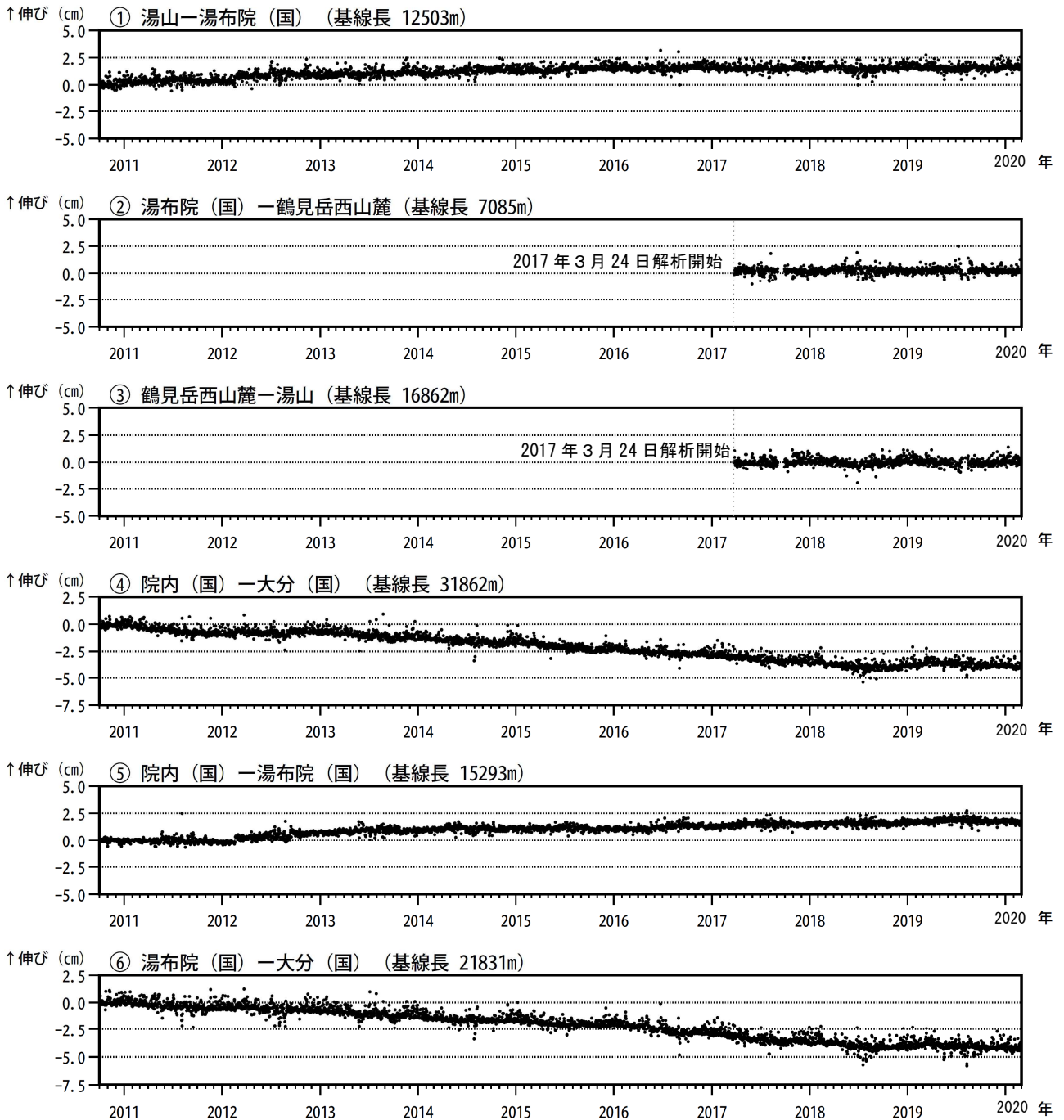
図4 鶴見岳・伽藍岳 GNSS連続観測による基線長変化（2010年10月～2020年2月）
