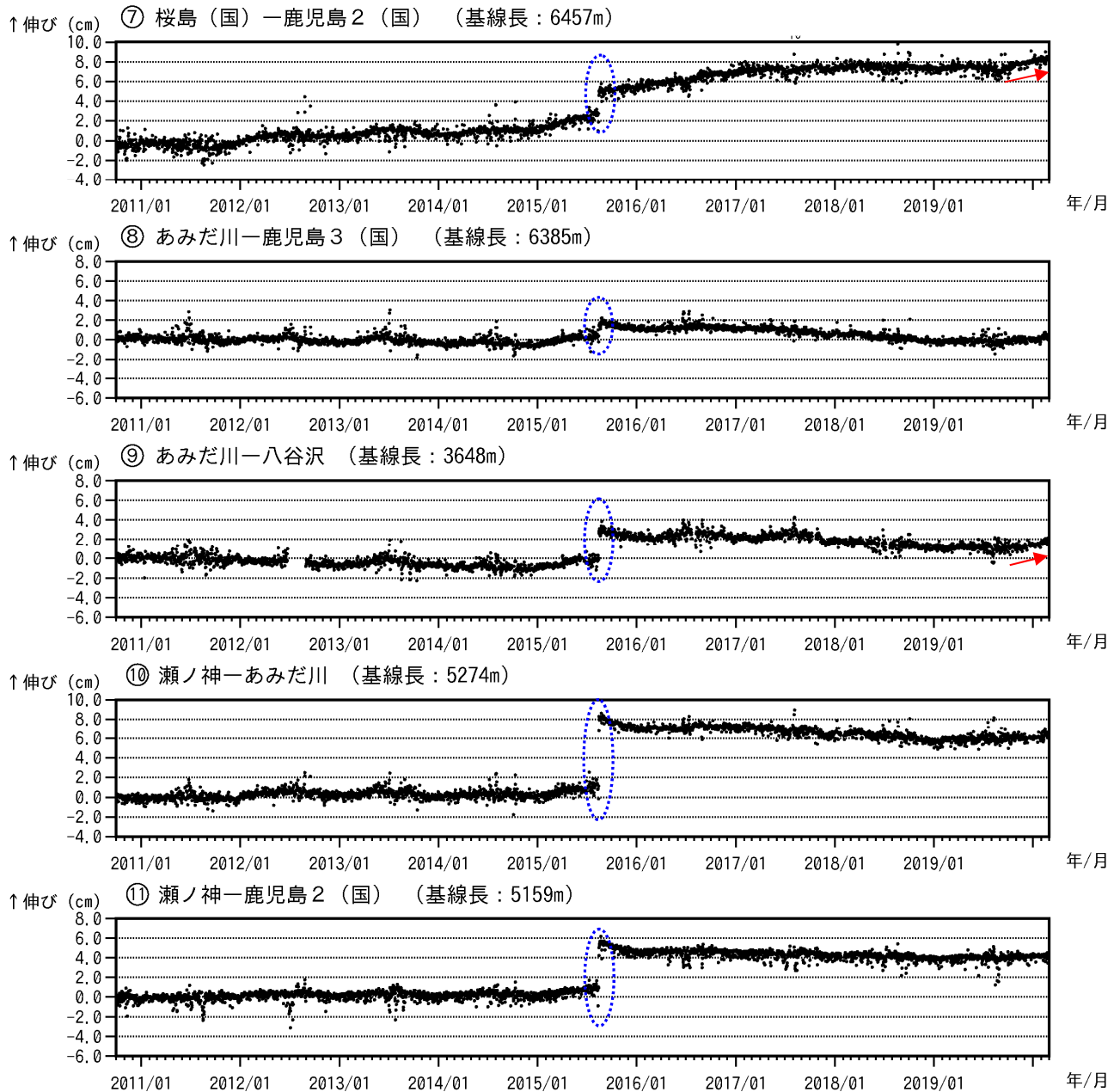
図 8-2 桜島 GNSS 連続観測による基線長変化（2010 年 10 月～2020 年 2 月）
