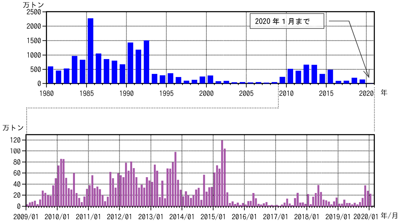
図10 桜島 鹿児島県が実施している降灰の観測データから推定した火山灰の総噴出量 (上段：1980年1月～2020年1月の年別値、下段：2009年1月～2020年1月の月別値)
