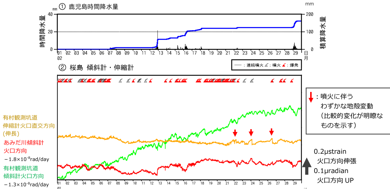
図 7-2 桜島 傾斜計及び伸縮計による地殻変動の状況（2020年2月）
