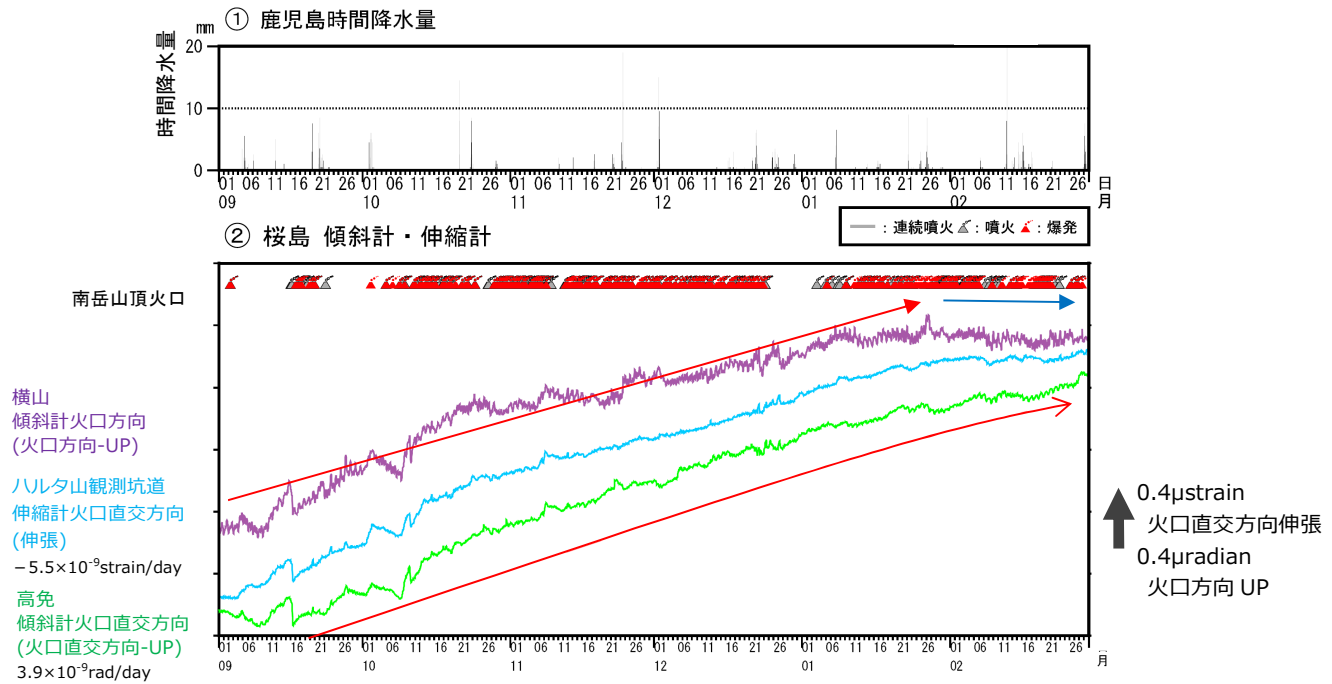
図 7-1 桜島 傾斜計及び伸縮計による地殻変動の状況（2019年9月～2020年2月）
