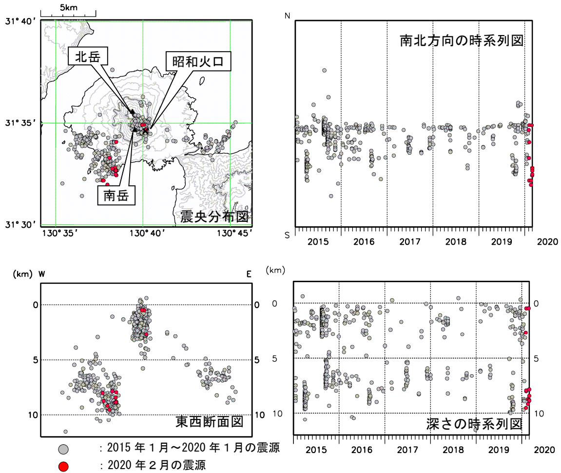
図4 桜島 震源分布図（2015年1月～2020年2月）
