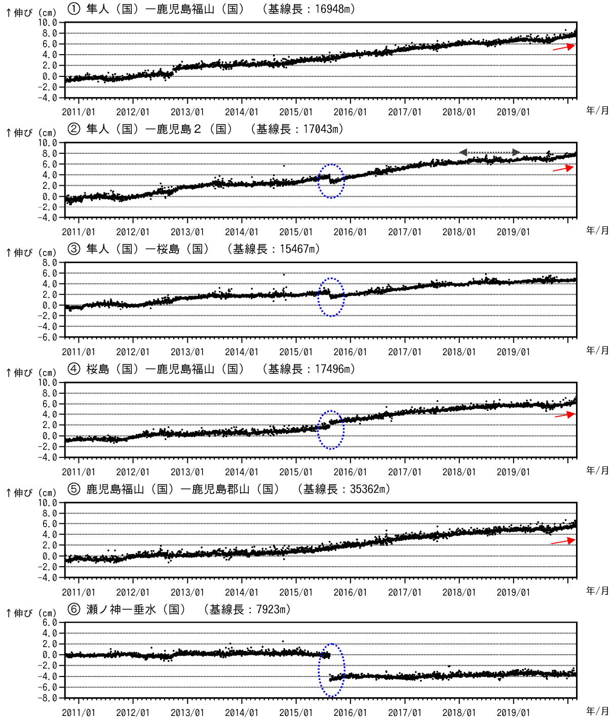
図 8-1 桜島 GNSS 連続観測による基線長変化（2010 年 10 月～2020 年 2 月）
