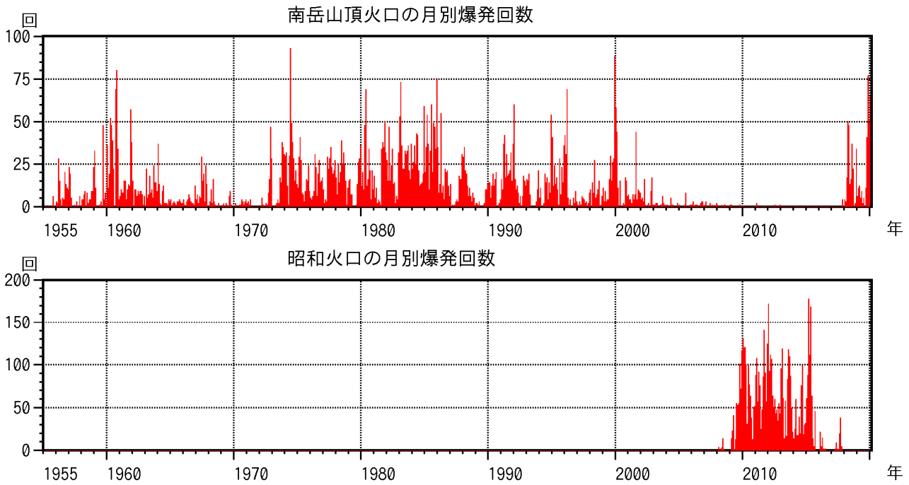
図 5-1 桜島 南岳山頂火口（上図）と昭和火口（下図）の月別爆発回数 （1955年1月～2020年2月）
