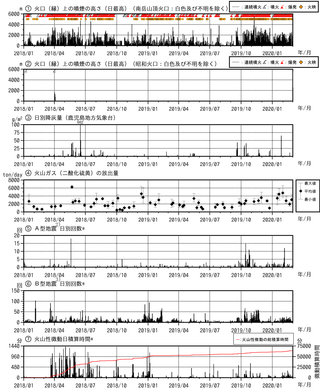
図6 桜島 最近2年間の活動経過図（2018年1月～2020年2月）
