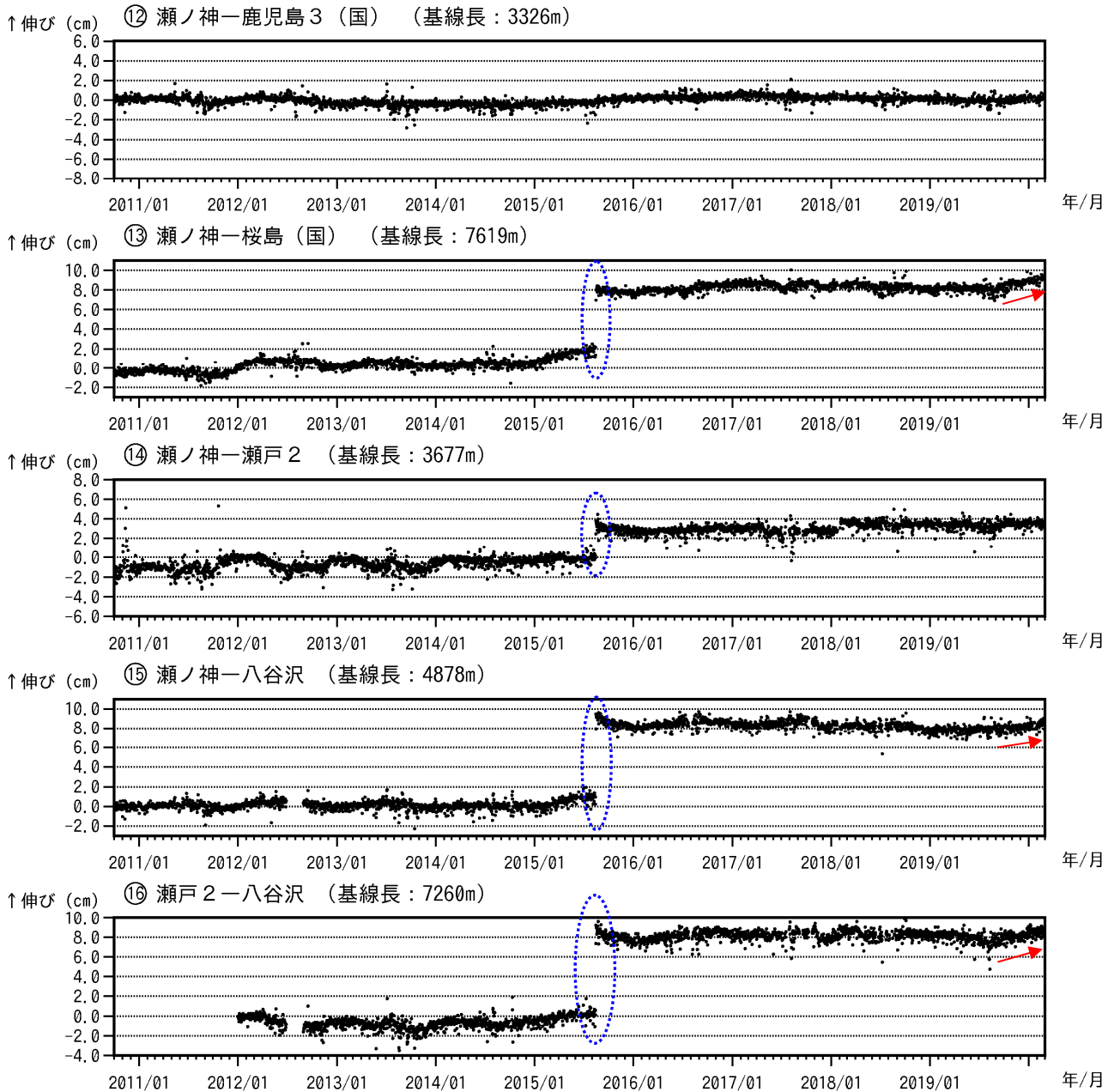
図 8-3 桜島 GNSS 連続観測による基線長変化（2010 年 10 月～2020 年 2 月）
